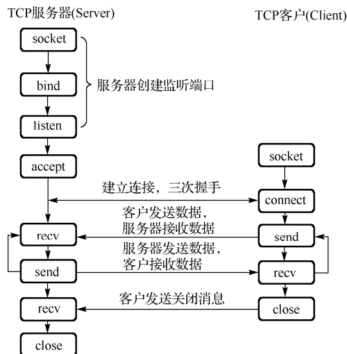
图 13-1 基于 TCP 的服务器和客户程序的双方通信过程
