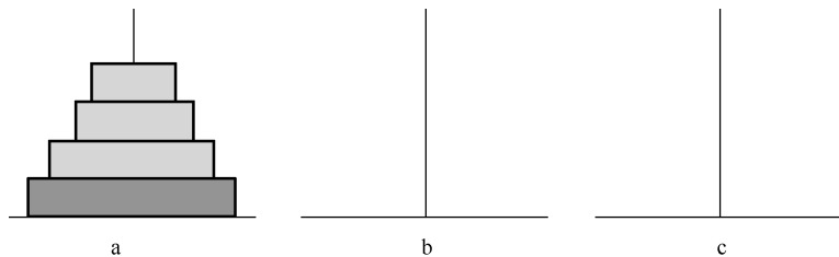
图3-2 汉诺塔问题
