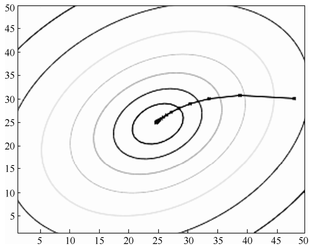
图 3-11 更新过程
