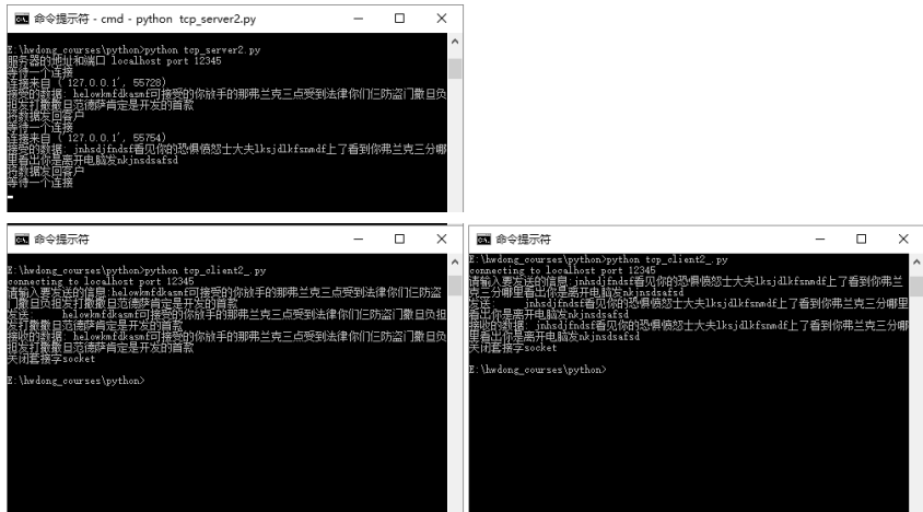
图 13-2 多连接 TCP 服务器程序和客户程序
