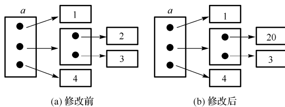
图 2-2 修改 a[1] 引用的 list 对象
