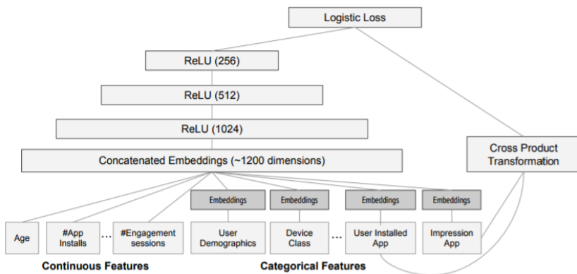
图5.4 WnD模型 (2)
