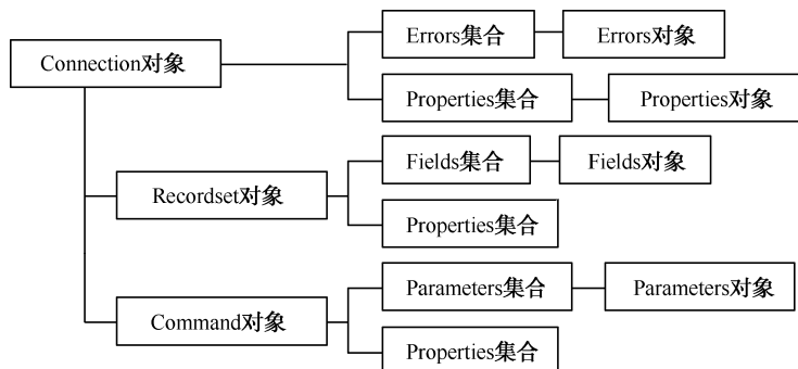
图 13-5 ADO 对象模型
