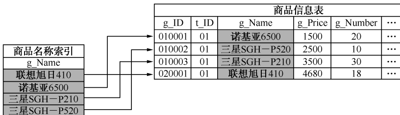
图 7-1 商品名称索引和商品信息表的关系
