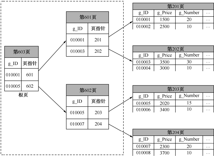
图 7-4 聚集索引查找顺序
