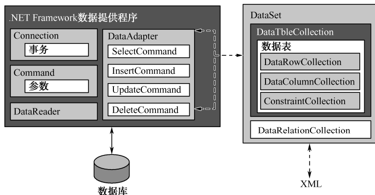
图 13-23 ADO.NET 体系结构
