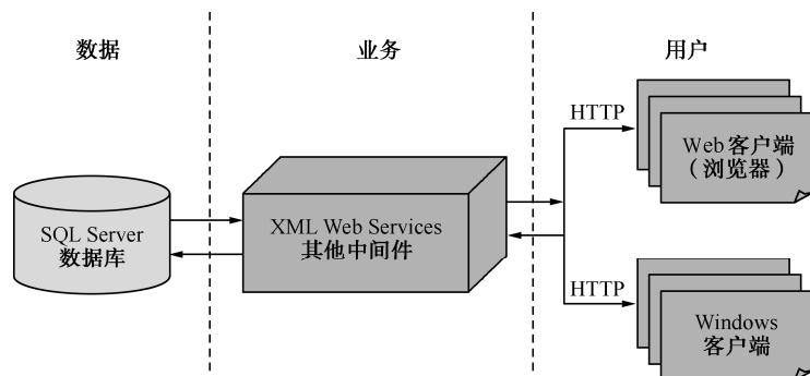
图 13-1 典型 SQL Server 数据库应用系统
