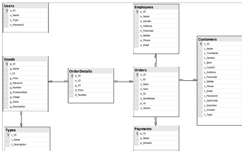
图 5-33 WebShop 数据库关系图
