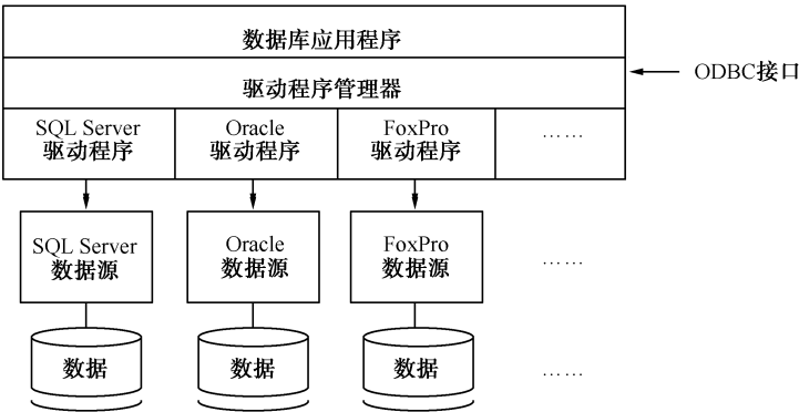
图 13-6 ODBC 体系结构
