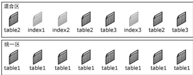
图 3-9 混合区和统一区
