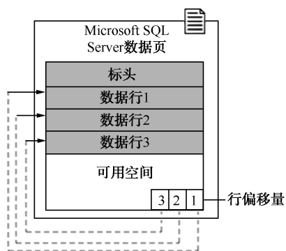
图 3-8 数据文件页结构
