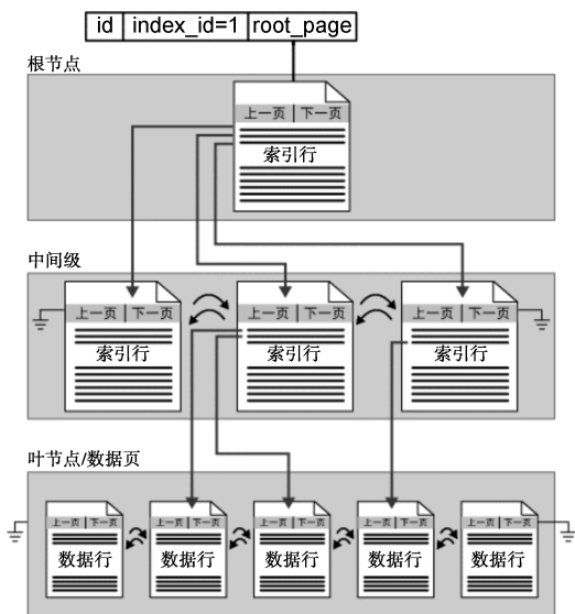
图 7-3 单个分区中的聚集索引结构
