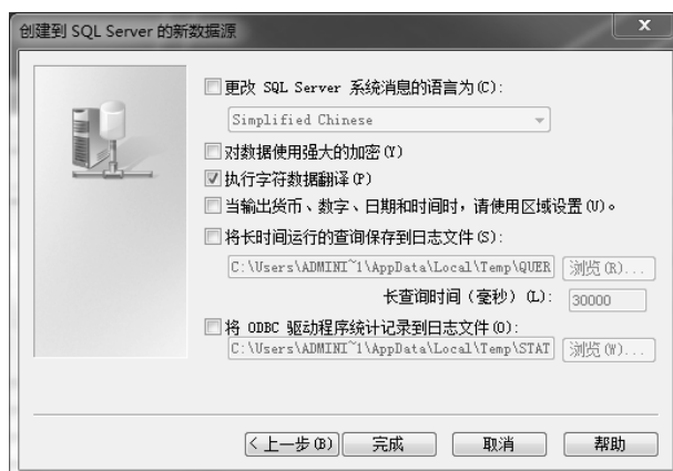
图 13-13 其他设置
