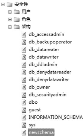
图 11-41 新建架构
