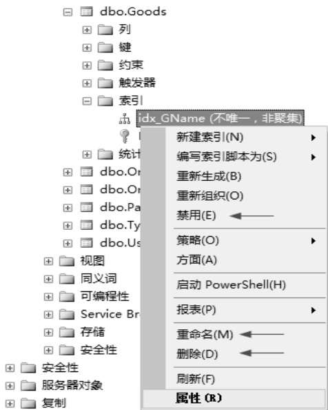
图 7-9 具体操作
