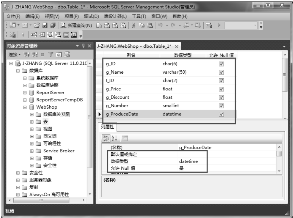
图 4-4 新建表
