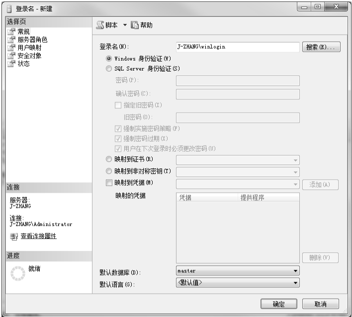
图 11-8 新建登录名
