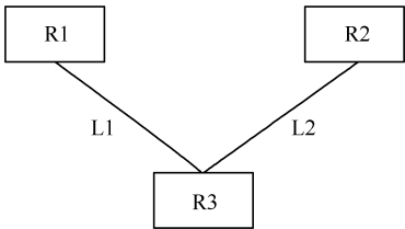
图 2-4 联系命名
