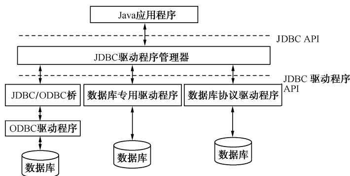
图 13-7 JDBC 工作原理
