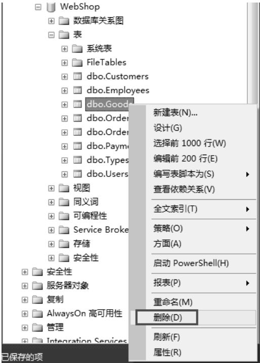
图 4-13 “删除”表
