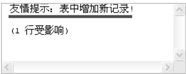
图 9-7 验证触发器
