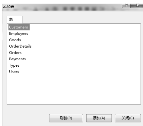
图 5-32 选择表
