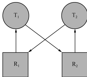
图 10-11 死锁状态
