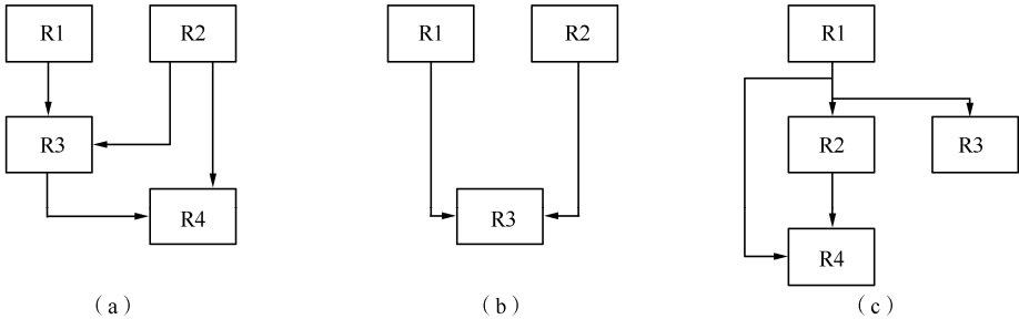
图 2-3 网状模型
