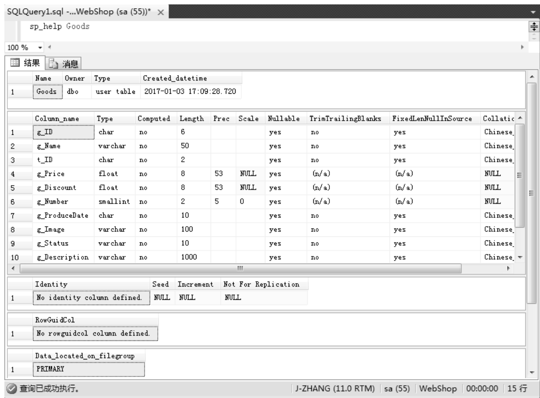
图 4-17 查看表信息
