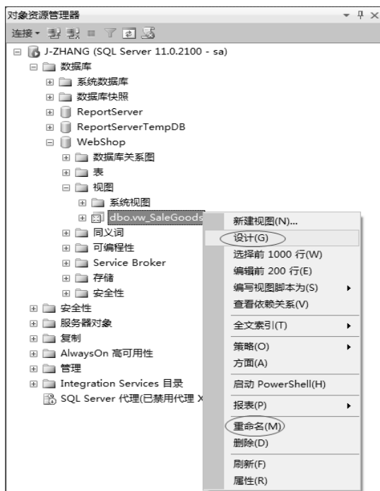
图 6-10 选择修改
