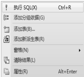
图 6-6 执行 SQL
