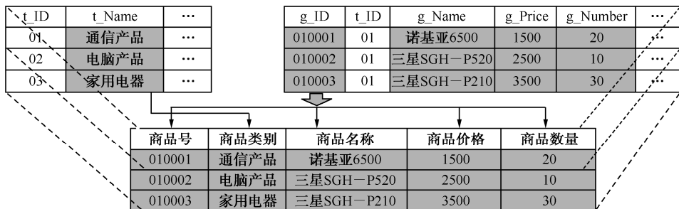
图 6-1 典型视图
