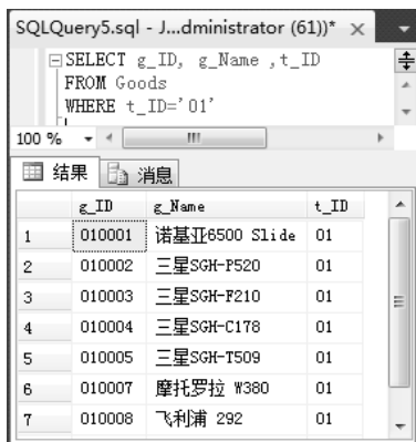
图 5-42 子查询
