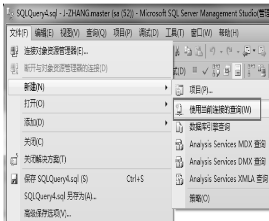
图 3-23 新建查询
