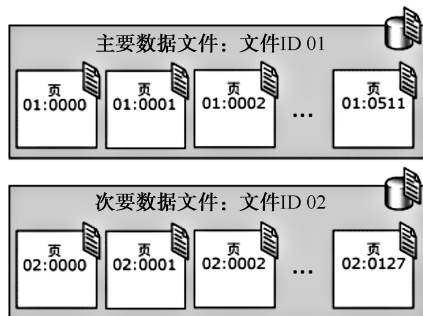
图 3-7 数据文件页
