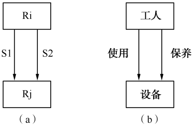
图 2-5 复合链
