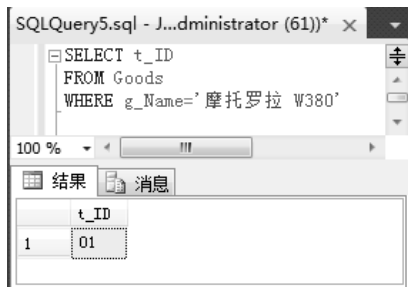
图 5-41 父查询
