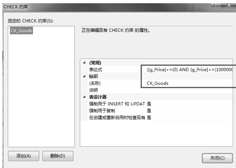
图 4-25 添加约束
