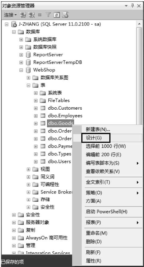
图 4-10 选择修改表
