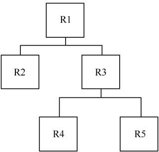
图 2-2 层次模型
