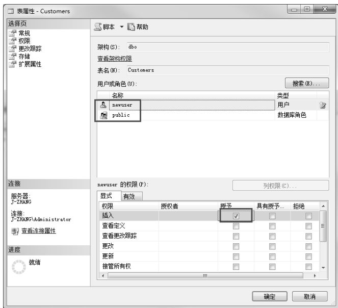
图 11-33 “权限”选项卡
