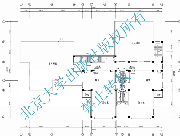
三层给排水水平面图 1:100
