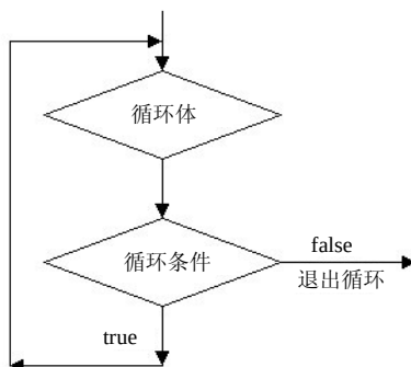
图4.6 while语句流程图
