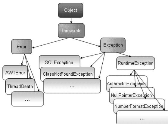
图14.1 异常类的继承结构
