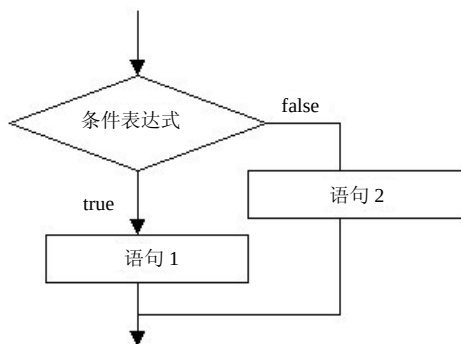
图4.2 if-else语句流程图
