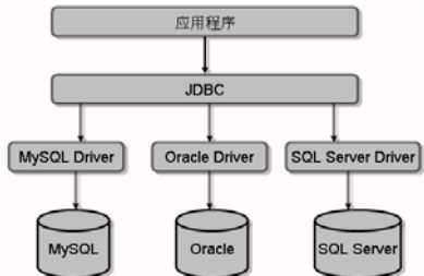
图18.2 JDBC工作模式
