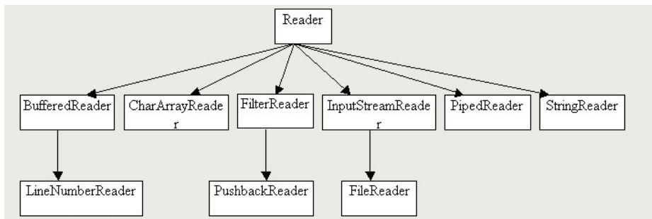
图15.7 Reader的体系结构
