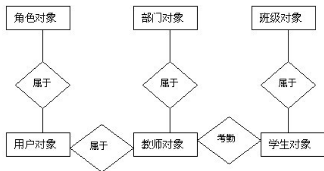
图22.10 实体之间的关系E-R图
