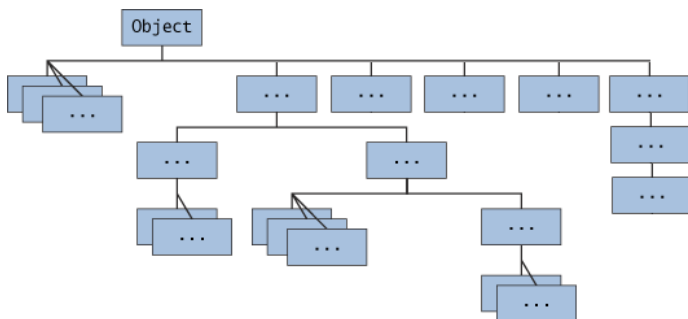
图7.1 Java平台中所有的类都继承自Object
