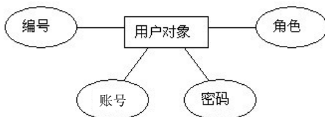
图22.9 用户对象实体E-R图
