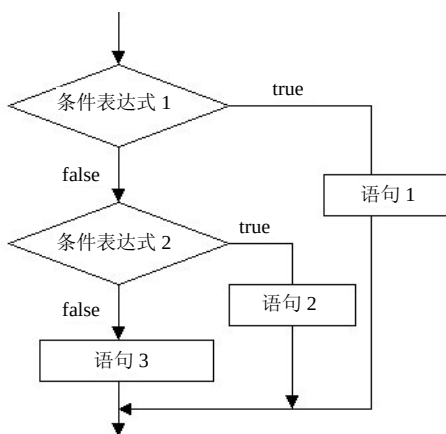
图4.3 if-else-if语句流程图
