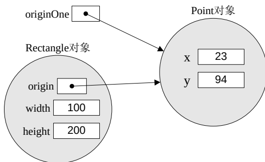
图6.3 两个引用指向同一个对象
