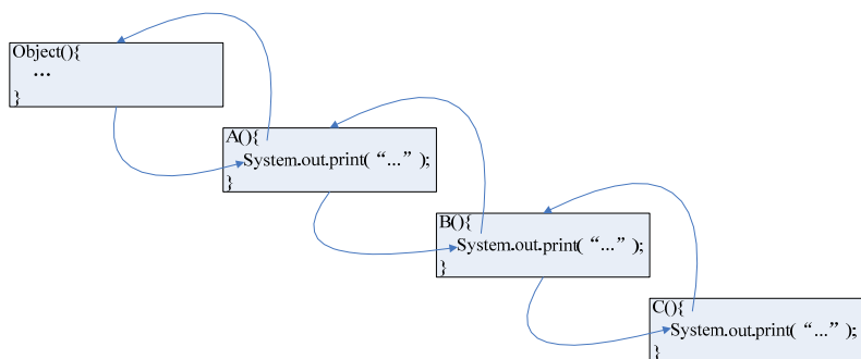
图7.2 Java中的构造方法链
