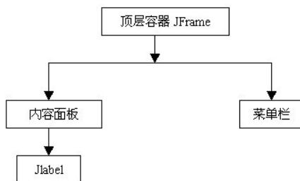
图10.4 容器层级
