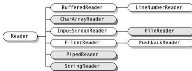
图15.3 Reader继承图
