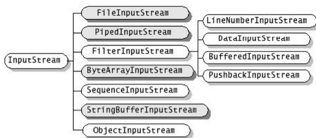
图15.1 InputStream继承图
