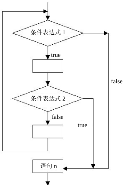
图4.8 使用break语句的流程图
