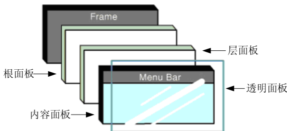
图10.5 根面板组件列表
