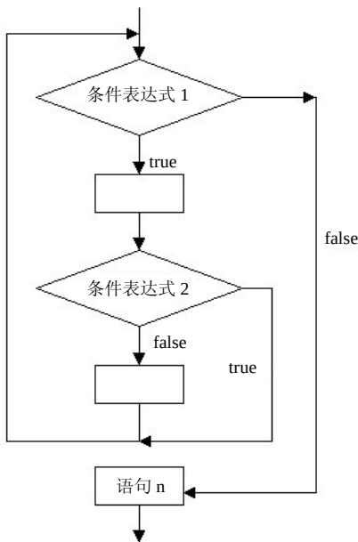
图4.9 使用continue语句的流程图
