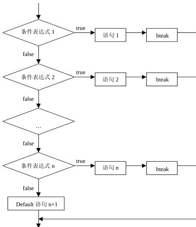
图4.4 switch语句流程图
