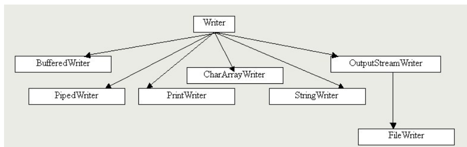
图15.8 Writer的体系结构
