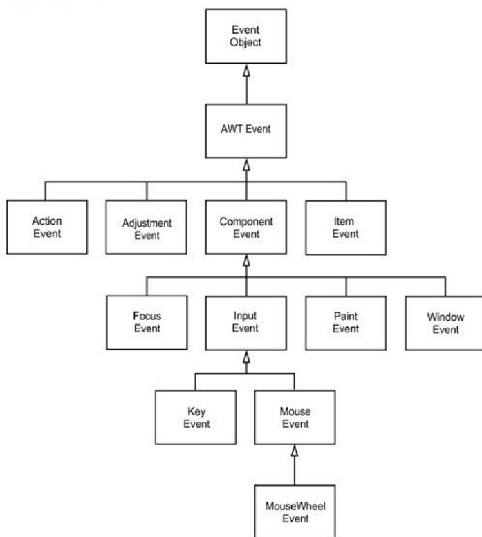
图13.3 所示事件继承关系
