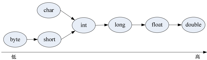
图2.1 数据类型级别与取值范围
