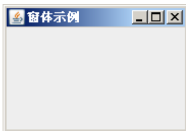
图10.6 简单窗体
