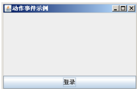
图13.4 登录界面
