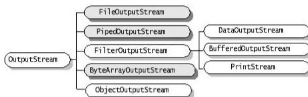
图15.2 OutputStream继承图
