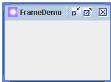
图10.10 窗口设置
