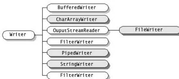
图15.4 Writer继承图
