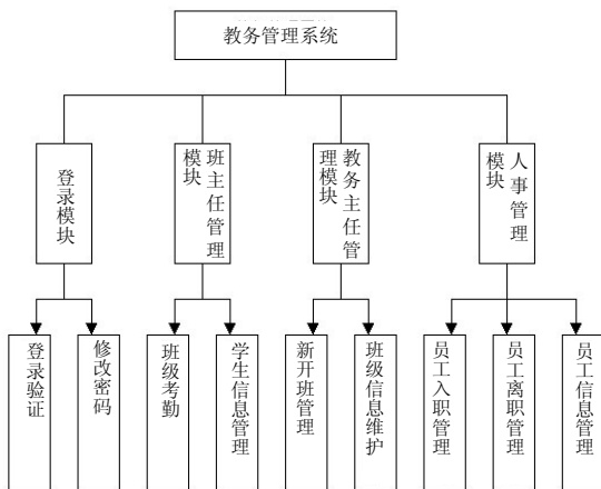
图22.1 系统总体模块设计
