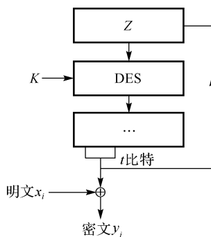
图 1.1.5 OFB 方式示意图
