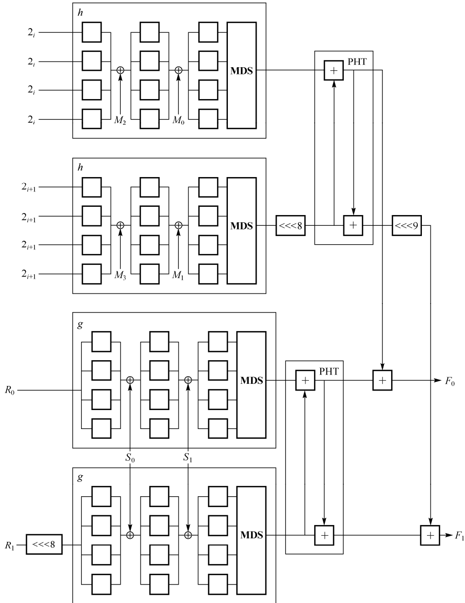
图 1.43.3 q_0 和 q_1 置换的逻辑框图
