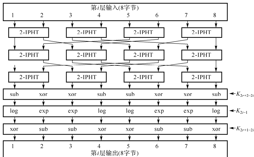
图 1.22.2 SAFERK-64 加密算法的脱密过程层函数结构
