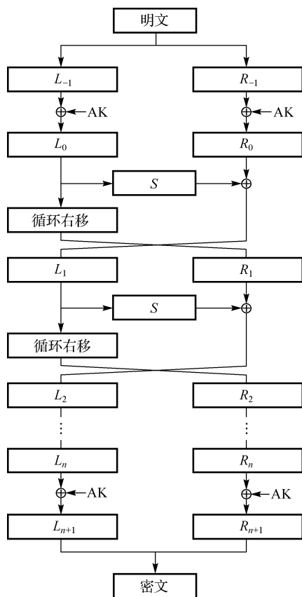
图 1.9.1 Khufu 加密算法
