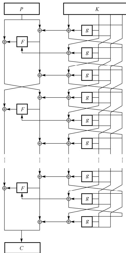
图 1.6.2 LOKI91 加密算法的结构框图和层密钥生成过程
