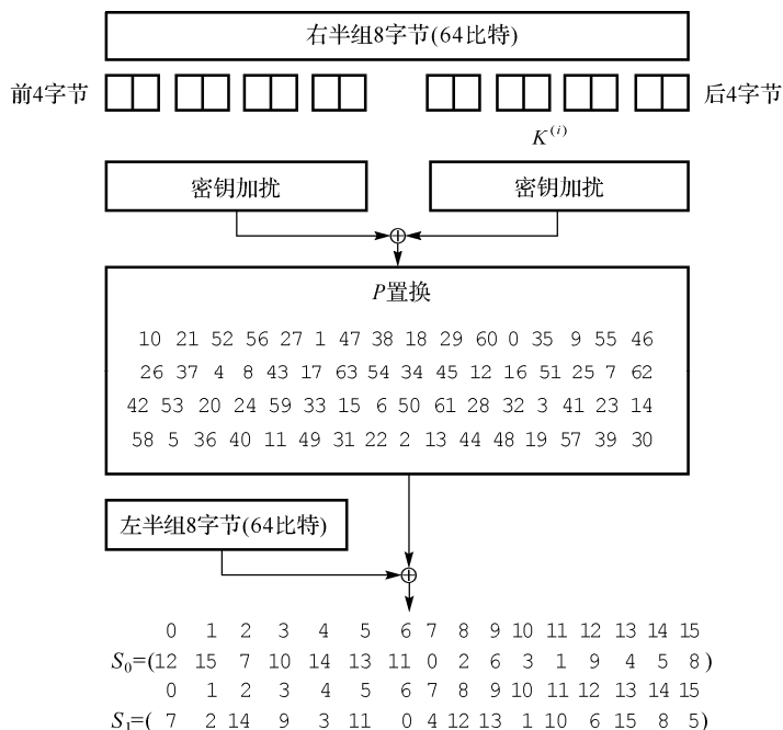
图 1.2.2 C-I-D 变换
