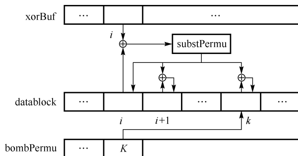
图 1.37.2 在每个字节上进行的 4 步基本运算
