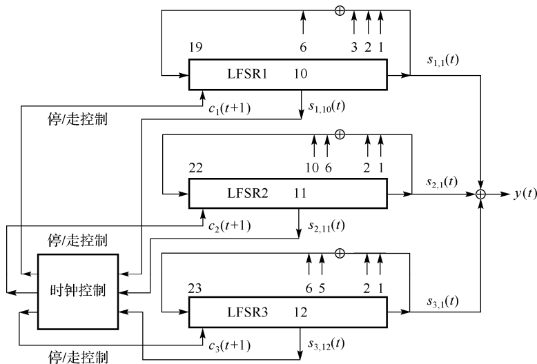
图 3.1.1 A5 加密算法的逻辑框图
