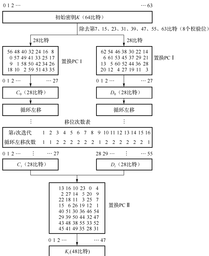
图 1.1.3 子密钥发生器
