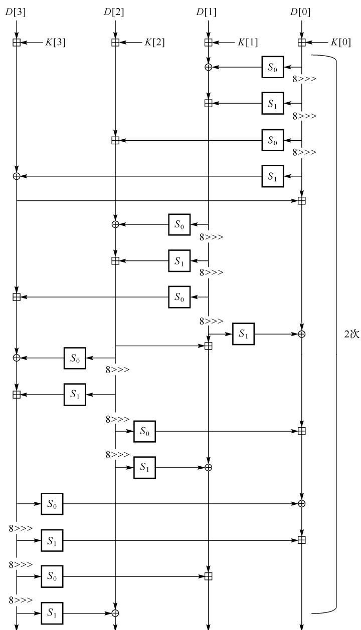
图 1.40.2 前向混乱部分的结构
