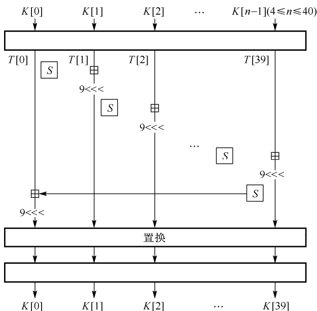
图 1.40.6 密钥扩展的框架结构
