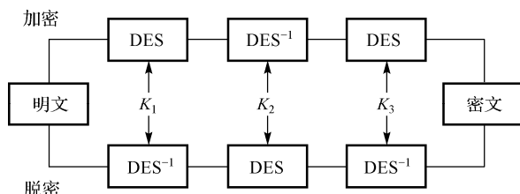
图 1.4.1 三重 DES 加密算法框图
