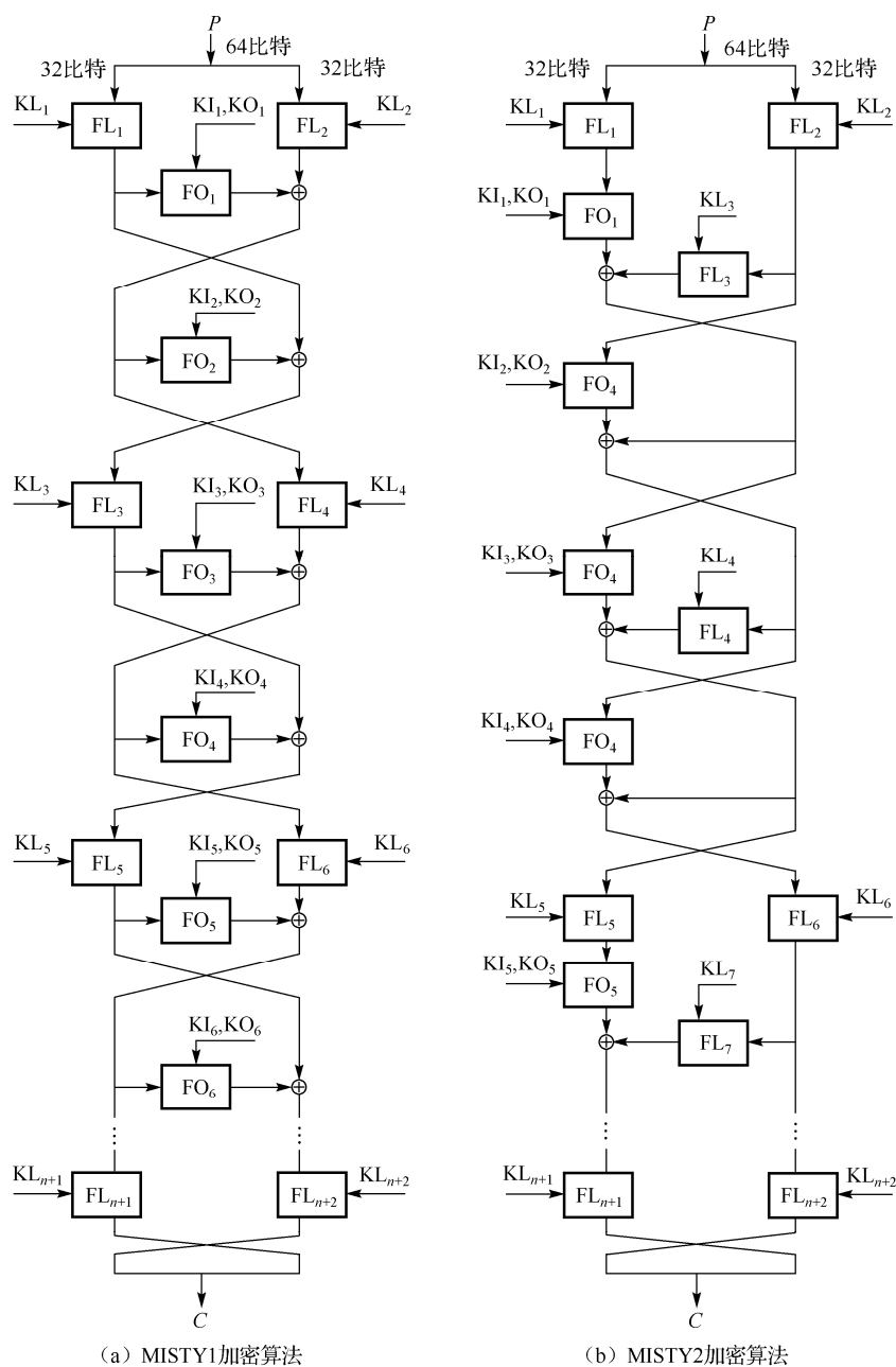
图 1.12.1 MISTY1 加密算法和 MISTY2 加密算法的结构
