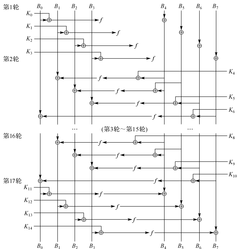
图 1.3.1 NewDES 加密算法
