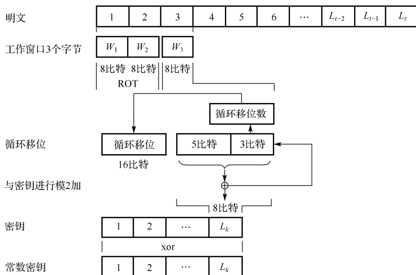
图 1.28.1 Madryga 加密算法的逻辑框图
