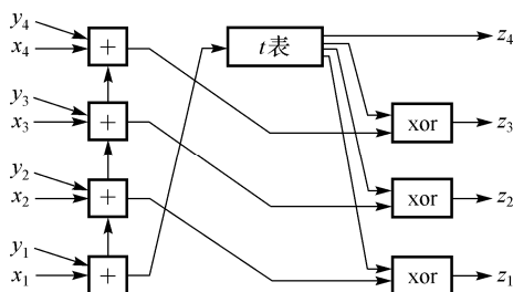
图 3.7.2 WAKE 加密算法的 t 表生成逻辑框图
