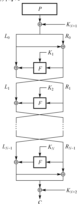
图 1.5.1 FEAL 加密算法框图
