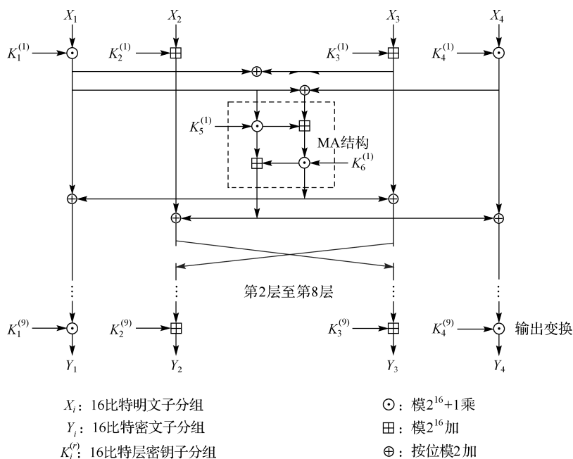
图 1.20.1 IDEA 加密算法
