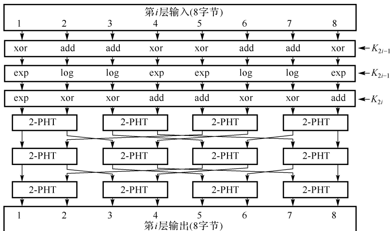
图 1.22.1 SAFERK-64 加密算法的加密过程层函数结构
