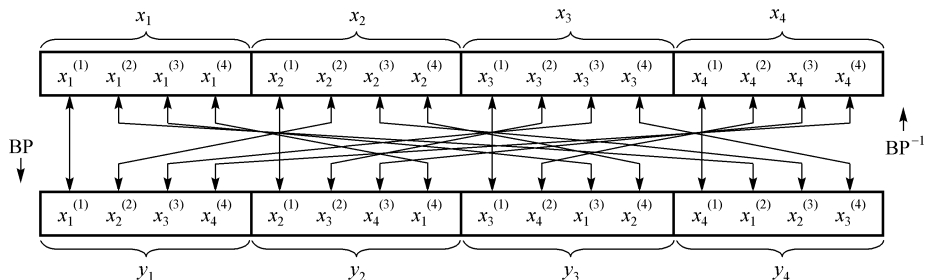
图 1.36.2 E2 加密算法 BP 函数的逻辑框图
