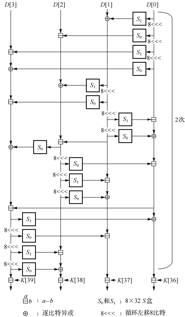
图 1.40.5 后向混乱部分的结构
