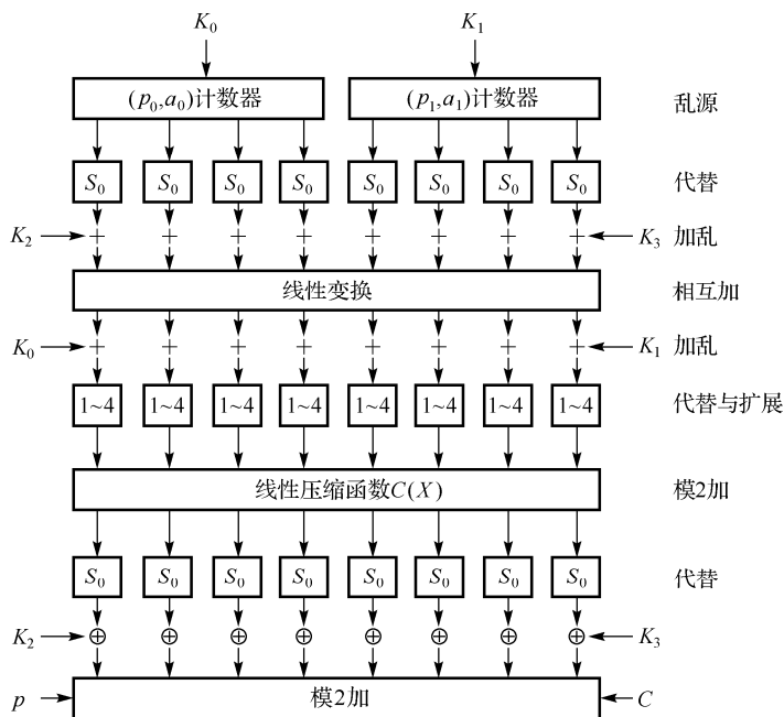
图 3.6.1 TWOPRIME 加密算法编制框图
