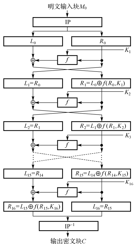
图 1.1.1 DES 加密算法
