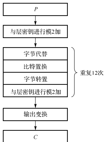
图 1.33.1 CRYPTON 加密算法的结构
