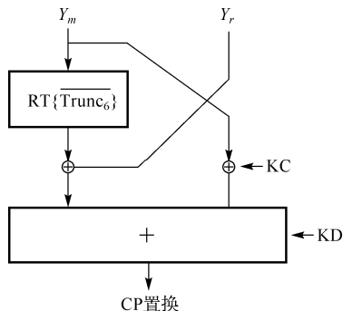
图 1.35.1 DFC 加密算法置换 CP 逻辑框图
