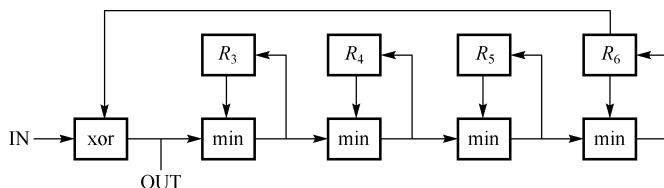
图 3.7.1 WAKE 加密算法的逻辑框图
