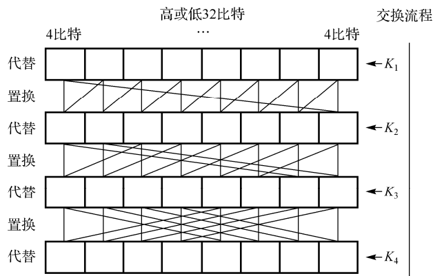
图 1.31.1 MULTI2 加密算法的代替-置换结构
