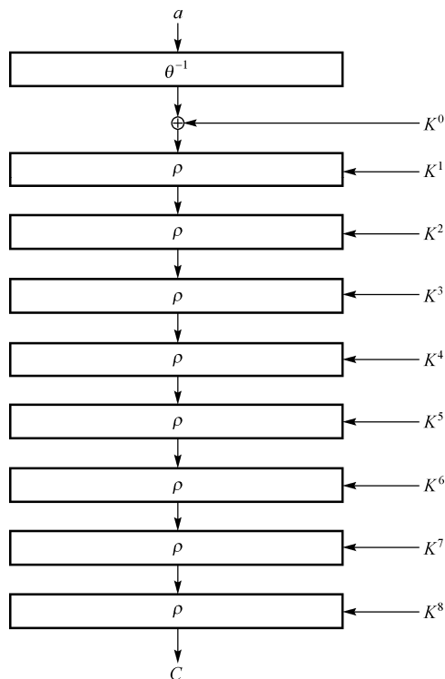
图 1.25.1 SQUARE 加密算法的结构框图
