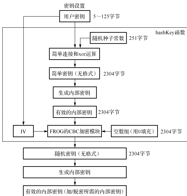
图 1.37.3 FROG 加/脱密算法的密钥设置过程
