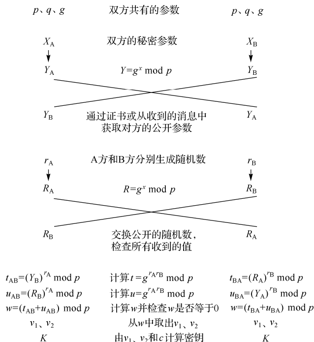
图 4.4.2 A 方和 B 方之间 KEA 交换关系图
