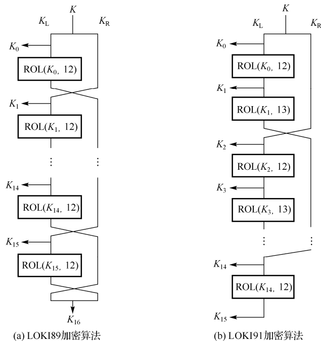
图 1.6.1 LOKI89 加密算法和 LOKI91 加密算法的层密钥生成规律
