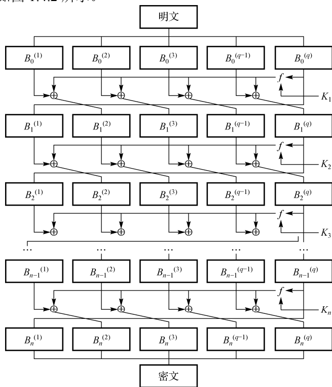
图 1.4.2 GDES 加密算法编制框图
