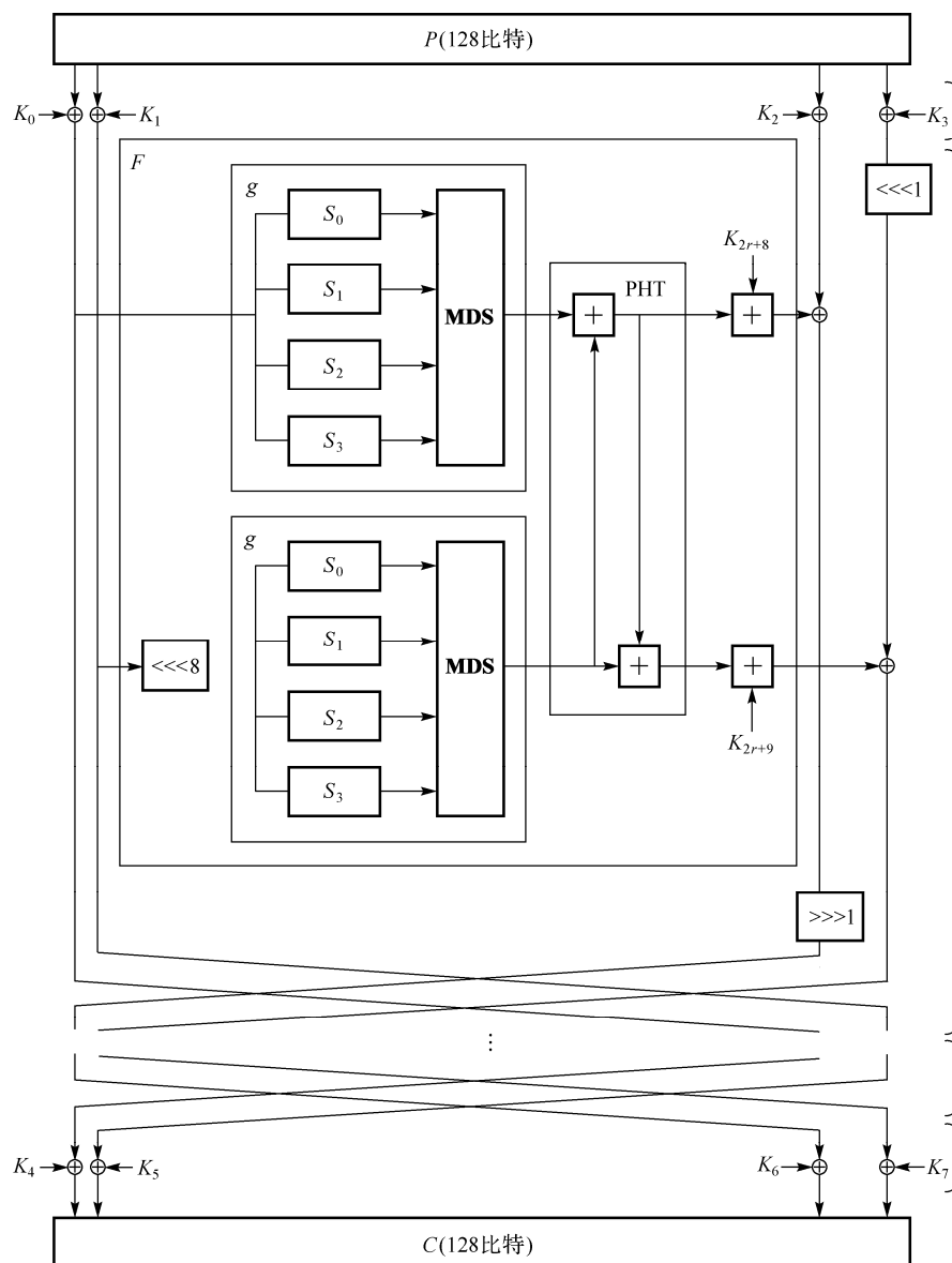
图 1.43.1 Twofish 加密算法的框架
