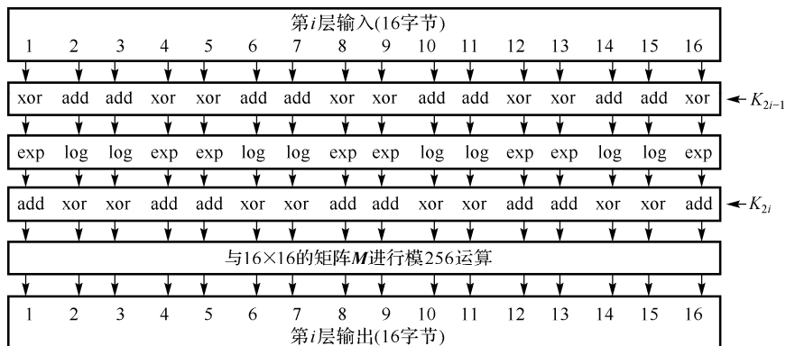
图 1.22.3 SAFER+加密算法的层函数结构
