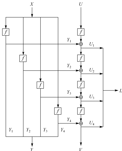
图 1.36.4 E2 加密算法密钥编制中所用的 G 函数的逻辑框图
