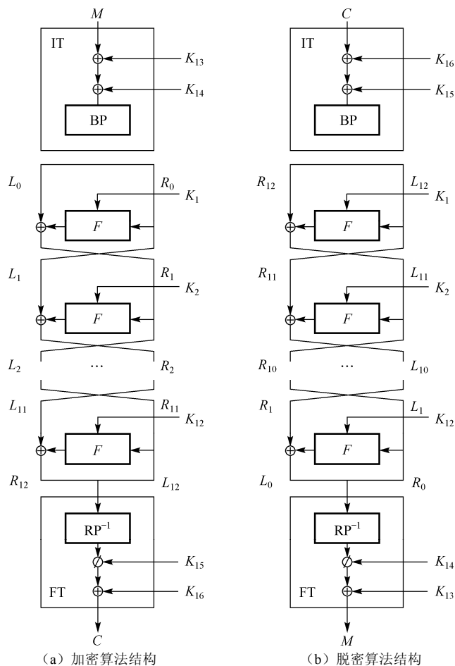
图 1.36.1 加/脱密 E2 算法的结构
