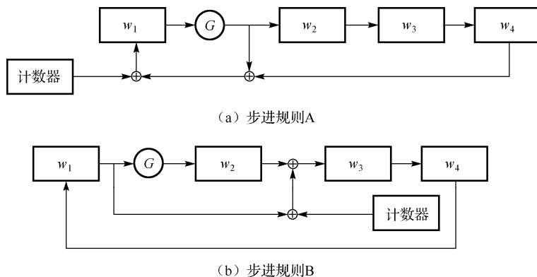
图 1.17.1 SKIPJACK 算法的两种步进规则
