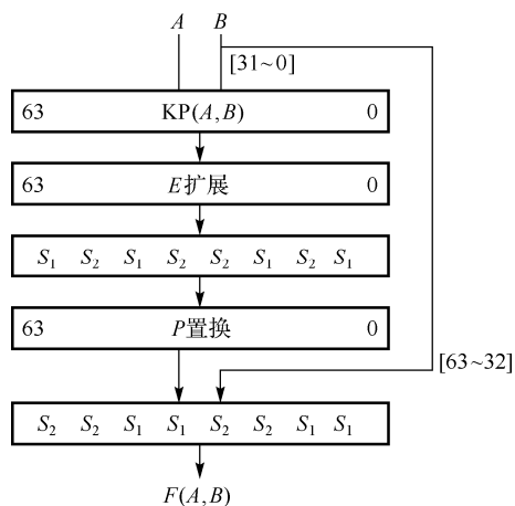
图 1.6.3 F(A,B) 函数的组成示意图
