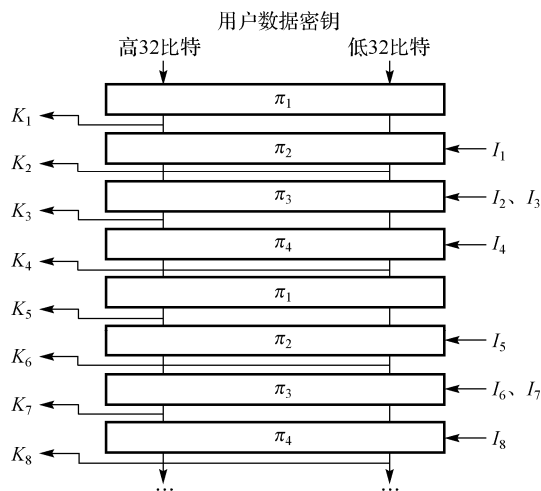
图 1.31.4 MULTI2 加密算法加密过程所需的加密密钥的生成过程
