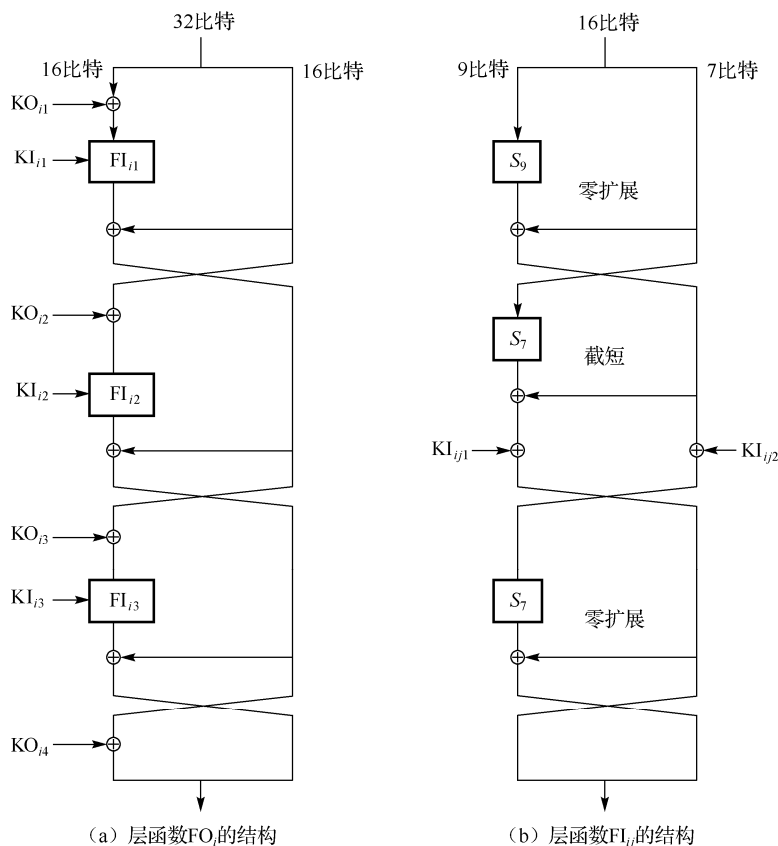
图 1.12.2 MISTY1 加密算法和 MISTY2 加密算法层函数的结构
