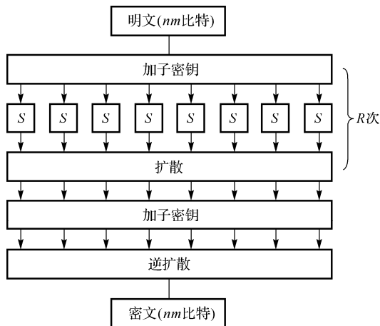
图 1.24.1 SHARK 加密算法的结构
