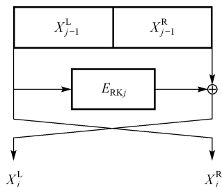
图 1.34.1 DEAL 算法 1 圈逻辑框图
