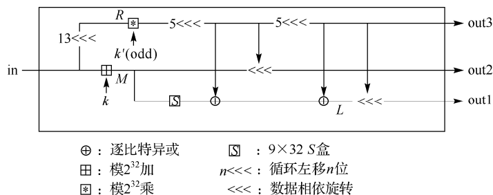
图 1.40.4 E 函数逻辑框图
