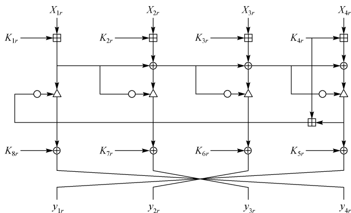
图 1.30.2 VINO 加密算法的层变换
