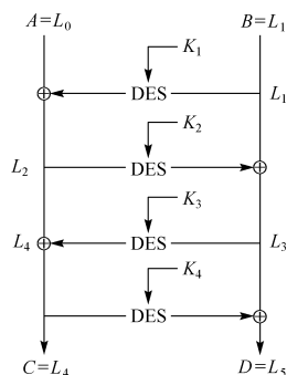
图 1.4.3 Ladder-DES 加密算法框图
