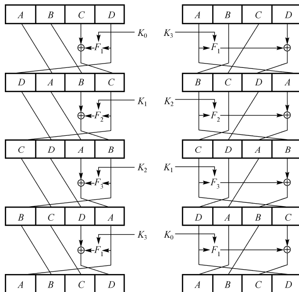
图 1.10.1 CAST-256 加密算法的两种层变换
