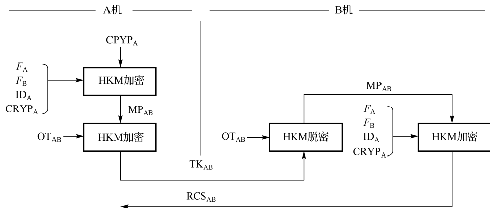
图 3.10.1 HKM/HFX 传真加密系统以注册方式进行通信的流程
