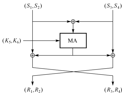
图 1.20.2 IDEA 加密算法中的对合结构
