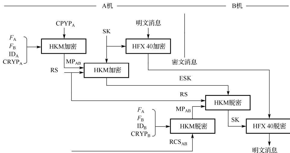
图 3.10.2 自动工作方式的通信流程
