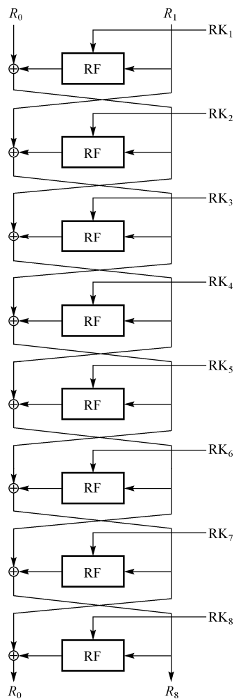
图 1.35.2 DFC 脱密算法的逻辑框图
