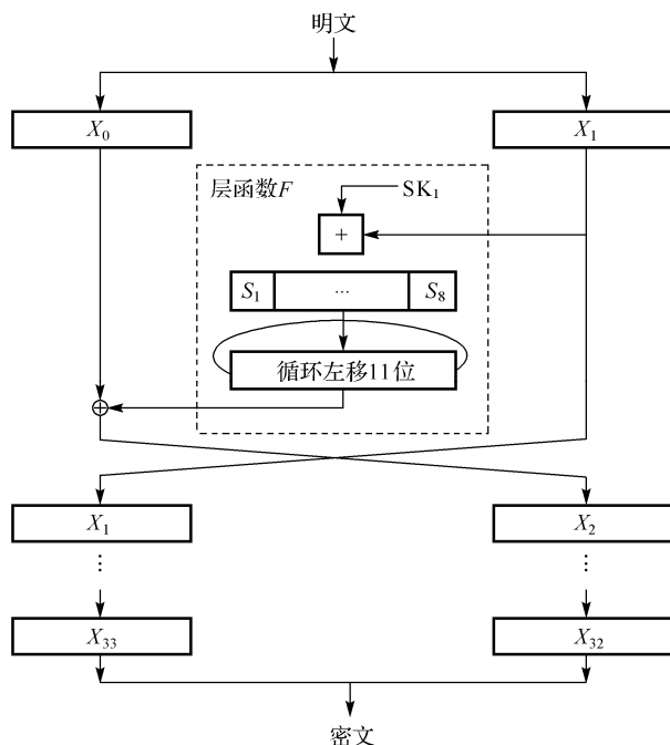
图 1.7.1 GOST 加密算法框图
