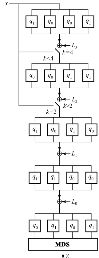
图 1.43.2 h 函数的逻辑框图
