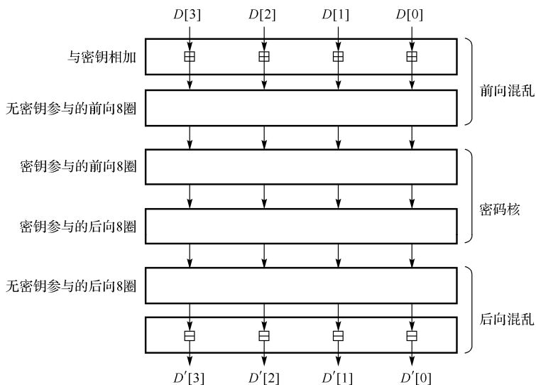
图 1.40.1 MARS 加密算法结构框架
