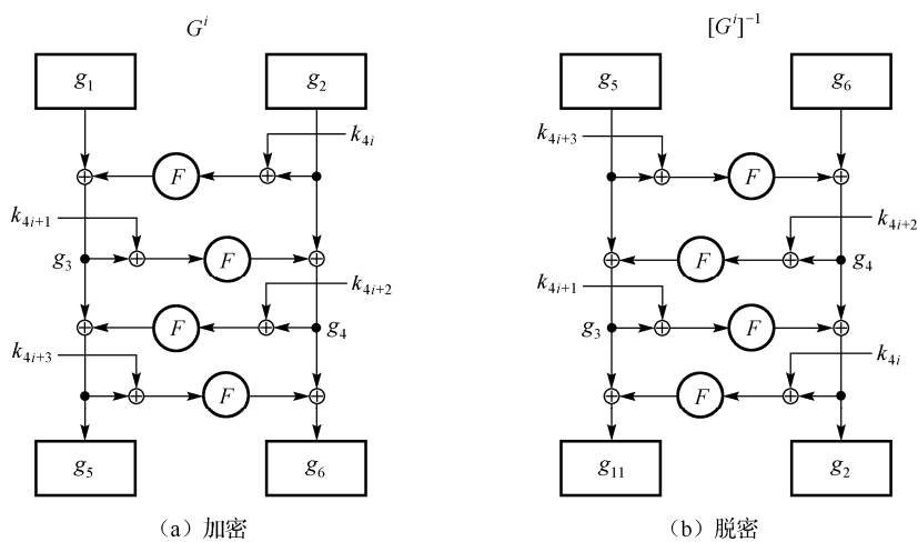
图 1.17.2 SKIPJACK 加密算法 G 置换
