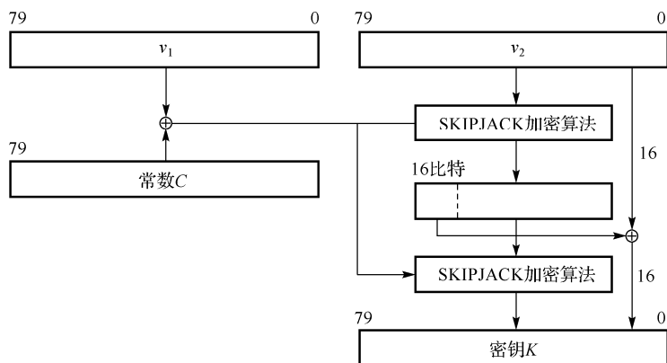
图 4.4.1 生成消息加密密钥的逻辑框图
