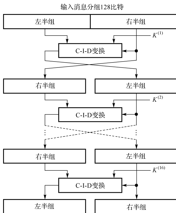
图 1.2.1 Lucifer 加密算法
