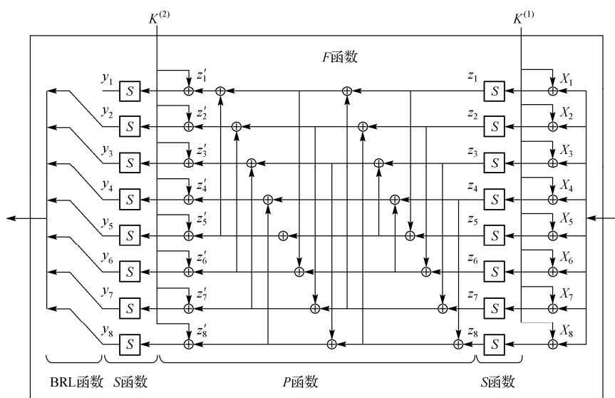
图 1.36.3 包含 S 、 P 、BRL 函数的 F 函数
