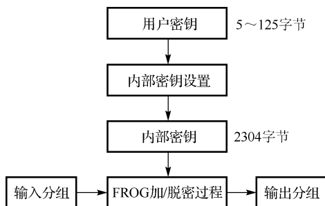
图 1.37.1 FROG 加/脱密算法的整体结构
