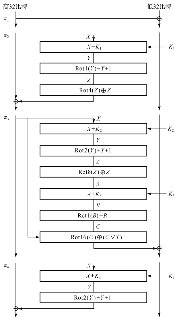
图 1.31.2 MULTI2 加密算法的 4 个基本函数
