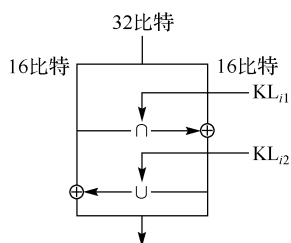
图 1.12.3 层函数 FL_i 结构
