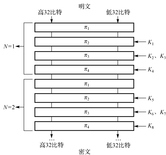
图 1.31.3 N 级 MULTI2 加密算法加密流程
