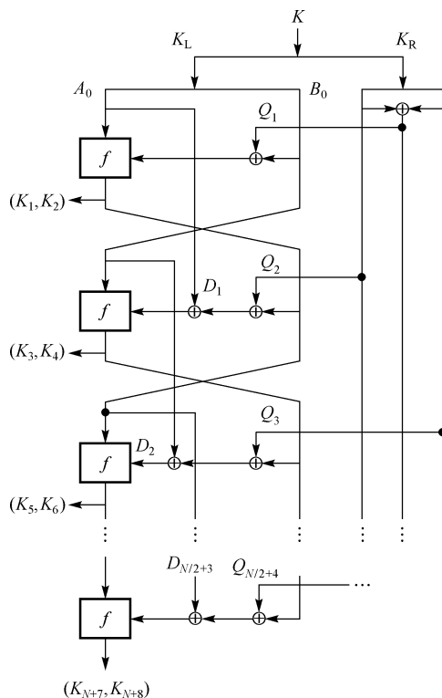
图 1.5.2 FEAL 加密算法的层密钥生成框图
