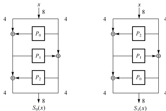
图 1.33.3 CRYPTON 加密算法的 S_0 和 S_1
