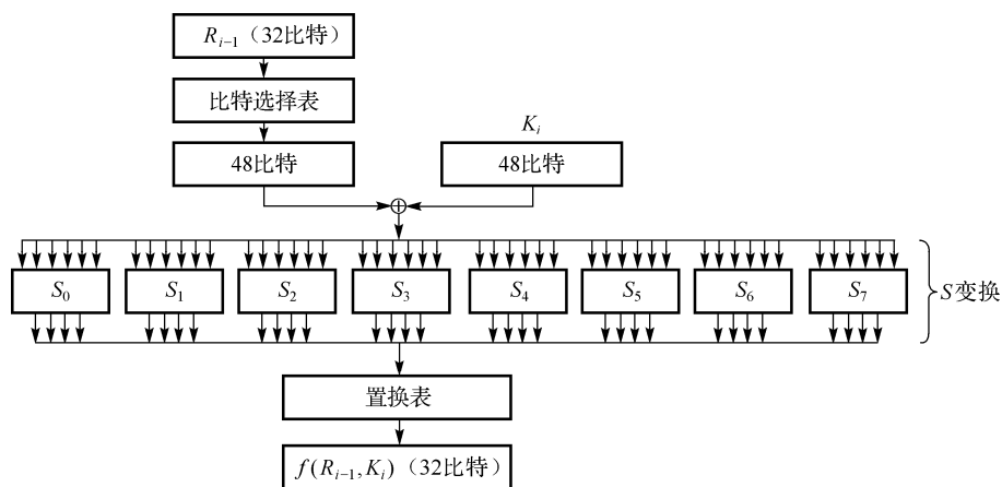
图 1.1.2 f 函数框图
