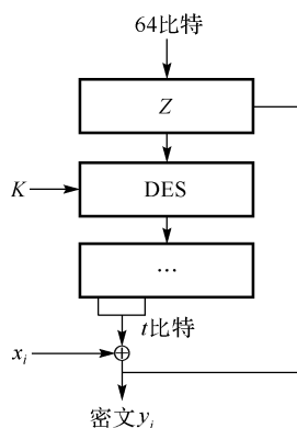
图 1.1.4 CFB 方式示意图
