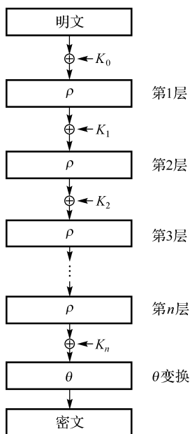
图 1.23.1 加密过程的逻辑框图
