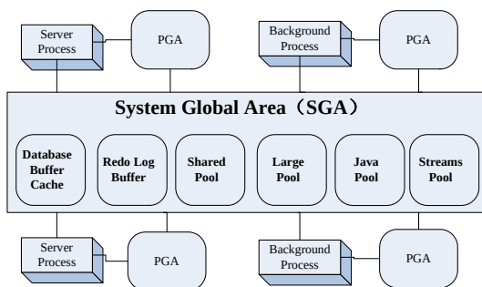
图 9-1 Oracle 内存结构
