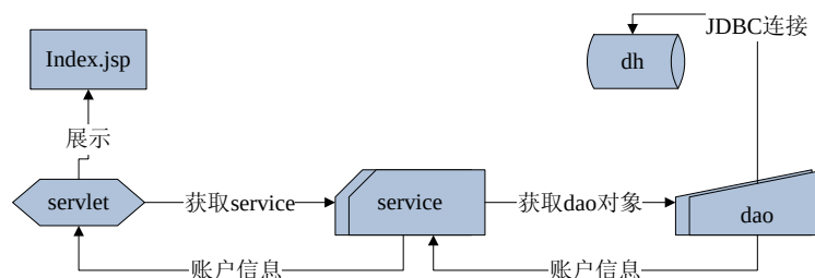
图 24-38 账户信息展示流程
