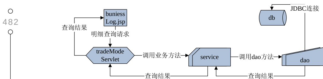
图 24-40 交易明细查询流程
