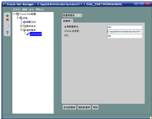
图 4-6 数据库服务设置
