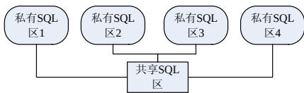
图 9-4 共享 SQL 区和私有 SQL 区的关系
