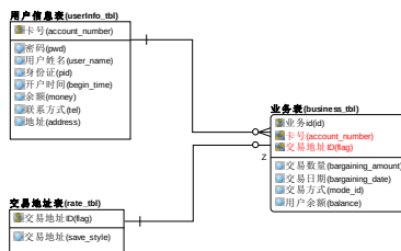
图 24-7 用户属性和表
