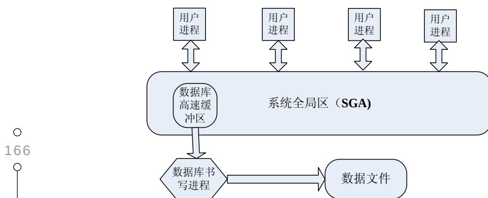
图 10-6 数据库书写进程的工作原理
