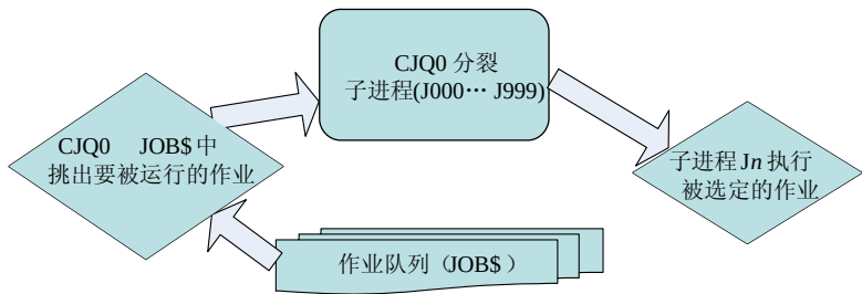
图 10-7 作业队列的工作原理
