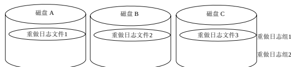
图 12-3 重做日志成员的分布
