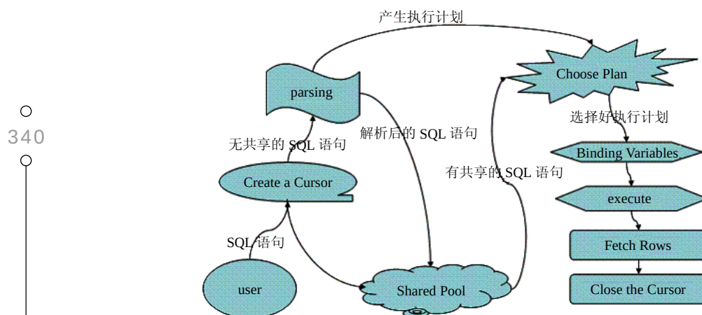
图 17-2 SQL 语句的执行过程
