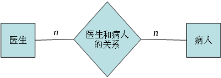
图 1-3 多对多关系
