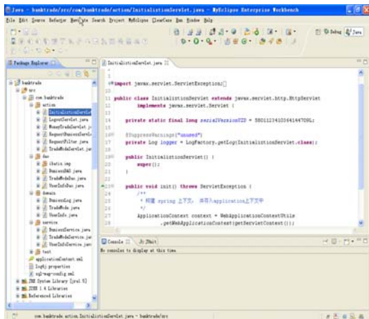
图 24-35 层次展示
