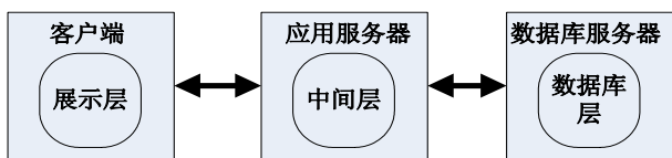
图 1-5 软件架构
