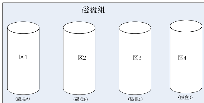
图 8-6 条块化（Striping）
