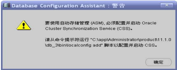
图 8-18 警告
