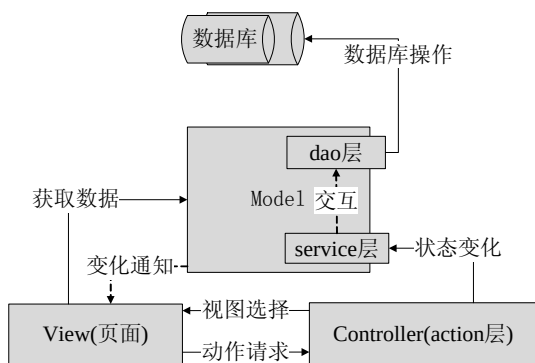
图 24-36 MVC 框架
