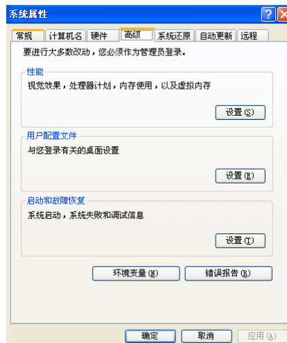
图 24-15 高级界面
