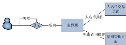
图 24-5 系统流程
