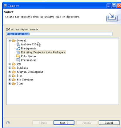
图 24-33 Import 界面
