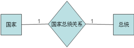
图 1-1 一对一关系
