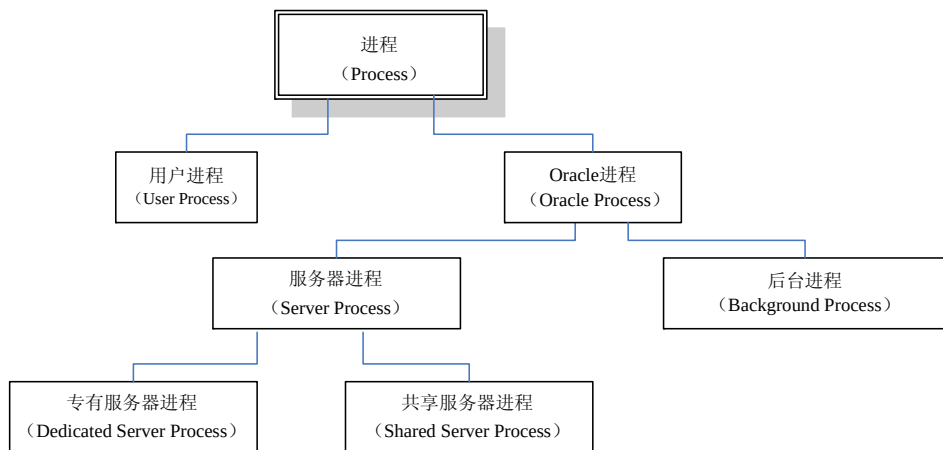
图 10-1 进程分类
