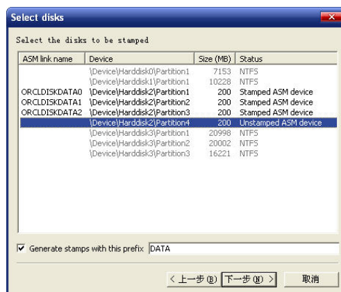
图 8-15 标记磁盘
