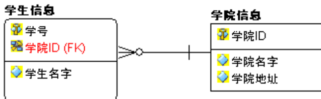
图 16-5 外键关系
