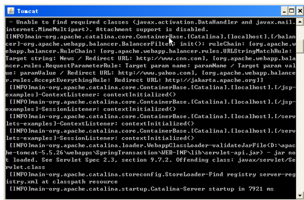
图 24-31 启动 Tomcat
