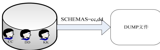
图 15-3 模式导出
