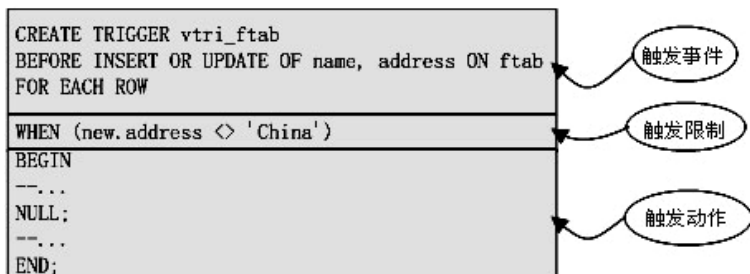
图 19-2 触发器的组成
