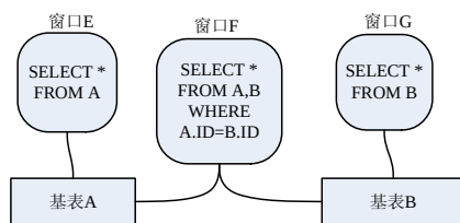
图 18-1 视图的窗口作用
