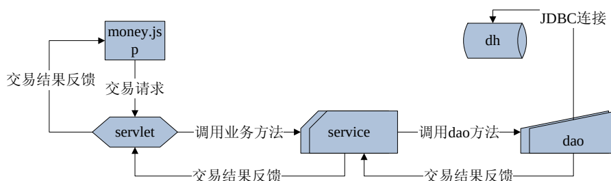
图 24-39 RMB 交易流程
