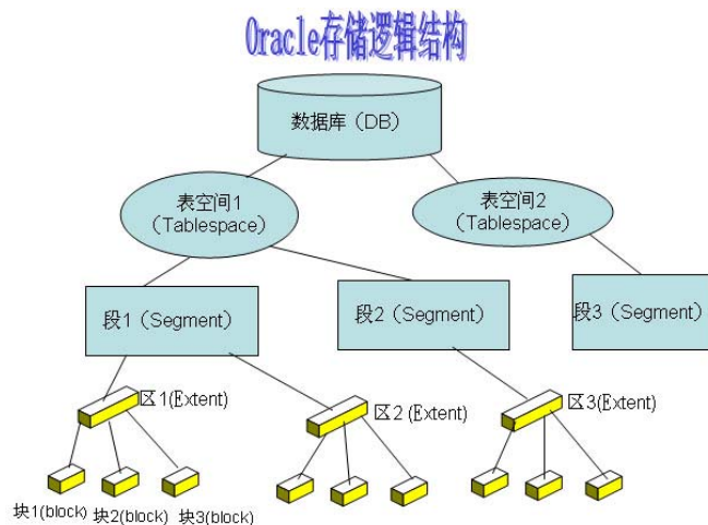
图 7-7 Oracle 存储逻辑结构
