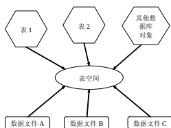
图 7-4 表空间和数据文件的关系
