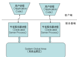
图 2-23 专有服务器模式的体系结构
