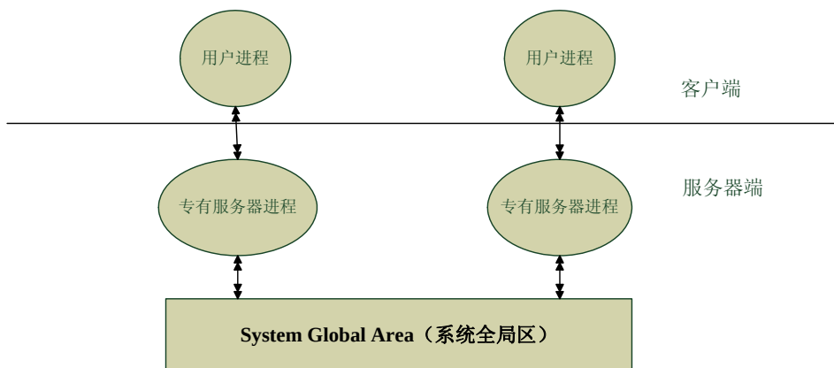
图 10-2 专有服务器进程的功能
