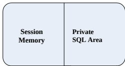
图 9-3 PGA 的组成
