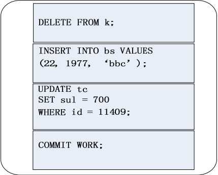
图 16-1 事务
