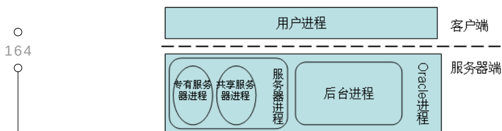
图 10-4 进程的位置
