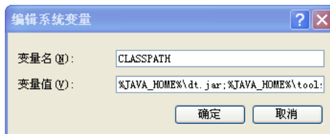
图 24-17 新建 CLASSPATH
