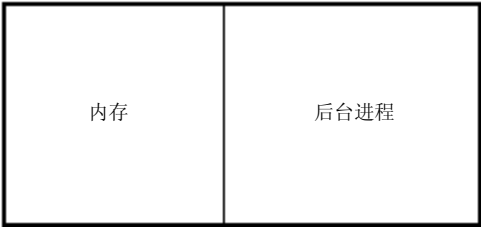
图 13-2 实例的组成
