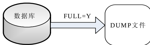
图 15-2 全库导出
