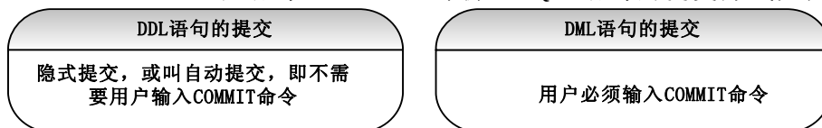
图 16-2 COMMIT
