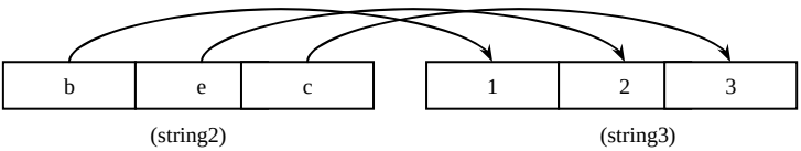
图 16-4 TRANSLATE 函数参数
