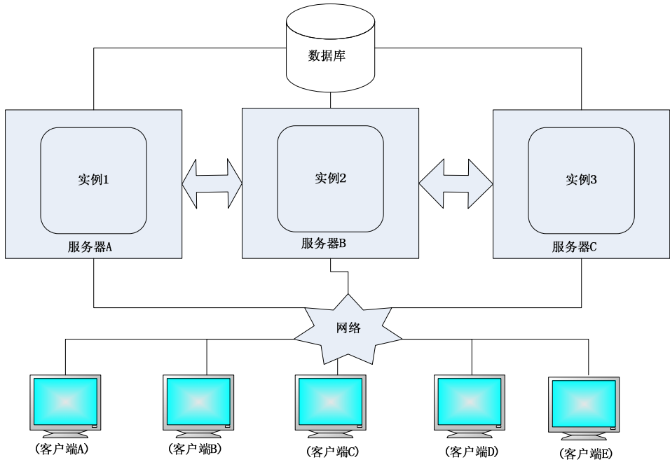
图 13-3 数据库和实例的关系
