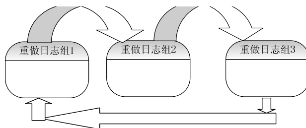
图 12-2 重做日志组的循环使用
