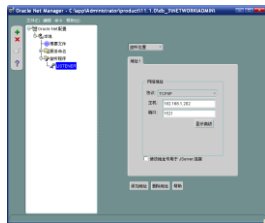
图 4-5 指定监听地址和端口号
