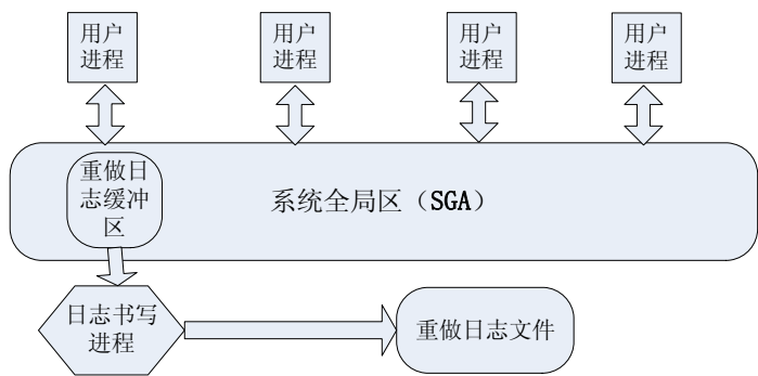
图 10-8 日志书写进程的工作原理
