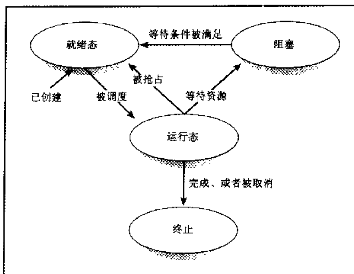
图 2.1 线程状态转换
