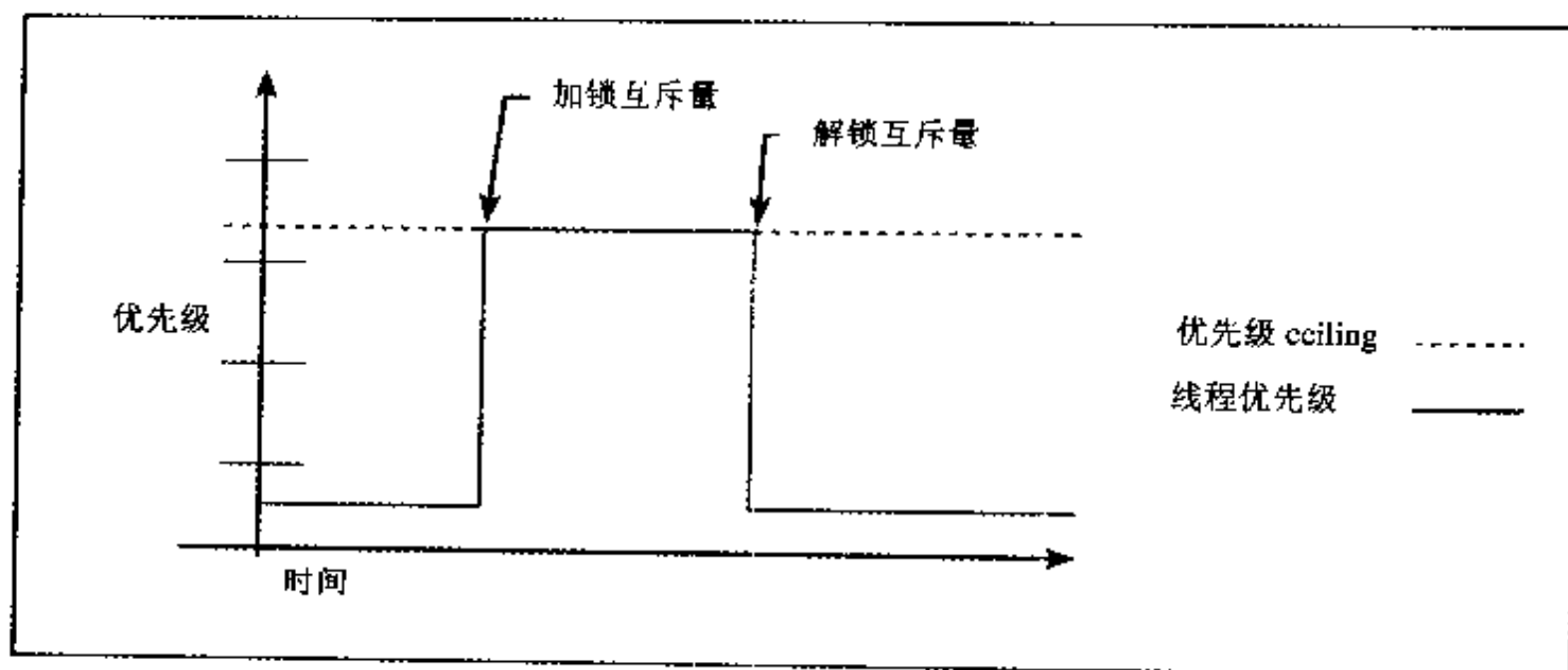
图 5.3 优先级 ceiling 互斥量操作
