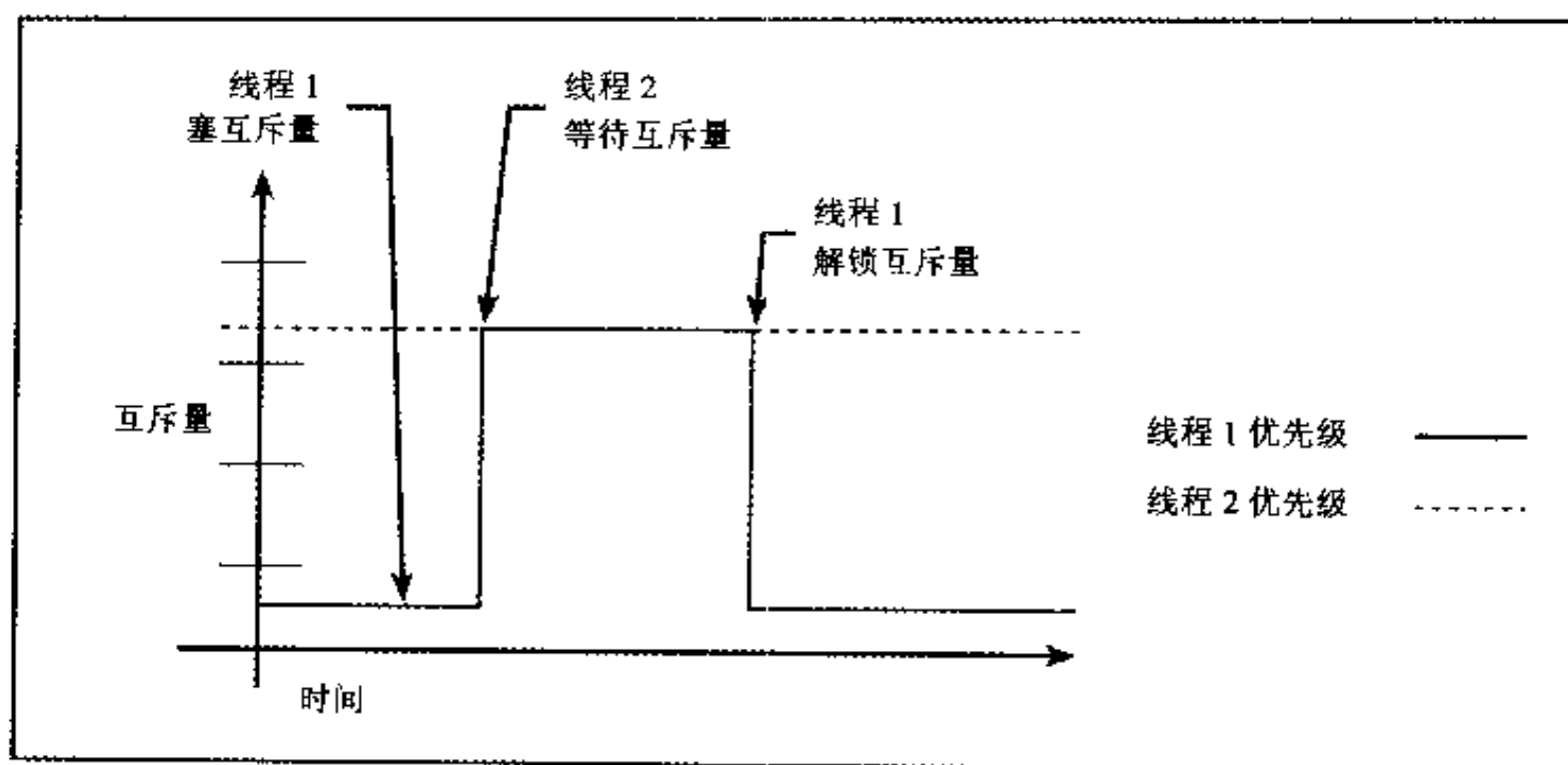
图 5.4 优先级继承互斥量操作
