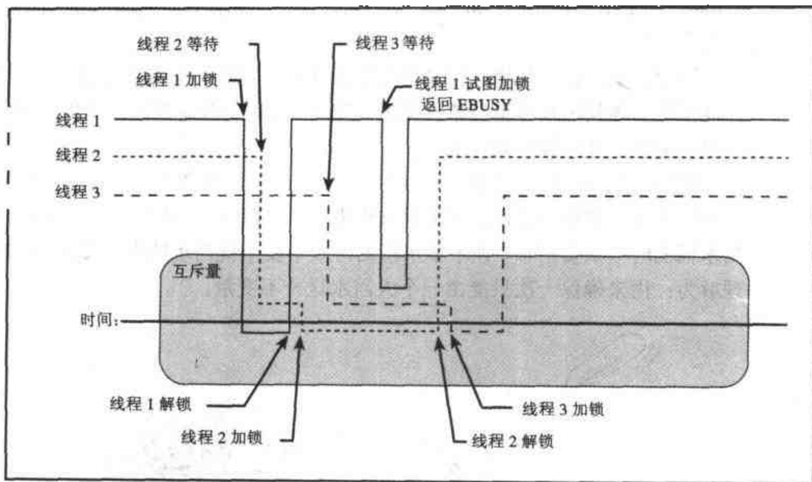
图 3.2 互斥量操作
