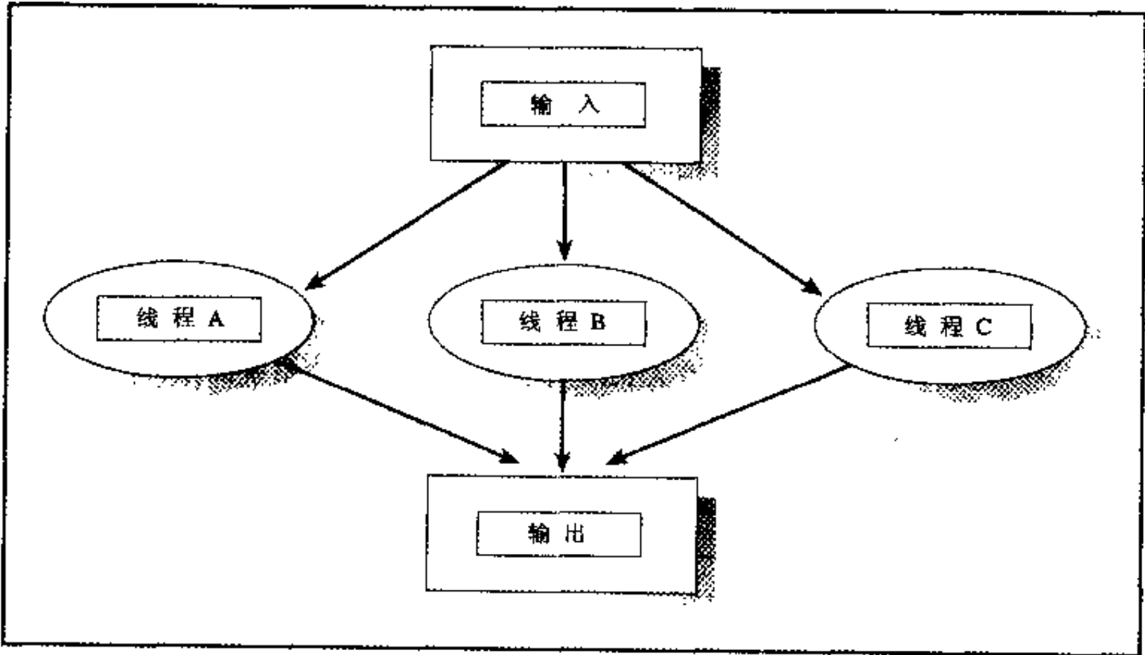
图 4.2 工作组模式
