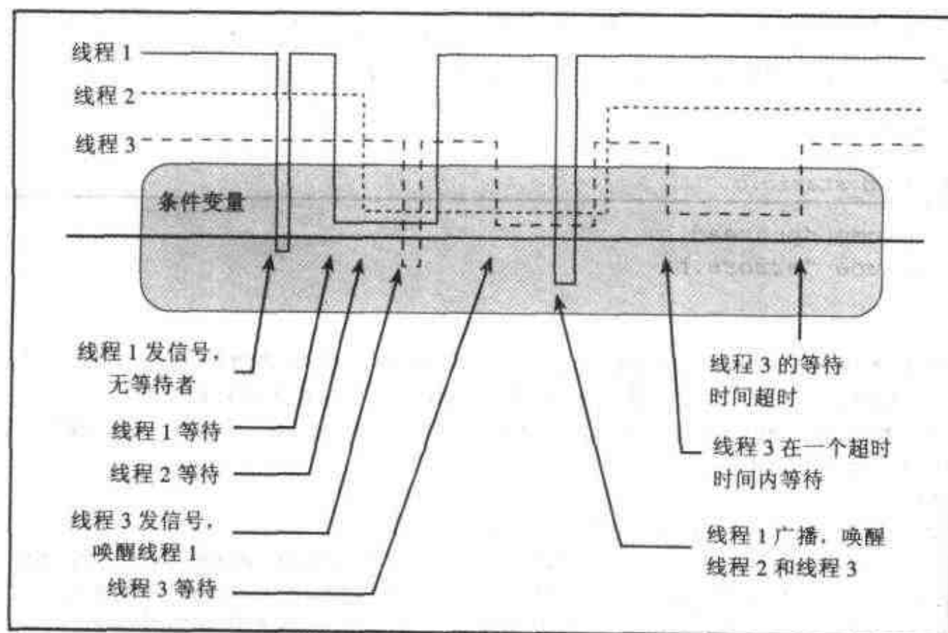
图 3.4 条件变量操作
