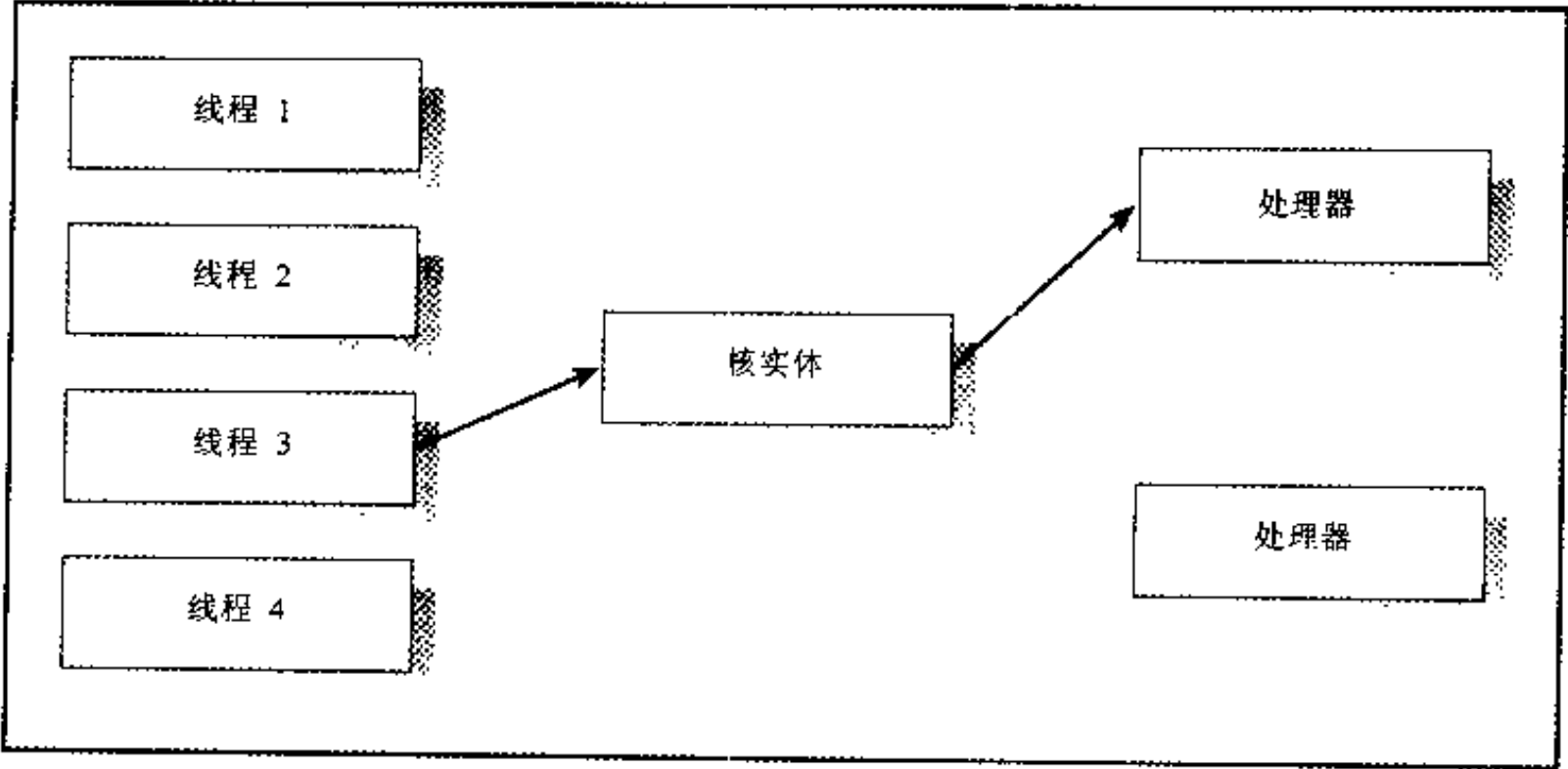
图 5.5 多对一线程图
