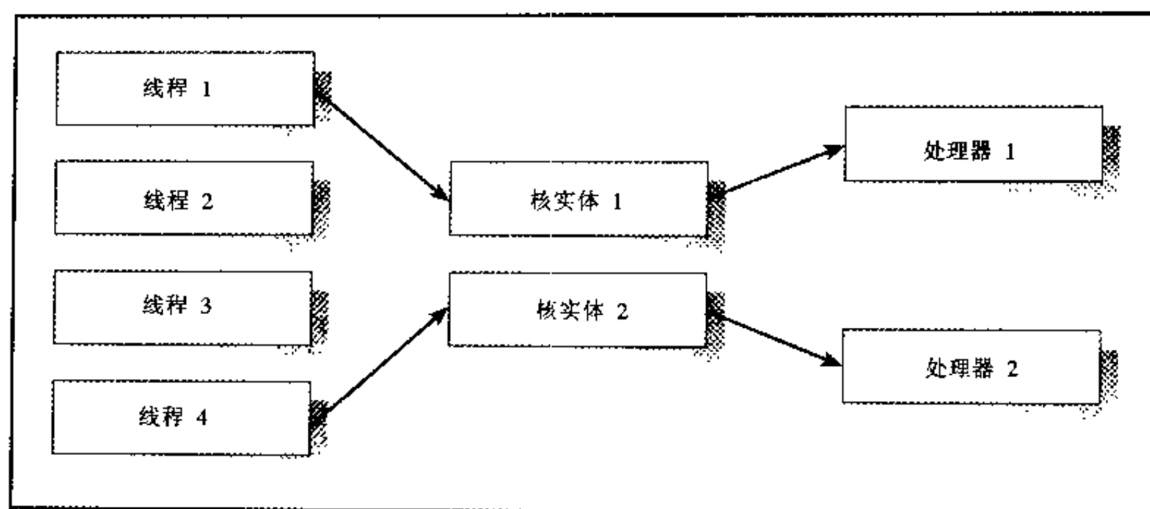
图 5.7 多对少线程图
