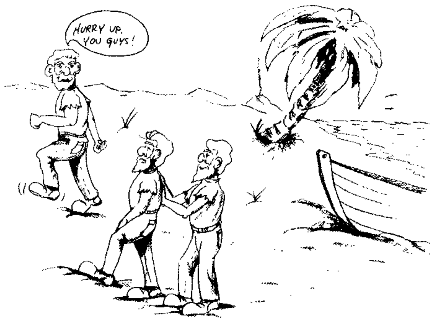
图 7.1 Barrier 类比
