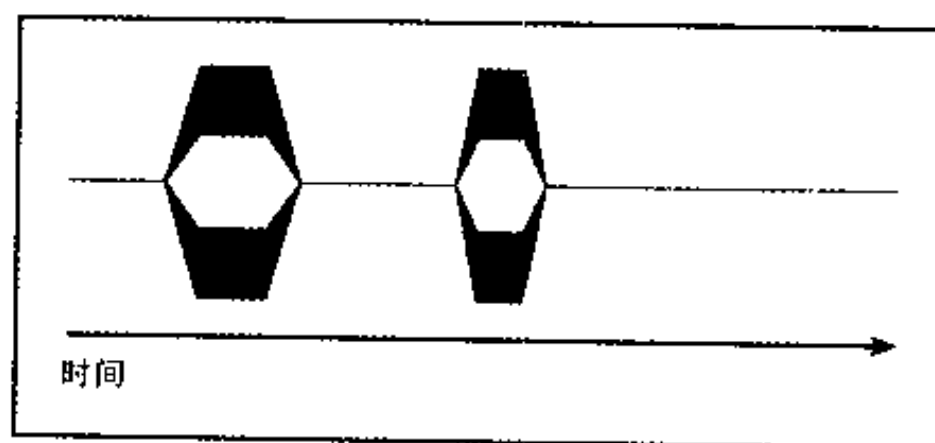
图 1.2 时间-并行图
