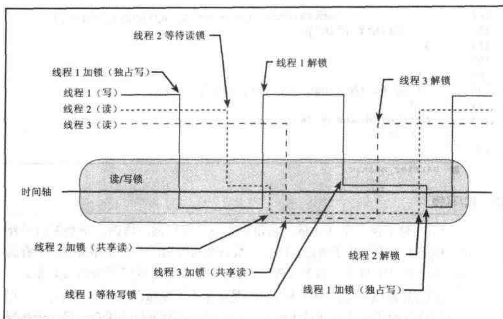
图 7.3 读/写锁操作
