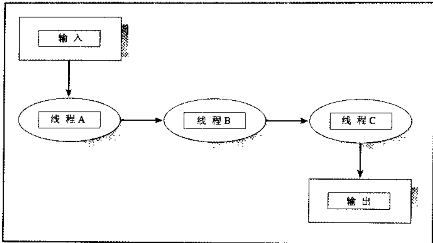
图 4.1 流水线
