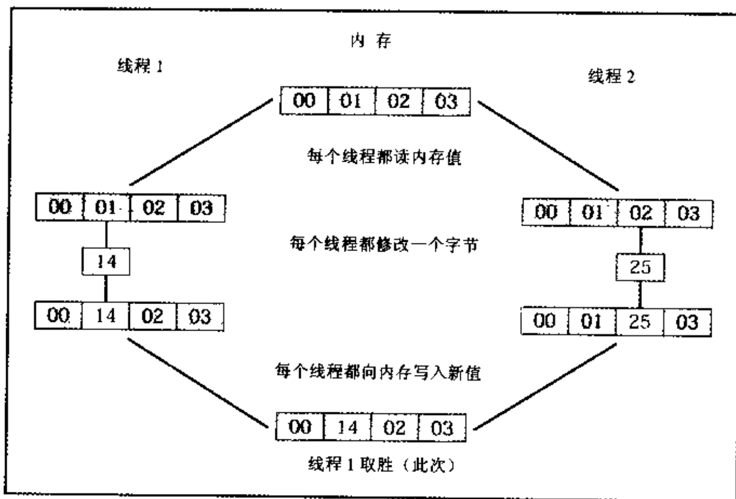
图 3.8 内存冲突
