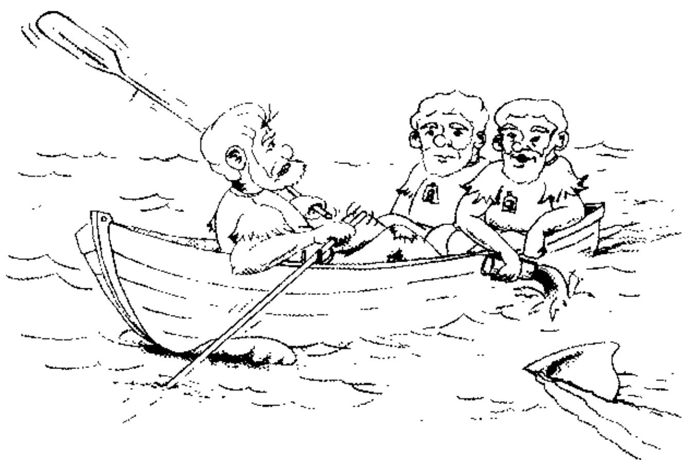
图 3.1 互斥量类比
