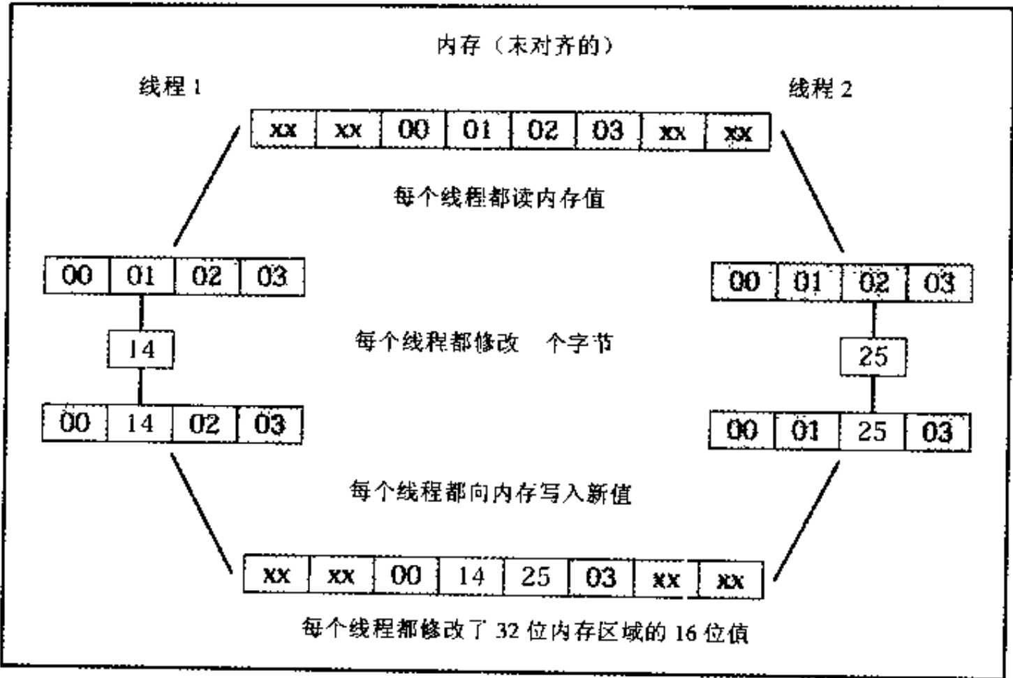
图 3.9 word tearing
