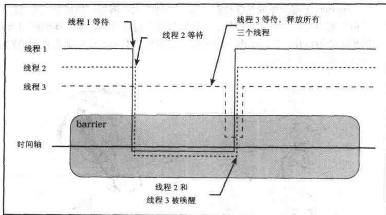
图 7.2 Barrier 操作
