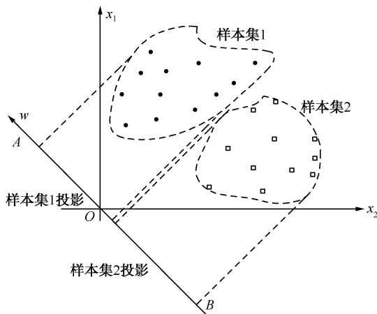
图 11.14 Fisher 线性判别示意图
