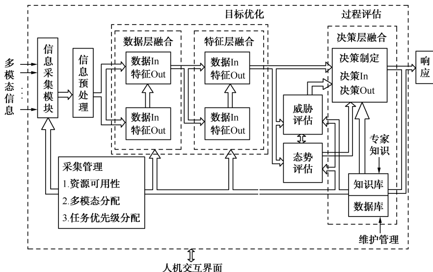
图 9.2 多模态信息融合的一般功能模型 [7]
