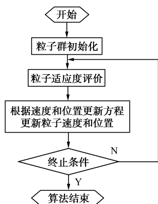
图 6.1 粒子群优化算法的流程图
