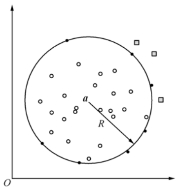
图 10.2 SVDD 中超球边界与支持向量
