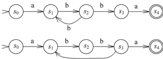
图 8-6 等价的 DFA 和 NFA
