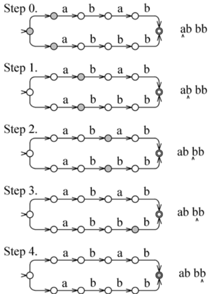
图 8-9 经过优化的 NFA 匹配过程
