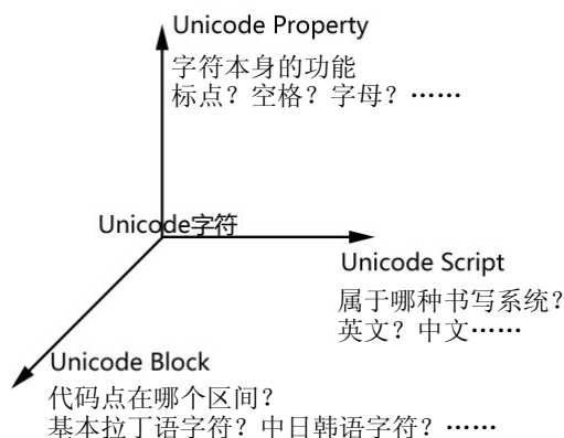
图 7-3 Unicode 字符的三种属性
