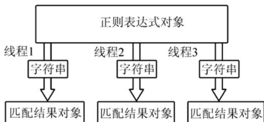
图 6-3 多线程环境下正确的处理模式
