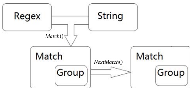
图 10-1 .NET 中与正则表达式相关的类
