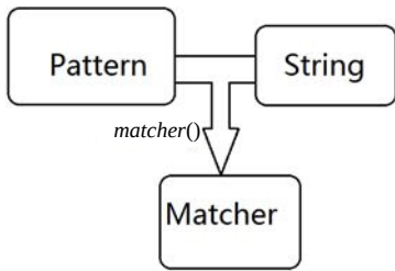
图 11-1 Java 中与正则表达式相关的类
