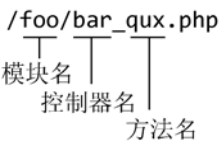
图 3-2 URL 的结构
