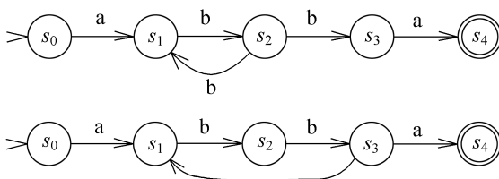
图 8-6 等价的 DFA 和 NFA
