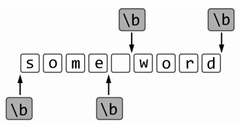
图 4-1 单词边界的匹配
