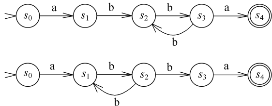
图 8-4 两台完全等价的自动机
