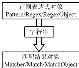
图 6-2 正则表达式操作中对象间的关系
