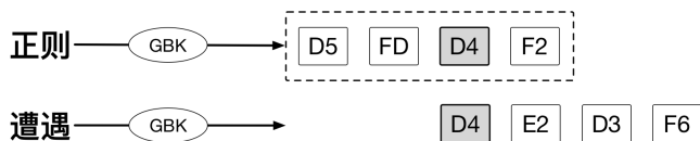
图 7-2 GBK 编码匹配出错原理
