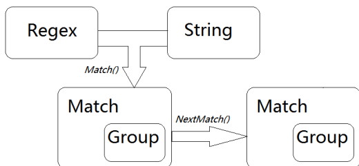
图 10-1 .NET 中与正则表达式相关的类
