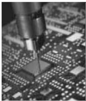
图 7.4 底部填充胶应用实例
