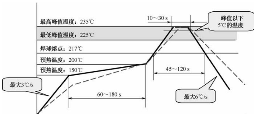
图 5.33 推荐的混装温度曲线（焊球全熔化）
