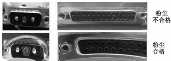
图 9.36 粉尘验收标准对比
