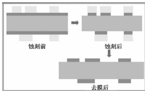
图 3.12 内层蚀刻
