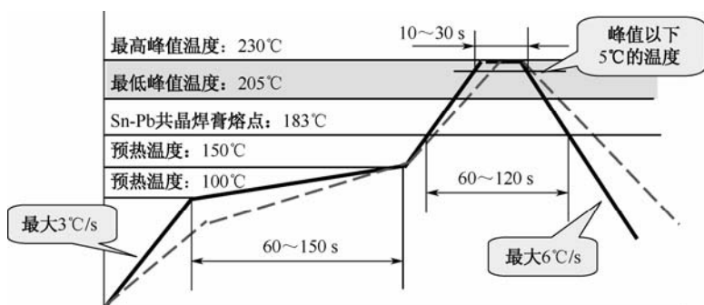
图 5.31 推荐的有铅工艺再流焊接温度曲线
