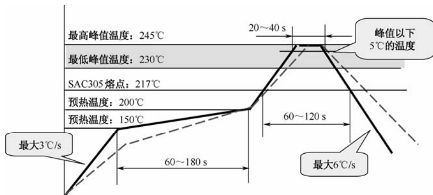
图 5.32 推荐的无铅工艺再流焊接温度曲线
