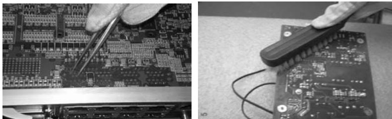
图 5.15 PCB 清洗方法
