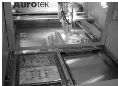
图 9.46 左右工作台交替作业
