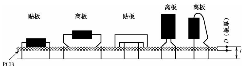
图 2.58 短插元器件
