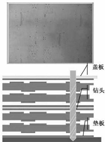
图 3.16 钻孔
