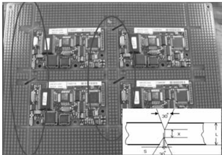
图 10.53 V 形槽连接设计
