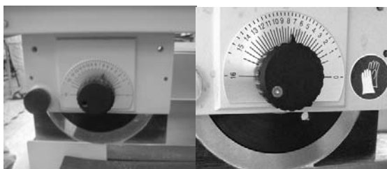
图 9.13 MEASTRO 4M 分板机上下刀片间隙调整
