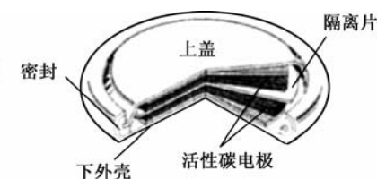
图 2.20 双层式电容器
