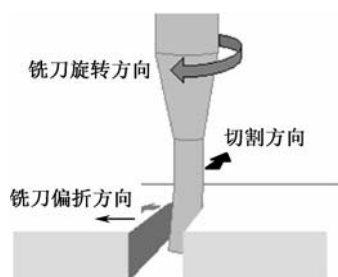
图 9.44 铣刀的偏折
