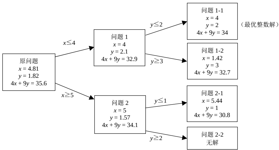
图 3-4 整数规划问题的解决步骤
