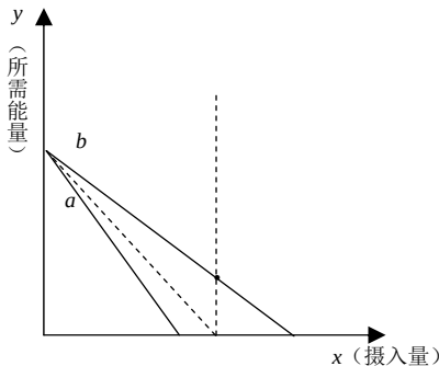
图 2-7 所需能量和摄入量之间的线性关系
