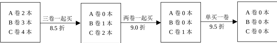
图 4-8 每次都是最优策略
