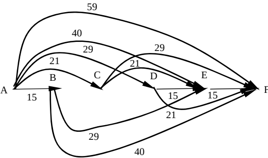
图 6-31 删掉连线 B—D 和 C—D
