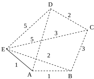
图 6-34 选择 A—E 连线
