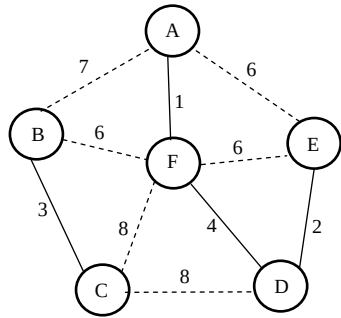
图 6-22 选择最短连线 F—D
