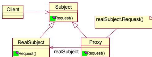
图 8-23 代理模式的 UML 类模型
