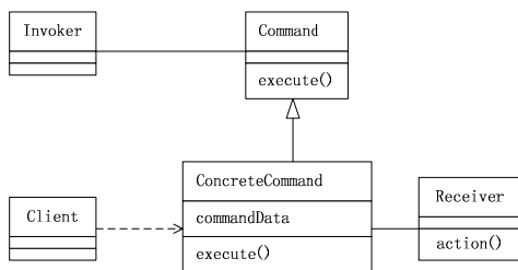
图 8-42 Command 类图
