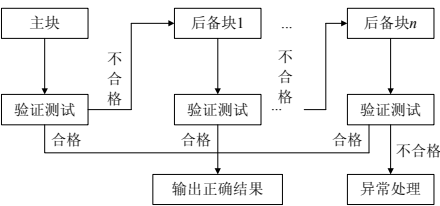
图 11-3 恢复块方法
