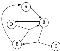
图 2-14 R 关系函数依赖示意图
