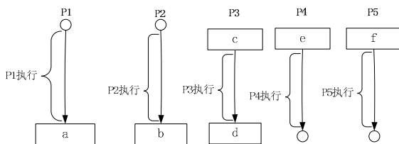
图 1-18 PV 操作控制过程
