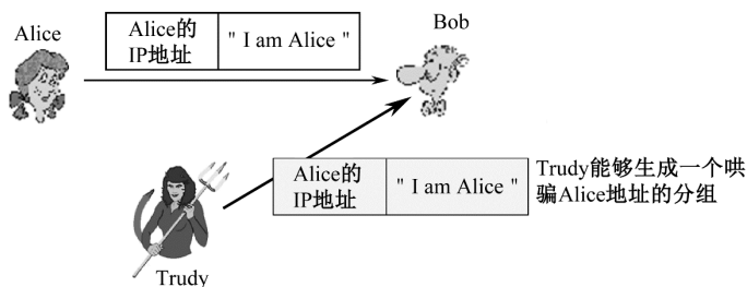
图 5-3 身份鉴别协议 ap2.0
