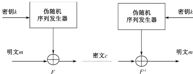
图 4-3 序列密码的加密、解密过程
