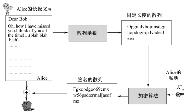
图 5-8 对报文摘要进行数字签名的实现过程
