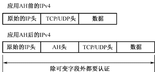
图 10-11 传输模式下 AH 协议报文封装
