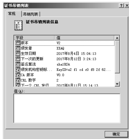
图 5-24 证书吊销列表
