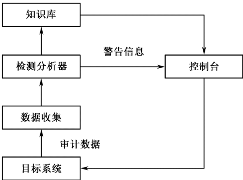
图 9-4 基于主机的入侵检测系统模型
