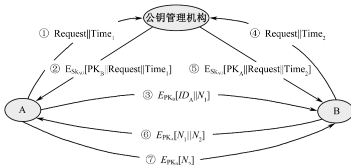
图 5-10 公钥管理机构分配公钥过程
