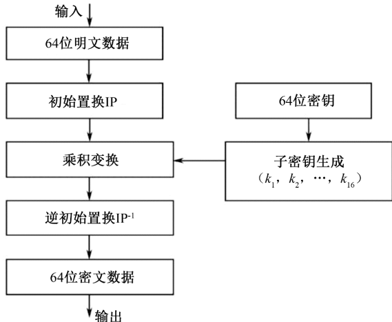
图 4-8 DES 加密过程
