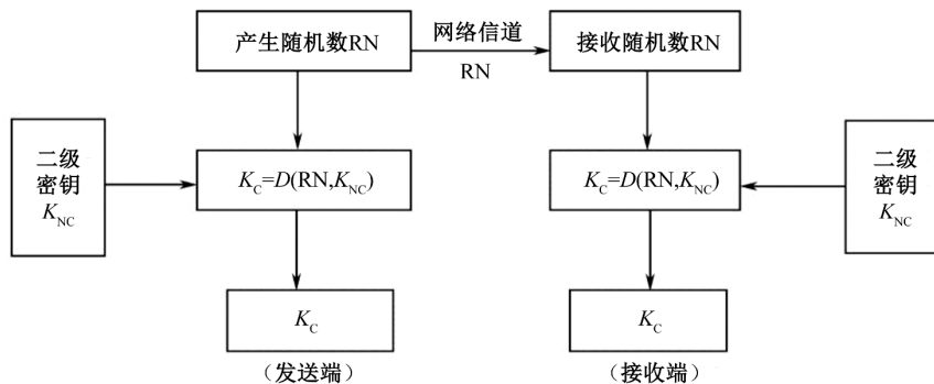
图 4-23 初级密钥的网络分配
