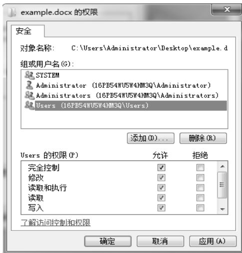
图 6-6 Windows 文件系统权限
