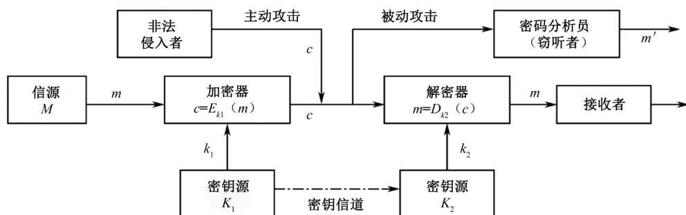
图 4-1 典型密码系统的组成
