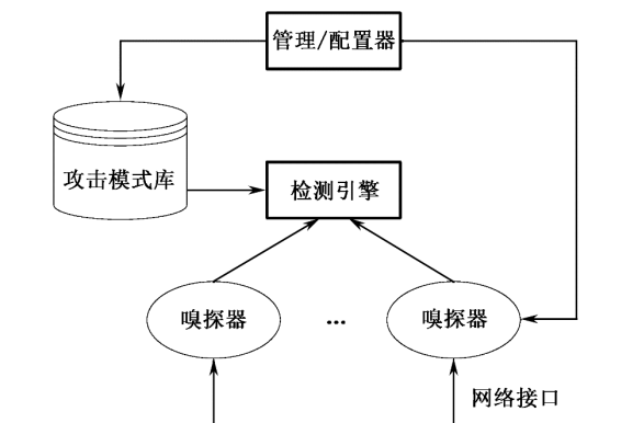
图 9-5 基于网络的入侵检测系统模型
