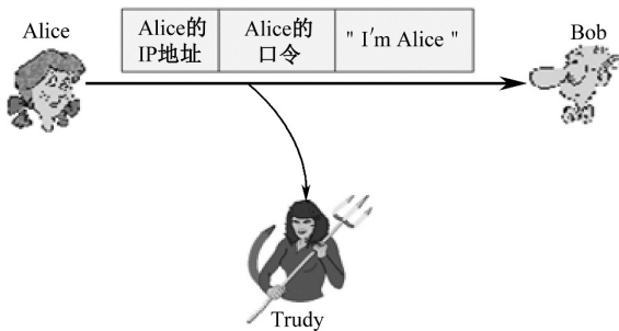
图 5-4 身份鉴别协议 ap3.0
