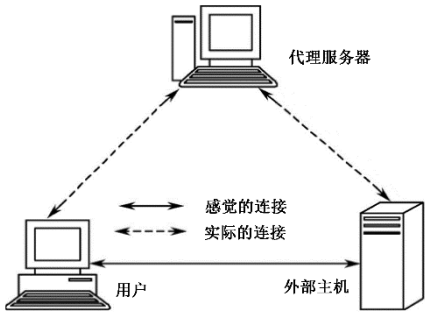
图 8-4 应用代理的实现过程
