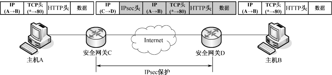
图 10-7 隧道模式的典型应用
