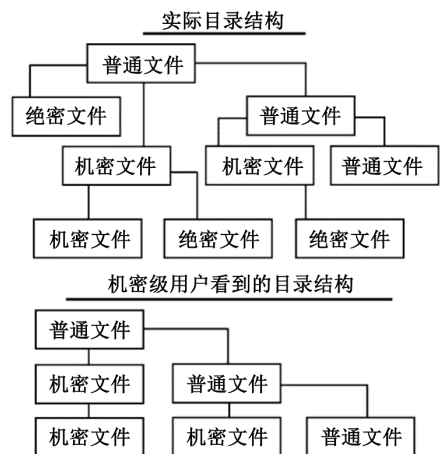
图 6-2 一个机密级用户所能看到的目录结构
