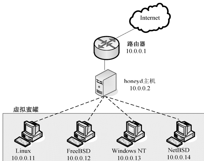
图 11-1 Honeyd 主机与其虚拟系统之间的关系
