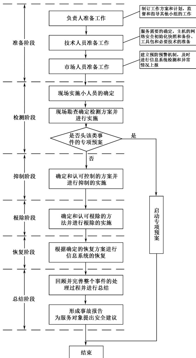
图 12-3 网络安全应急响应的一般流程
