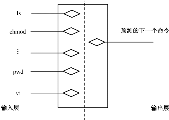
图 9-9 神经网络检测思想
