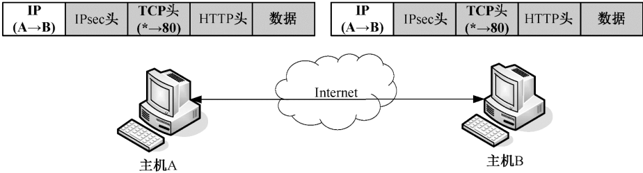
图 10-5 传输模式的典型应用
