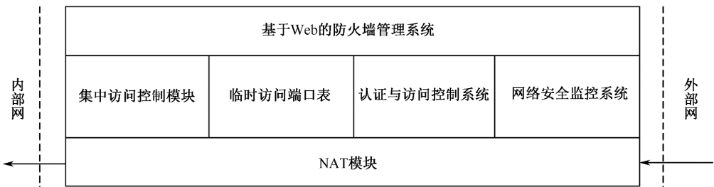
图 8-5 基于 NAT 的复合型防火墙系统的总体结构模型
