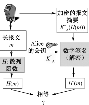
图 5-9 接收者对签名进行验证的过程
