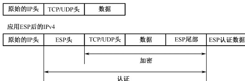
图 10-14 传输模式下 ESP 报文封装
