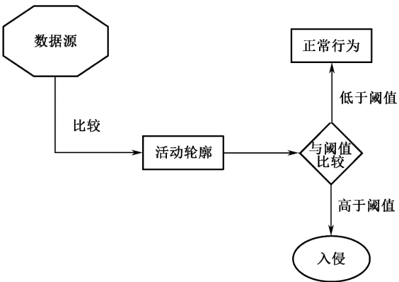
图 9-8 异常检测模型
