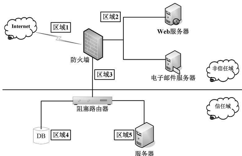
图 9-7 入侵检测系统部署
