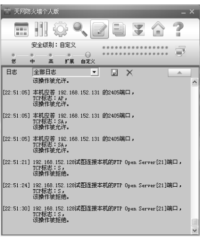
图 8-12 天网防火墙日志
