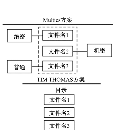
图 6-1 文件的安全级
