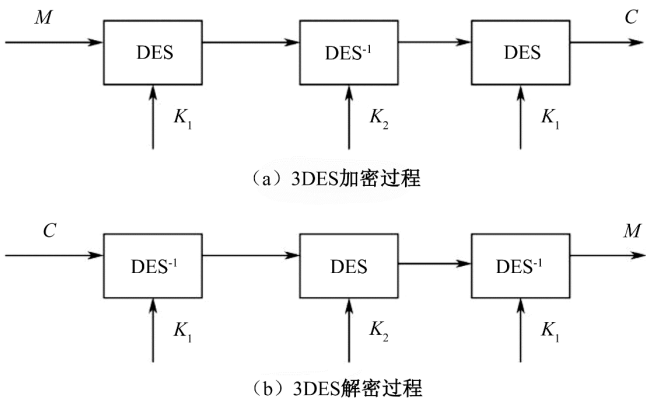
图 4-17 两密钥 3DES 加/解密过程
