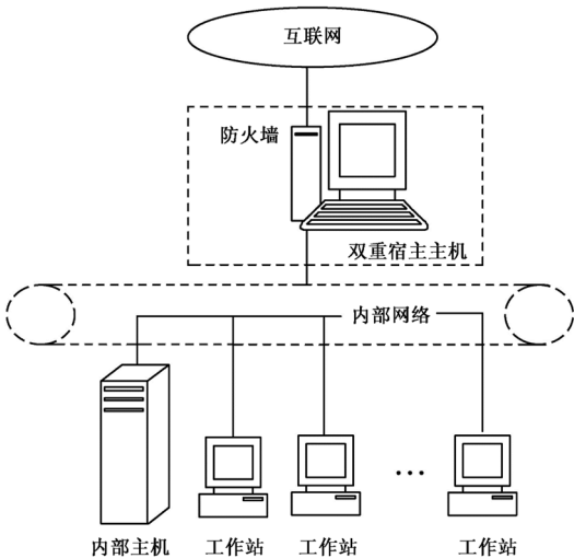
图 8-6 双重宿主主机体系结构
