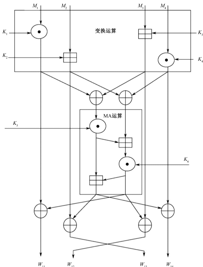
图 4-19 IDEA 一个单循环的加密过程
