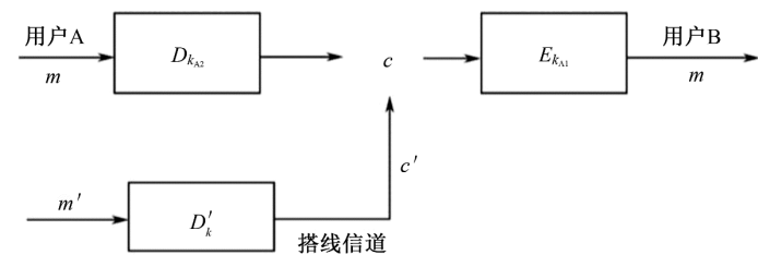
图 4-6 双钥密码认证过程
