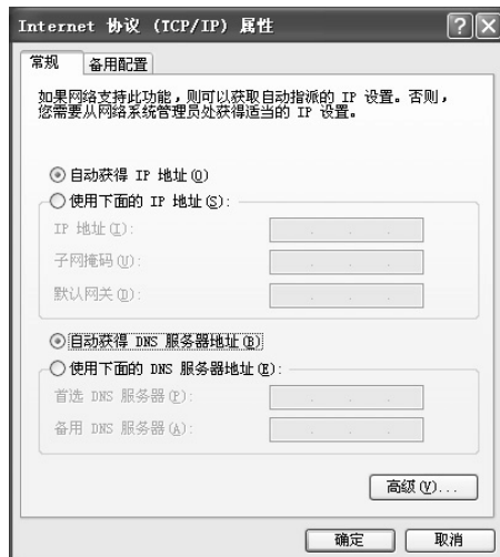
图 7-4 “Internet 协议 (TCP/IP) 属性”对话框
