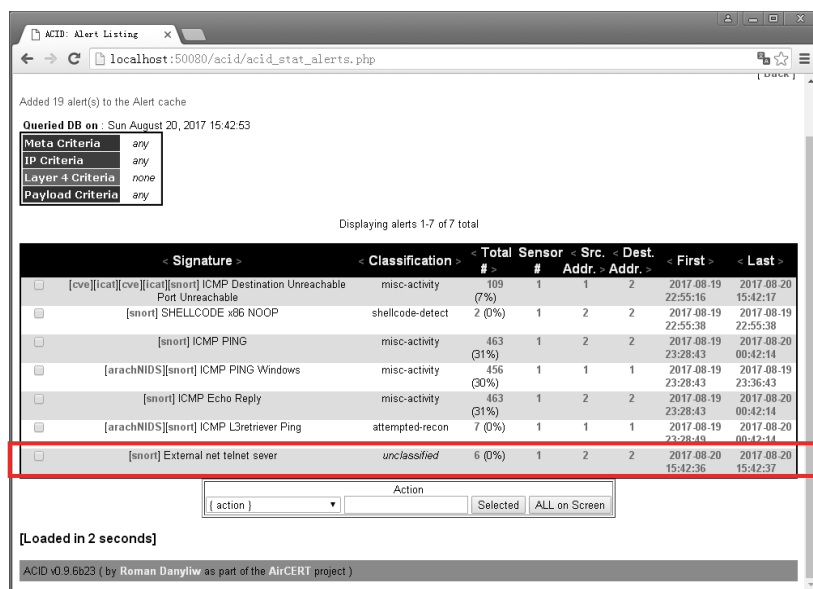
图 9-13 snort 中对 Telnet 连接的警告
