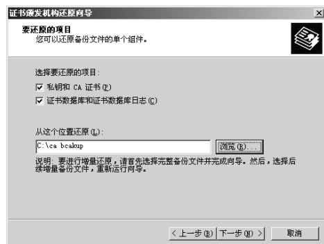
图 5-21 还原 CA
