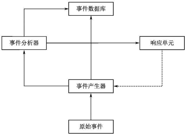
图 9-2 CIDEF 模型
