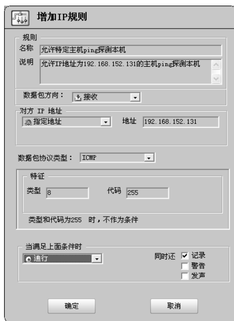
图 8-14 自定义 IP 规则配置
