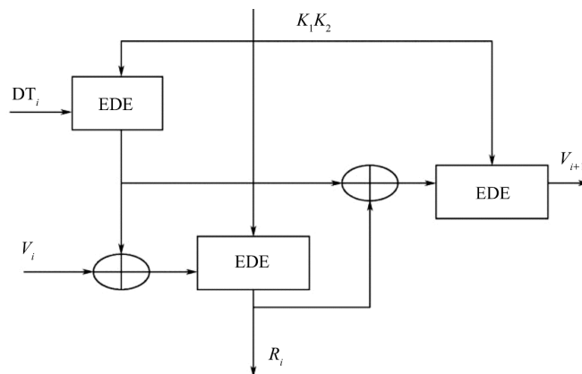
图 4-20 ANSI X9.17 算法结构
