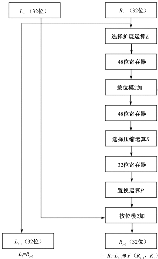
图 4-10 乘积变换框图
