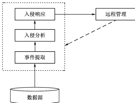
图 9-3 入侵检测系统的功能结构
