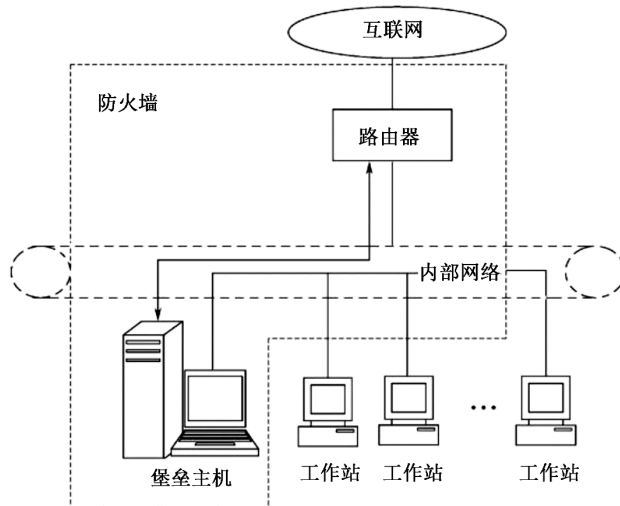
图 8-7 主机过滤体系结构
