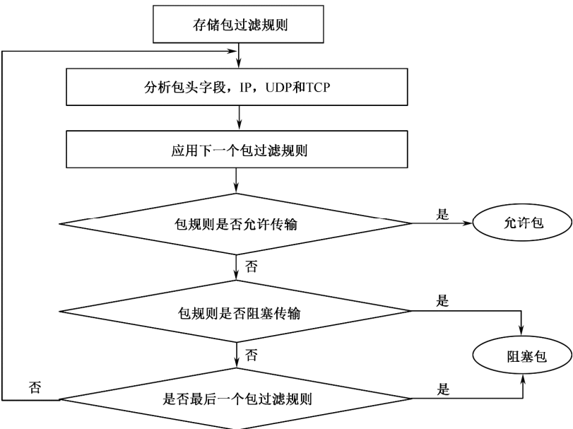
图 8-2 包过滤操作流程图
