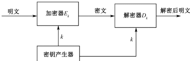
图 4-2 单钥密码系统
