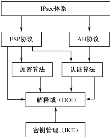
图 10-3 IPsec 体系结构
