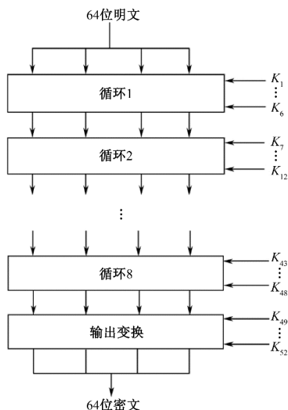
图 4-18 IDEA 加密过程
