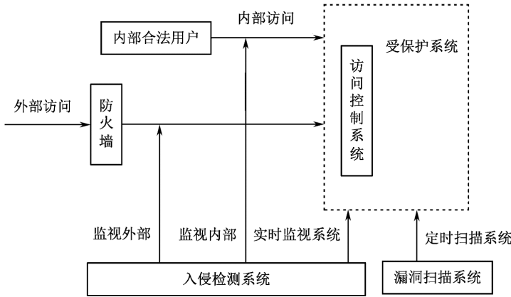
图 9-1 入侵检测系统的作用
