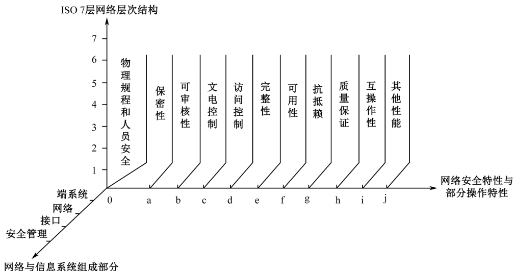
图 2-3 DISSP 的安全体系结构框架
