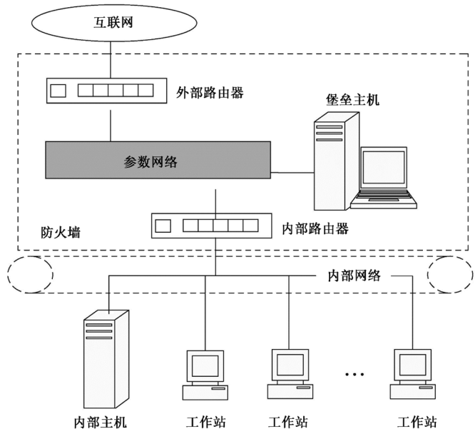
图 8-8 子网过滤体系结构
