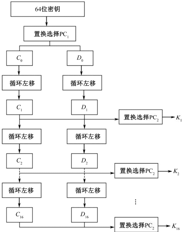
图 4-14 子密钥的生成过程
