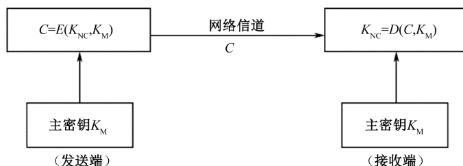
图 4-22 二级密钥的网络分配过程
