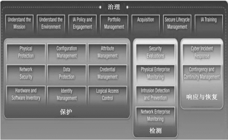
图 2-8 CGS 2.0 框架
