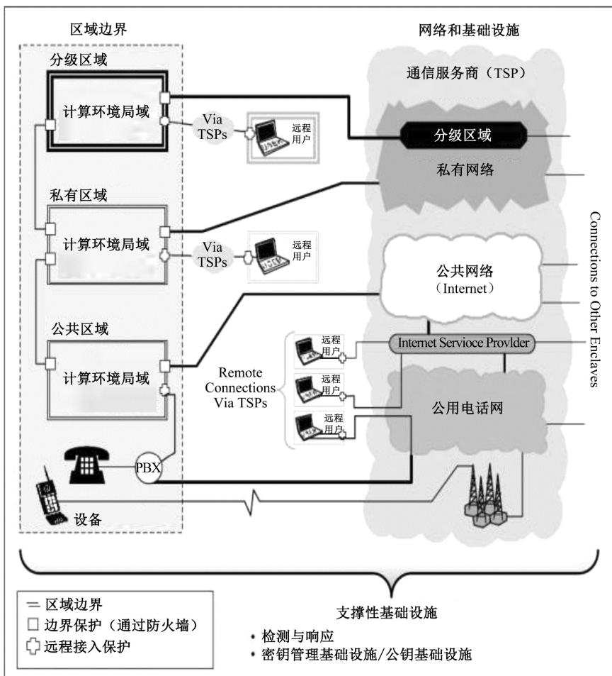
图 2-6 IATF 焦点域
