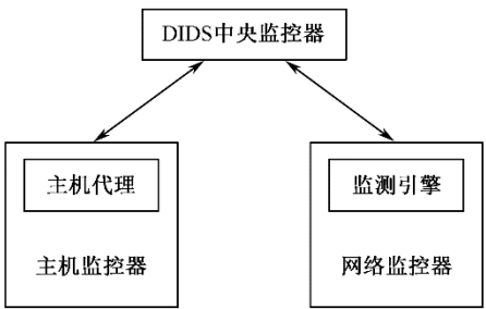
图 9-6 DIDS 结构
