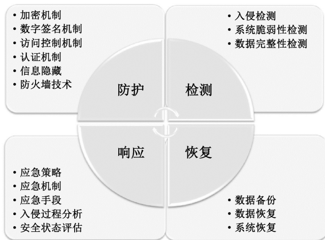
图 2-4 PDRR 模型
