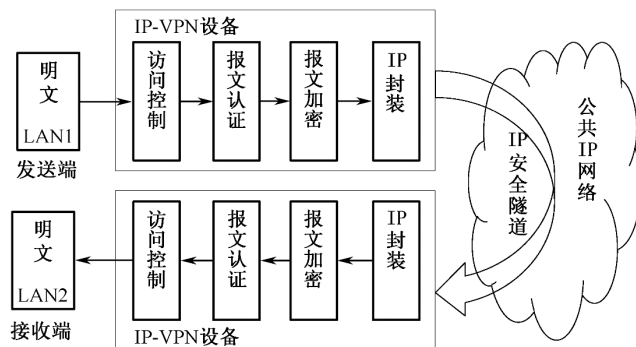
图 10-1 VPN 技术基本原理
