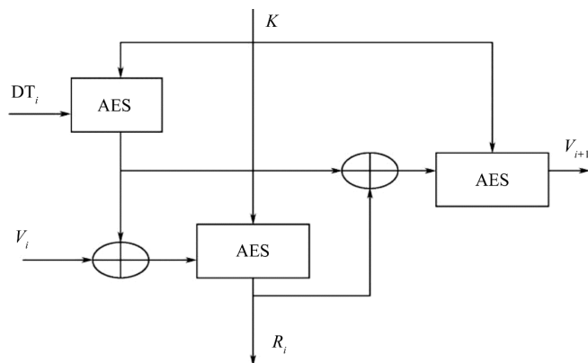
图 4-21 新的随机数产生算法
