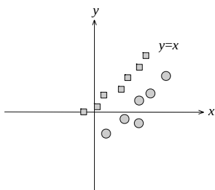
图 3-3 y = x 不能对数据点进行划分的示例
