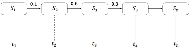
图 12-2 马尔科夫过程示例
