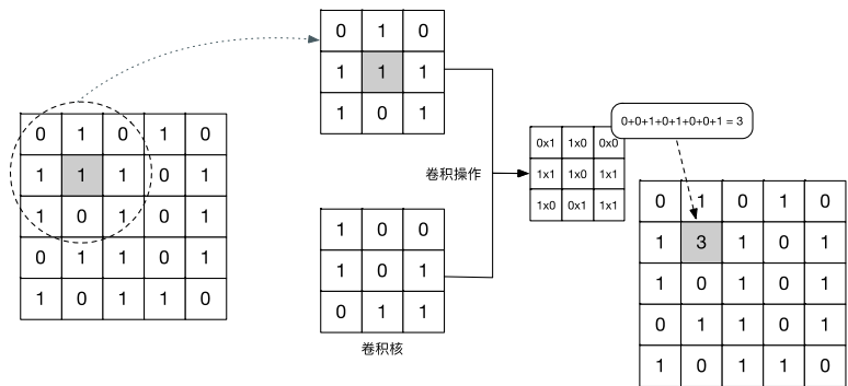
图 8-7 卷积操作的示例
