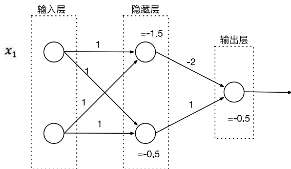
图 5-7 异或问题的解决示例
