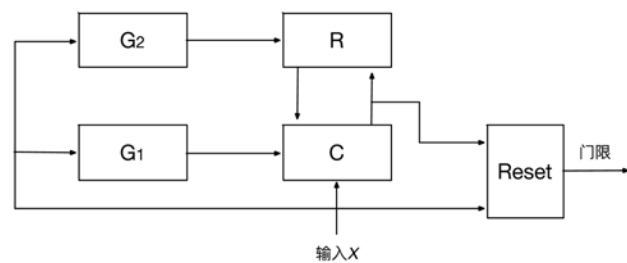
图 7-6 ART I 型网络的基本结构示例
