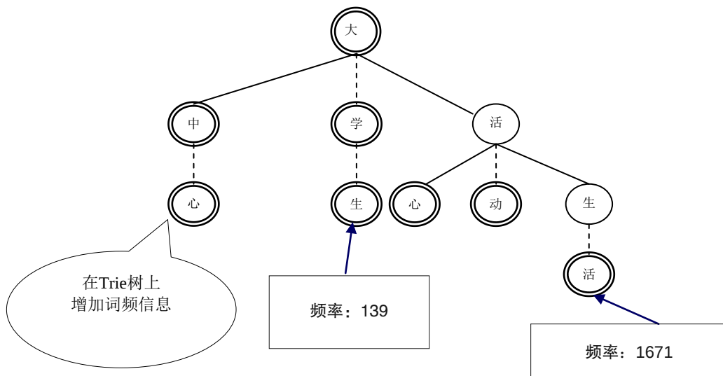
图 2-17 一元词典 Trie 树
