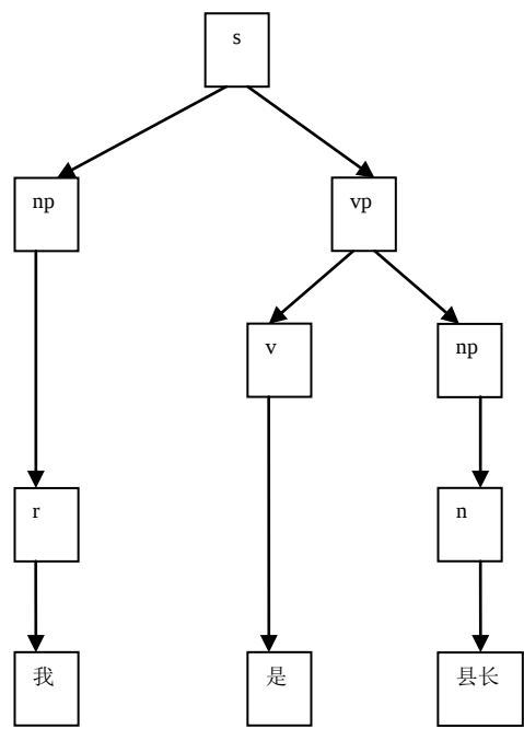
图 4-2 短语结构的句法树
