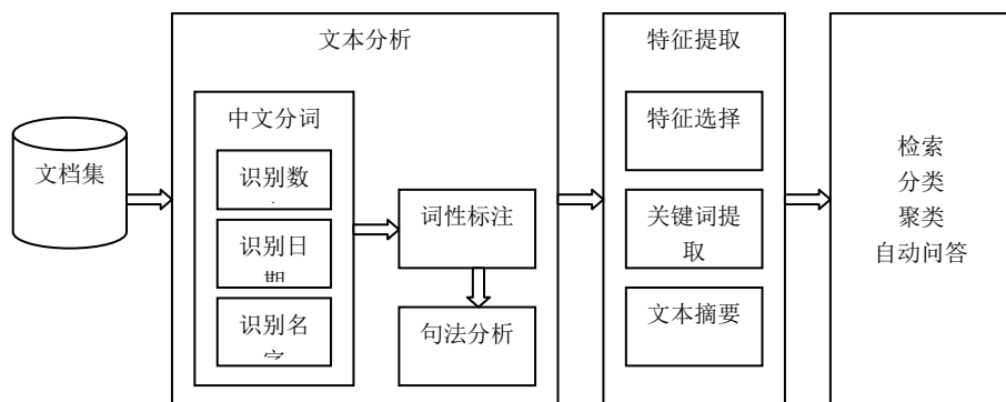
图 1-2 文本挖掘相关技术的结构
