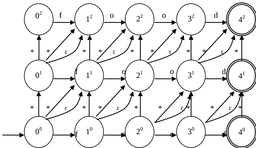
图 6-2 编辑距离自动机
