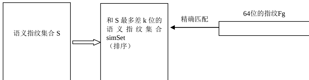
图 5-7 生成法查找近似语义指纹
