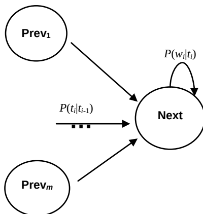
图 2-38 寻找当前节点的最大概率
