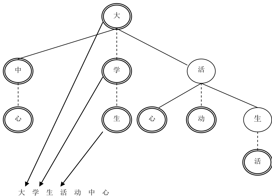
图 2-16 用三叉树全切分字符串
