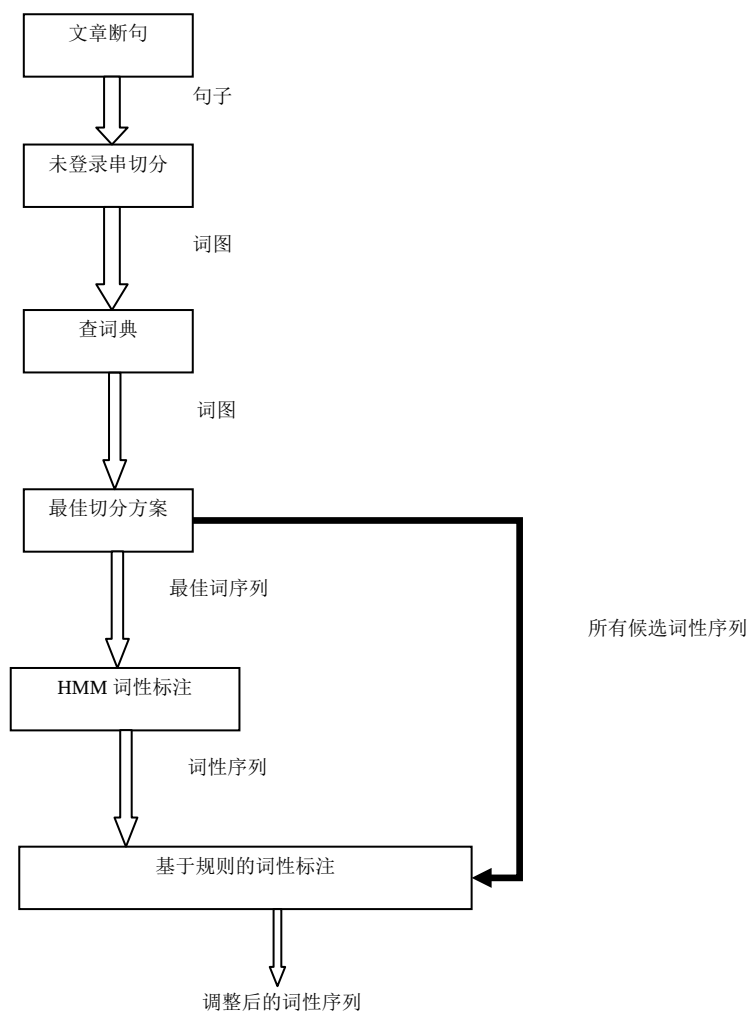
图 3-1 英文分词流程图
