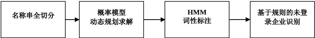
图 2-53 企业名分词流程
