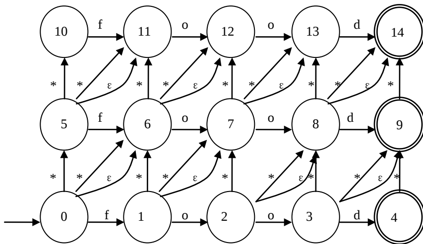
图 6-3 编辑距离自动机中的状态编号
