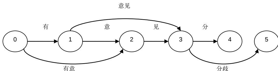
图 2-13 中文分词切分词图
