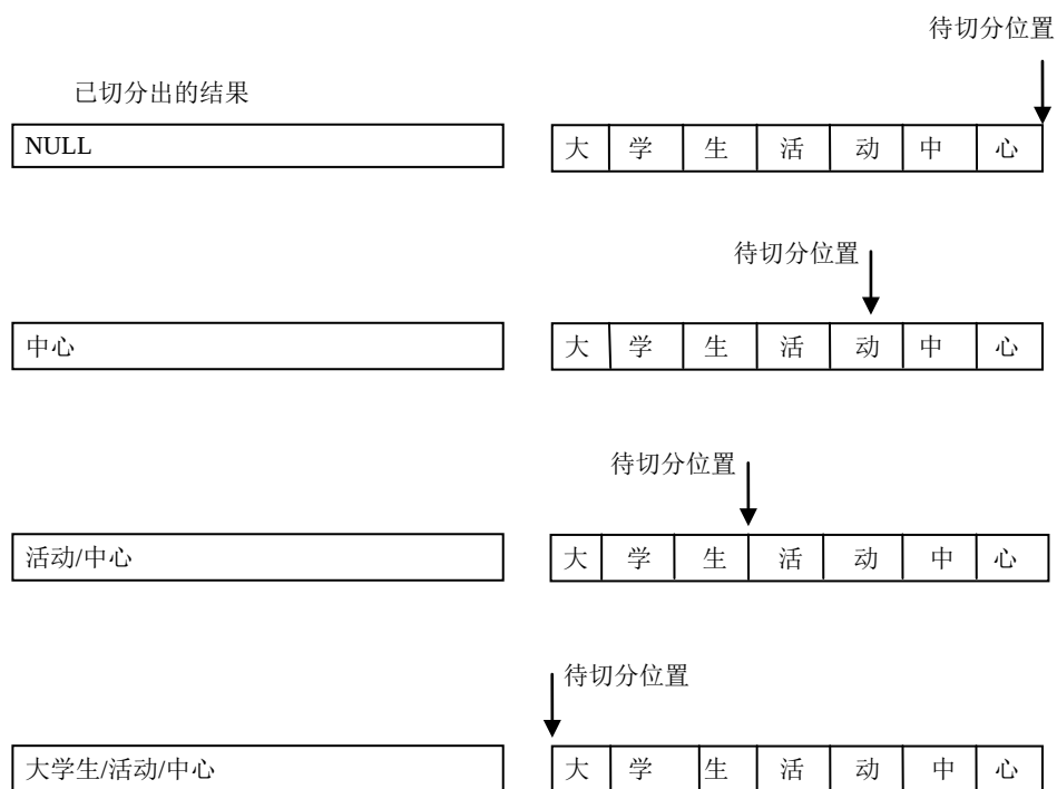
图 2-9 逆向最大长度匹配切分过程
