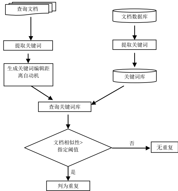
图 5-3 关键词排重流程
