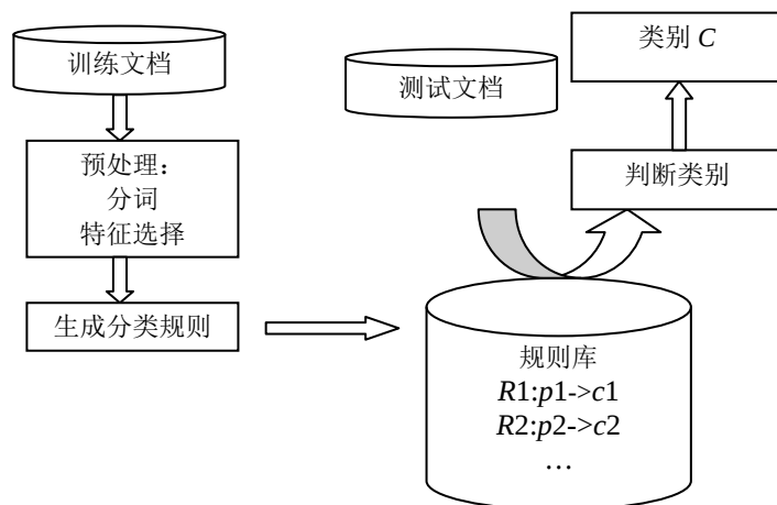
图 8-6 基于规则的文本分类流程图
