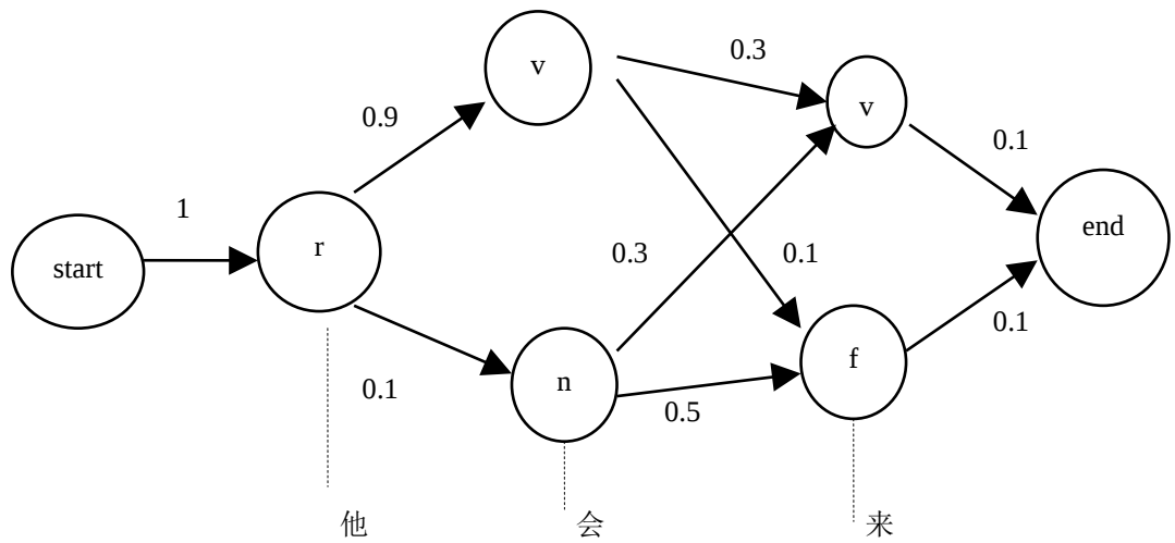
图 2-34 “他/会/来”的转移概率图
