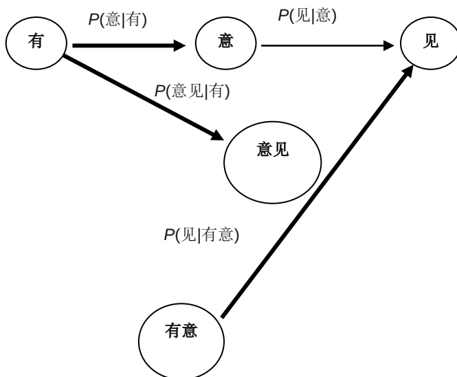
图 2-26 节点“见”的最佳前驱节点是节点“有意”
