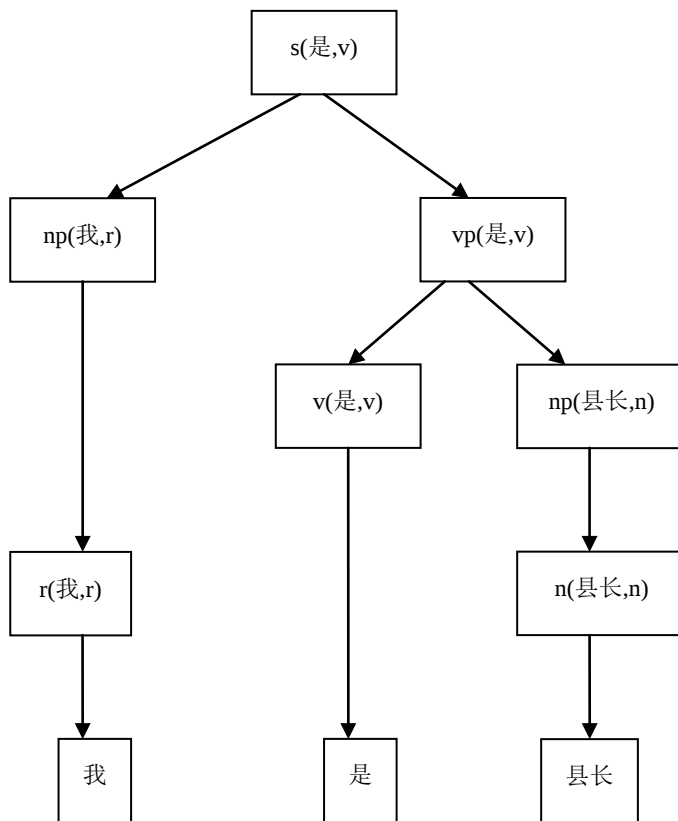
图 4-3 词汇化的句法树
