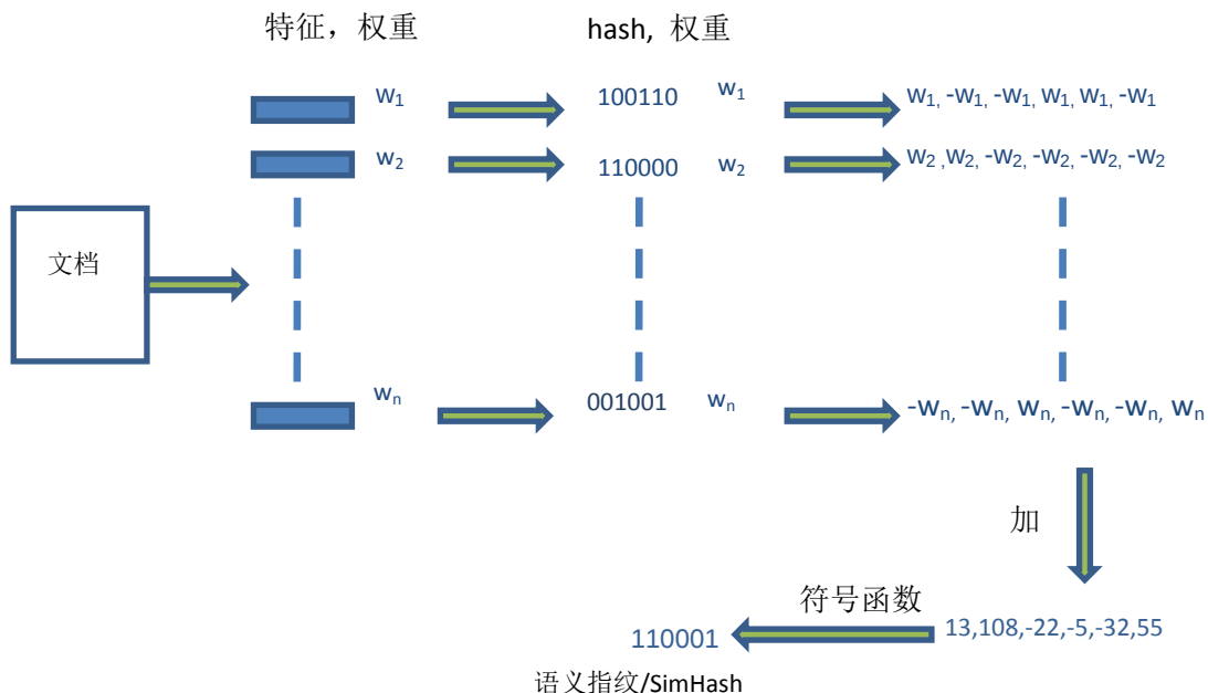
图 5-4 语义指纹计算过程
