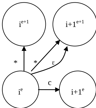
图 6-4 编辑距离自动机中的状态转换
