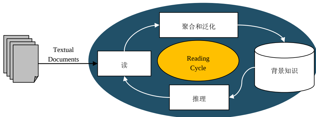
图 10-7 机器阅读
