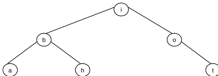
图 2-4 二叉搜索树
