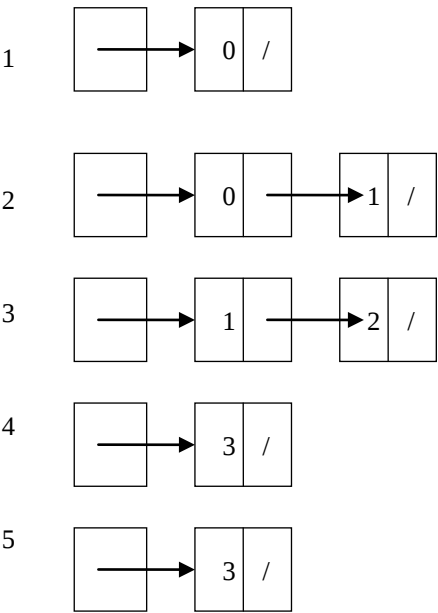
图 2-14 逆邻接表
