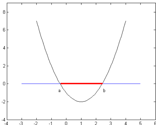
图 8-5 二次判别函数
