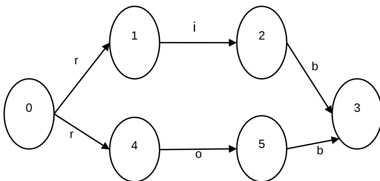
图 2-42 标注图
