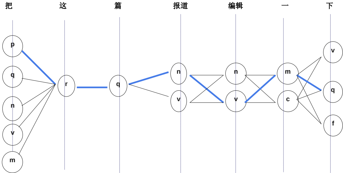
图 2-32 词性标注
