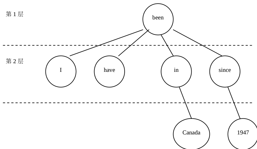
图 4-9 依存树
