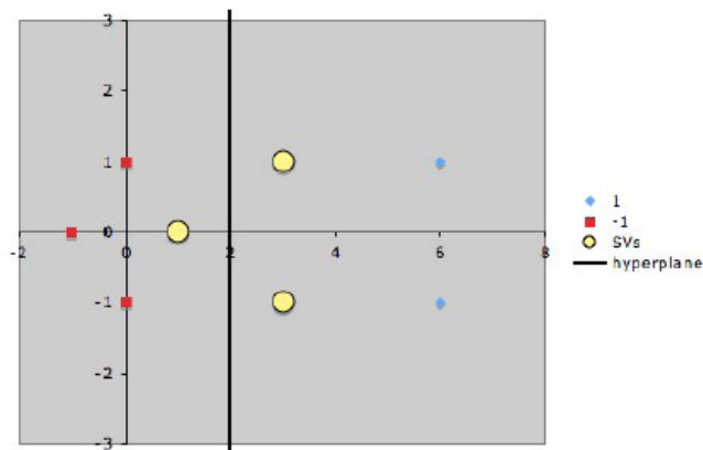
图 8-3 超平面
