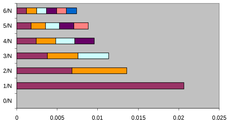
图 2-49 词的概率图
