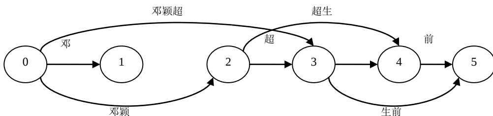
图 2-48 人名词图
