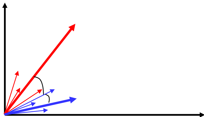
图 5-1 向量的夹角
