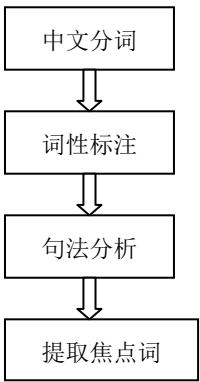
图 10-1 问句分析
