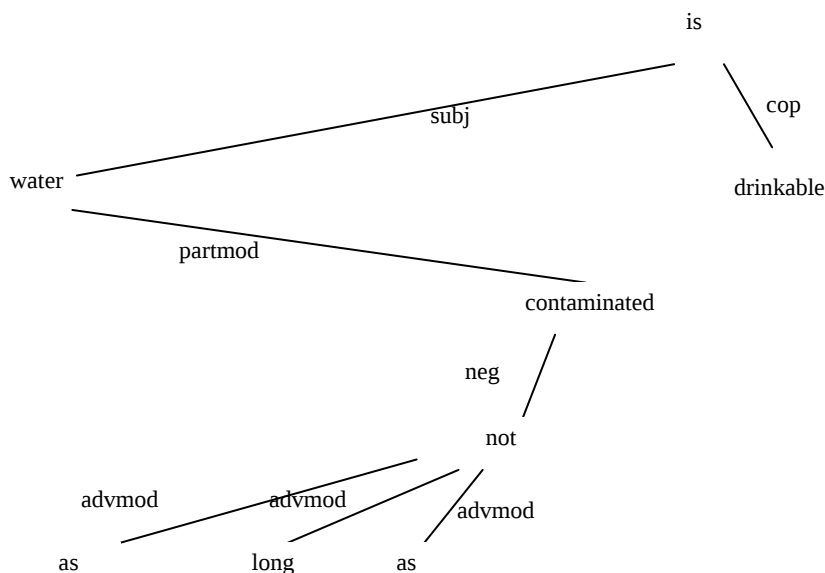
图 4-8 英文依存树
