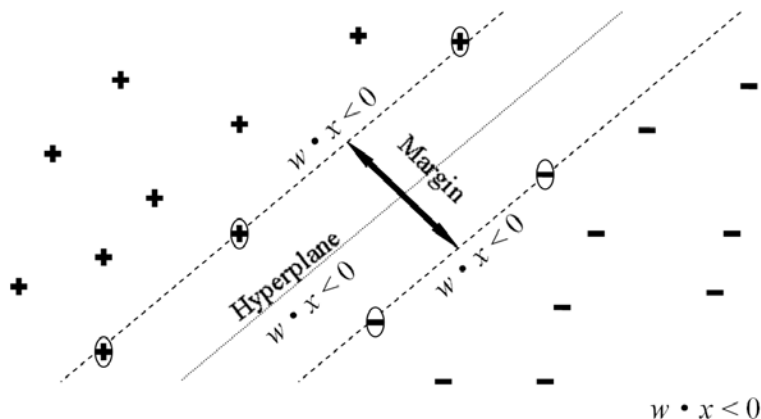
图 8-1 分类间隔
