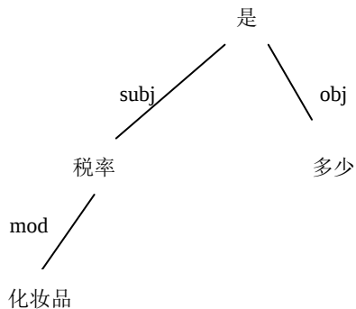
图 10-3 依存树举例
