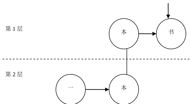
图 4-6 中文依存树
