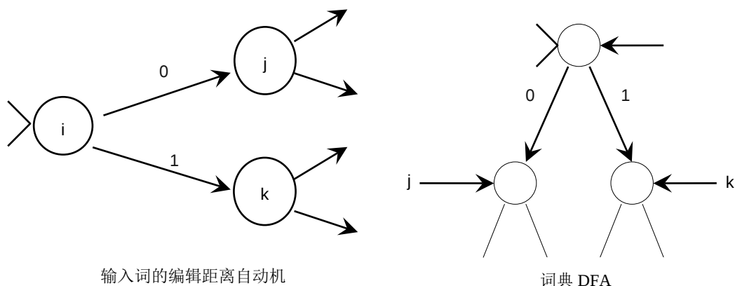
图 6-5 DFA 取交集
