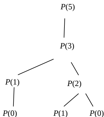
图 2-11 最大概率问题分解图
