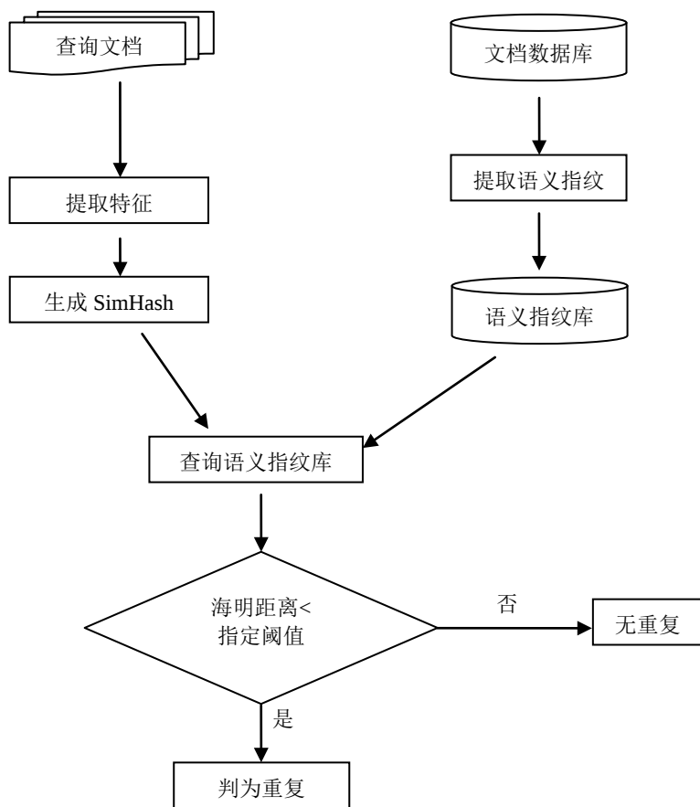
图 5-5 文档排重计算过程
