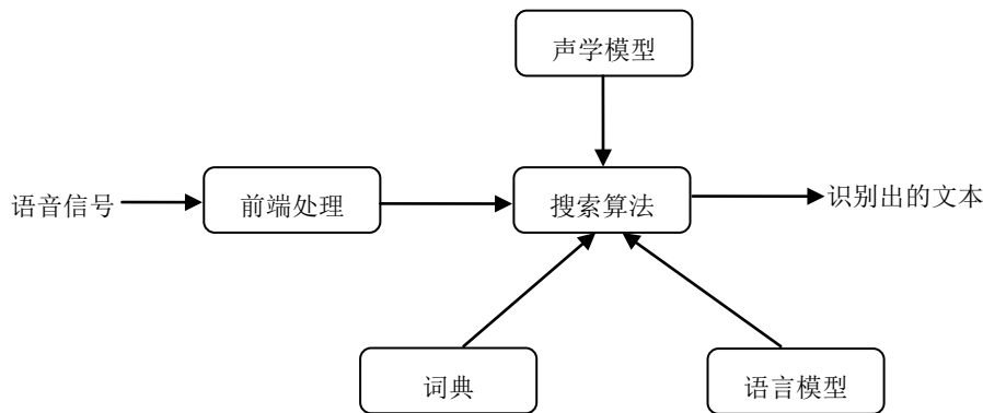
图 11-1 语音识别结构
