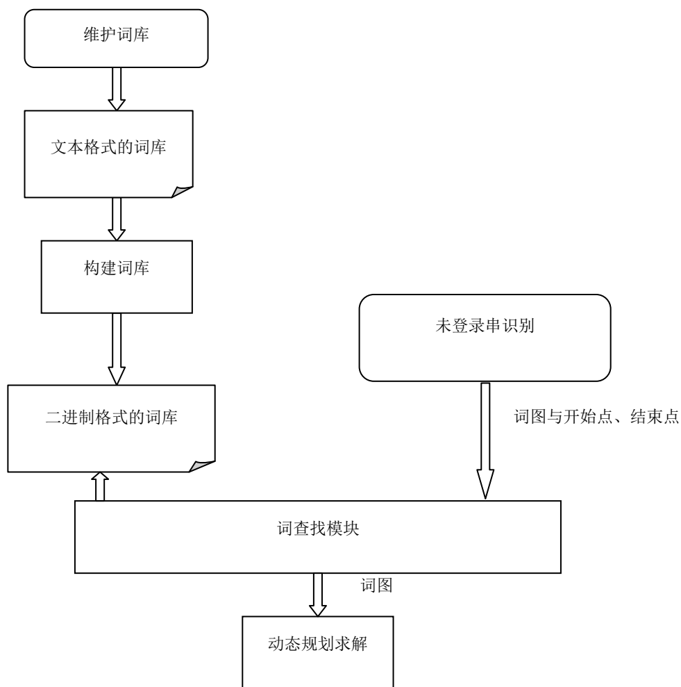
图 2-19 扩展的中文分词结构图
