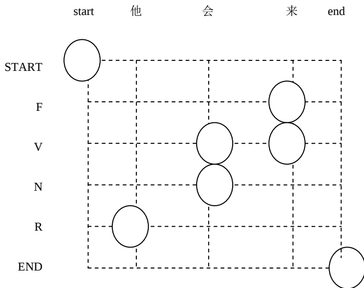
图 2-36 维特比求解格栅
