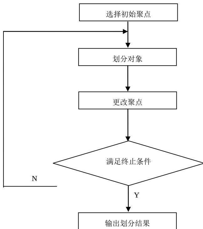
图 8-7 K 均值算法流程图
