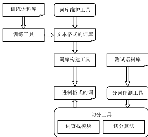
图 2-8 中文分词结构图
