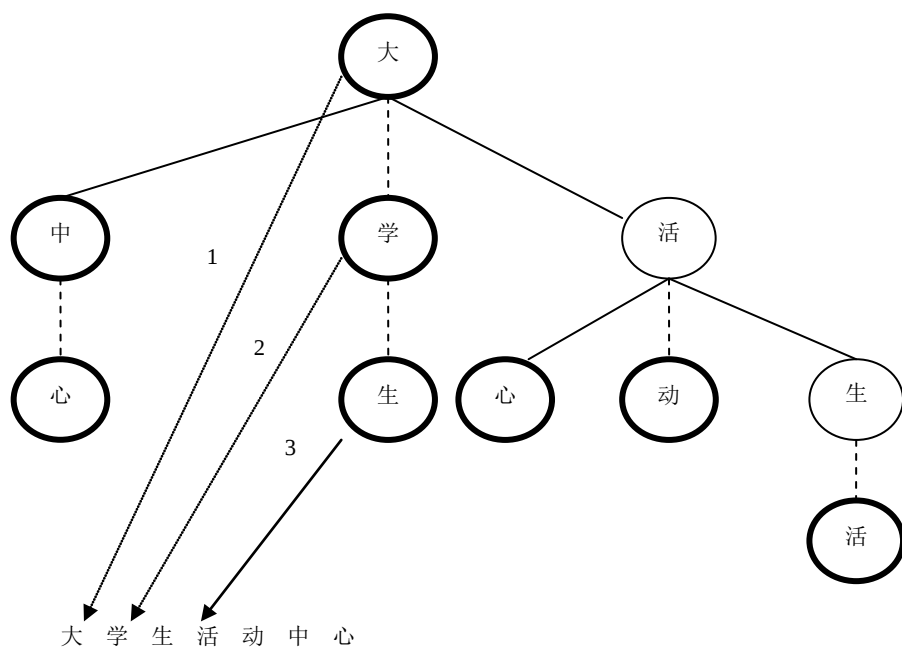
图 2-8 找最长匹配词
