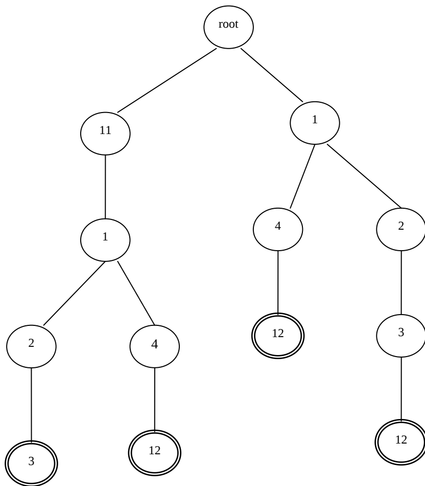
图 2-46 人名识别规则组成的标准 Trie 树
