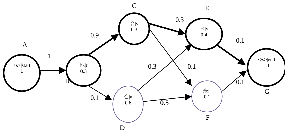
图 2-39 维特比求解过程
