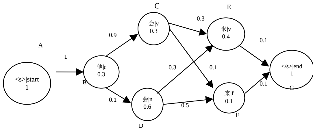
图 2-35 “他/会/来”的转移概率加发射概率图
