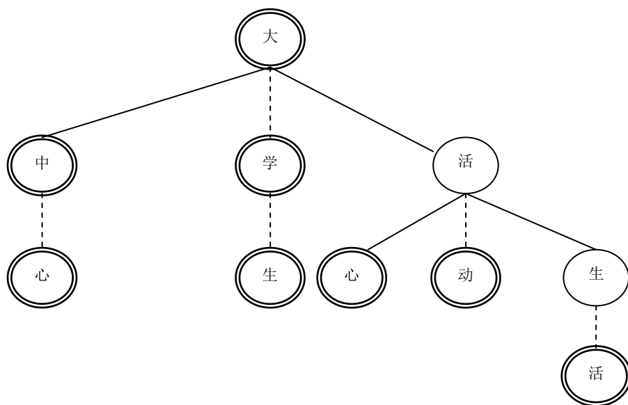
图 2-7 三叉树
