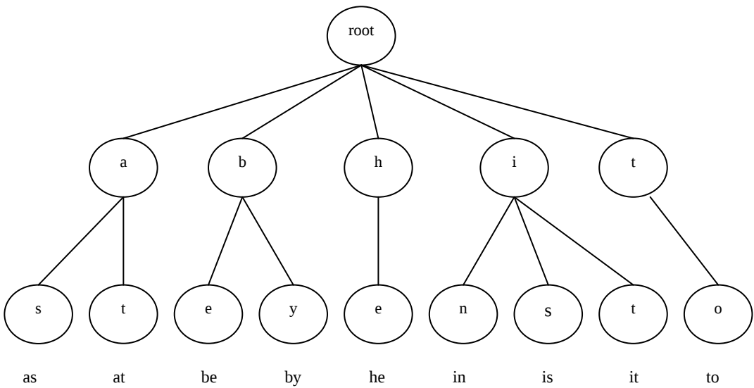
图 2-3 标准 Trie 树
