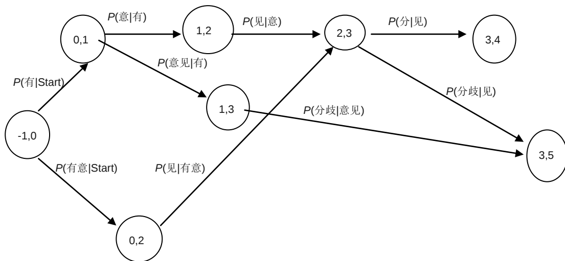
图 2-23 二元词图
