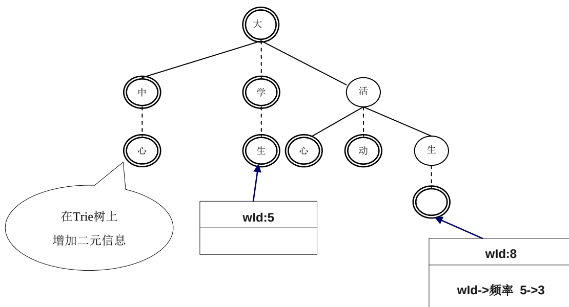
图 2-20 词典 Trie 树
