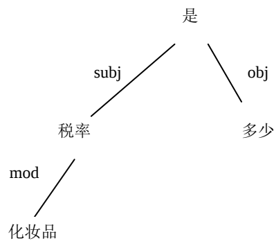
图 10-8 依存树举例
