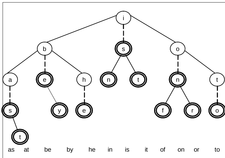
图 2-5 三叉树
