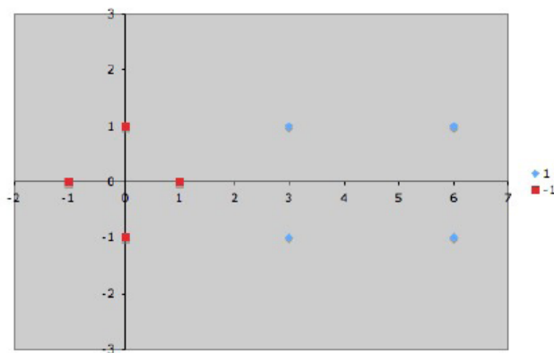
图 8-2 二维空间中的样本点
