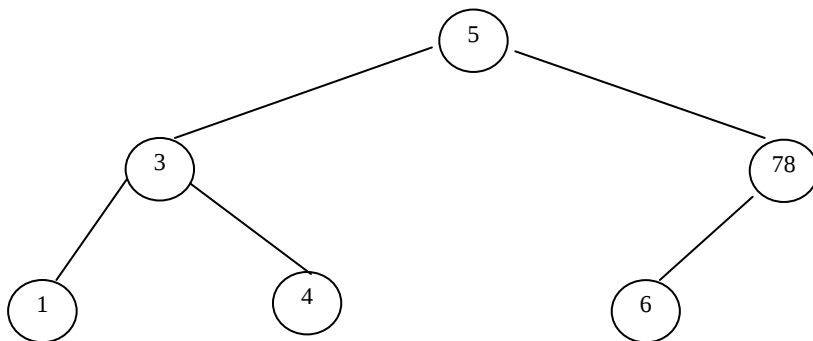
图 2-21 完全二叉树
