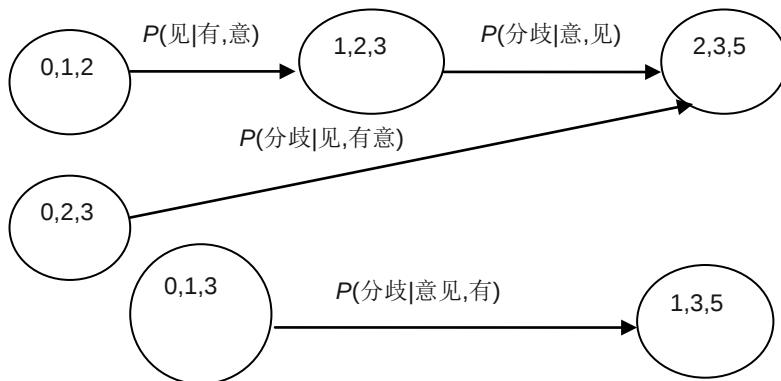
图 2-28 词表示的三元切分词图
