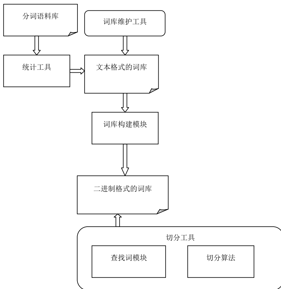
图 2-18 中文分词结构图
