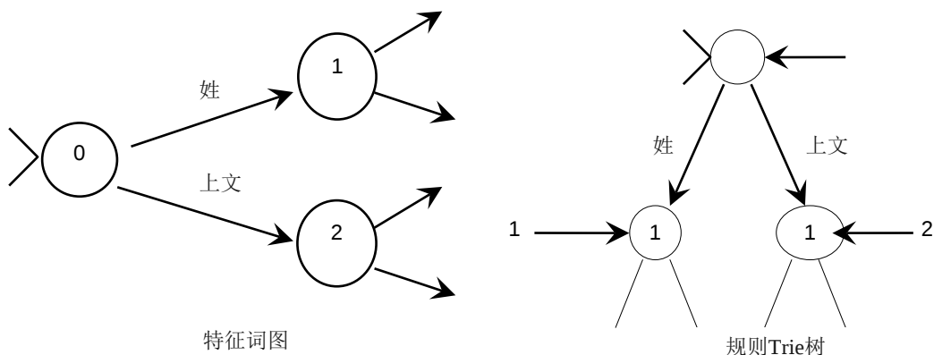
图 2-47 从人名特征词图上找匹配规则
