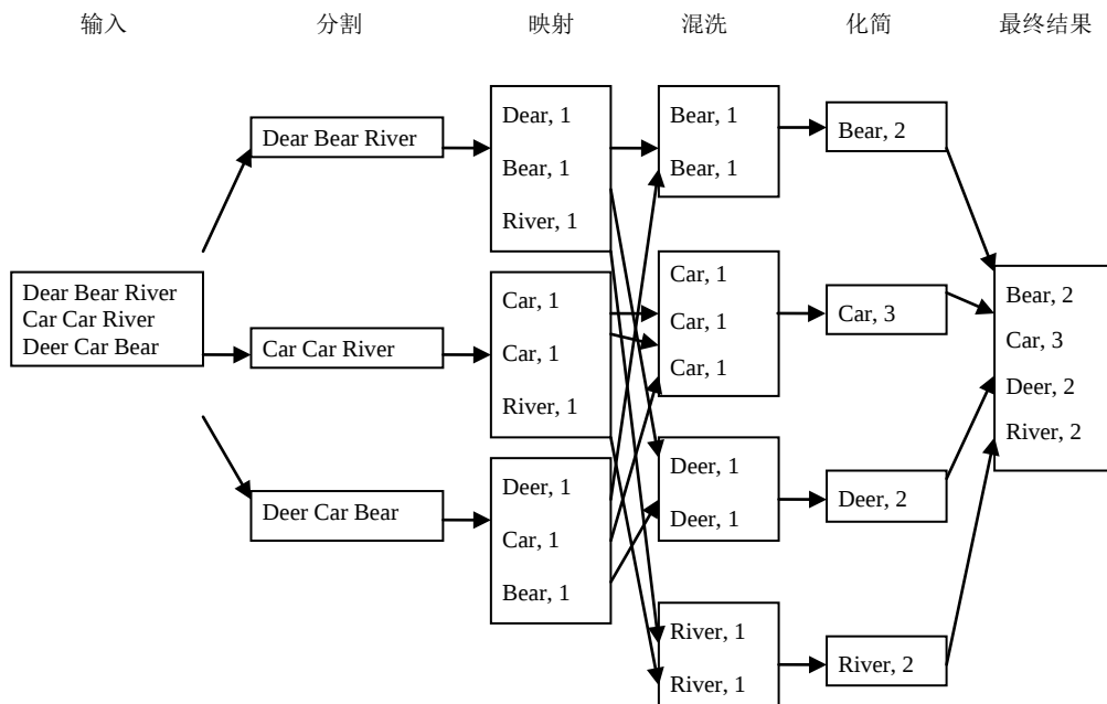
图 1-1 统计词频的例子
