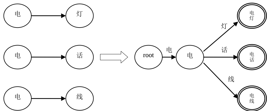
图 2-2 从链表到 Trie 树
