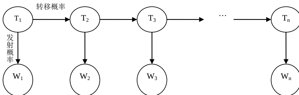
图 2-33 词性标注中的隐马尔可夫模型
