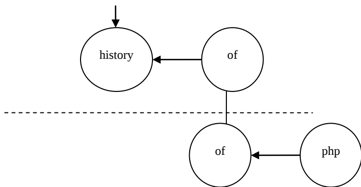
图 4-10 “history of php”依存树
