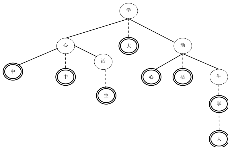
图 2-10 逆 Trie 树词典
