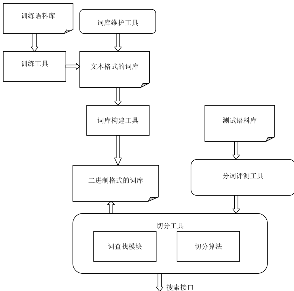
图 2-29 中文分词结构图
