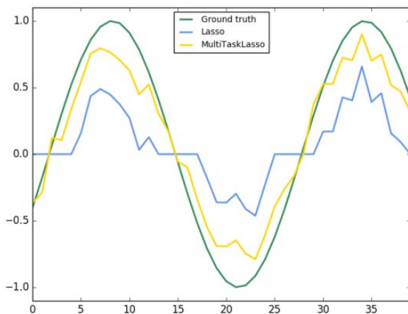
图 6-3 多任务 LASSO 回归算法
