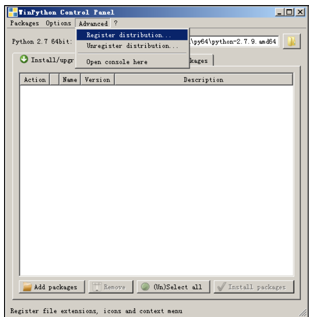
图 2-14 系统关联
