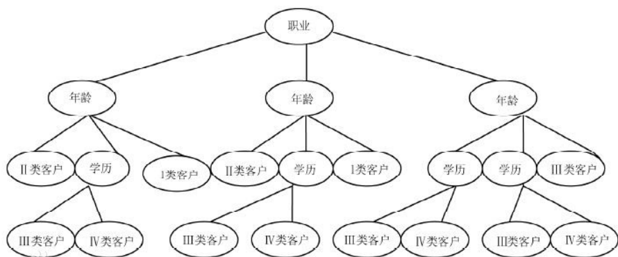
图 7-1 决策树算法
