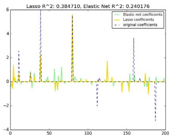
图 6-2 最小绝对值收缩和选择算法
