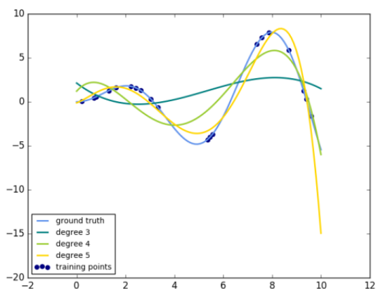
图 6-16 多项式函数回归算法
