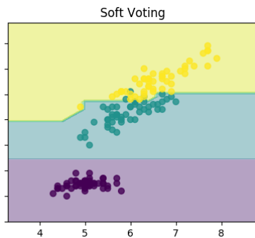
图 6-34 投票算法
