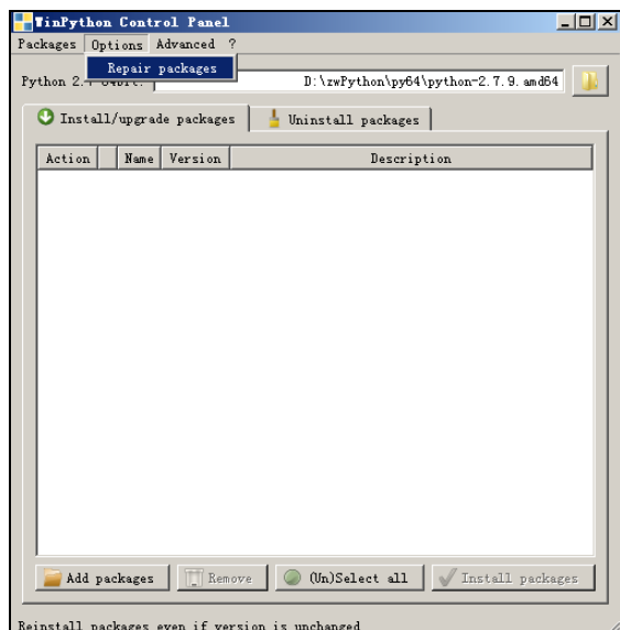
图 2-13 模块库维护
