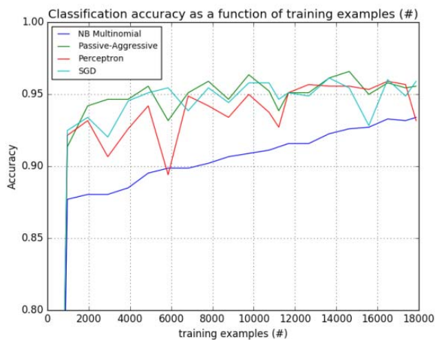
图 6-11 感知器算法
