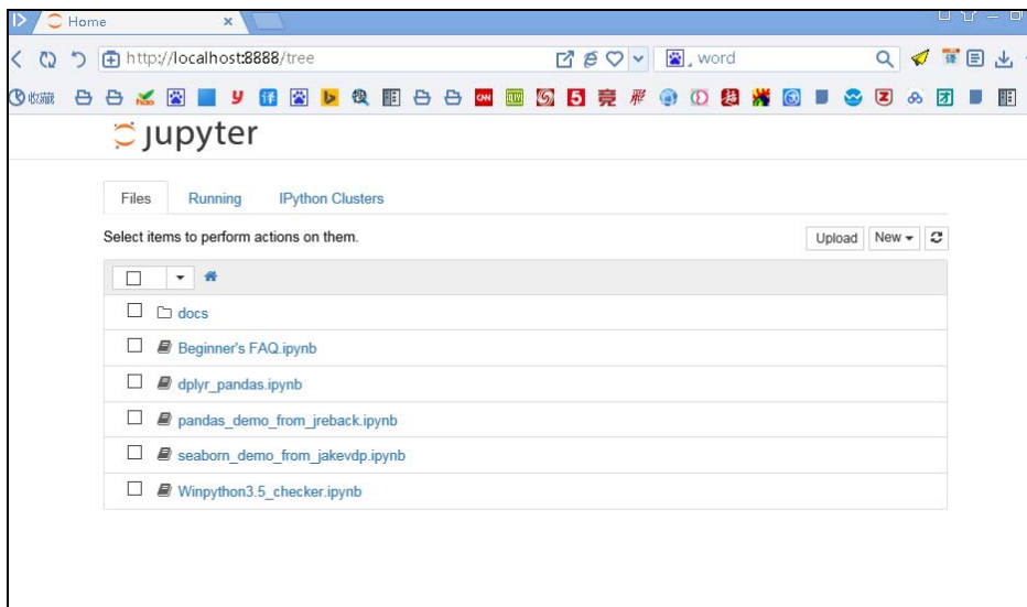
图 2-10 Notebook 模式
