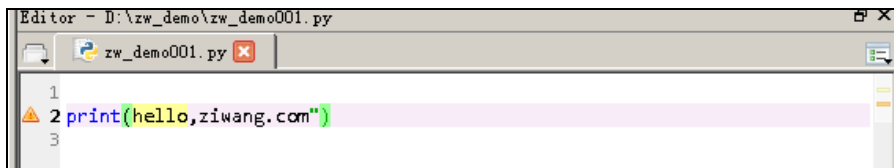
图 3-2 修改代码
