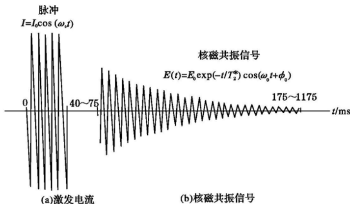
图 2 核磁共振激发和接收到的信号
