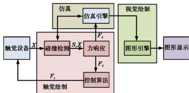
图3 触觉绘制系统结构
