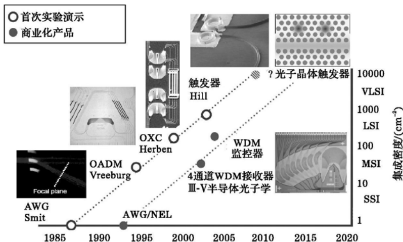
图 2 集成光学的摩尔定律 [8]
