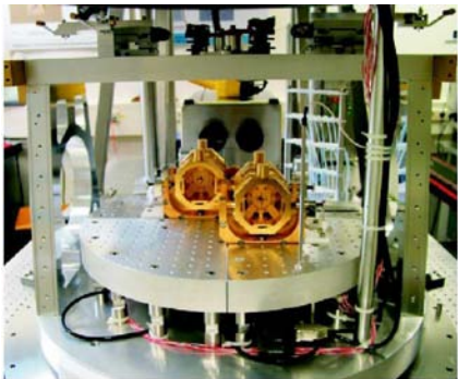
图3 德国 PTB 的纳牛力值标准装置
