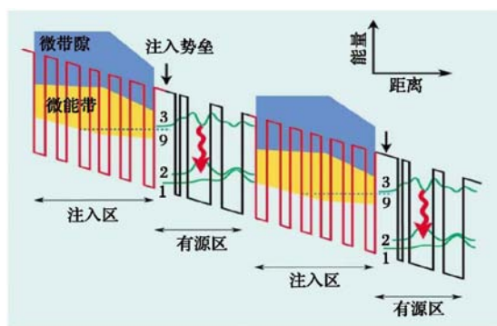
图 3 量子级联激光器中的量子设计和能级示意图
