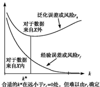
图 1 经验风险与泛化风险
