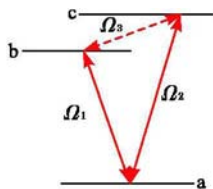
图1 红宝石 V 型三能级结构示意图
