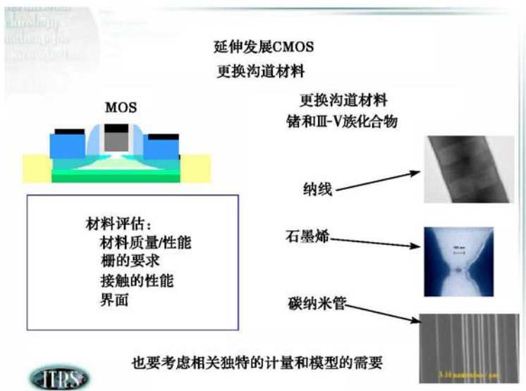
图7 改变沟道材料的方法延伸发展 CMOS [3]
