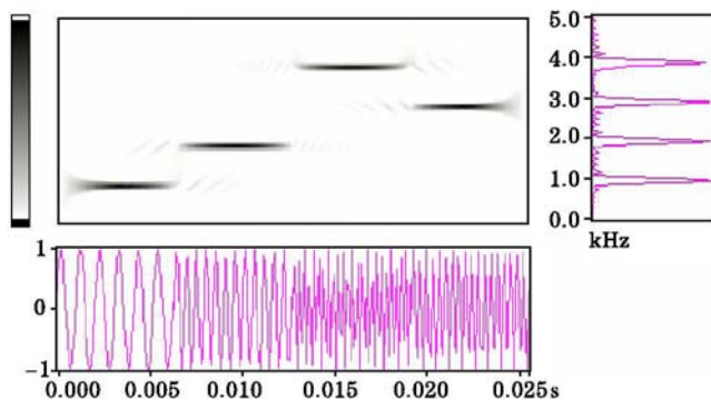
图 1 四段跳频信号的时频谱
