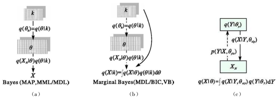
图 4 最短编码与 Bayes 方法
