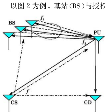
图2 认知无线电谱感知示意图
