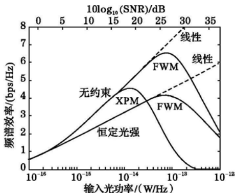
图 1 光纤非线性效应对频谱效率的限制
