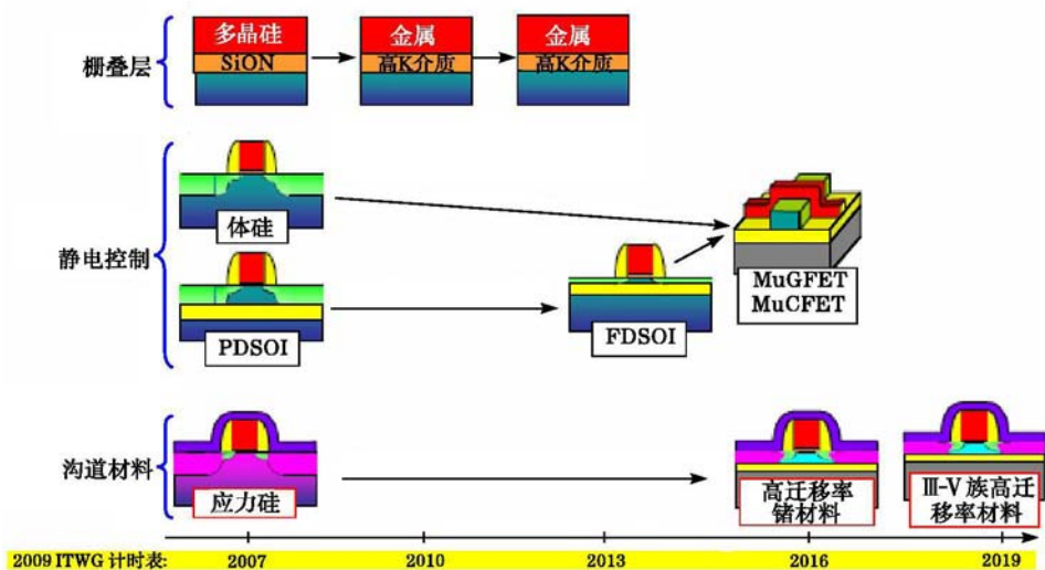
图5 等比例缩小工艺技术的发展趋势 [3]
