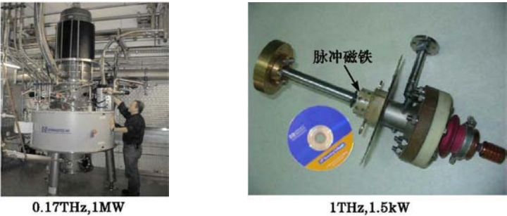
图3 太赫兹回旋管
