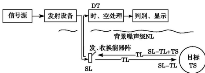
图1 主动声纳信号强度变化示意图
