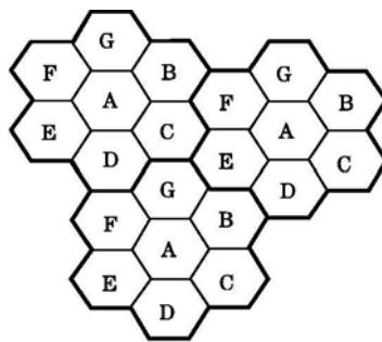
图1 蜂窝系统的小区划分
