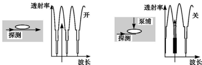
图 7 纳米硅波导环共振器全光开关工作原理
