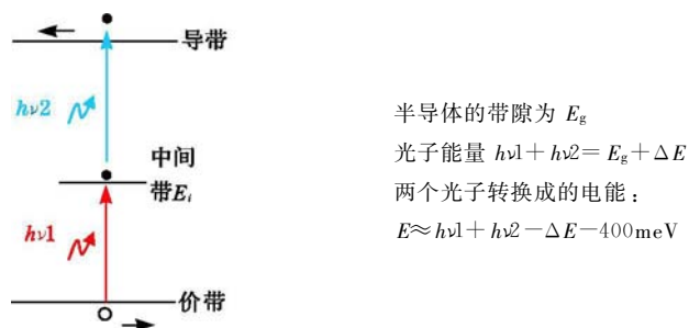
图3 半导体中间带光子级联吸收过程
