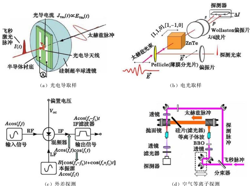
图 7 太赫兹波相干探测原理
