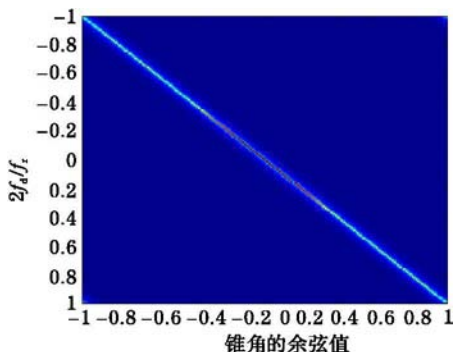
图1 单基正侧面阵雷达杂波功率谱
