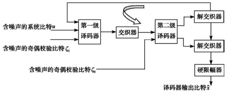
图 1 Turbo 解码器原理示意图
