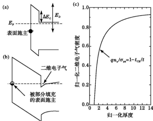
图 1 AlGaIn/GaN 异质结构表面态与二维电子气形成
