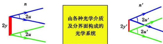
图1 光学成像系统拉赫不变量示意图
