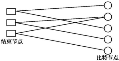
图 2 Tanner 图
