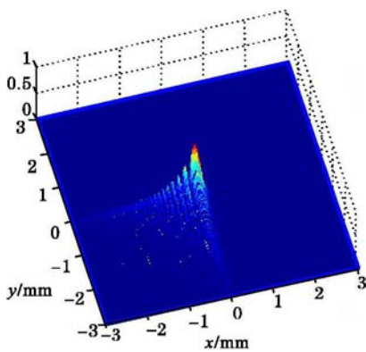
(b) Airy 无衍射光束
