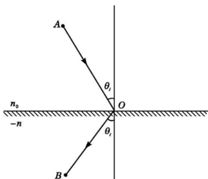
图 7 负折射现象
