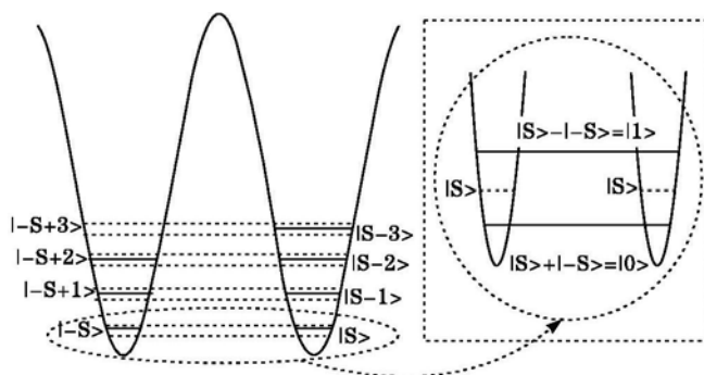
图 3 宏自旋的 S 态和 -S 态组成对称和反对称态 ( |0> 为对称态, |1> 为反对称态 )
