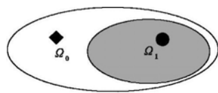
图 1 全局最优与局部最优
