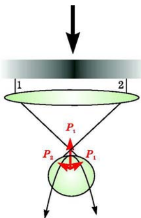
图2 光镊原理图
