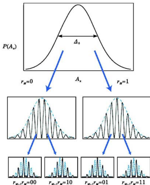
图 1 Giedke 小组的介观自旋集测量结果 [5]
