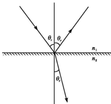
图3 光的反射定律和折射定律
