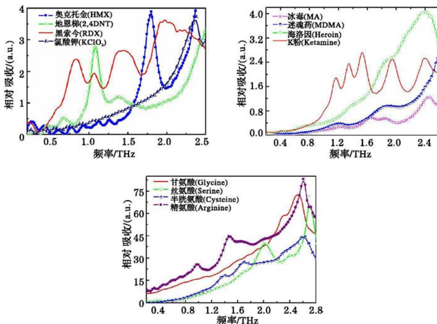
图 8 太赫兹光谱
