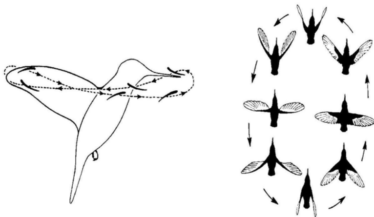
图8 蜂鸟悬停时的扑翼轨迹
