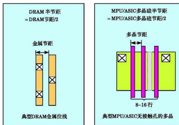
图 2 集成电路特征尺寸示意图 [3]
