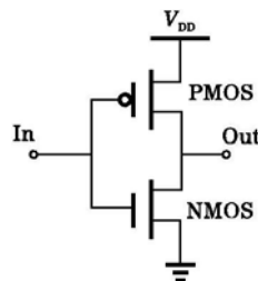
图2 CMOS反相器逻辑图
