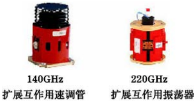
图2 太赫兹扩展相互作用速调管
