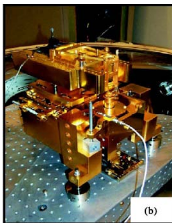
(b) 静电力天平
