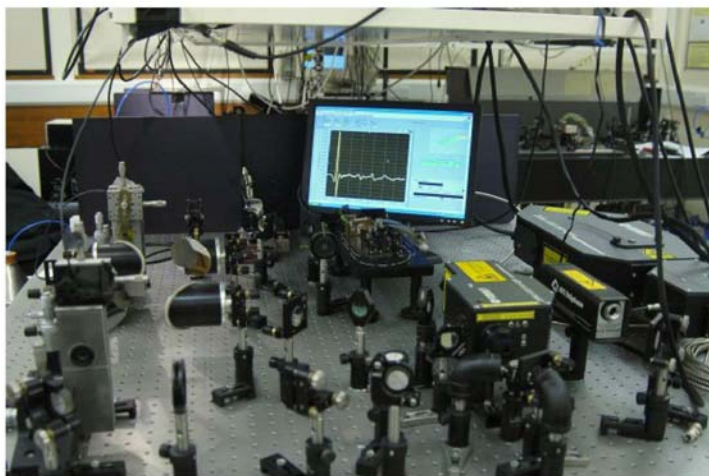
图3 太赫兹时域光谱仪 [11]
