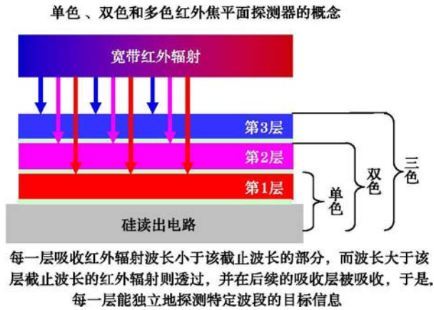
图 1 单色、双色和多色红外焦平面探测器的剖面结构与工作原理图
