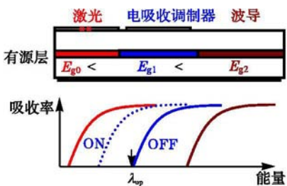
图 1 多种光子器件单片集成及激光器、电吸收调制器和波导的吸收带示意图
