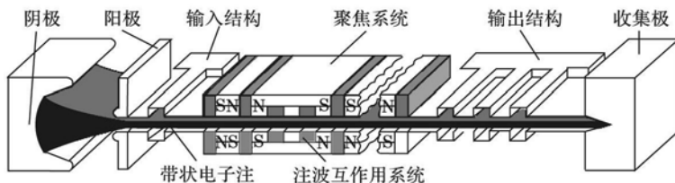
图 1 带状电子注真空电子器件示意图
