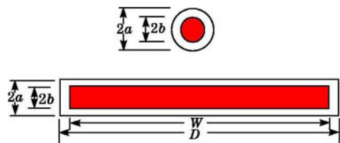
图 2 圆柱状电子注与带状电子注截面比较示意图
