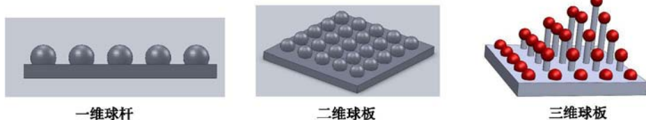
图 1 构想中为校正测量精度所设计的空间标准件
