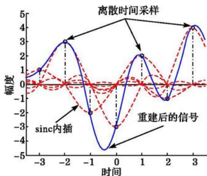
图 1 利用 sinc 函数重建连续信号
