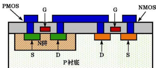
图1 CMOS工艺示意图
