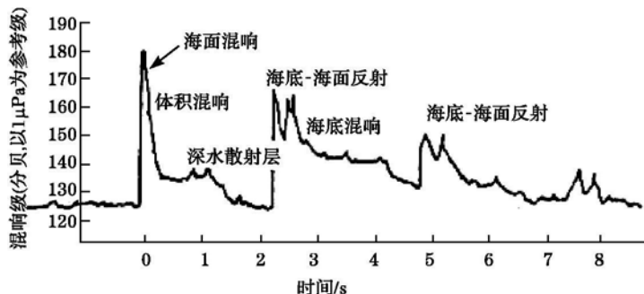
图4 水听器测得的海水混响
