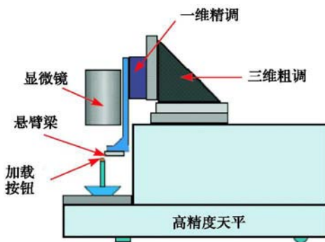
图4 韩国 KRISS 的原子力显微镜悬臂梁校准系统
