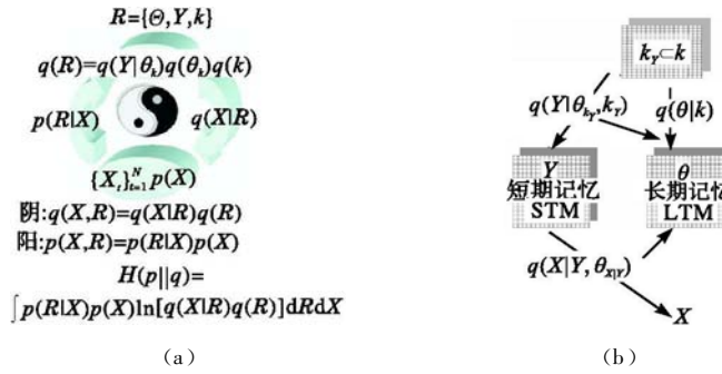
图 5 BYY 系统与最大和谐原理
