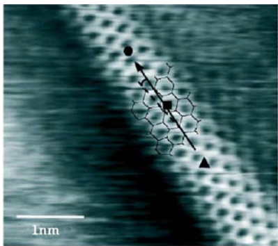
图1 扫描隧道显微镜观测到的碳纳米管原子结构 [3]
