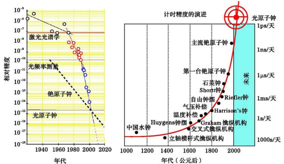
(a) 光频率标准精度的发展和微波频标的对比
