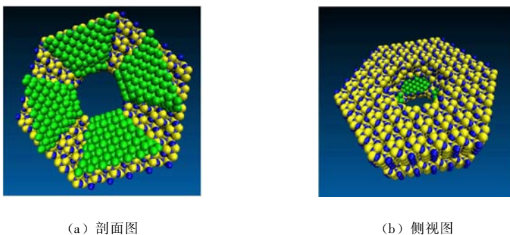
图 3 绝缘层-电极-绝缘层三明治结构的纳米孔
