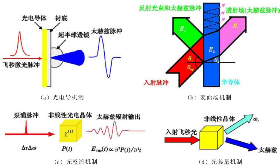
图 4 太赫兹波光学产生方法
