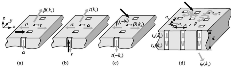
图1 综合考虑一维孔链的基本散射过程建立光学异常透射的金属表面等离子模型 [5] (a)~(c)中的入射波(黑色箭头)依次为金属表面等离子体波、孔链基模、入射平面波
