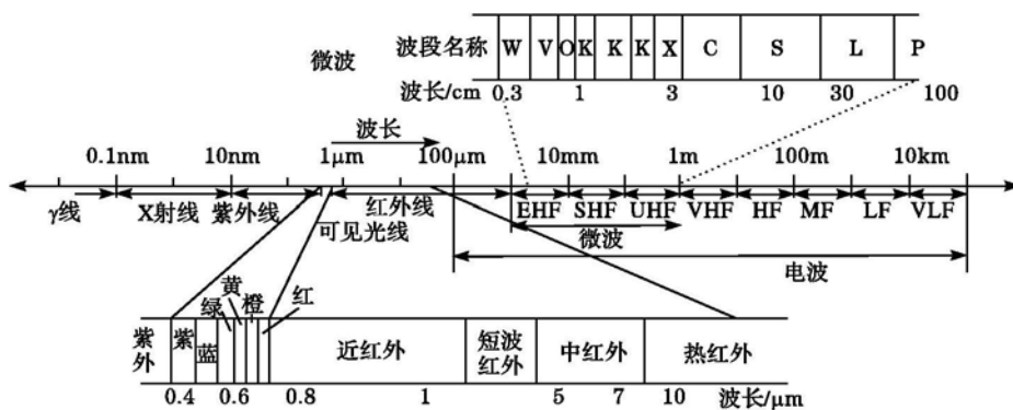
图 1 电磁波谱图
