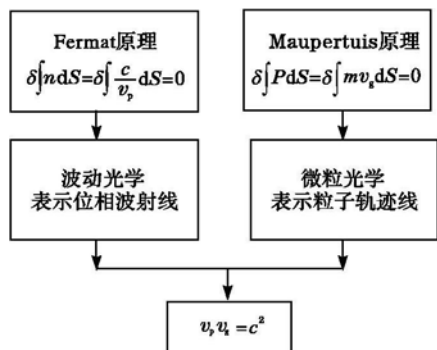
图5 两种极值原理对应两种不同光速
