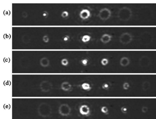
图3 利用旋涡光栅探测光学旋涡(拓扑指数为 -4, -2, 0, +2, +4 )的实验结果 [7]
