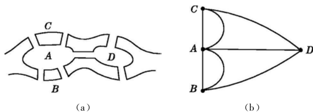
图 4 七桥问题及其对应网络图
