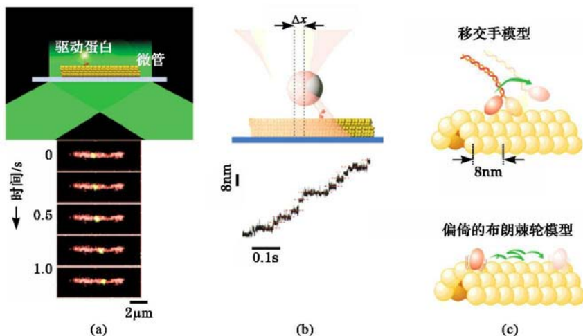
图 5 光镊研究驱动蛋白马达沿微管运动 [3]
