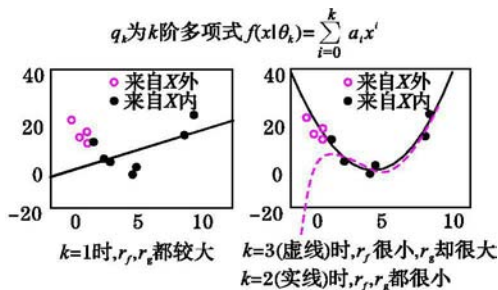
图 2 多项式曲线拟合
