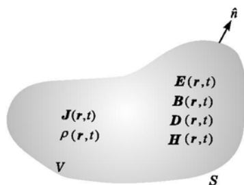
图 10 电磁最小作用量问题
