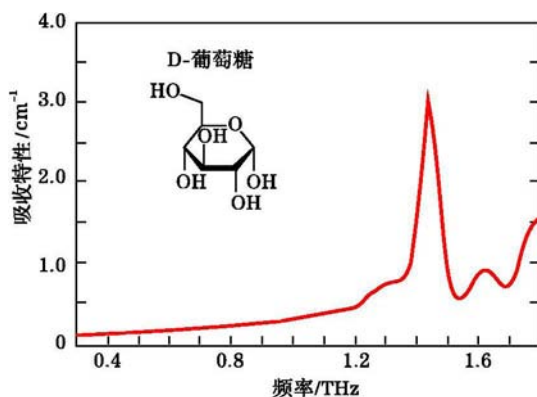
图5 D-葡萄糖 [14]
