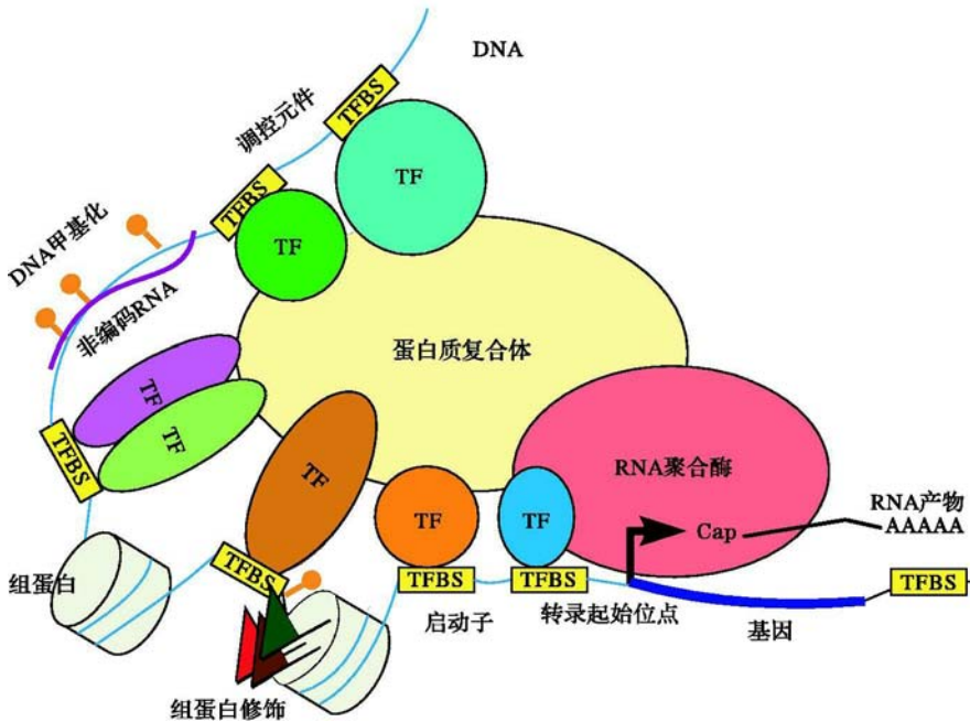
图 1 基因转录调控示意图
