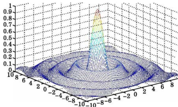
(a) 零级 Bessel 无衍射光束
