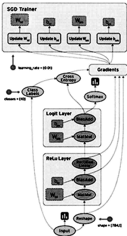
图 3-10 Google Tensorflow 搭建神经网络
