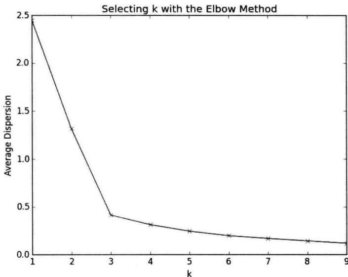
图 2-15 “肘部”观察平均距离与类簇数量的关系
