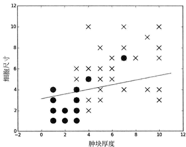
图 1-4 使用 10 条训练样本得到的二类分类器(绿色直线)(见彩图)
