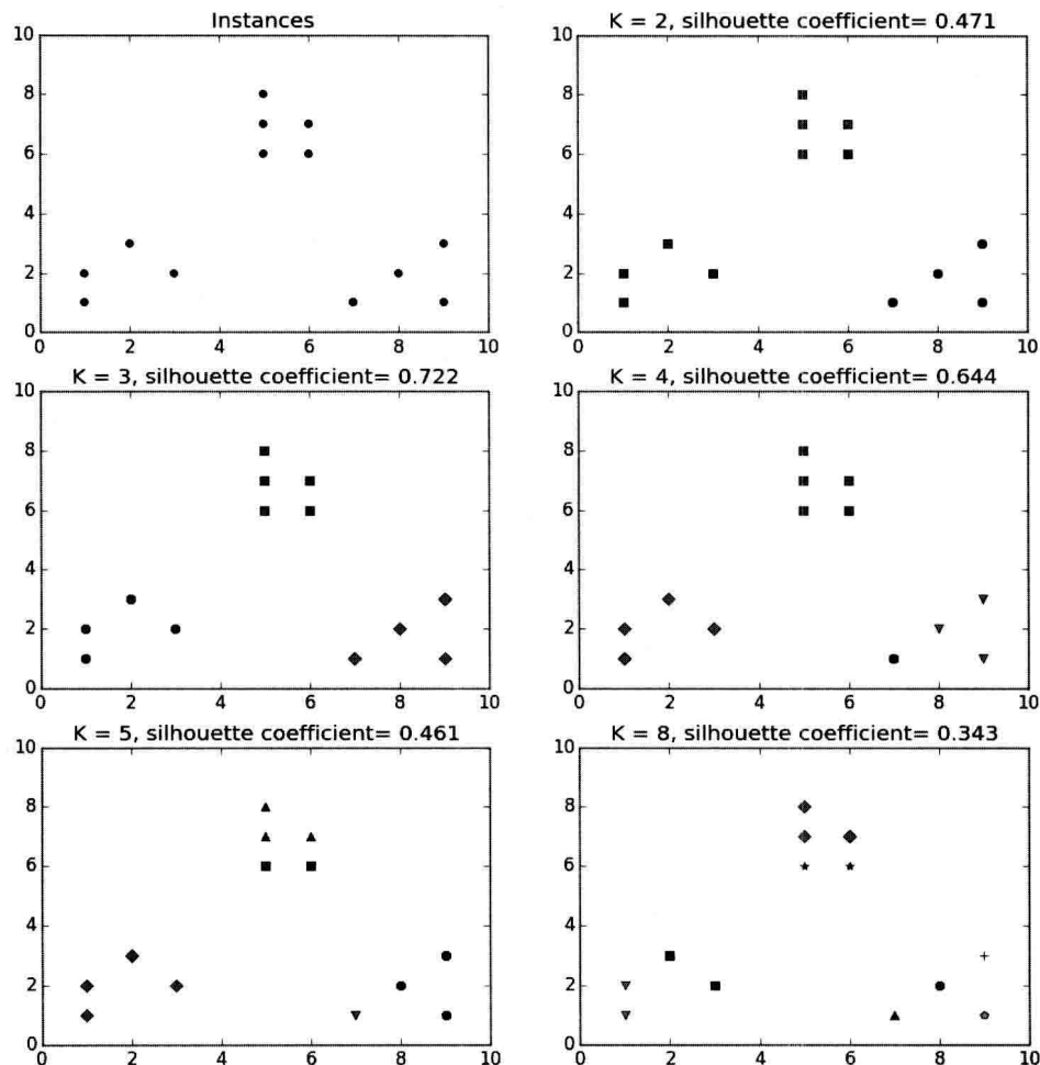
图 2-11 利用轮廓系数评价不同类簇数量的 K-means 聚类结果示例(见彩图)
