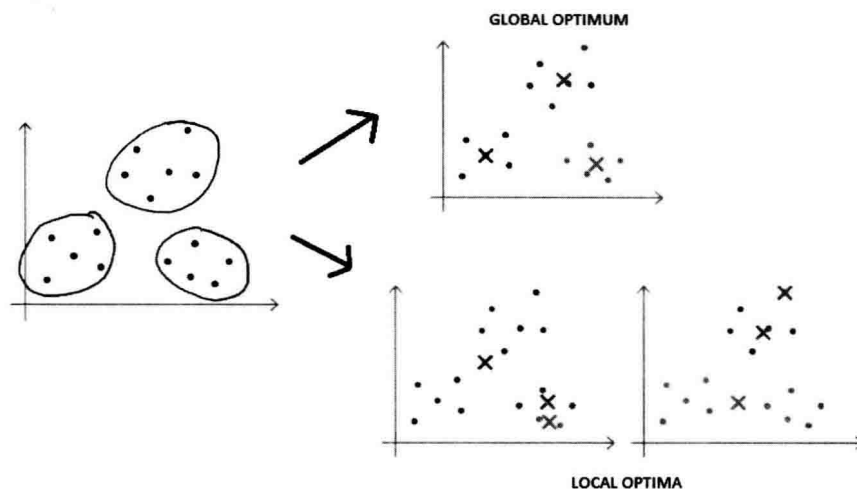
图 2-13 K-means 算法迭全局最优解与局部最优解的比较, 图片摘自于互联网 ① (见彩图)
