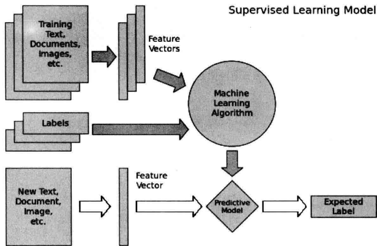
图 2-1 监督学习基本架构和流程(见彩图)①
