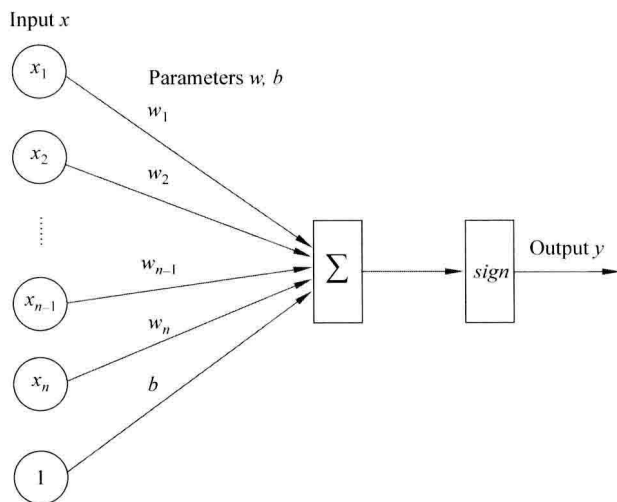
图 3-12 罗森布拉特感知机(Perceptron)模型
