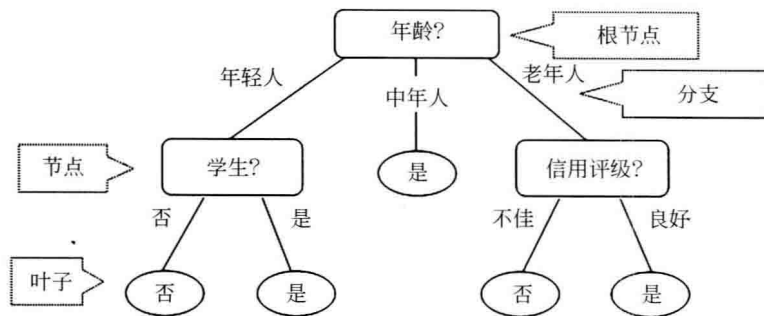
图 2-7 信用卡申请自动审核任务的决策树模型
