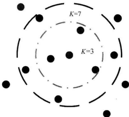
图 2-6 K 近邻算法展示样例(见彩图)
