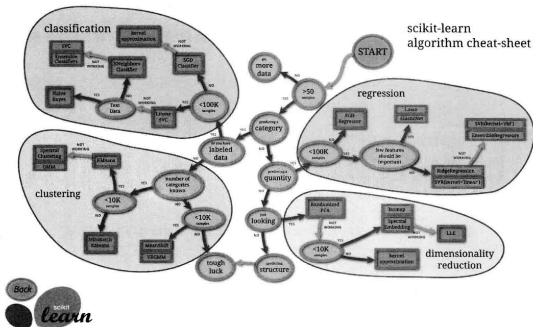
图 2-8 Scikit-learn 工具包模型使用建议(图片来源于 http://scikit-learn.org/stable/tutorial/machine_learning_map/index.html )(见彩图)
