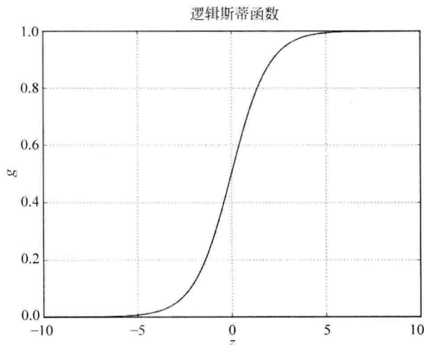
图 2-2 逻辑斯蒂函数图像
