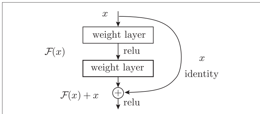
图8-12 ResNet的构成要素(引用自文献[24]): 这里的“weight layer”是指卷积层
