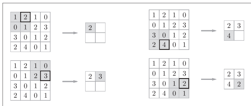
图7-14 Max池化的处理顺序
