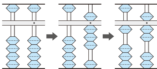
图24 计算8 + 9时
