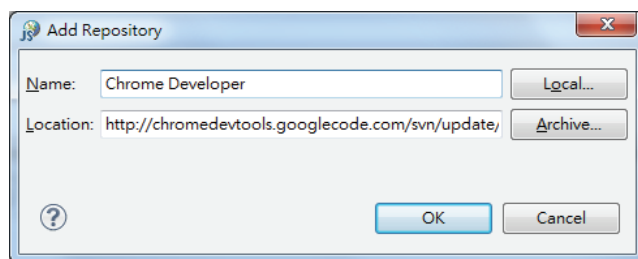
图3-9 Add Repository
