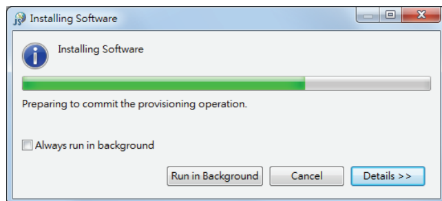
图3-13 安装过程
