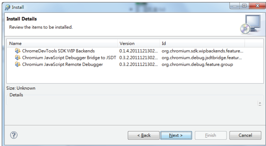
图3-11 计算依赖
