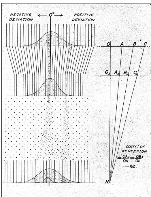
图 5-7 1877 年版本的高尔顿“钉板”，显示出为了保持恒定的种群分散，靠近顶部的倾斜的滑道如何补偿了下方增加的分散，以及位于上层的两个身高群体的后代如何通过这个过程追踪到下层
