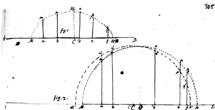
图 3-6 伯努利 1769 年绘制的曲线，其中 figure 1 使用的权重基于 figure 2 的曲线（Bernoulli 1769）
