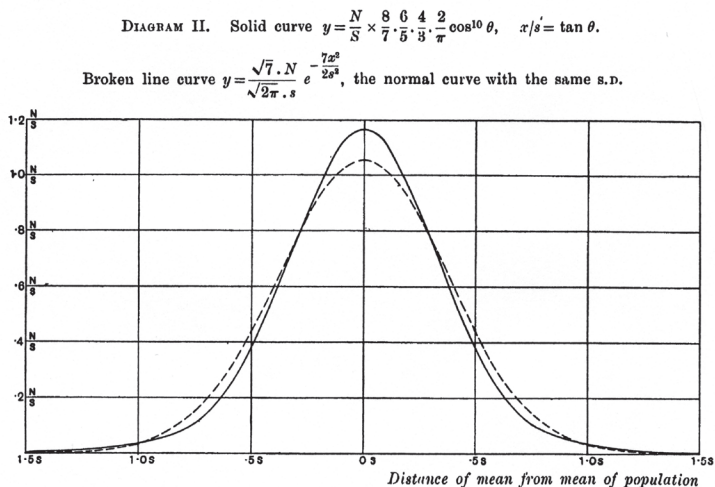
图 4-2 1908 年论文示意图，比较正态分布和 t 分布（自由度为 9）的密度（Gosset 1908）
