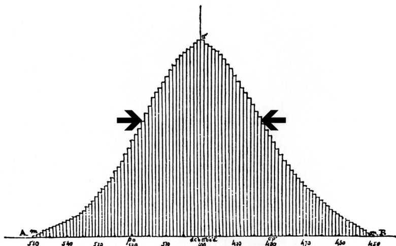
图 2-2 一张显示棣莫弗两个拐点的图片（和 1730 年讨论的一样），叠加在一张 n=999 的对称二项分布图上，由凯特勒绘于 19 世纪 40 年代
