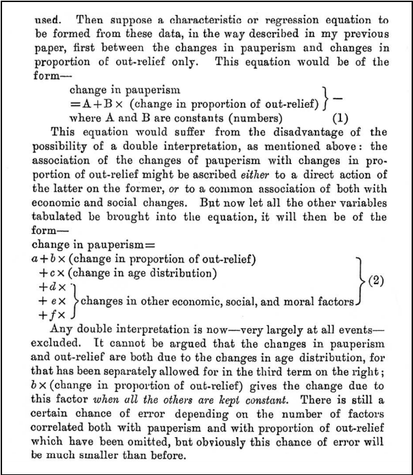
图 7-2 尤尔描述贫困变动的多元回归方程（Yule 1899）
