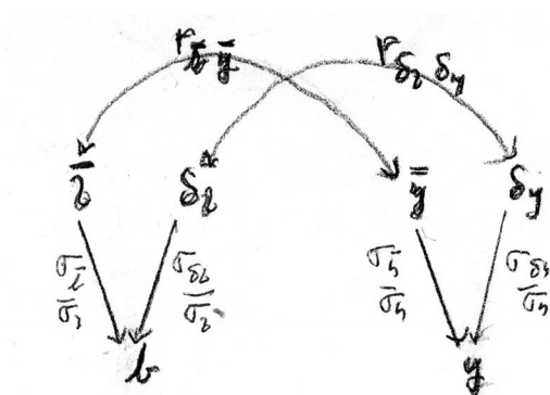
图 5-16 休厄尔·赖特 1917 年的第一个路径分析，根据 1975 年 4 月赖特和作者的私人通信重新画出（Wright 1975）
