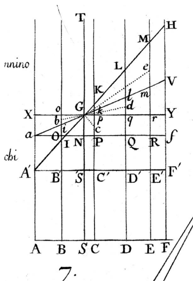
图 7-1 博斯科维奇自己的图，来自 1770 年的一份出版物，展示了表示球体的线 XY ，和表示为 a 、 b 、 c 、 d 和 e 的 5 个 XY 的残差点。博斯科维奇通过自己的算法发现的线是 GV ，是 XY 残差计算的斜率（Maire 与 Boscovich 1770）
