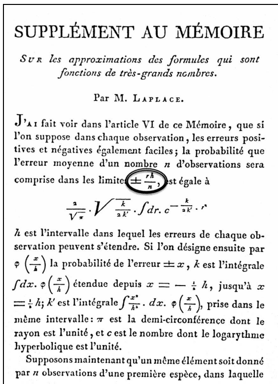
图 2-3 拉普拉斯关于中心极限定理的第一次清晰表述。这里他所用的 c 是我们现在常用的 e , k'/k 表示方差, 积分表示等于平均误差不超过给定限制的概率 (画圈的部分), 但分母中的 n 应该是 \sqrt{n} (Laplace 1810)
