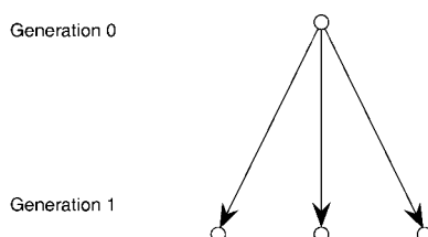
图 5-3 在一代的后代中产生的变异
