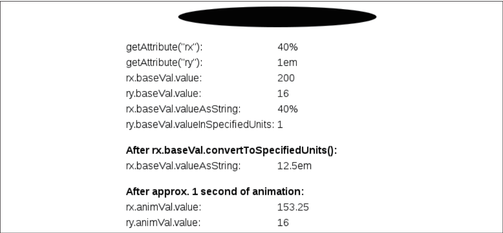
图 14-1：使用 baseVal 和 animVal 取值的动画
