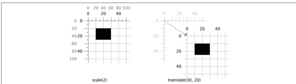
图 6-11：先缩放后平移的工作原理
