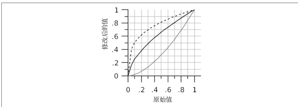
图 11-11：伽马曲线函数
