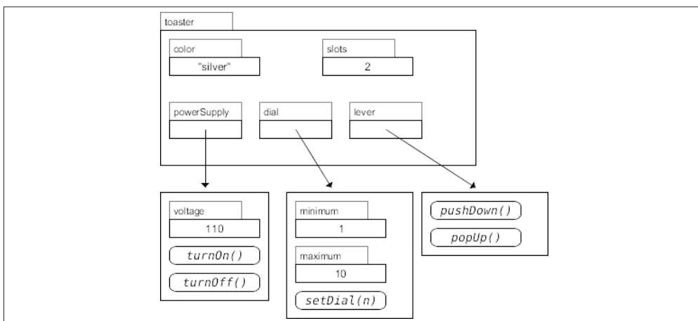
图 C-4：烤面包机对象
