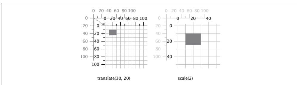
图 6-9：先平移后缩放的工作原理
