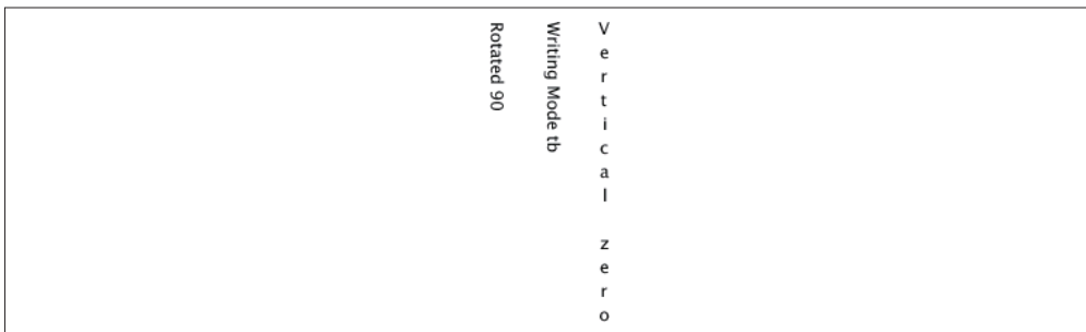
图 9-12：纵向文本
