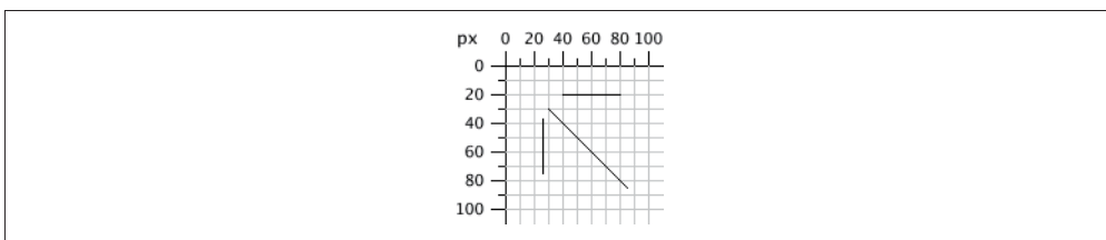
图 4-1: 线段
