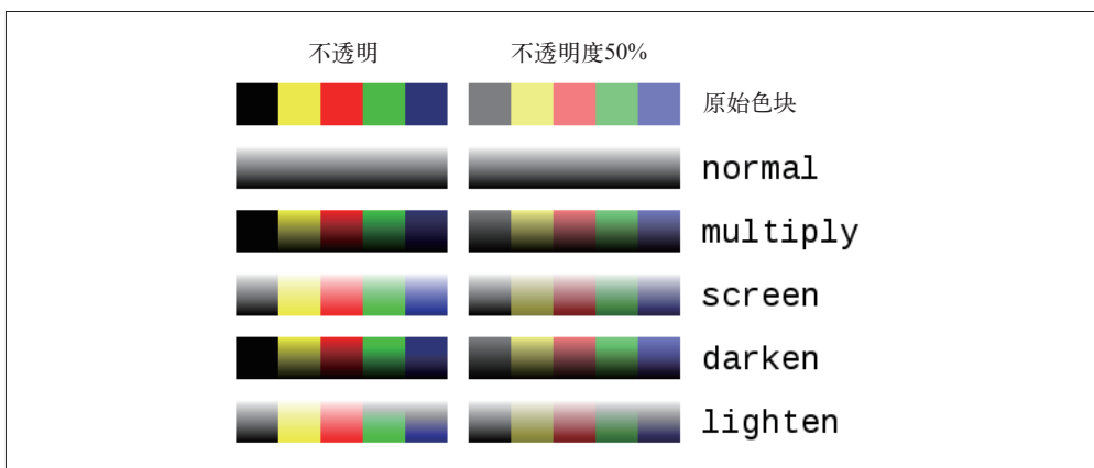
图 11-17: <feBlend> 的效果
