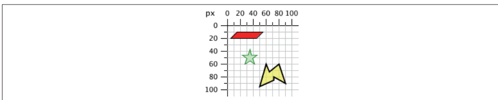
图 4-10：多边形
