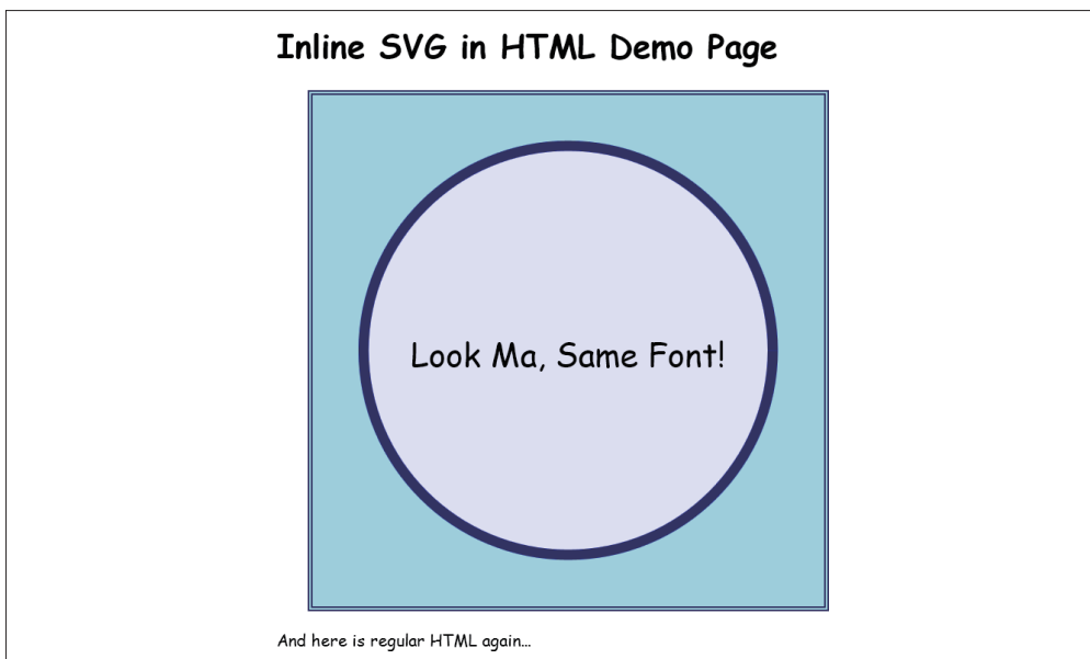
图 2-3: 示例 2-2 的结果
