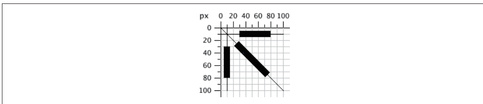
图 4-2: 演示 stroke-width
