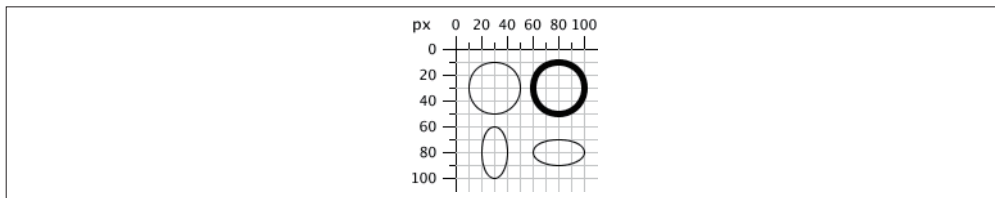
图 4-9：圆和椭圆
