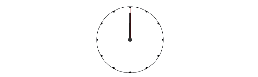
图 14-2: 模拟时钟
