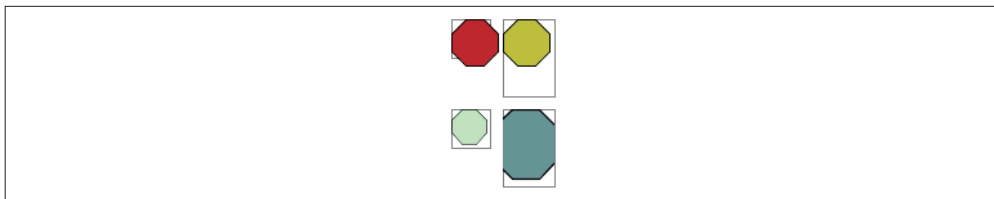
图 5-7: 组合与 symbol
