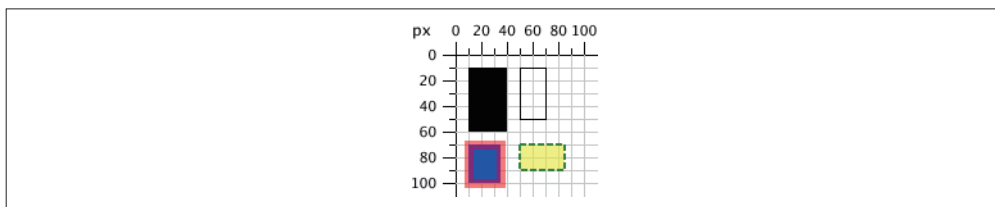
图 4-6: 矩形
