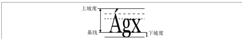
图 9-2: 符号的度量
