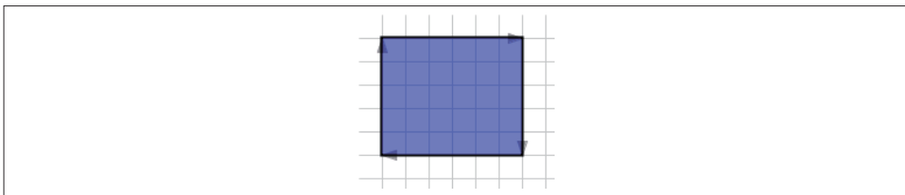
图 1-2: 矢量长方形
