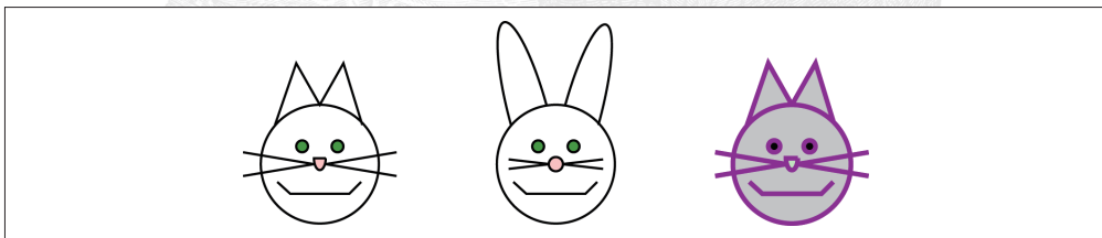
图 5-1：结构与表现
