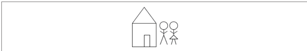
图 5-4: 分组火柴人
