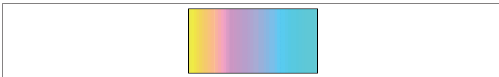
图 8-8：三色渐变
