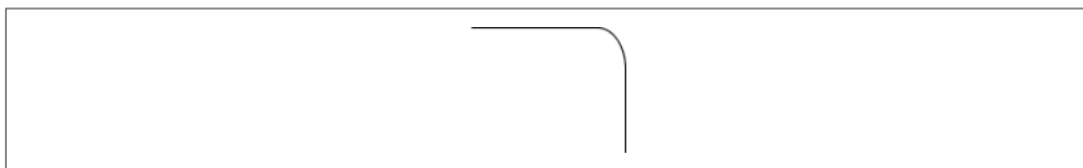
图 7-16: 线和圆弧
