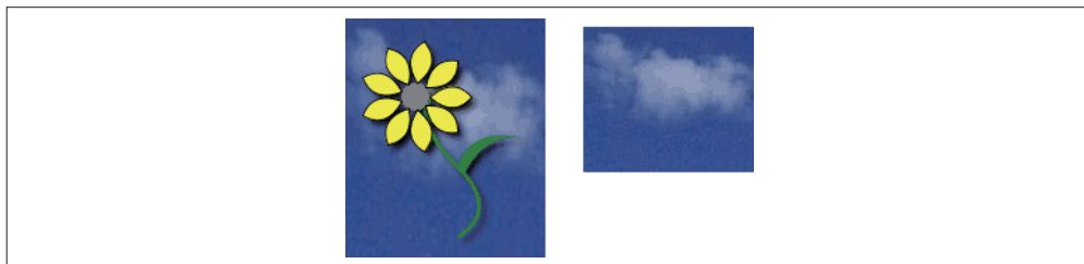
图 11-9：<feImage> 效果
