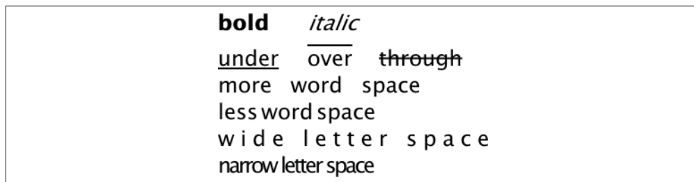
图 9-4：文本样式
