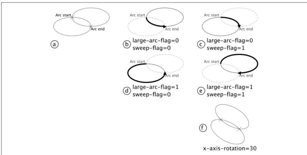
图 7-5：椭圆弧命令
