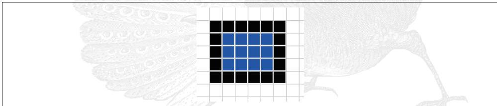
图 1-1：栅格长方形
