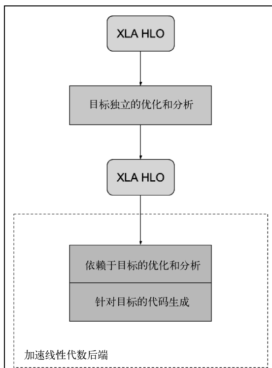
图9-4 加速线性代数编译过程（来源： https://www.tensorflow.org/images/how-does-xla-work.png ）
