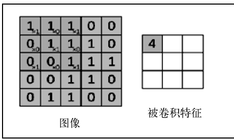
图4-4 输入图像、卷积核和被卷积特征
