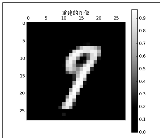
图5-6 重建的图像
