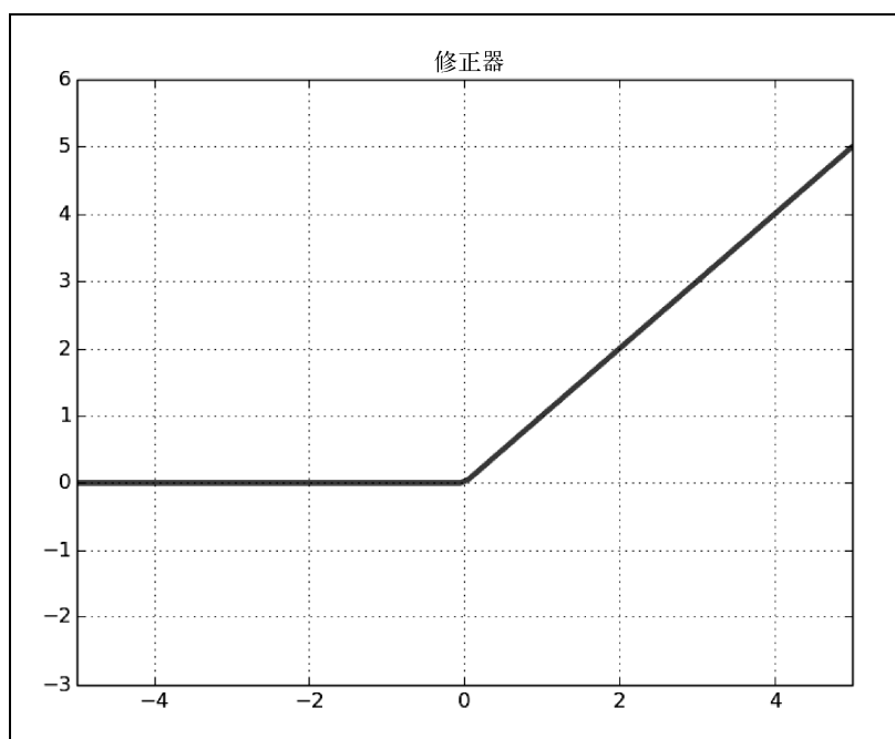
图3-9 ReLU函数
