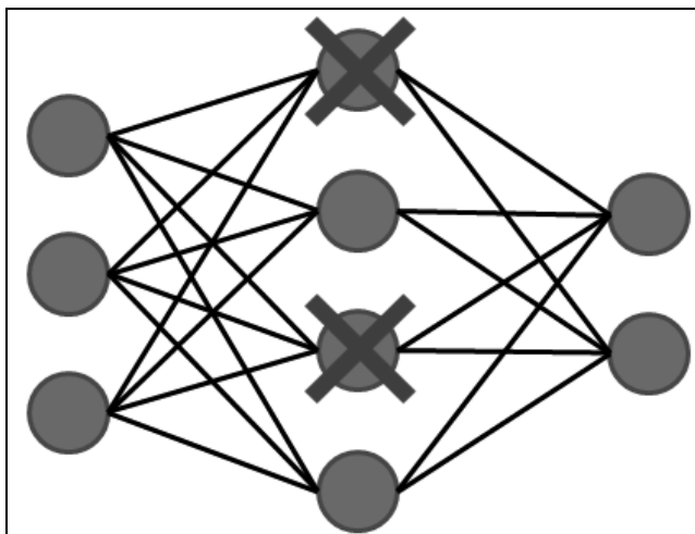
图3-11 dropout示意图
