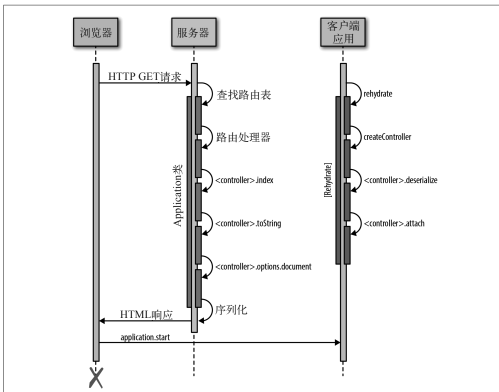
图 10-1: 客户端 rehydration
