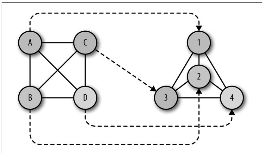
图 3-1：同构的图
