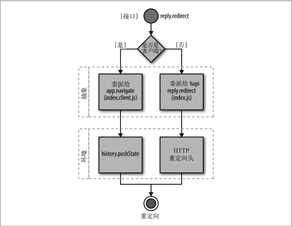
图 9-2: 同构重定向
