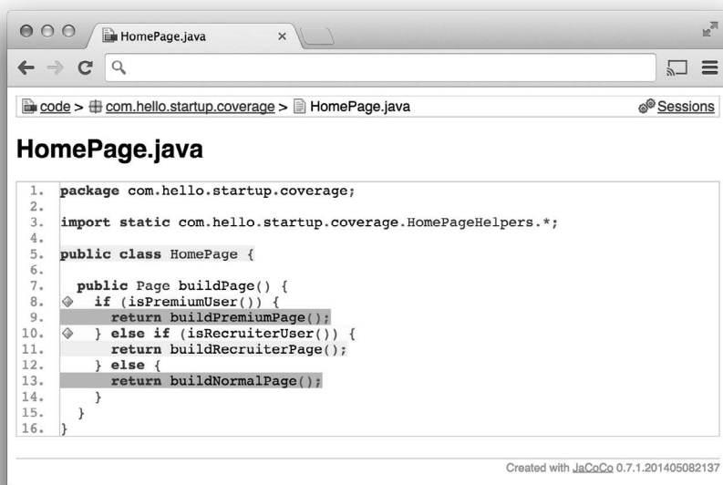
图 7-1: JaCoCo 代码覆盖
