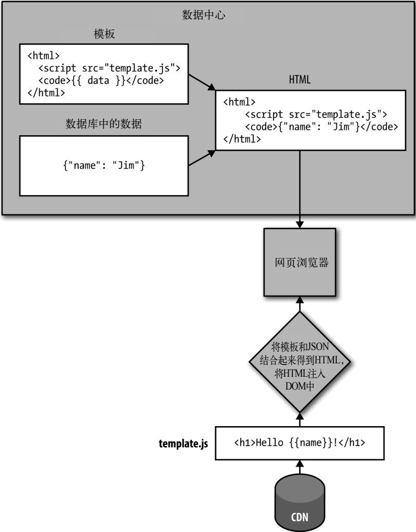
图 5-3: 客户端渲染
