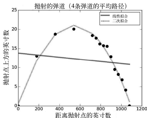
图18-12 轨迹图
