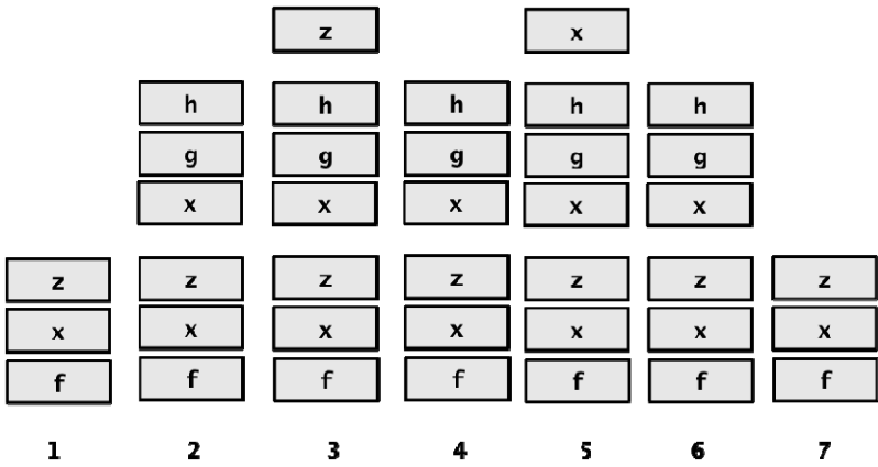
图4-3 栈帧
