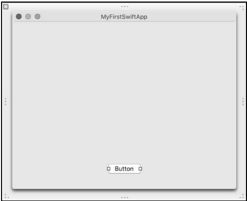
图7-12 包含UI元素Push Button的窗口
