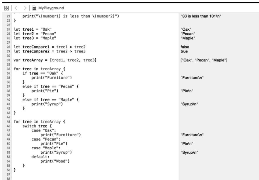
图3-13 包含在for循环中的switch-case语句
