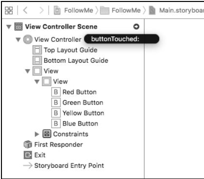
图9-18 连接到方法buttonTouched
