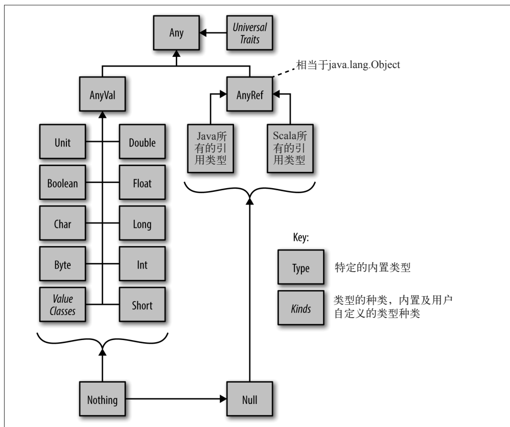
图 10-1: Scala 的类型层次结构
