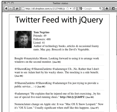
图 16-13 jQuery 代码获取到一条 JSON 格式的 feed（本例中，是本书其中一位作者的 Twitter 数据流），解析它，并将结果显示在页面上
