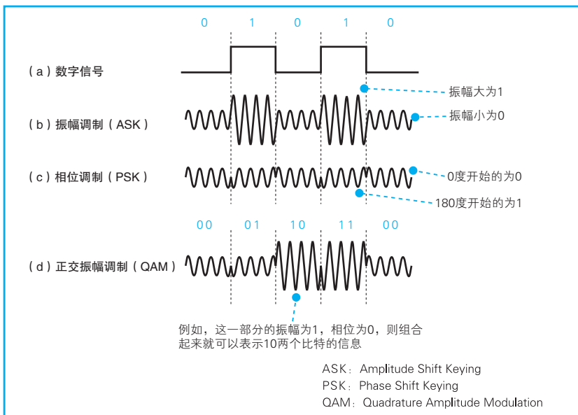
图 4.4 信号的调制
