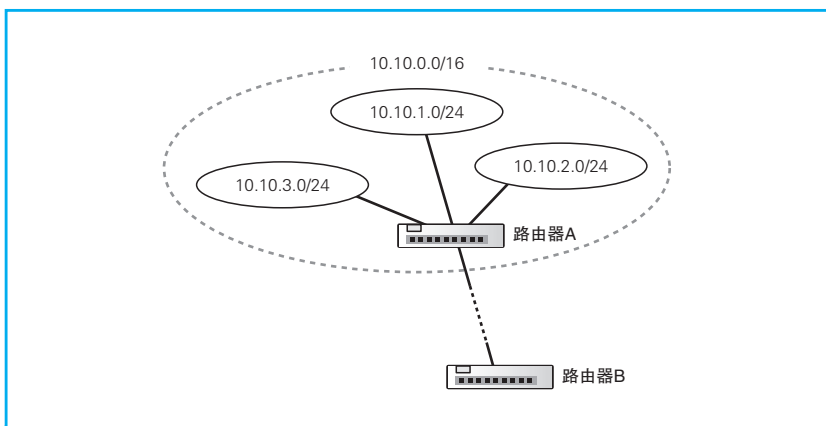
图 3.14 路由聚合
