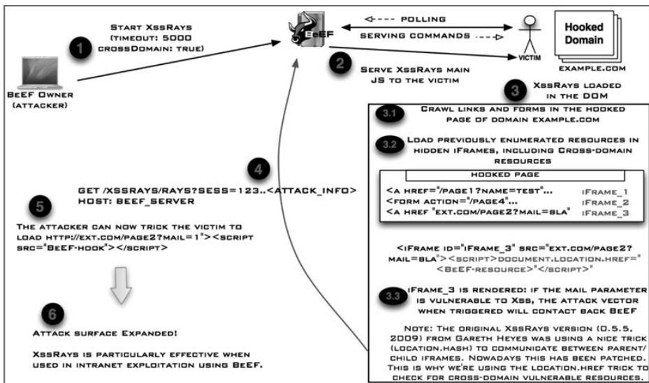
图9-15 XssRays的高层构架
