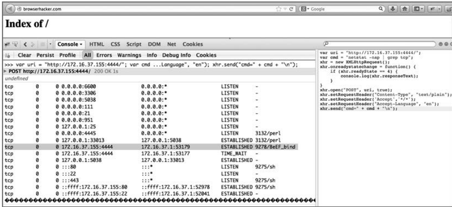
图10-32 向BeEF Bind发送netstat命令
