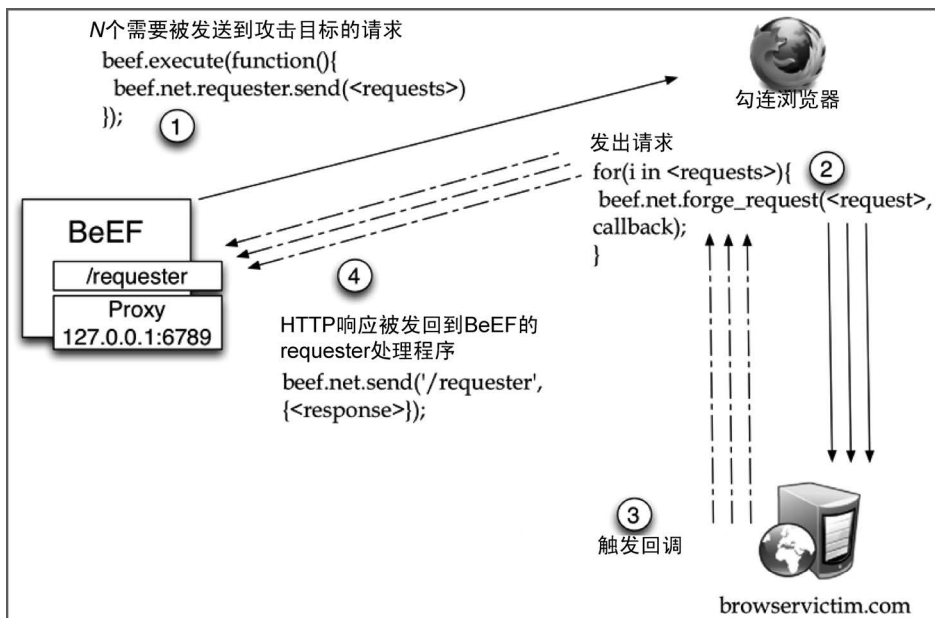
图9-16 BeEF的Tunneling Proxy内部的架构流程
