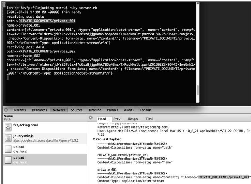
图4-18 跨域发送POST数据
