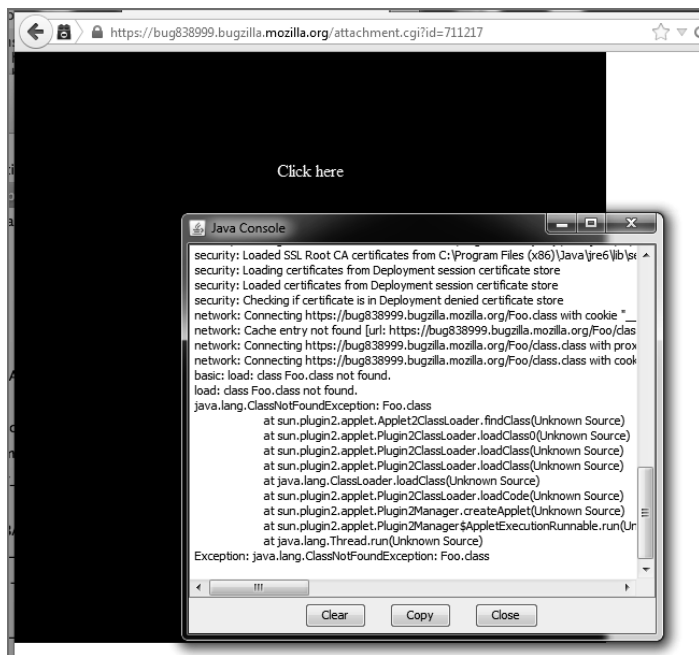
图8-8 绕过点击播放执行一个未签名的Java小程序
