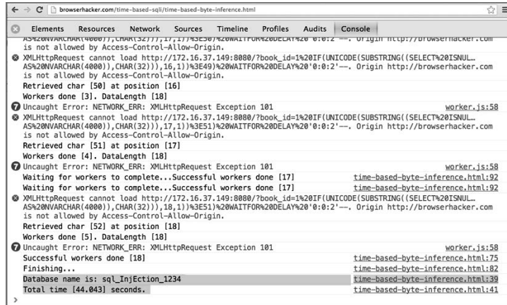
图9-13 5个工作进程在Chrome中取得了数据库名称
