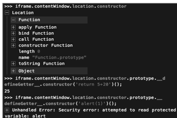
图4-5 尝试执行受限行为时，会发生安全错误
