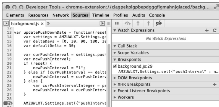
图7-10 调试扩展
