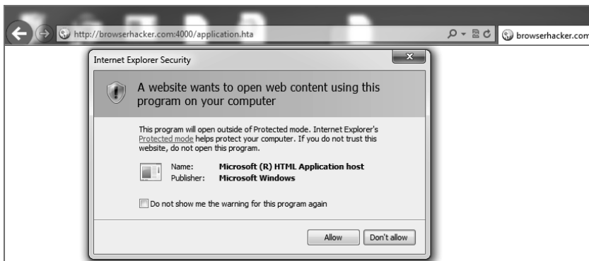
图5-17 HTA警告
