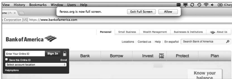
图5-8 全屏警告
