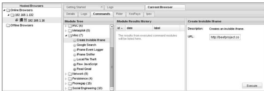
图6-32 执行BeEF的Create Invisible IFrame模块
