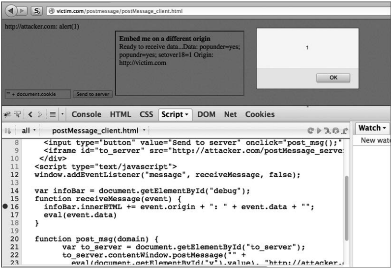
图3-4 响应被求值，JavaScript被执行
