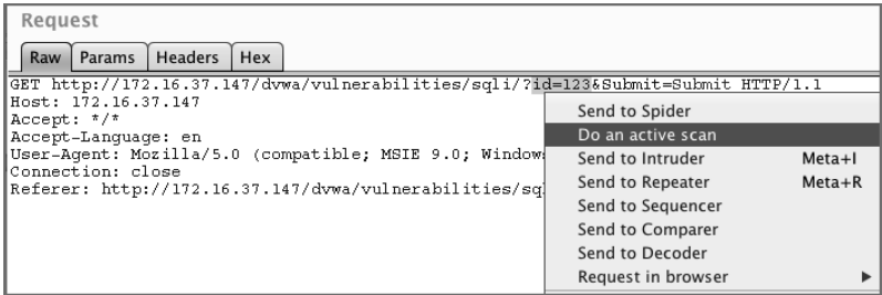
图9-25 对特定资源进行活跃度扫描
