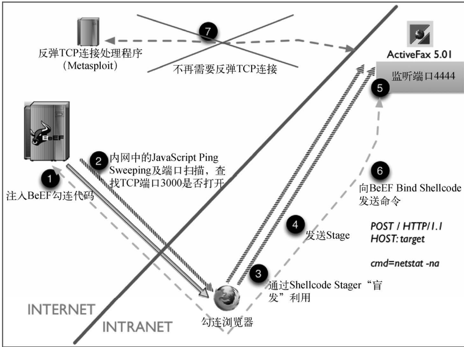
图10-30 通过BeEF Bind Shellcode实现ActiveFax利用的示意图
