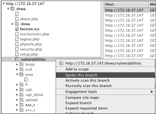
图9-24 为Burp的Spider添加一个网站资源分支
