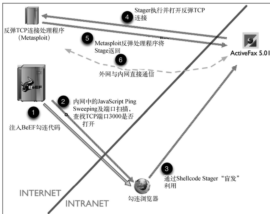
图10-24 使用反弹Meterpreter Shellcode利用ActiveFax漏洞的流程
