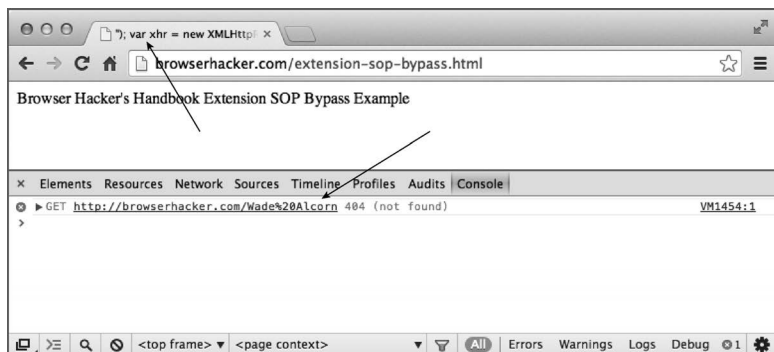
图7-16 在Chrome扩展中绕过SOP
