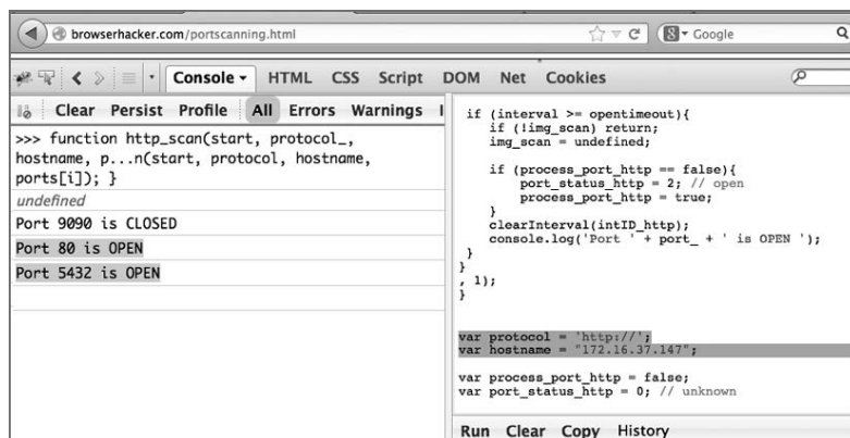
图10-9 在内部网络中发现某系统中的开放端口
