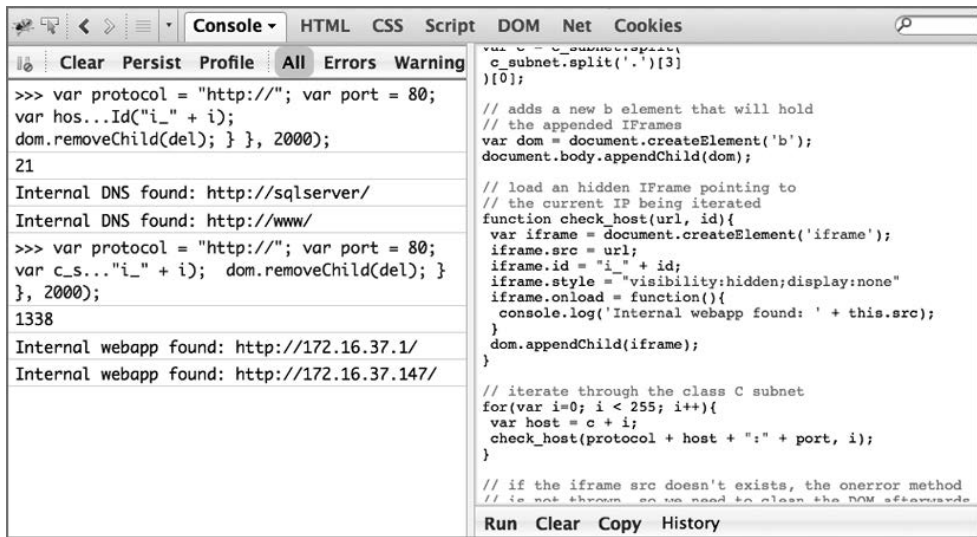
图9-2 发现内网设备及域名
