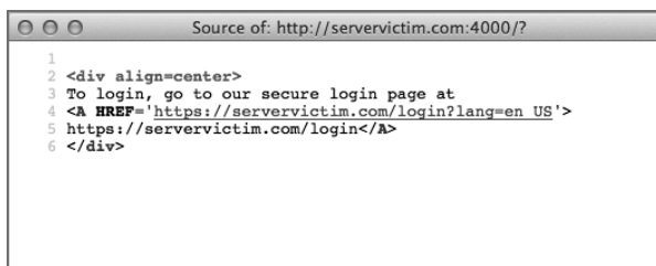
图6-20 未经XSS的登录页面源
