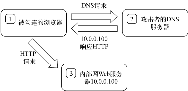
图3-7 返回1位
