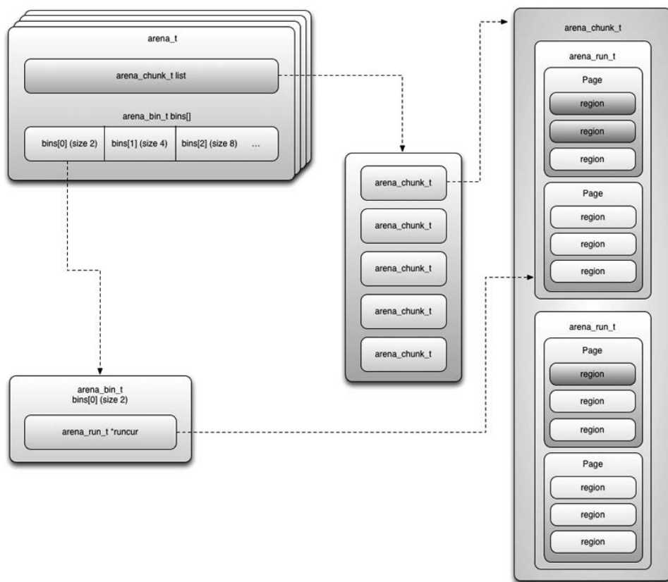
图6-27 jemalloc的架构 38
