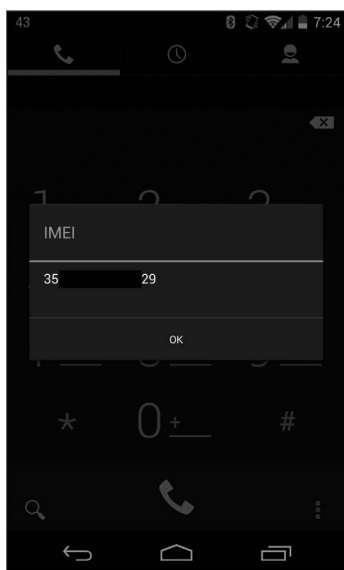
图6-25 安卓IMEI
