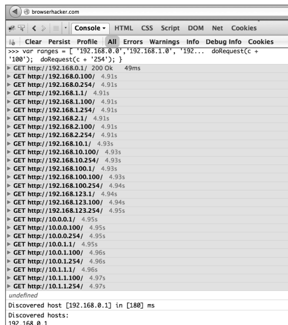
图10-2 成功找到192.168.0.1
