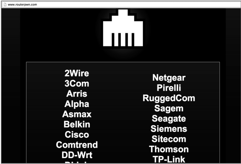
图9-40 Routerpwn： www.routerpwn.com
