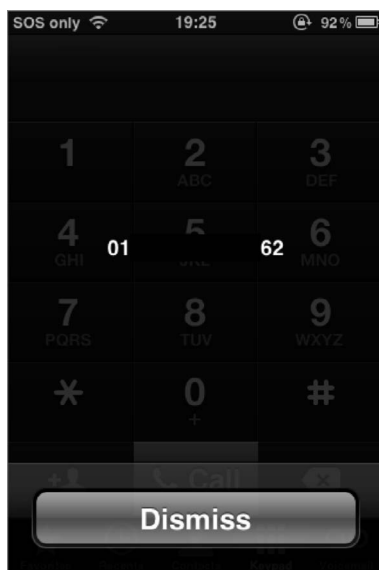
图6-26 iPhone IMEI
