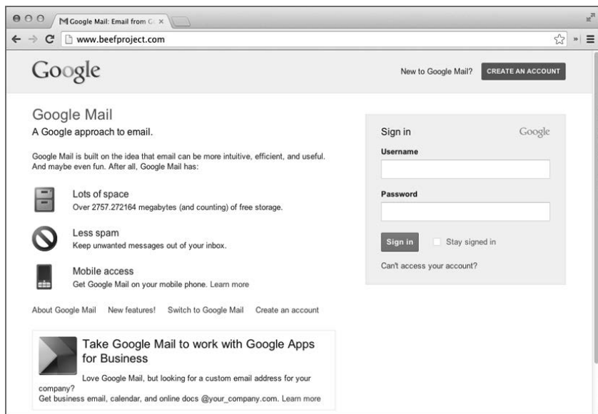
图5-16 Gmail钓鱼
