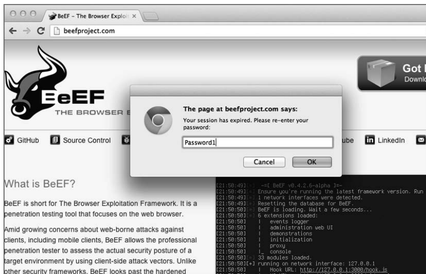
图5-13 对话框提示
