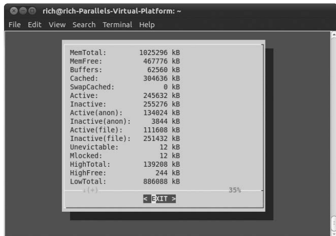
图18-8 用textbox对话选项显示的meminfo命令输出
