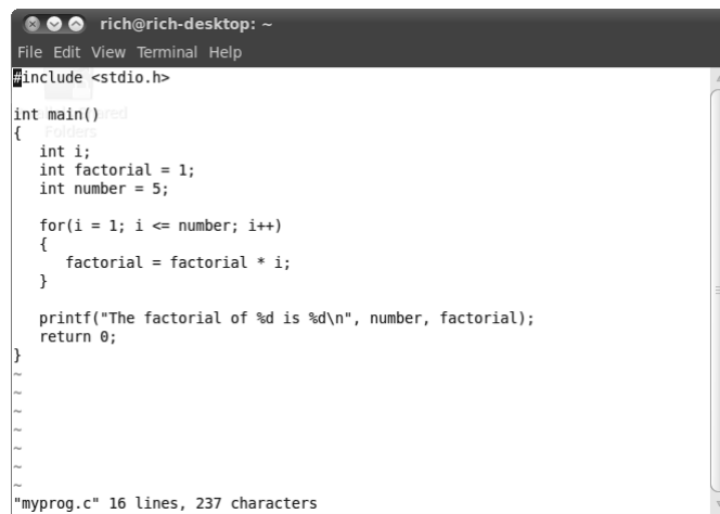
图10-1 vim的主窗口
