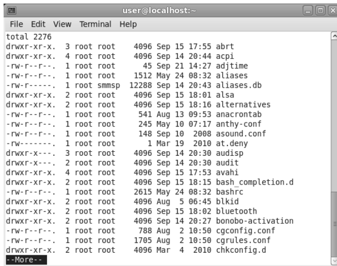
图11-2 和ls命令一起使用more命令
