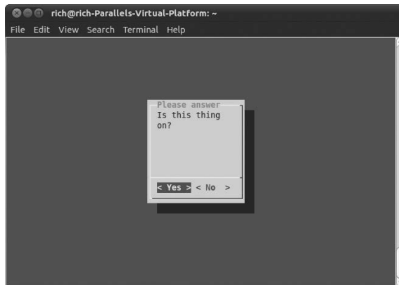
图18-3 在dialog命令中使用yesno部件
