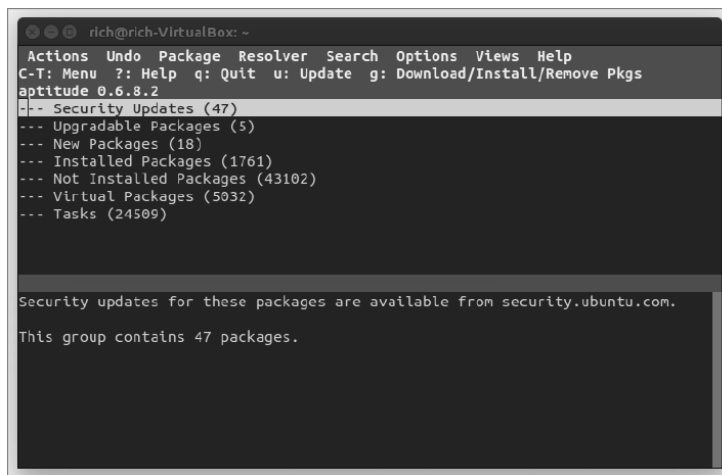
图9-1 aptitude主窗口
