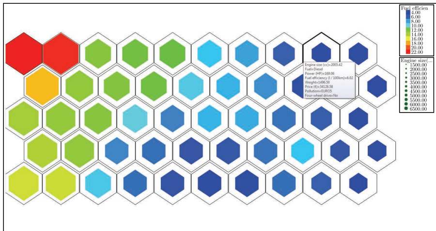
图 17-5 一个 SOM，颜色和大小取决于二维原型向量的两个坐标，可以将鼠标移到神经元上来显示原型的值（通过 LIONoso.org 提供的软件，另见彩插）
