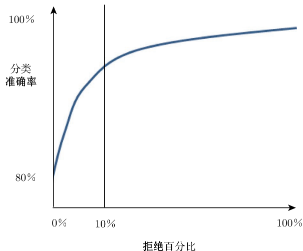
图 13-8 准确率-拒绝的折中曲线。可以通过拒绝一些疑难的实例来得到更高的精度
