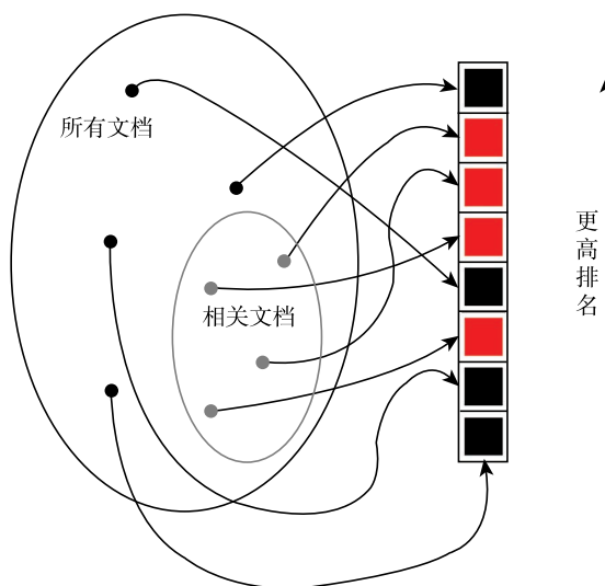
图 25-5 一个排名的例子
