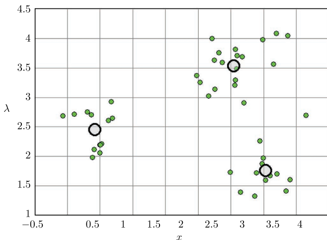
图 15-4 K 均值聚类, 独立的数据点和聚类原型如图所示
