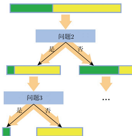
图 6-4 树构建中的递归步骤：经过问题 2 初步纯化后，将同样的方法应用在左边和右边的实例子集上。在这个例子中，问题 3 就足以完全净化这些子集。不需要在纯子集上执行额外的递归调用
