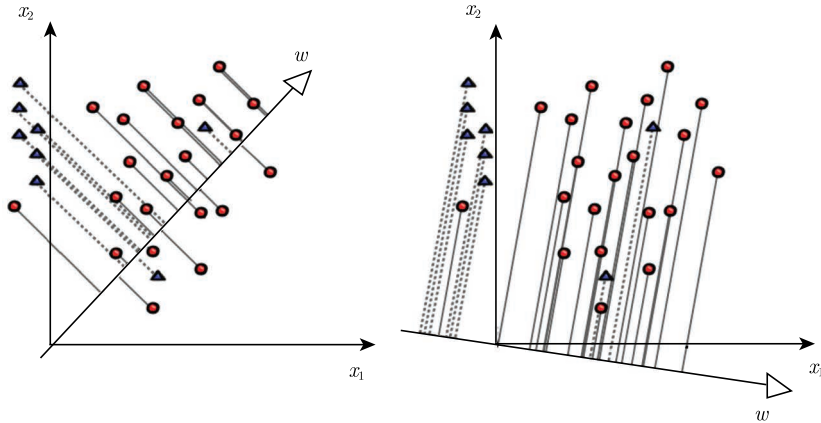
图 18-4 费希尔线性分类模型(三角形表示一个类,圆形表示另一个类):左边的一维投影将两个类混合在一块了,而右边的投影通过投影样本散度可以最佳地分开这两个类的投影点
