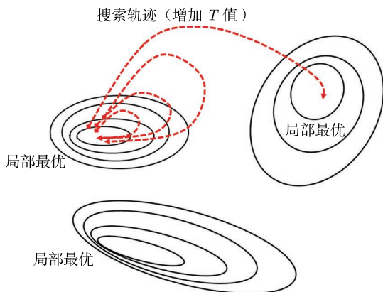
图 22-6 RSO 自适应禁忌。图中描述了 3 个局部最优和优化函数的过程（虚线）。从一个局部最优开始，RSO 在该吸引域内不断搜索，越来越远离该最优点，直到进入另一个吸引域内
