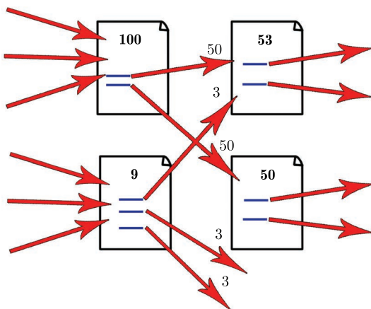
图 25-10 在 PageRank 算法中重新计算网页的排名,初始排名沿着链出链接分发到其他网页(改编自原始论文)
