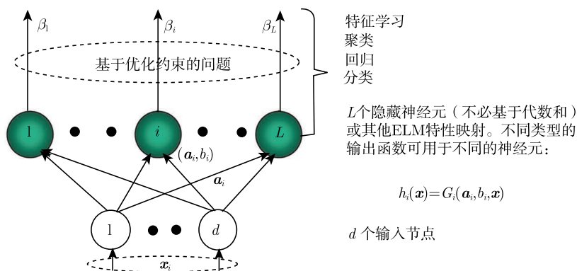
图 14-8 超限学习机的隐藏层可以包含不同种类的可计算节点（改编自参考文献[63]）
