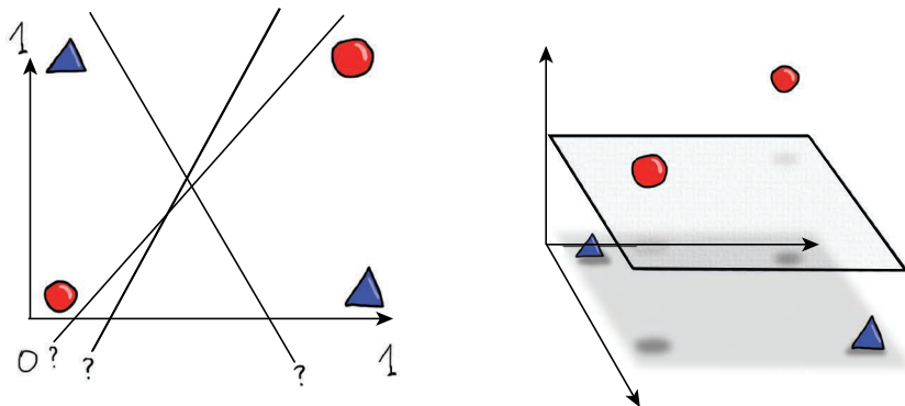
图 4-2 不能进行线性分离的情形（XOR 函数，左）。可以通过将点以非线性方式映射到更高维度的空间，通过超平面获得线性分离
