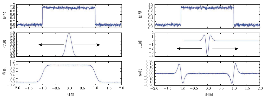
图 10-6 卷积的两个例子：(左) 高斯平滑；(右) 高斯差分边界增强
