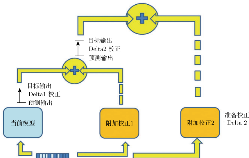
图 13-7 加性模型中的贪心逐步向前法，通过添加新的组件的迭代来取消剩余的误差
