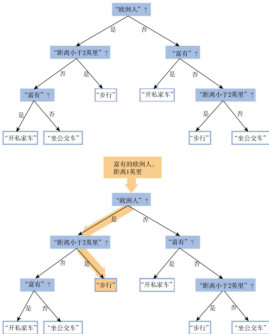
图 6-2 决策树 (上图), 以及同一棵树中达到分类的一种情况 (下图)。抵达拆分节点的数据点根据测试函数的结果被发送到其左子节点或右子节点
