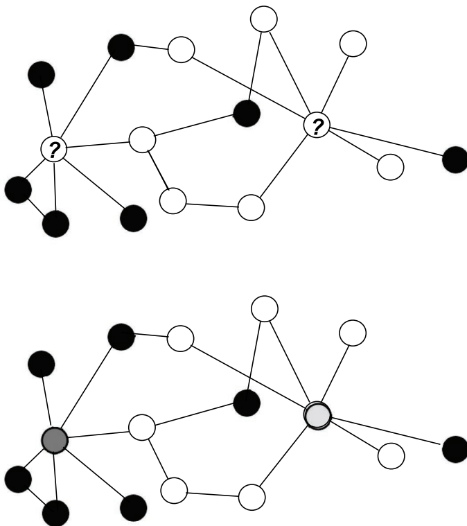
图 20-3 通过图中相邻点的平均值计算未知点的值
