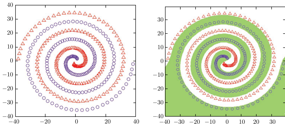
图 12-1 SVM 学习双螺旋的分类问题，两个类分别用圆圈和三角形表示。这幅图展示了 SVM 卓越的泛化性能
