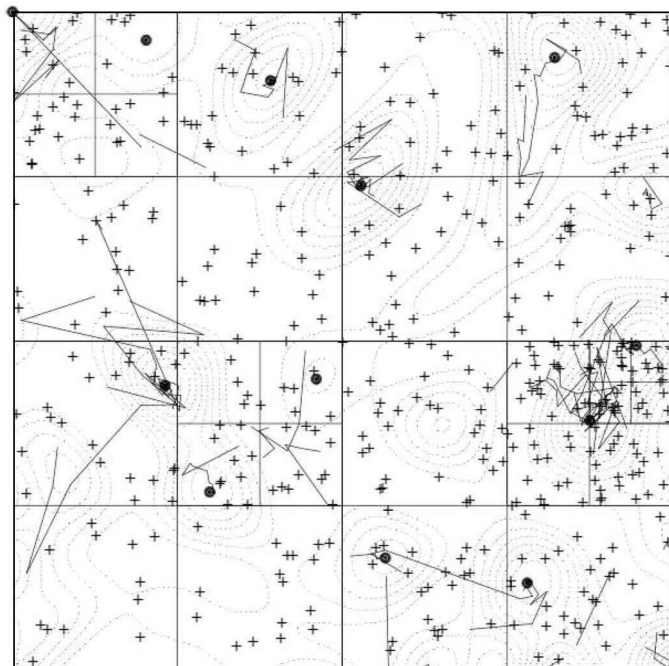
图 23-4 一棵包含适应度平面和求值点的 CoRSO 树: 求值点(加号)、局部极值点(实心点)、LS 堆积(折线)。本图改编自参考文献 [17]
