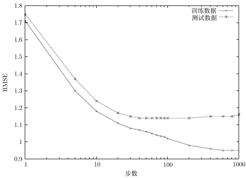
图 26-2 一个实际的分解过程：训练和测试性能表示为梯度下降的迭代步数的函数
