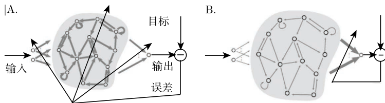
图 14-7 （左图）递归神经网络传统的基于导数梯度的训练方法需调整所有的连接参数（粗箭头），而（右图）储备池计算只需修改连接递归神经网络和输出之间的连接参数即可（改编自参考文献 [79]）
