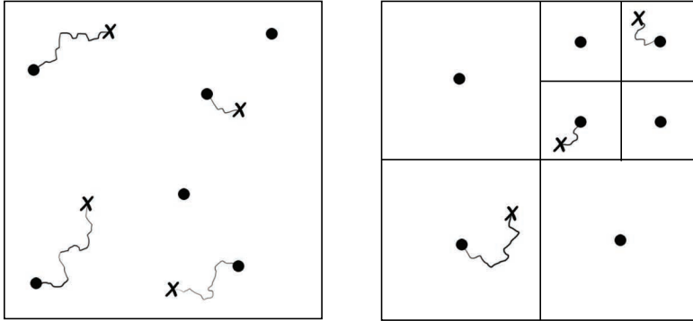
图 23-1 分配局部搜索器的不同方式: 模因算法 (左图) 和政治类比 (右图)。叉号表示起始点, 圆圈表示使用局部搜索得到的局部最优。在右图中, 每个个体负责构型空间的某个区域, 比如政治上通过选区来划分区域, 企业中为不同的区域分配不同的营销经理。局部搜索流如图所示
