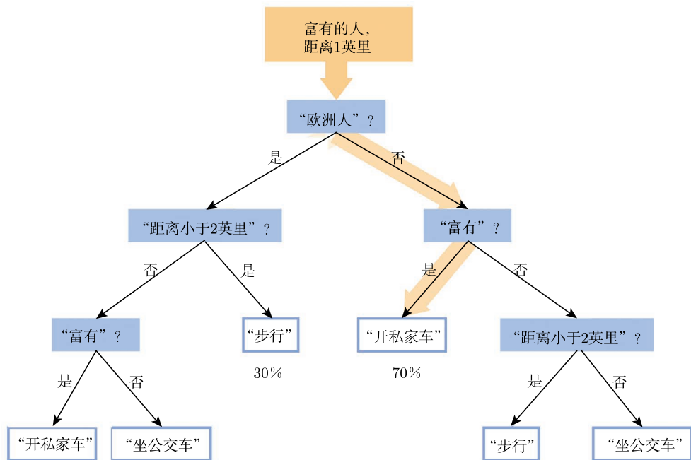
图 6-6 缺失的身份信息。到达顶部节点的数据点被发送到其左侧和右侧的两个子节点，权重根据答案“是”和“否”在训练集中出现的频率而有所不同
