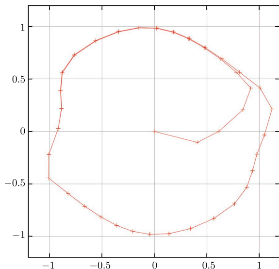
图 14-2 递归神经网络沿着环形训练：没有初始输入的情况下的输出序列
