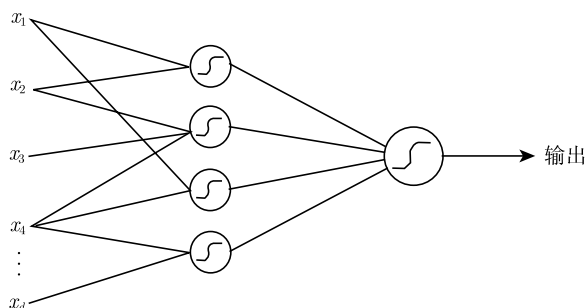
图 9-3 多层感知器：中间（隐藏）层的 S 型传递函数引入的非线性，使得创建任意连续函数变成可能。图中展示了单隐藏层
