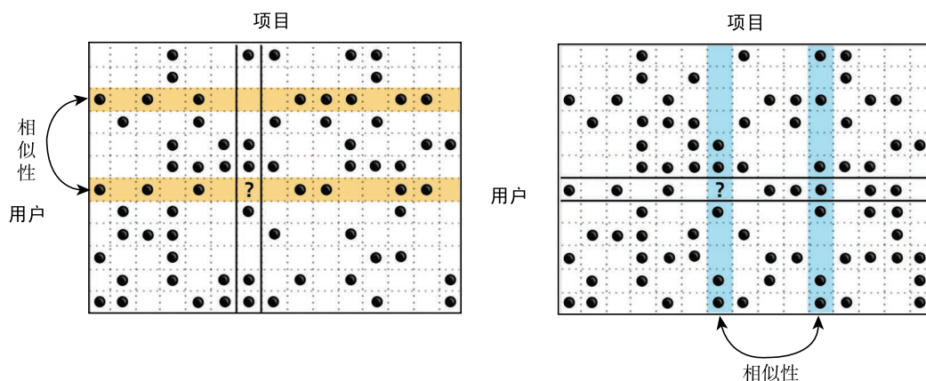
图 26-1 协同推荐。要预测未知值，可以计算已知值的加权平均，权重取决于用户或项目之间的相似性
