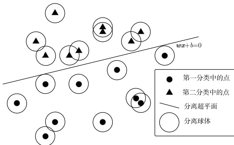
图 11-3 假设空间约束。该分离超平面必须最大化边界。直观来说，没有太靠近边界的点，使得输入数据中的一些噪声和将来由相同概率分布产生的数据不会破坏分类
