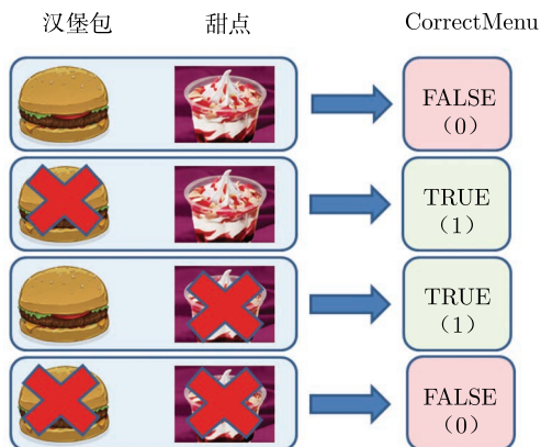
图 7-1 有两个二元输入和一个输出的分类器。单个特征分开来看都不具有信息量, 对于一个正确的输出, 这两个特征的结合是充分必要的
