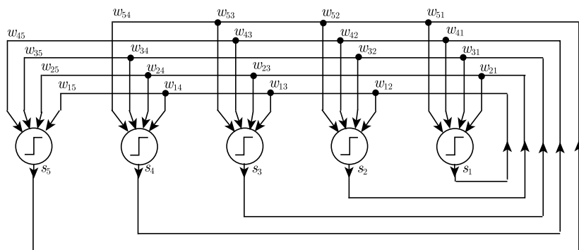
图 14-4 由 5 个神经元和反馈循环组成的霍普菲尔德网络
