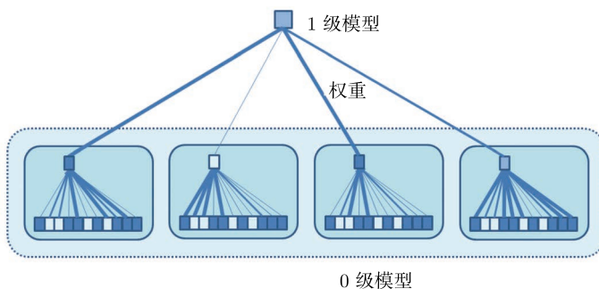
图 13-1 通过在模型之上增加附加模型来融合不同模型（堆叠）
