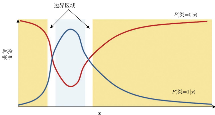
图 13-9 一个贝叶斯分类器中的过渡区域。如果拒绝落在接近边界的过度区域的实例,那么平均准确率将会上升
