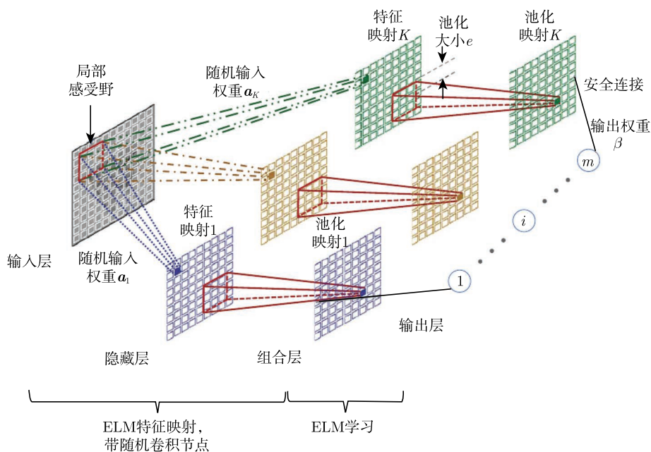
图 10-8 一个带有局部感受野的结构化的体系结构（卷积）和池化层（改编自参考文献 [53]）
