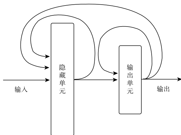
图 14-1 递归神经网络基本图解
