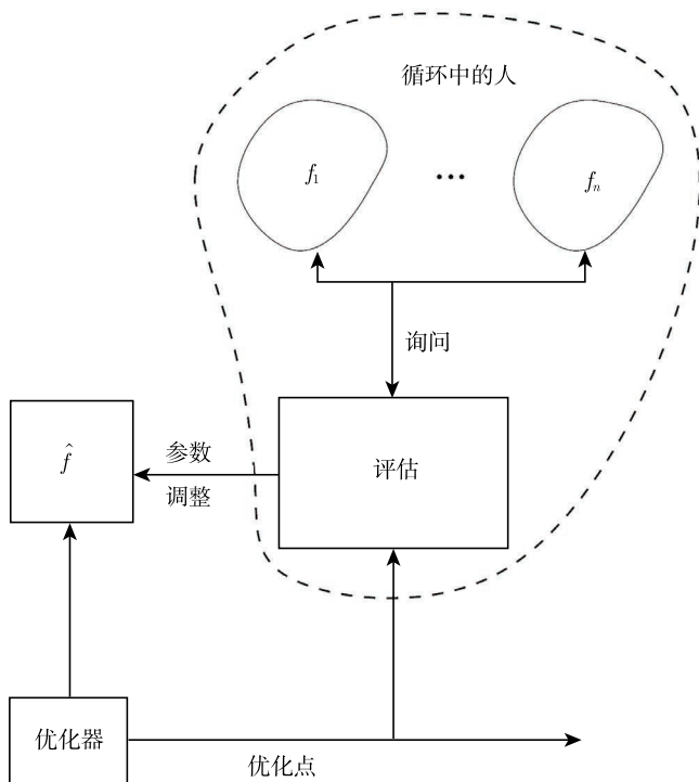
图 24-3 脑-计算机优化 (BCO): 对于交互的多目标优化, 从最终用户中学习问题的定义 (改编自参考文献 [10])。
