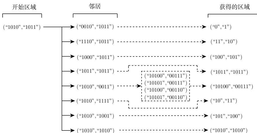
图 23-3 CoRSO: 区域 (1010,1011) 所有邻居的值
