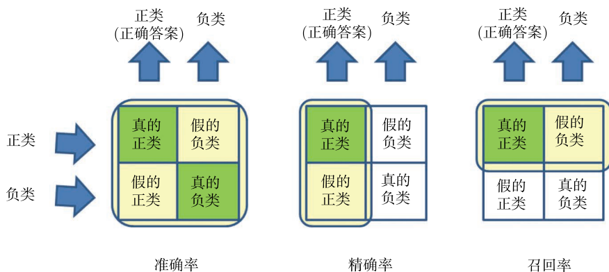
图 3-4 矩阵中的每一行报告一个类别的不同分类。你可以想象从左边进入，按不同的列进行分类，再从顶部退出的情况。准确率定义为正确答案占总体的比例，精确率定义为正确答案占标记为正类的比例，召回率定义为正确答案占本身是正类的比例。图中依据浅灰色区域的案例，对暗灰色区域的案例进行了划分
