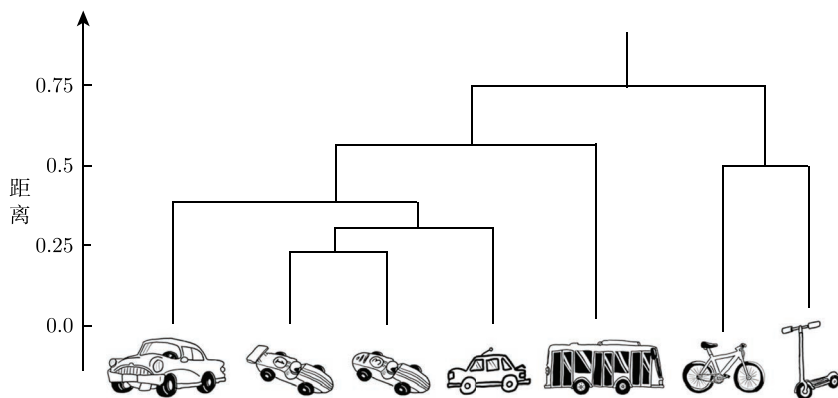
图 16-2 交通工具的自底向上聚类示意图
