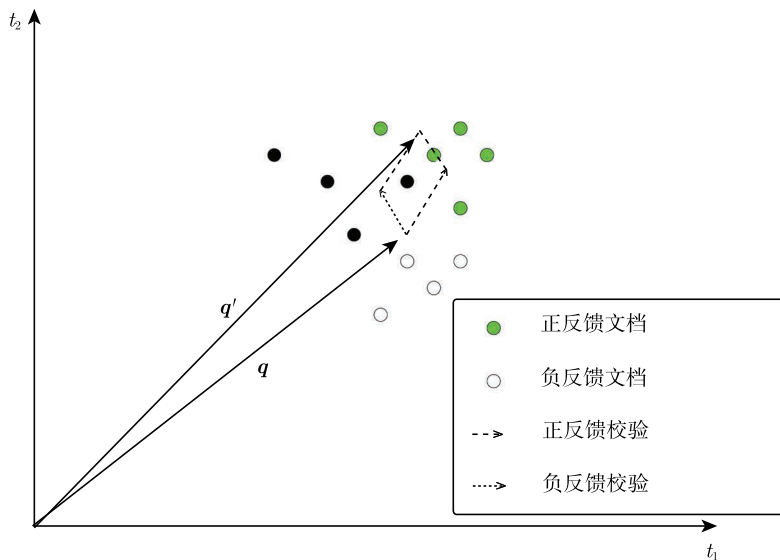
图 25-7 罗基奥方法
