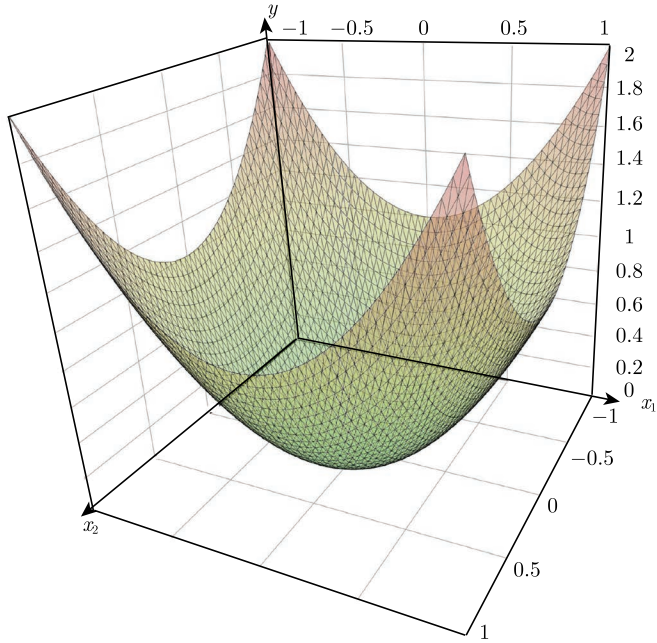
图 21-6 含有两个变量的二次正定型 f
