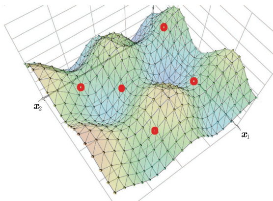
图 1-2 从样本中使用克里金法构造模型。一些样本在图中用点标示出来。表面的高度和颜色依赖于产金量（另见彩插）
