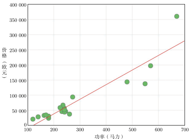
图 4-1 不同车型的价格与功率的数据。线性模型看起来像一条直线
