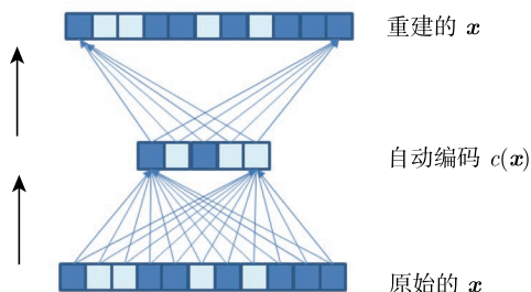
图 10-1 自动编码器
