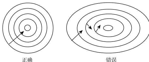
图 21-9 当搜索最小值的时候，梯度有时并不是合适的方向
