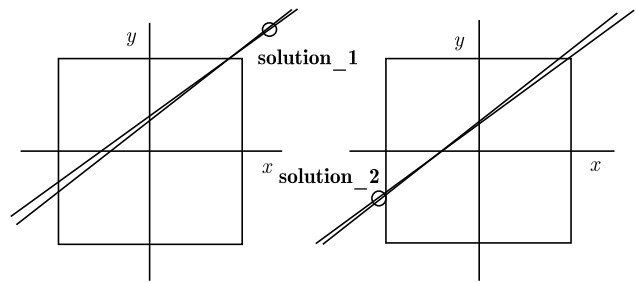
图 21-7 病态：数值解对于数据变化非常敏感，该图中两个线性方程十分相似，稍微改变线的方向将会极大地影响数值解
