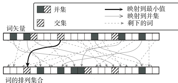
图 25-8 构建一个排列
