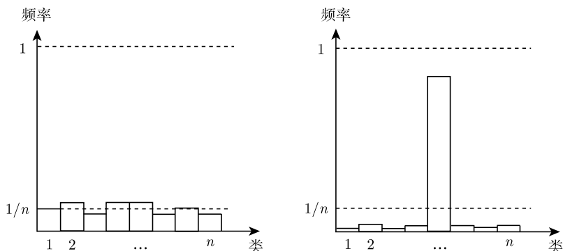
图 6-5 有着差别很大的熵的两个分布。高熵（左）：事件有相似的可能性，不确定性接近最高（ \log n ）。低熵（右）：事件有非常不同的可能性，不确定性非常小，接近零，因为某个事件占了大多数的概率
