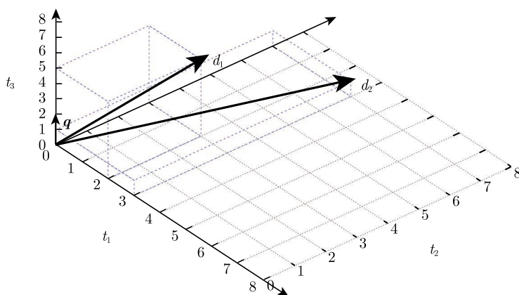
图 25-6 几何解释
