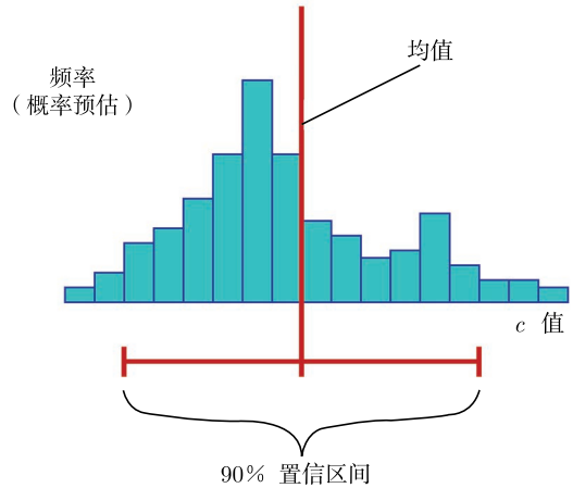
图 5-6 置信区间：从表征 c 估计值的分布的直方图中，可以推导出平均值区域周围 90% 的实例。也可以使用其他的置信水平，像 68.3%、95.4% 等（在正态分布的情况下对应于 \sigma 与 2\sigma 的历史概率值）
