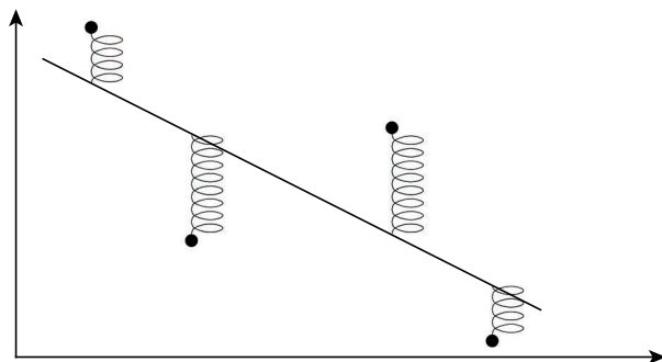
图 4-6 在物理学中，最小二乘拟合的原理类似于弹簧，最佳拟合的直线最小化整个系统中所有弹簧的势能（正比于弹簧长度的平方和）
