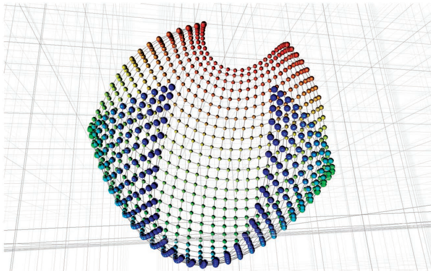
图 19-7 限制缺失的第一种解决方案：引入默认的互斥力
