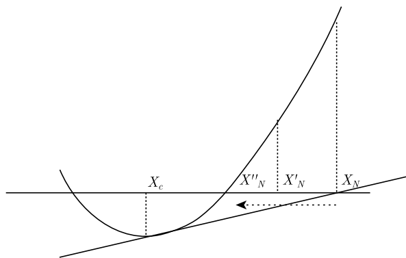
图 21-4 回溯：牛顿法的每一步都有方向
