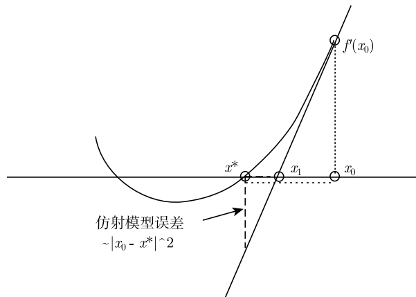
图 21-2 当起始点 x_0 离 x^* 很近时, 可以保证收敛
