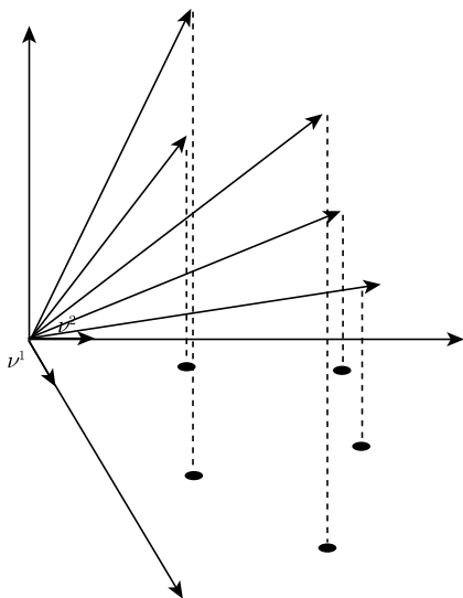
图 18-2 一个投影：每条虚线都连接着一个向量和其在由 \nu^1 和 \nu^2 定义的平面上的投影（在这种情况下，方向向量是 x 和 y 轴，通常情况下投影可以参照由任何两个不相关向量构成的平面）
