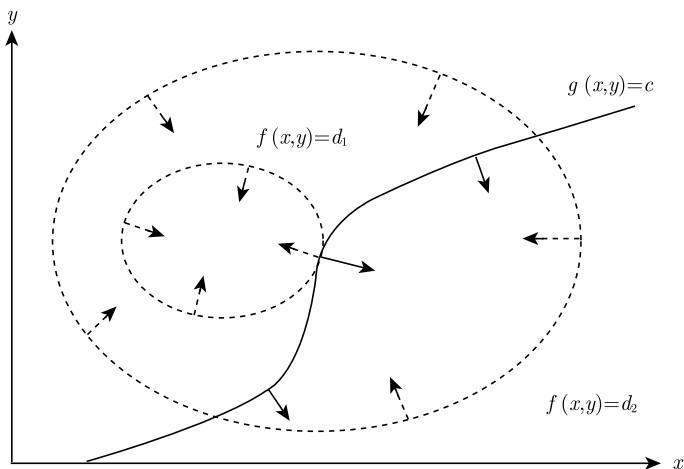
图 8-5 拉格朗日乘数法
