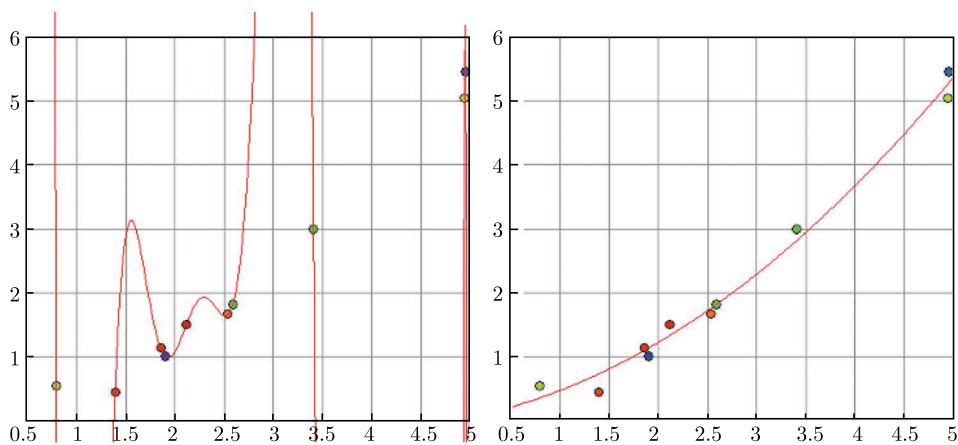
图 5-1 插值和拟合的比较。多项式的自由参数（等于其度数减 1）从数据点数目（左图）到 3 个（右图）的变化
