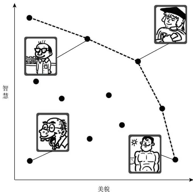
图 24-2 帕累托最优。所有像左下角那个人一样不占优的点都不会被列为最终候选。在帕累托边界(虚线)上的点需要进行权衡
