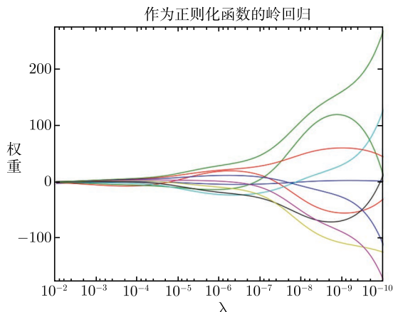
图 4-8 “岭”图，较大的 \lambda 值会导致总权重的收缩
