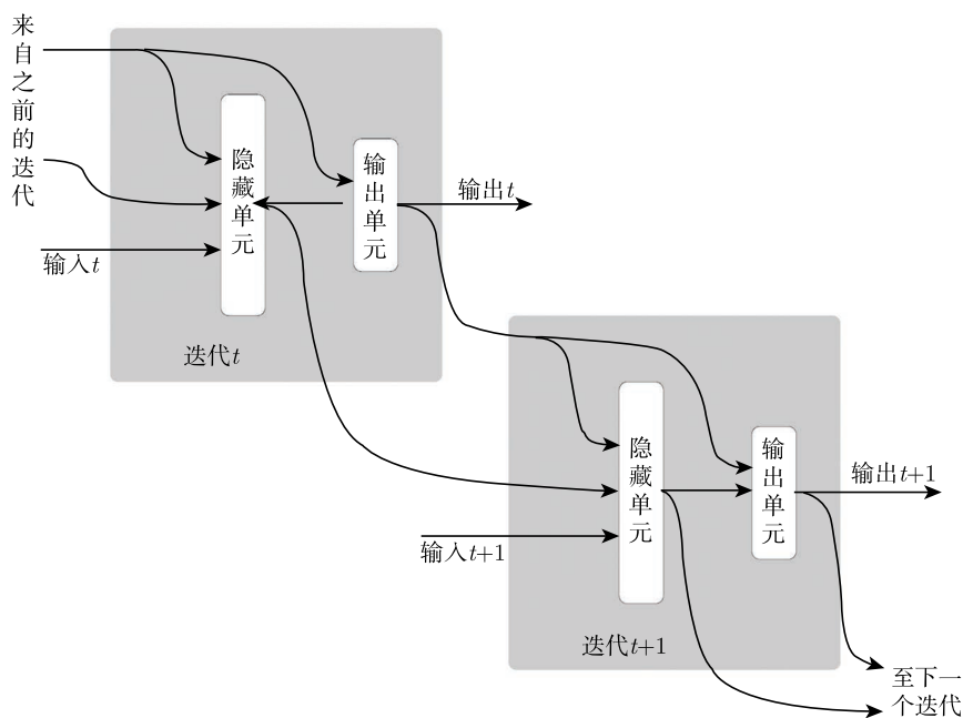
图 14-6 图 14-1 中的递归神经网络可以被瀑布状地展开成一个前馈网络，它的每一个前馈都是由当前迭代的输入和先前迭代的输入-输出组成
