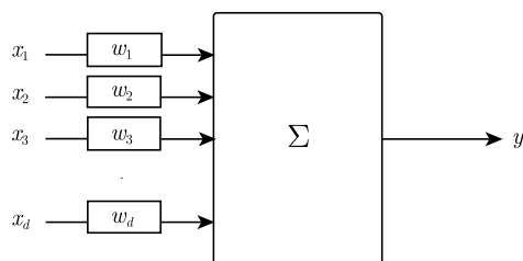
图 4-4 感知器：输入的加权和通过最终的“挤压”函数输出
