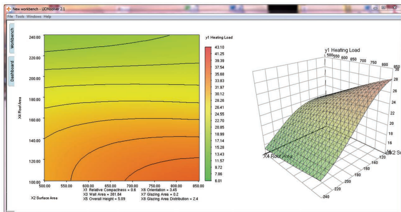
图 9-4 用 LION 软件 Sweeper 分析神经网络的输出。输出值和冬季加热房子消耗的能量,是输入参数的函数。图中展示了颜色编码的输出(左)和表面图(右)。非线性是可见的(另见彩插)
