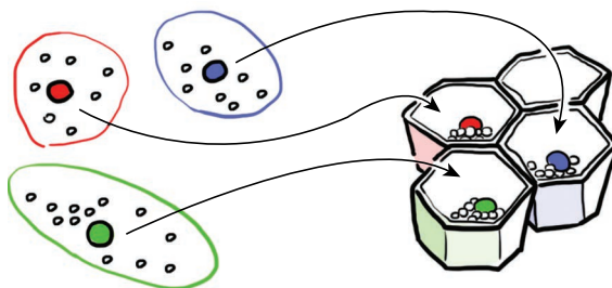
图 17-2 SOM 将多维空间中的实体映射到二维空间的神经细胞中，每个神经元拥有一个原型，并且每个实体都被映射到其最接近的那个神经元中
