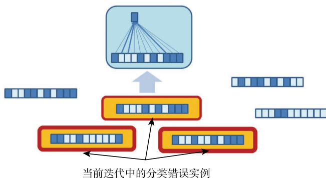
图 13-3 在提升法中，当训练新的模型添加到团体中时，当前迭代中分类错误的实例会被赋予更大的权重
