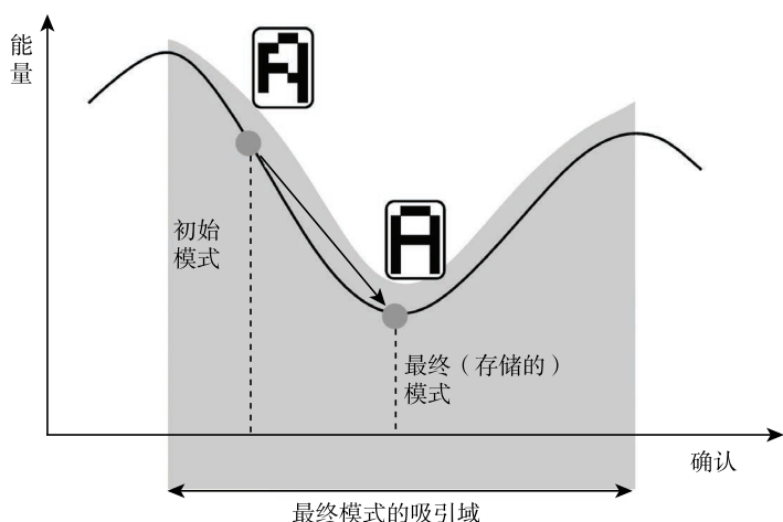
图 14-5 霍普菲尔德网络的能级相图，标出了其初始状态（曲线的上端），最终收敛的吸引状态和一个吸引域（阴影部分）
