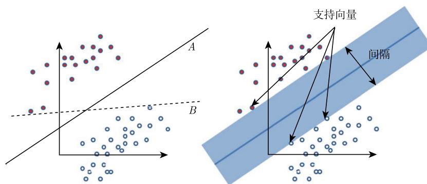
图 11-1 解释支持向量机的基础。线 A 的间隔比线 B 的要大。大的间隔会增加新实例落在分类器正确一侧的概率。支持向量是触及最大可能间隔的那些点
