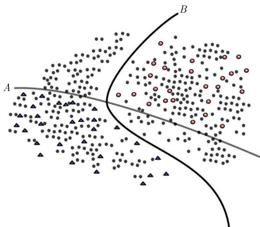
图 20-1 低密度分离假设。尽管界限 A 能完全区分两类，但是界限 B 更好，因为它穿过了一个低密度区域。未标记的数据会产生一个更好的分类器
