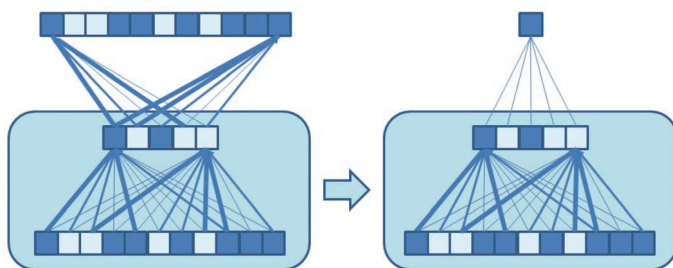
图 10-2 使用以未标记数据训练的自动编码器来初始化一个 MLP 网络
