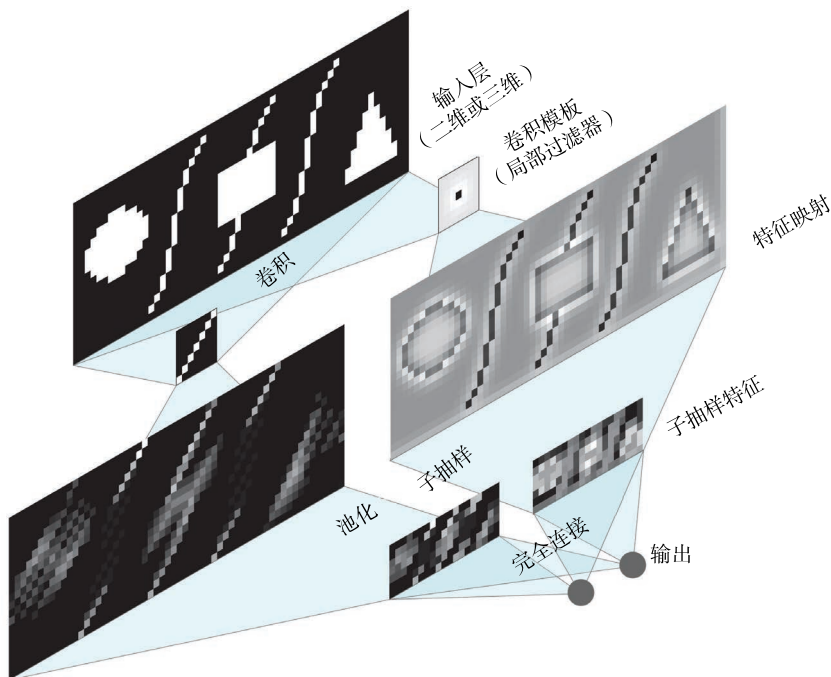
图 10-7 基本卷积网络：输入（图像像素）被针对一个输入权重的小型集合的卷积运算扫过，该卷积运算充当局部特征提取器。将所得的特征映射通过一个池化操作进行子抽样，而较小的神经元集合通过一个传统的完全连接输出层传递
