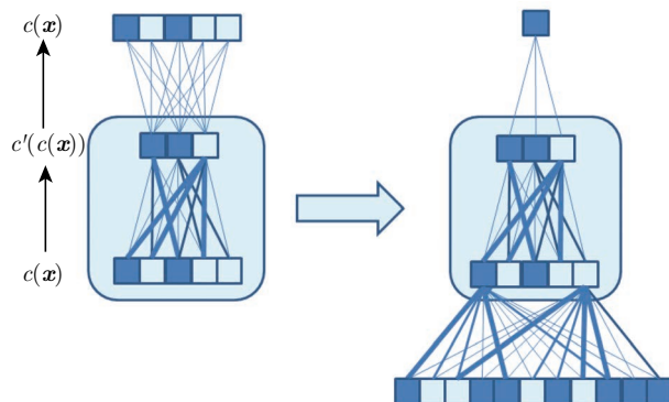
图 10-3 迭代训练自动编码器来构造更深的网络
