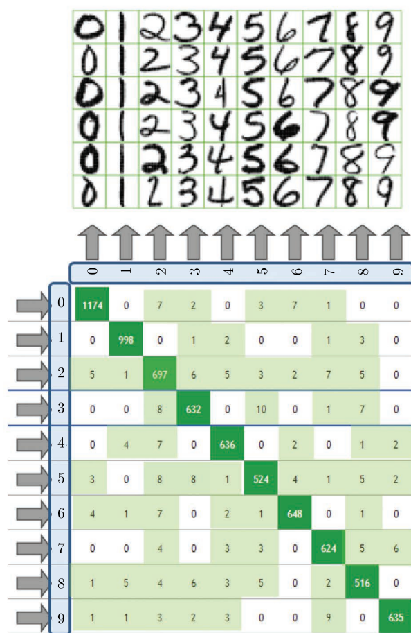
图 3-5 光学字符识别的混淆矩阵（手写的邮政编码数字）。其中的各种混淆也有道理可言。例如数字“3”被正确识别 632 次，被错认为“2”8 次，被错认为“5”10 次，被错认为“8”7 次。“3”从没有被错认为“1”或“4”，因为它们的形状差别太大了
