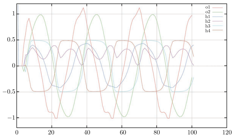
图 14-3 递归神经网络沿着环形训练：输出和隐藏层神经元（另见彩插）
