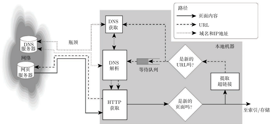
图 25-2 一个基本的爬虫结构：从网页中提取 URL 并加入队列；提前获取域名解析以防潜在的 DNS 瓶颈
