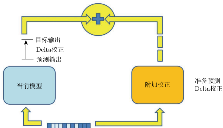
图 13-6 加性模型步骤：在训练实例上测量当前模型的误差。加入第二个模型是为了抵消这一误差
