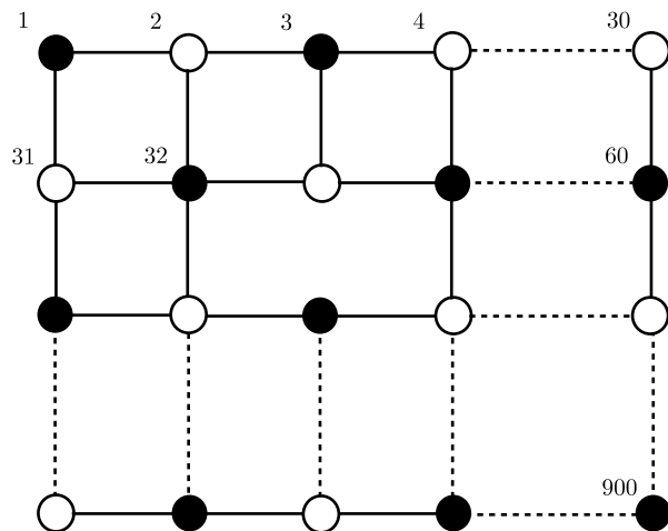
图 19-5 一个定义最邻近边的 30 \times 30 点阵
