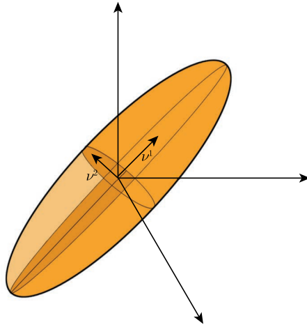
图 18-3 主成分分析，数据点分布在一个椭球体上。第一个本征向量在最长主轴的方向上，即沿着二维椭圆最长的轴，第二个本征向量在与第一个本征向量垂直的平面上
