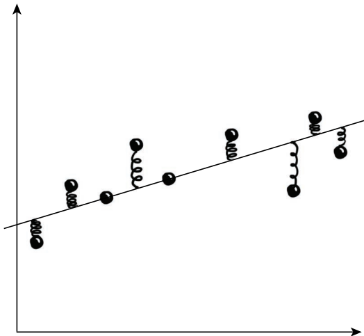
图 5-2 一条直线的拟合, 有一个物理的类比: 每个数据点与拟合直线间由弹簧连接。弹簧的强度正比于 1/\sigma_i^2 。能量最低的情况对应于最小的 \chi^2
