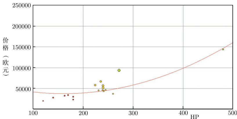
图 5-3 多项式拟合：作为发动机功率函数的车价
