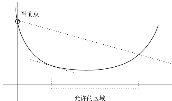
图 21-11 Armijo-Goldstein 条件
