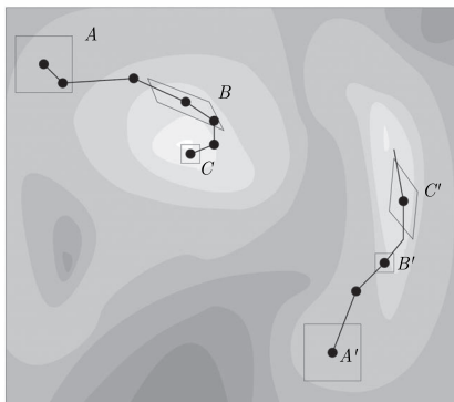
图 21-15 RAS 的几何示意图: 两条搜索轨迹得到两个不同的局部极小值, 改编自参考文献 [31]
