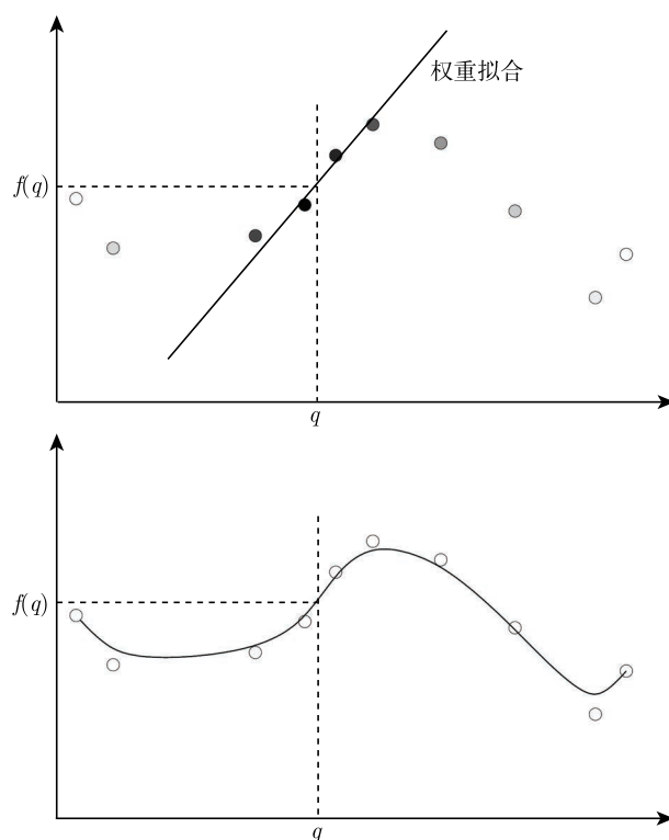
图 8-3 (上) LWR 模型在 q 点估值, 样本点的重要性由内部阴影表示; (下) 所有点的估值, 每个点对应一个不同的线性拟合
