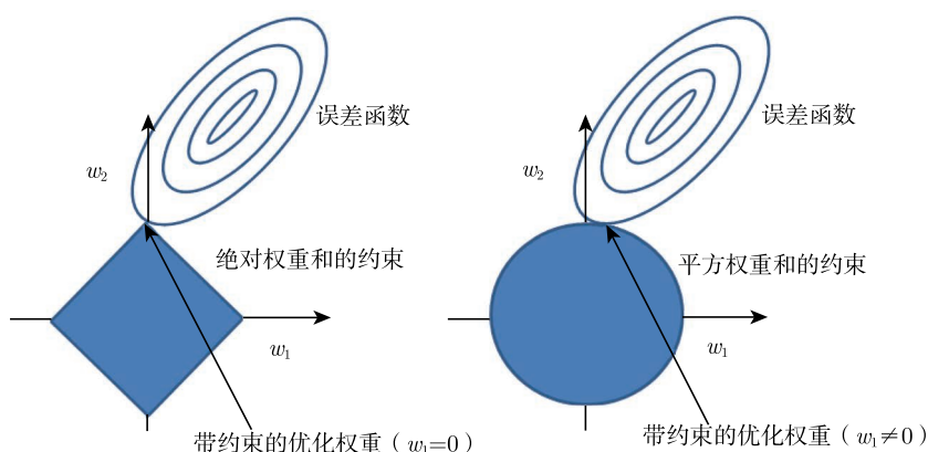
图 8-4 在 LASSO 中, 最好的解决方案出现在二次误差函数等高线接触正方形处, 有时会在正方形的角上, 对应某些零系数。相反, 岭回归的二次约束没有角来让等高线接触, 因此权重中很少会产生零
