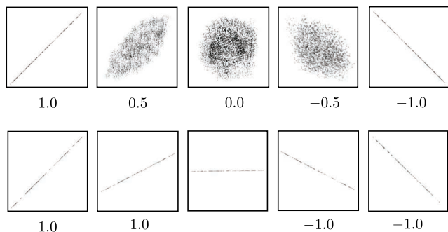
图 7-2 数据分布和对应的相关系数值的例子。记住，相关值都除以标准差，因此下面一排线性分布都有相同的最大相关系数（1 或 -1 ）
