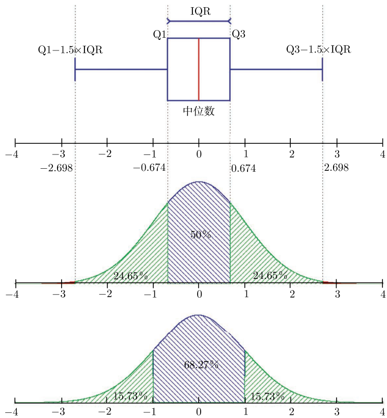
图 5-7 箱线图和正态分布之间的比较，横轴表示相对于标准偏差 \sigma 的位置。例如，在底部的图中，68.27% 的点落入距离平均值的一个标准差 \sigma 范围内
