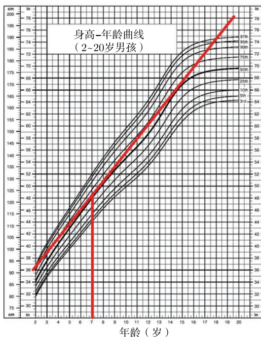
图 4-5 描述物理现象的函数一般都是平滑的。图中身高-年龄曲线可以用从 2~20 岁的切线逼近
