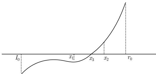
图 21-3 二分法示意图
