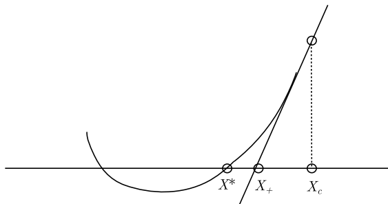
图 21-1 牛顿法的局部模型
