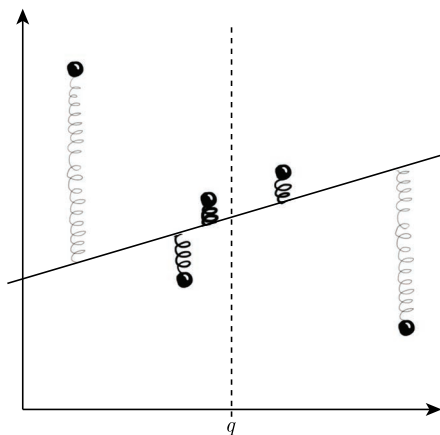
图 8-2 加权最小二乘拟合的弹簧类别（与图 4-6 比较）。现在，弹簧有不同的弹性常数，较粗意味着较硬，所以它们对整体势能的影响需要进行加权。对于上述情况，较硬的弹簧代表更靠近查询点 q 的那些点
