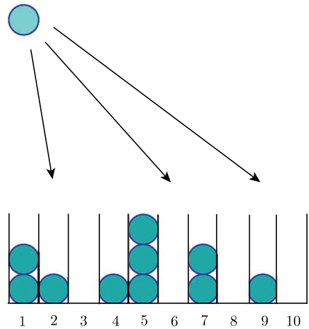
图 5-5 自助法：将 10 个球以均匀概率放在 10 个盒子里。自助法决定哪些实例和多少副本出现在自助样本里（实例 1 有两个副本，实例 2 有一个副本，实例 3 没有副本，等等）
