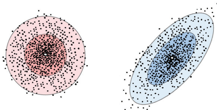
图 16-3 左图使用欧几里得距离作为差异性度量, 而右图使用马氏距离, 因其数据点分布呈椭球形
