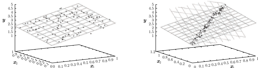
图 4-7 一个分布均匀的训练数据集（左侧）会得到一个稳定的数值模型，而一个糟糕的数据点选择将会得到许多差异很大的拟合平面，比如右侧图中的数据点几乎分布在一条直线上（引自参考文献 [9]）
