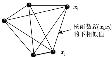
图 11-2 支持向量机学习的初始信息是每对输入点之间的相似性值 K(\mathbf{x}_i, \mathbf{x}_j) ，其中 K 被称为核函数。这些值，在某些条件下，可以理解为初始输入通过一个非线性函数 \phi(\mathbf{x}) 的映射后得到的标量积，但并不需要计算实际的映射，仅需要计算核的值（“核方法”）
