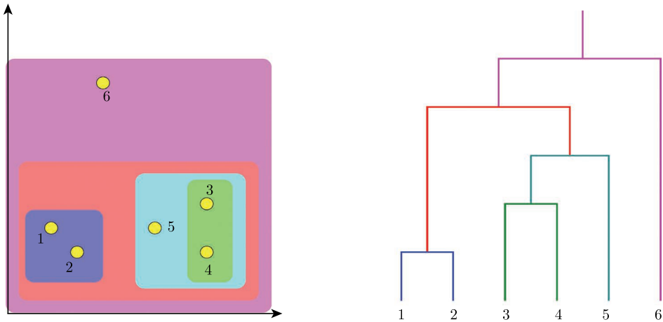
图 16-1 二维空间中数据点自底向上聚类示意图（使用标准欧几里得距离），每个数据点都由两个数值构成（另见彩插）
