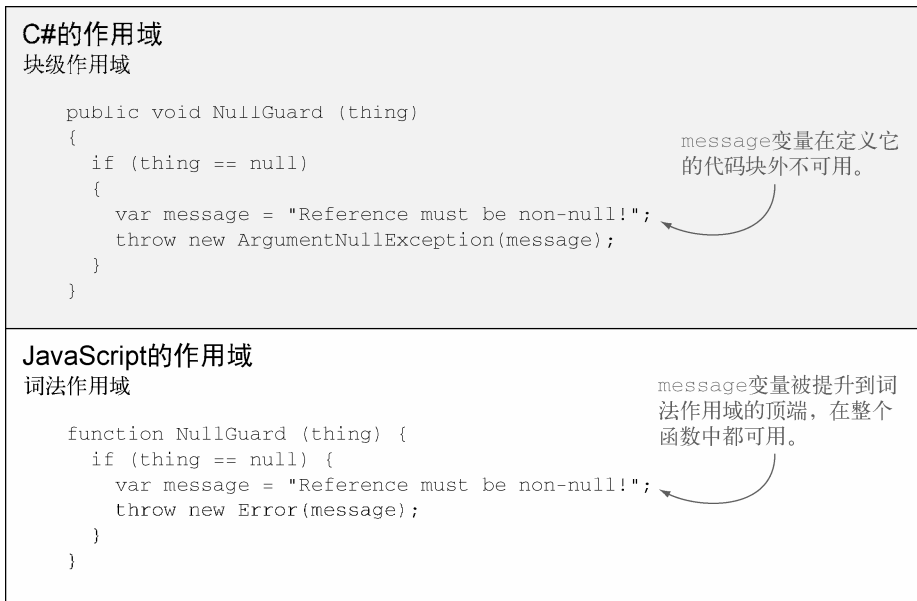
图5-2 作用域在不同语言中的差异
