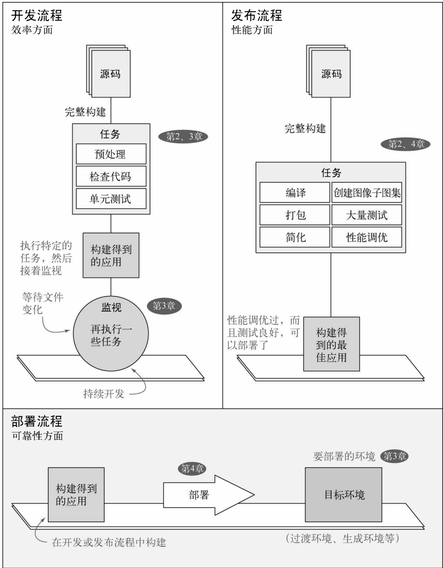
图2-4 构建和部署流程中关注的重点有所不同
