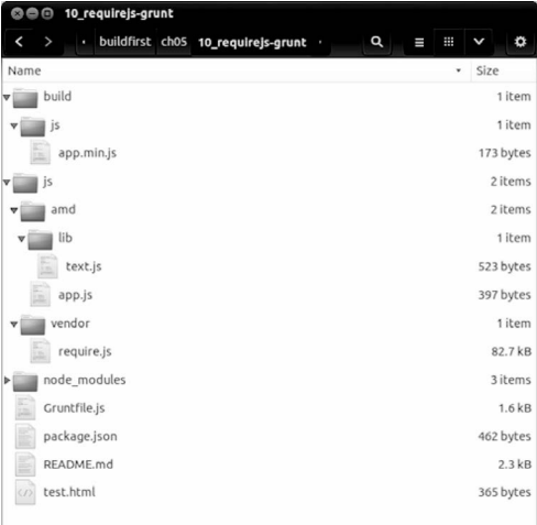
图5-4 在Grunt构建过程中使用RequireJS得到的典型目录结构
