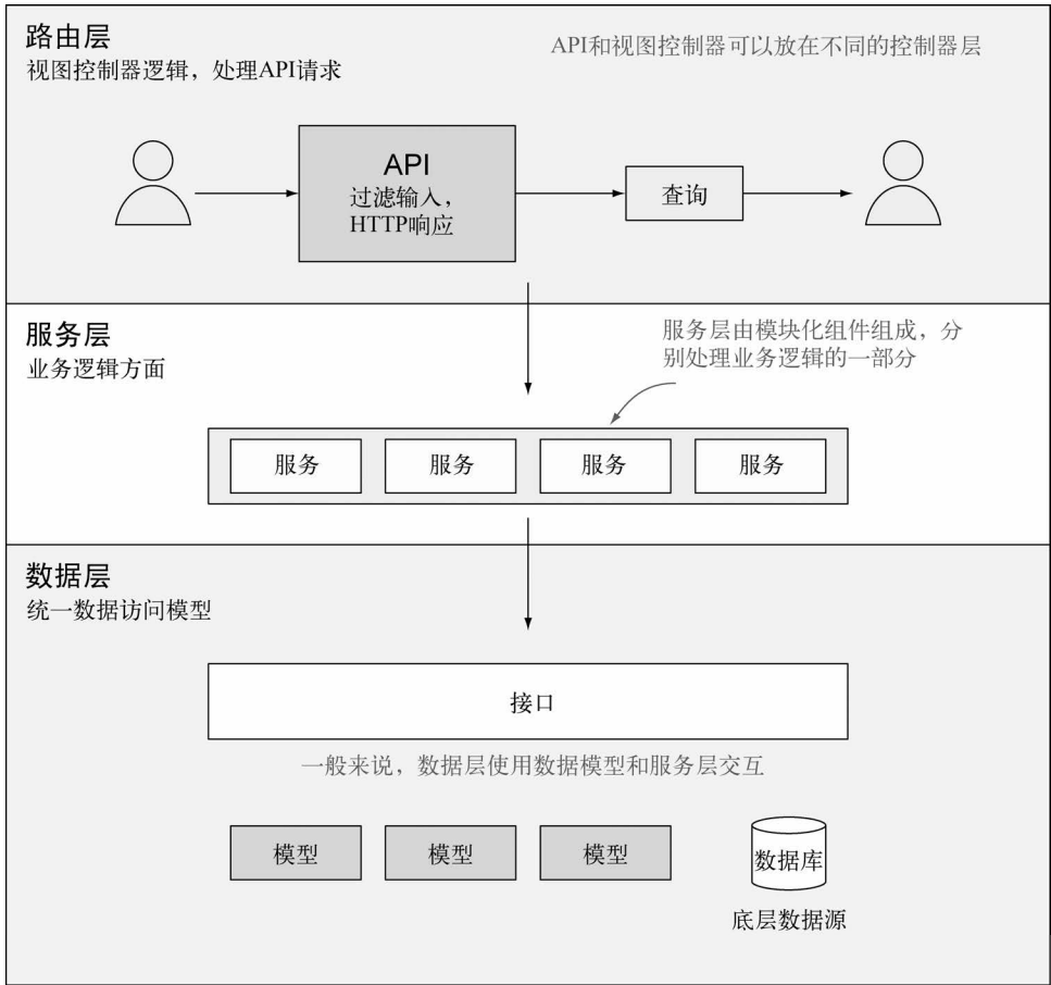
图9-1 三层服务架构概览
