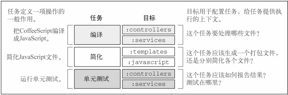
图2-1 Grunt一览：任务和目标都在配置中
