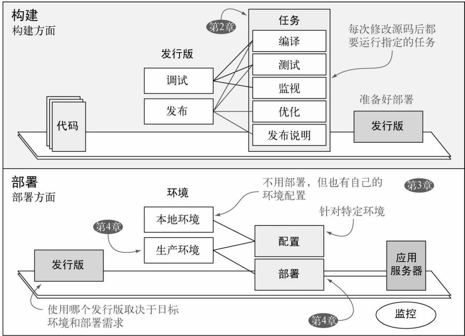
图1-2 构建优先原则中的构建和部署过程
