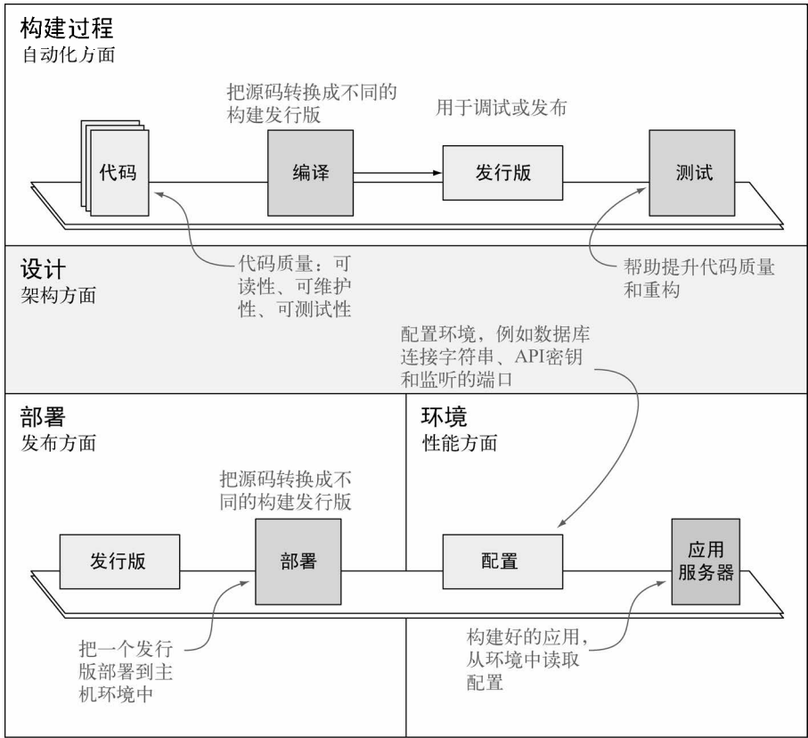
图1-1 概览构建优先原则关注的四个方面：构建过程，设计，部署和环境
