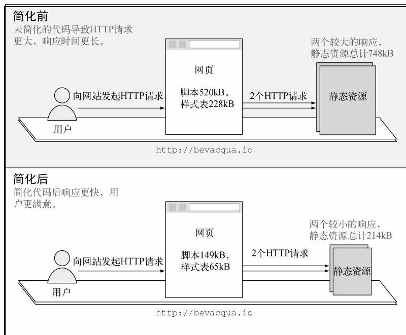
图2-6 简化静态资源，减小HTTP响应的长度
