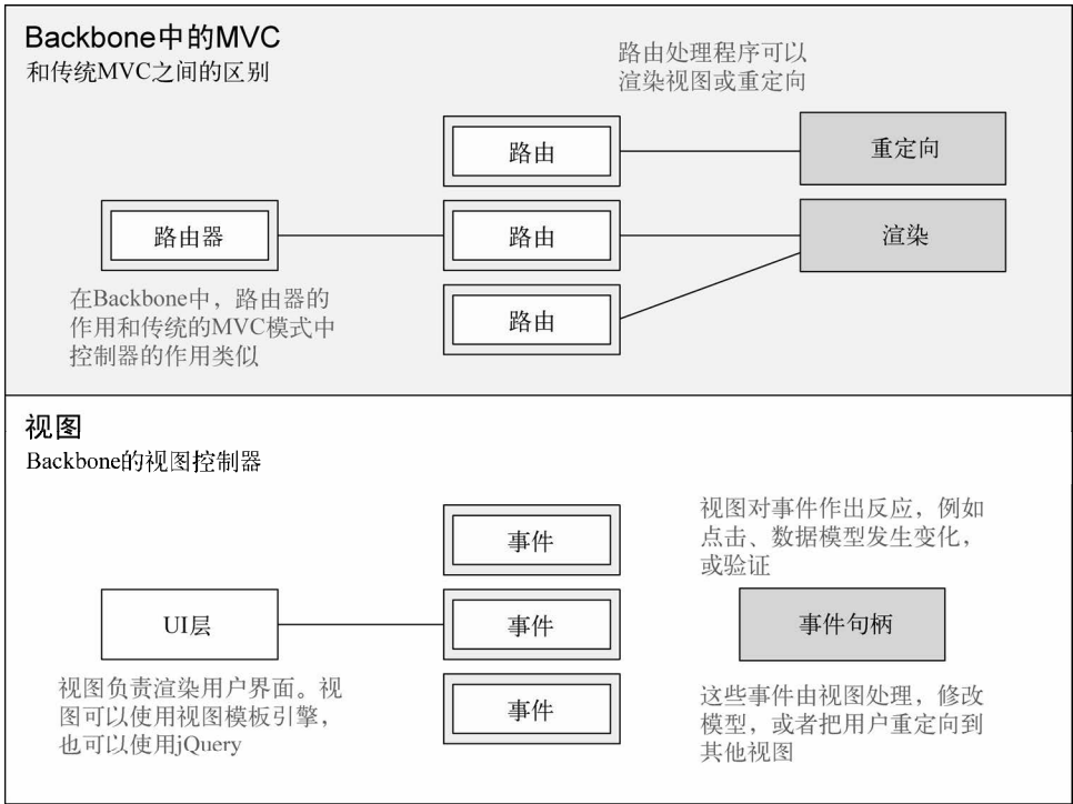
图7-3 Backbone处理MVC模式中面向用户部分（处理事件、验证和渲染UI）的方式
