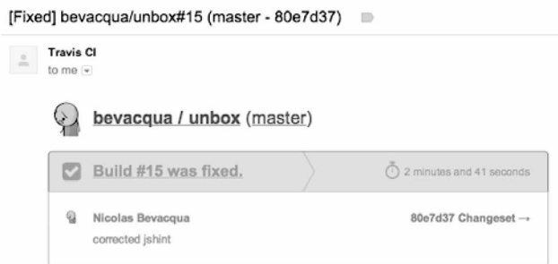
图4-5 Travis发送的通知邮件，告诉你构建问题修复了
