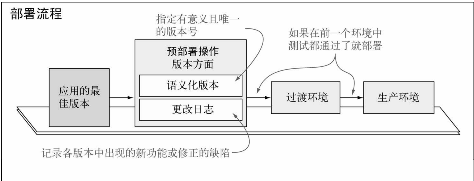
图4-2 发布前为应用设定版本号和逐步部署转出。在过渡环境中由QA团队测试能确保部署到生产环境之前应用是稳定的
