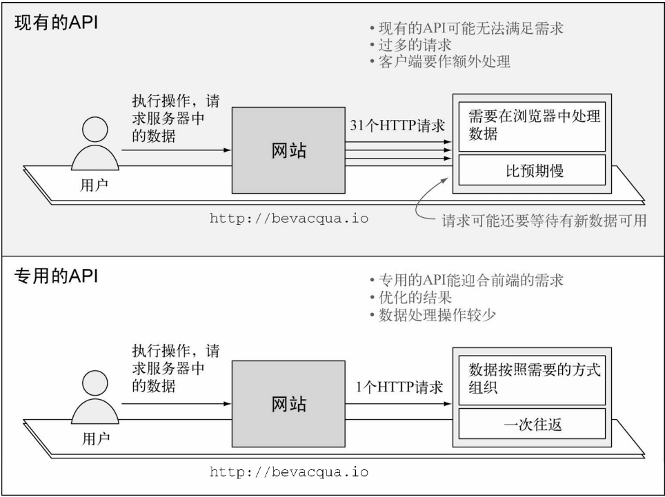
图6-1 在现有的API和专为前端设计的API之间权衡
