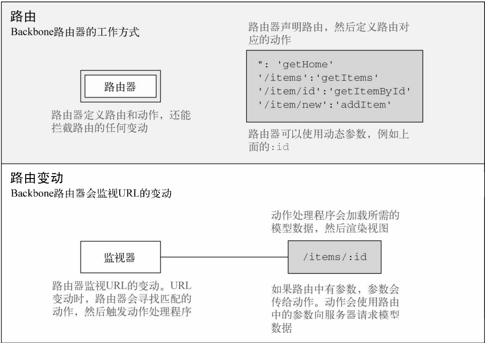
图7-4 Backbone的路由和路由监视器
