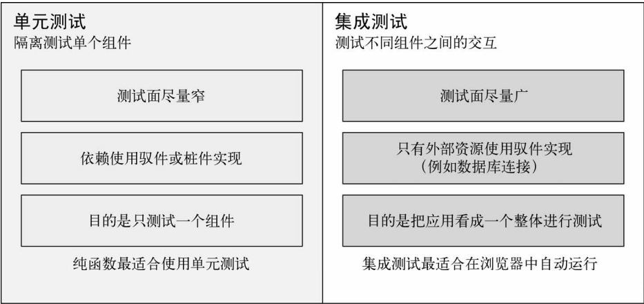
图8-1 单元测试和集成测试之间的区别。注意，这两种测试都要编写，二者之间不是相互排斥的。纯函数将在8.1.15节讨论
