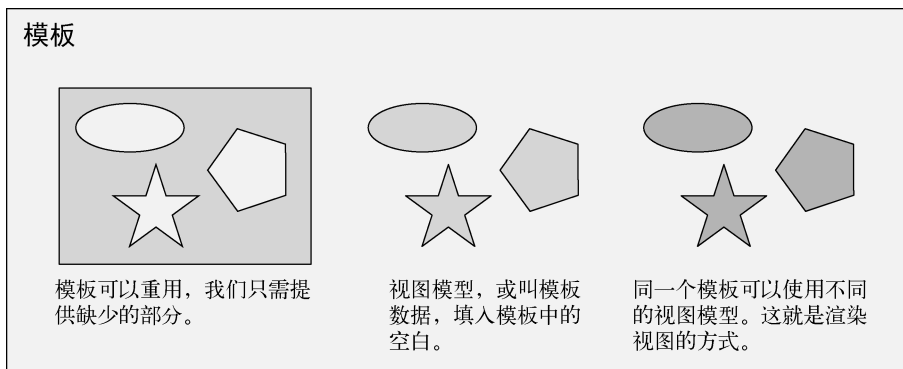
图7-1 不同的数据模型重用相同的模板
