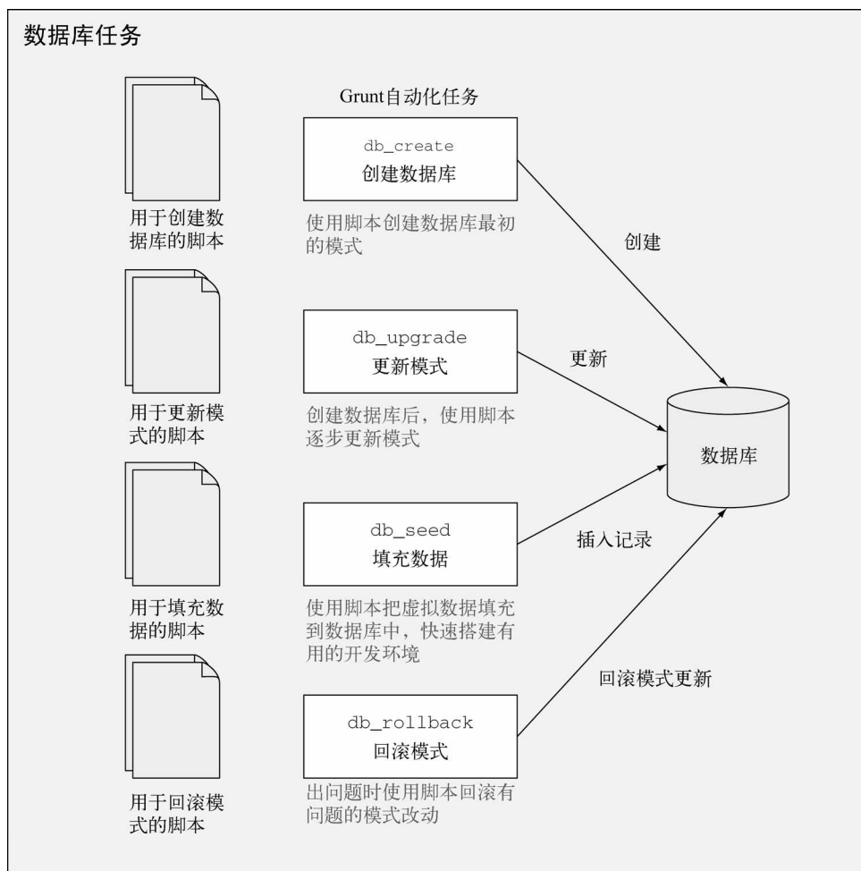
图2-7 任务与数据库实例的交互
