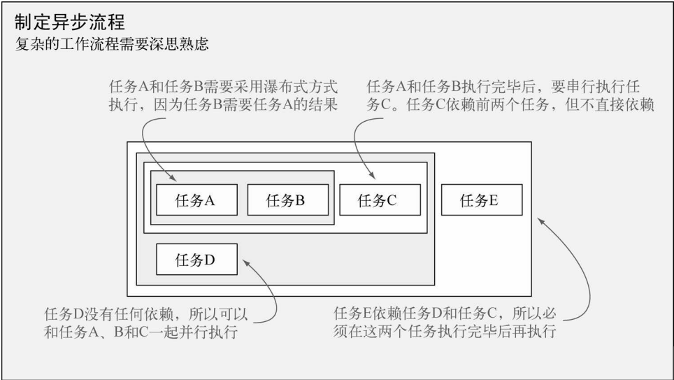
图6-4 剖析一个复杂的异步流程。提示：在脑海中要按照任务的需求区分各个任务
