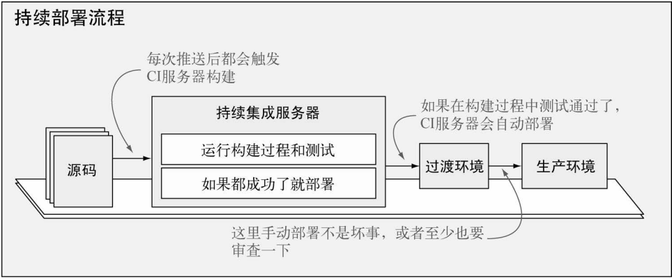
图4-6 建议使用的持续部署流程
