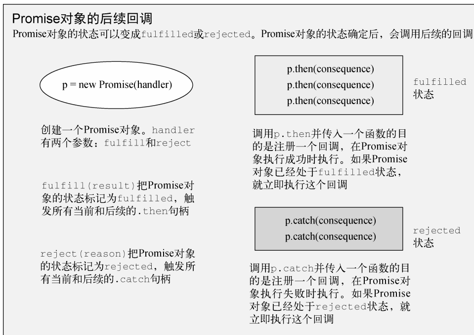
图6-5 Promise对象的后续回调
