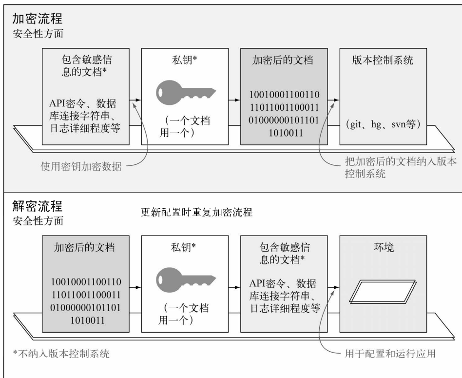
图3-3 使用RSA密钥加密和解密配置的流程
