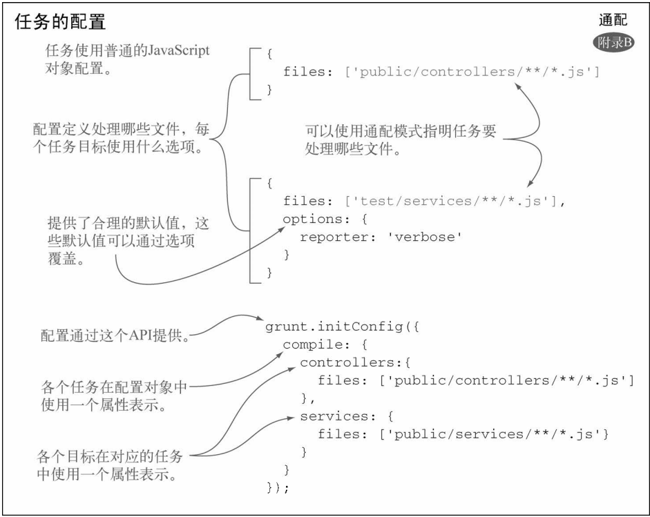
图2-2 Grunt任务配置的代码详解图。每个任务和任务目标都单独配置。
