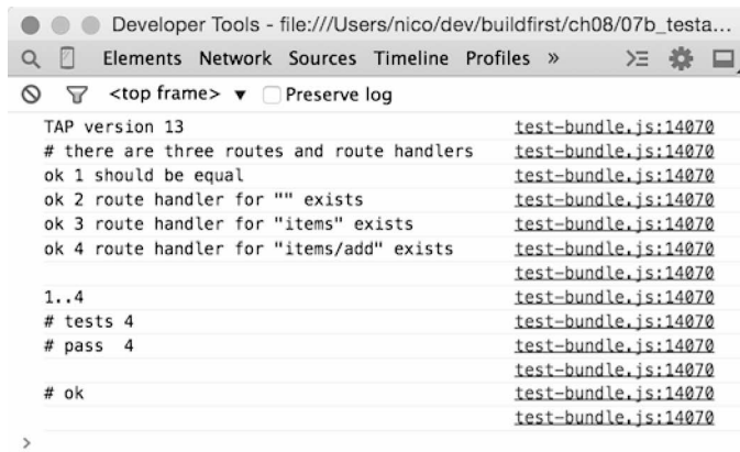
图8-5 开发者工具中显示的测试结果
