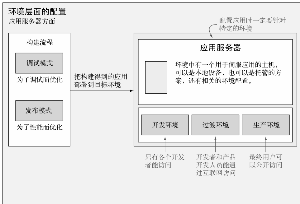
图3-2 环境层面的配置——环境、配置和发行版一起组成一个应用。环境的配置包括机密凭据和不同环境之间可能有所不同的配置。
