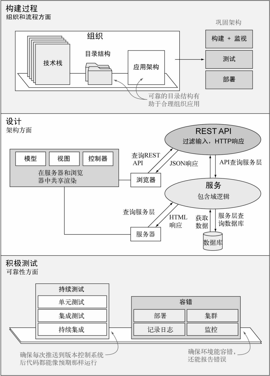
图1-4 务实的架构方式
