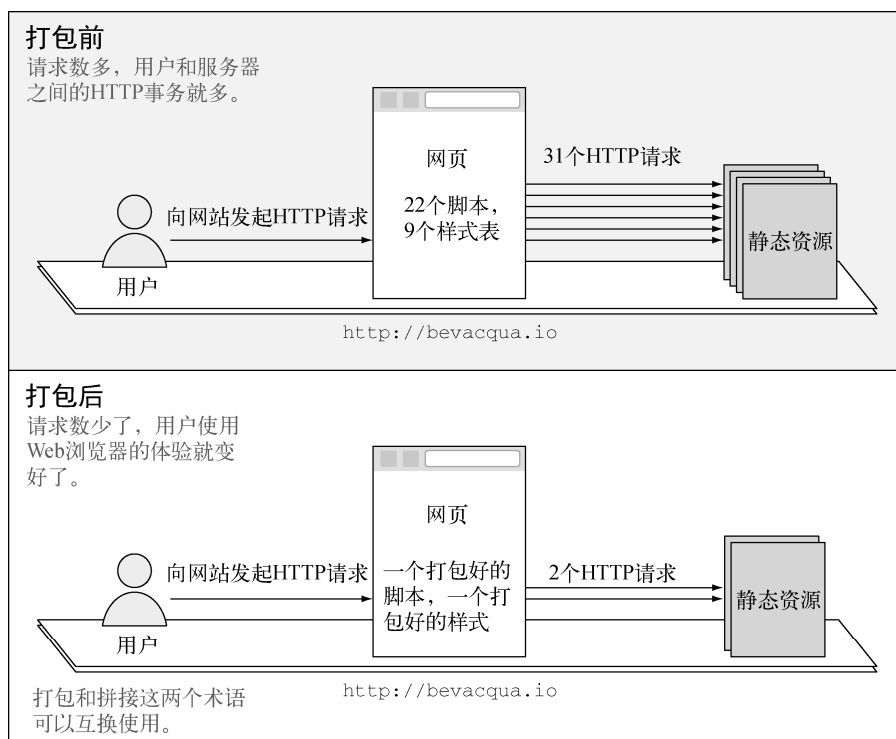
图2-5 打包静态资源，减少HTTP请求数
