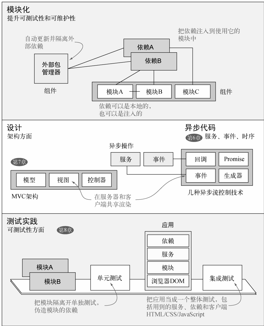
图5-1 模块化、好的架构和测试是设计可维护的应用的基础
