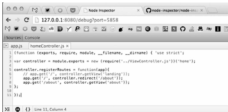
图4-7 使用Node检查器在Chrome中调试Node.js代码
