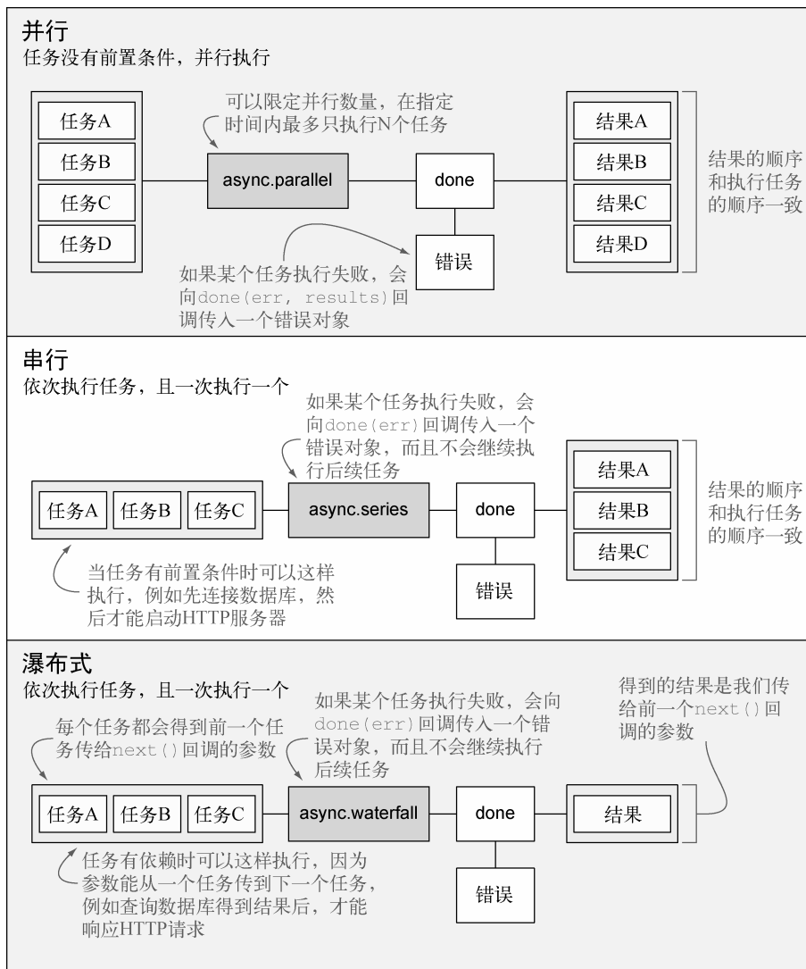
图6-3 比较async库中的并行、串行和瀑布式流程控制方法
