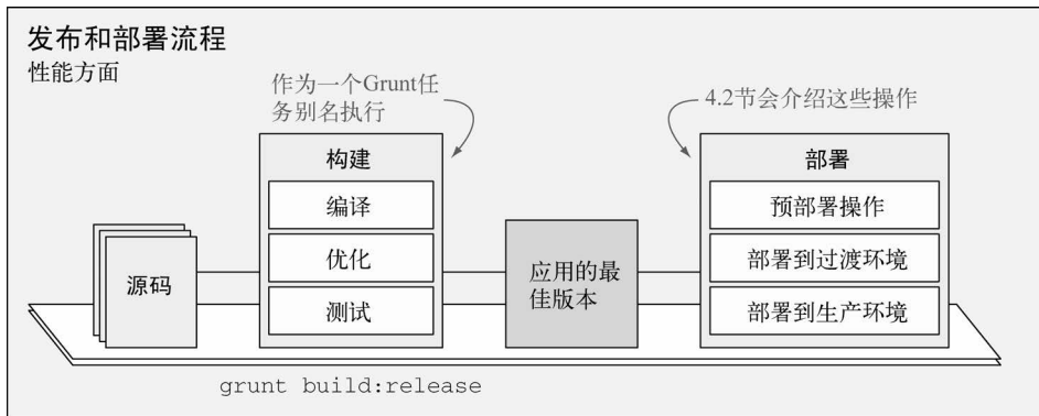
图4-1 推荐的发布和部署流程
