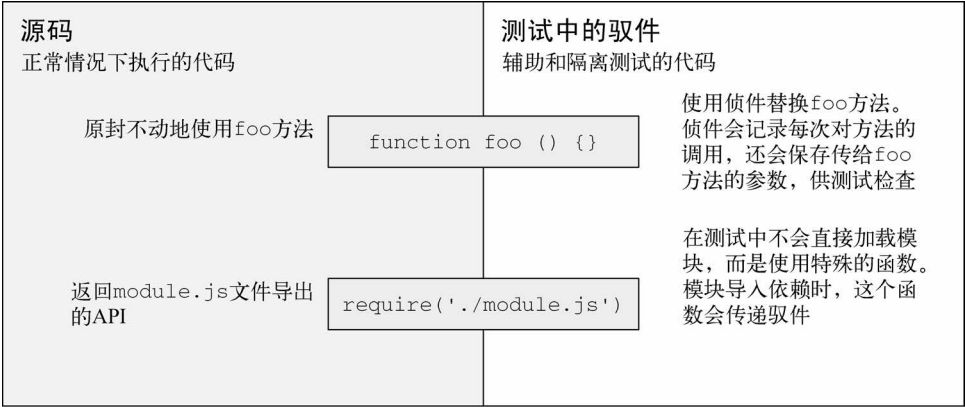
图8-2 测试时原封不动地使用源码与使用驭件的对比
