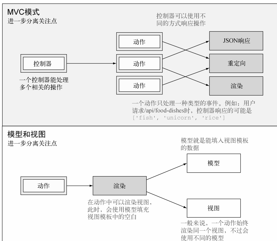
图7-2 MVC模式把关注点分离到控制器、视图和模型中
