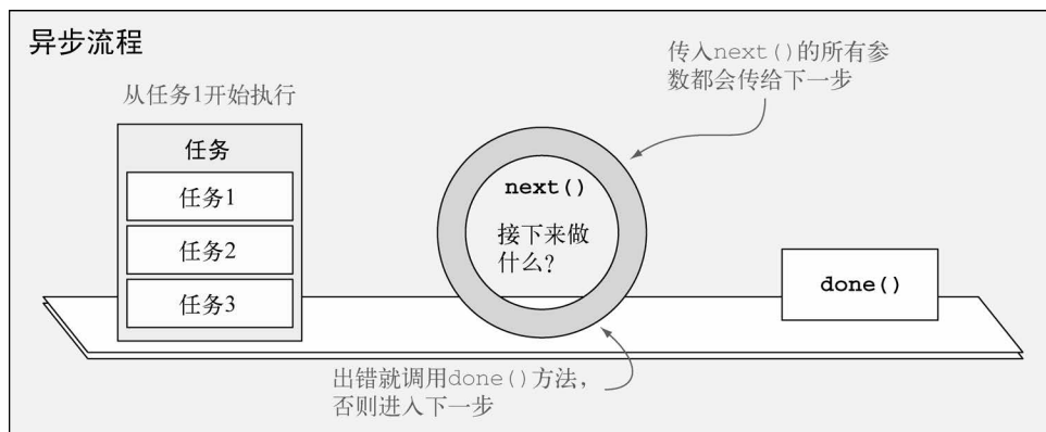
图6-2 理解异步流程方法
