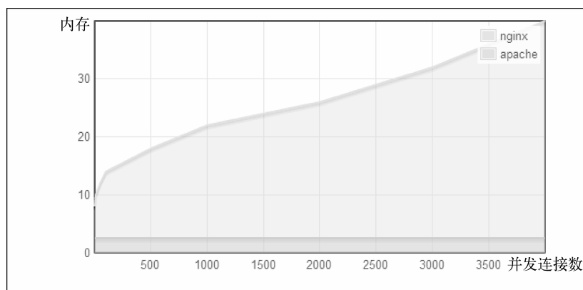
Apache和Nginx处理并发请求时的内存占用对比
