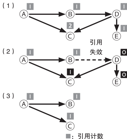
图 3 引用计数算法
