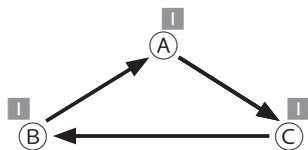
图4 无法回收,循环引用
