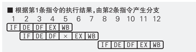
图 2 分支冒险
