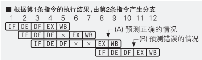
图 3 分支预测
