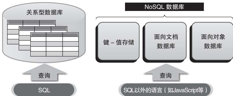
图 1 NoSQL 数据库
