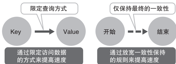
图 2 NoSQL 的优点
