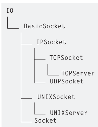
图 4 套接字相关的类
