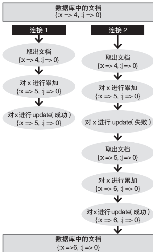
图3 成功的并发控制
