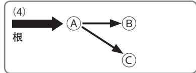
图 1 标记清除算法
