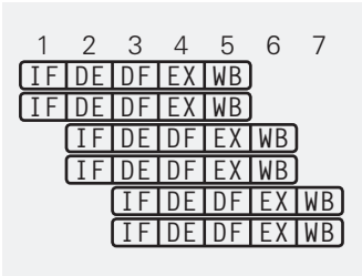
图 4 超标量执行
