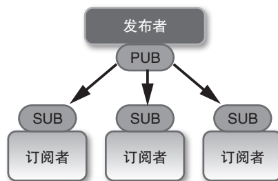
图 2 PUB/SUB 模型
