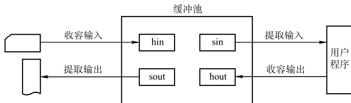
图 5-8 缓冲区的工作方式
