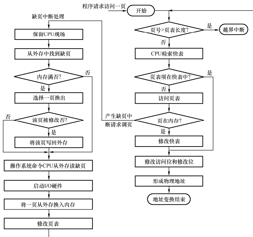
图 3-24 请求分页中的地址变换过程
