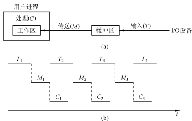
图 5-5 单缓冲工作示意图
