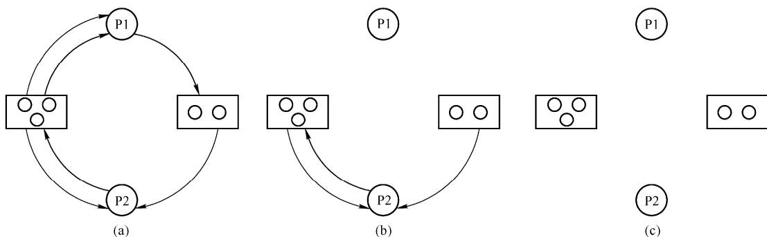
图 2-18 资源分配图的化简
