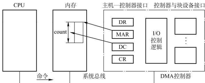
图 5-2 DMA 控制器的组成
