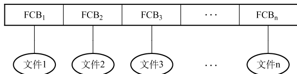
图 4-3 单级目录结构
