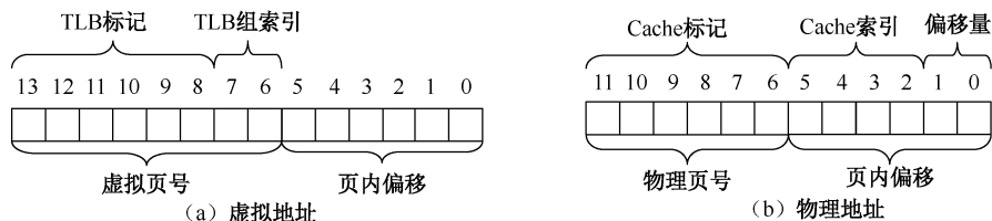
图 3-29 地址格式
