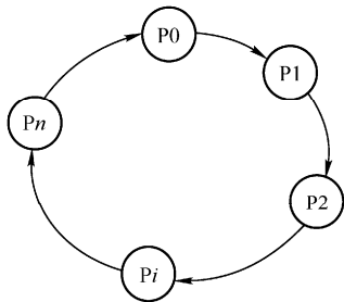
图 2-15 循环等待
