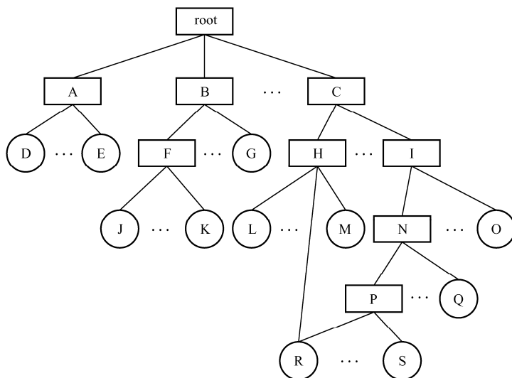
图 4-9 文件系统
