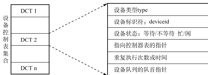
图 5-9 设备控制表
