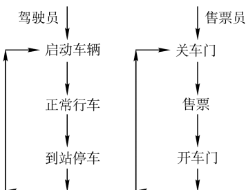
图 2-14 驾驶员和售票员
