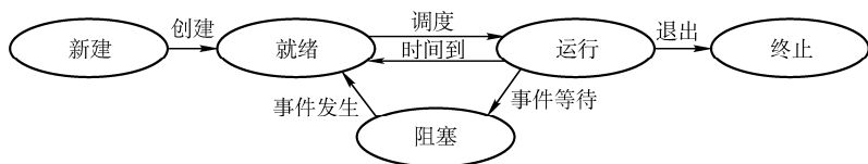
图 2-1 五种进程状态的转换
