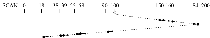
图 4-27 SCAN 磁盘调度算法
