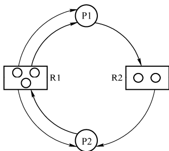
图 2-17 资源分配示例
