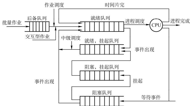
图 2-4 处理机的三级调度
