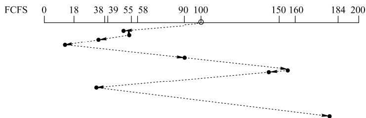
图 4-25 FCFS 磁盘调度算法
