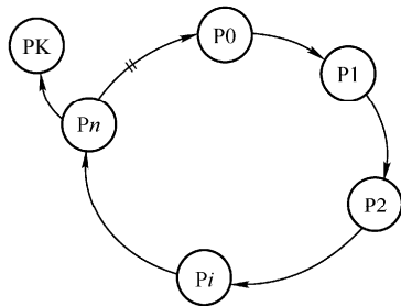
图 2-16 满足条件但无死锁
