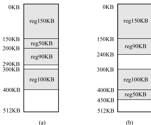
最先适配分配情况
