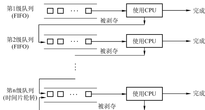
图 2-5 多级反馈队列调度算法
