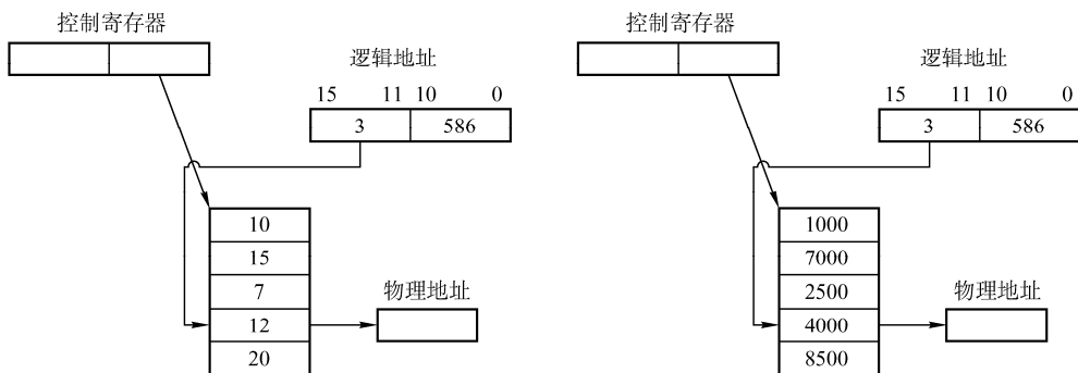
图 3-21 地址变换示意
