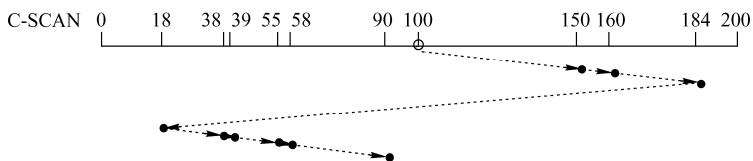
图 4-28 C-SCAN 磁盘调度算法
