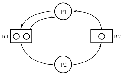
死锁点的资源分配图
