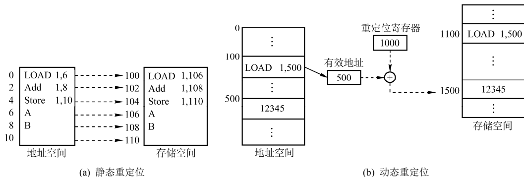
图 3-2 重定向类型
