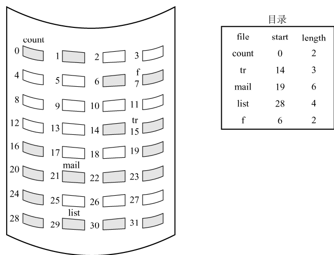
图 4-12 连续分配
