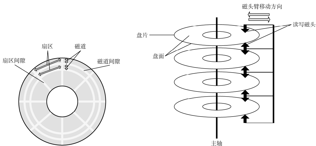
图 4-23 磁盘盘片
