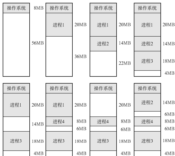
图 3-6 动态分区
