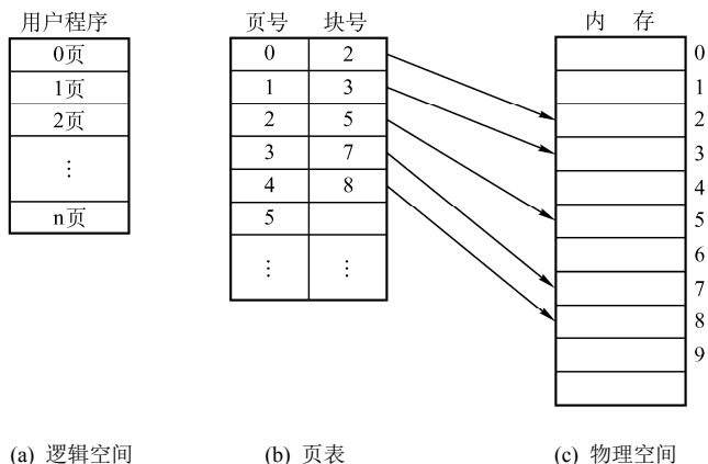
图 3-8 页表的作用
