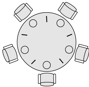
图 2-10 5 名哲学家进餐
