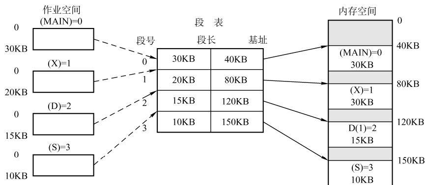
图 3-15 利用段表实现地址映射
