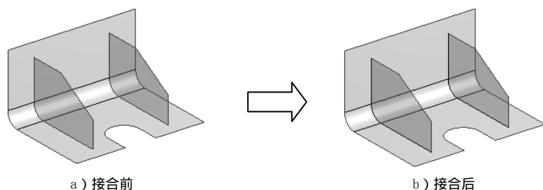
图 3.5.19 接合操作
