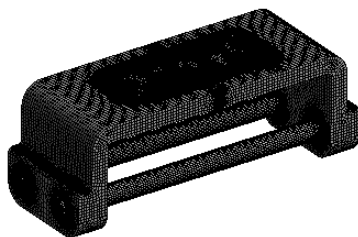
图 4.9.2 装配体网格划分
