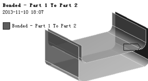
图 7.6.87 定义壳体接触（二）
