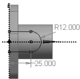
图 3.3.20 截面草图 3
