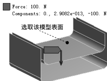
图 7.6.90 添加载荷力
