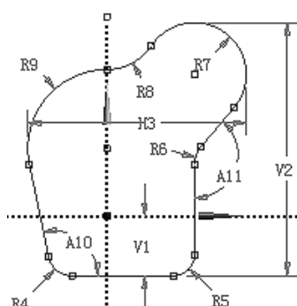
图 3.8.11 添加角度尺寸约束
