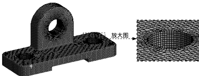
图 4.7.14 网格应用 Sizing 控制(二)
