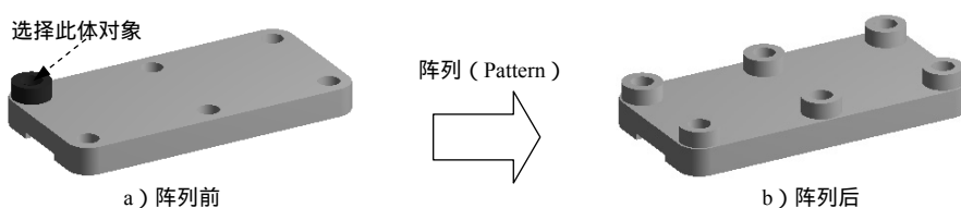
图 3.4.34 创建矩形阵列
