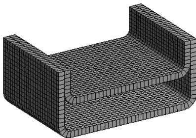
图 7.6.80 划分网格
