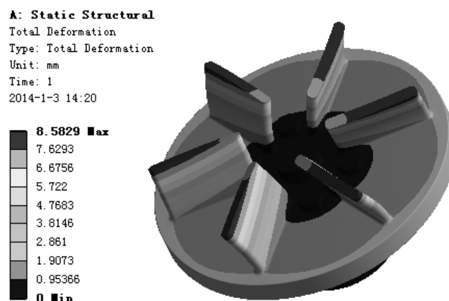
图 7.6.14 位移变形结果图解
