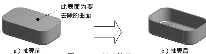
图 3.3.43 抽壳特征
