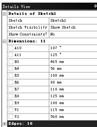
图 3.8.12 修改尺寸
