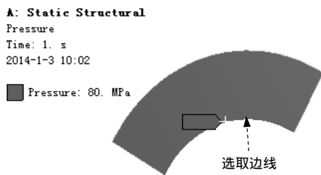
图 7.5.37 添加压强载荷
