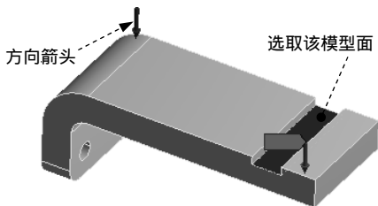
图 7.2.10 添加载荷力
