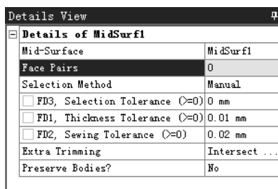
图 3.5.17 “Details View”对话框
