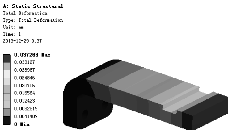
图 7.2.13 位移变形结果图解
