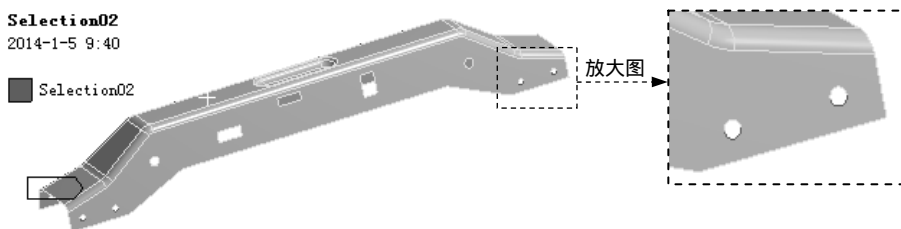
图 9.5.16 创建命名选择集 Selection02
