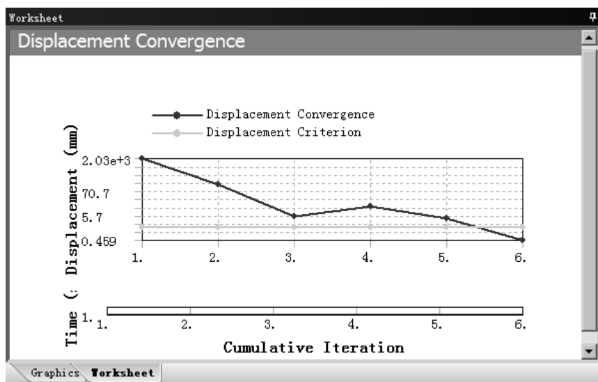
图 8.6.20 位移收敛图表
