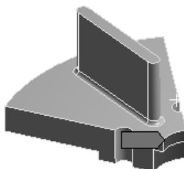
图 9.2.11 添加固定约束
