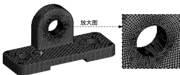
图 4.7.12 网格应用 Sizing 控制一
