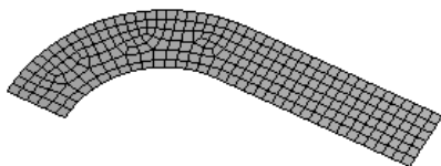
图 7.5.57 划分网格
