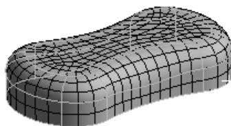
图 4.4.2 网格划分
