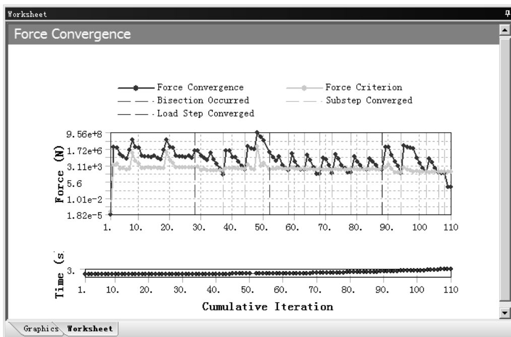
图 8.5.3 收敛曲线
