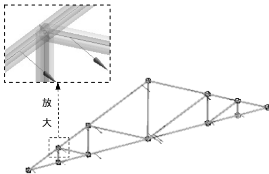
图 3.7.17 梁结构建模
