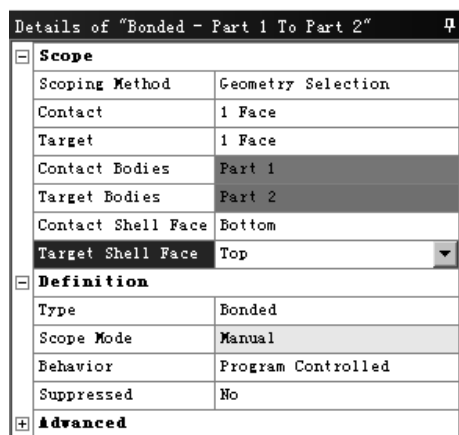
图 7.6.83 “定义接触参数”对话框
