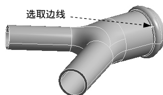
图 4.4.9 分割边（二）
