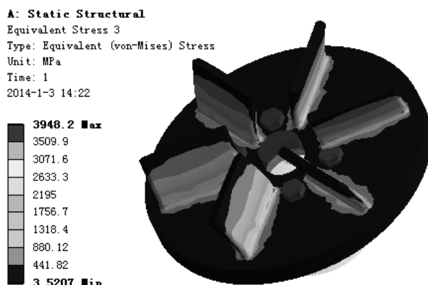
图 7.6.16 应力结果图解 (fan wheel)
