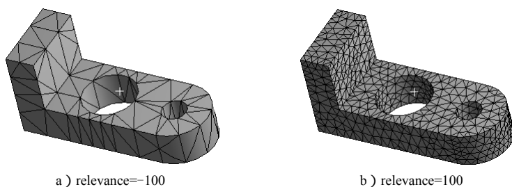
图 4.2.5 控制网格划分总体质量
