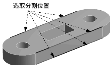
图 4.4.41 分割边（二）
