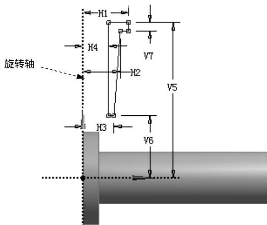
图 3.13.20 草图 4
