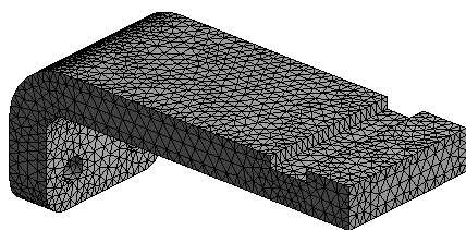
图 7.2.6 全局网格控制
