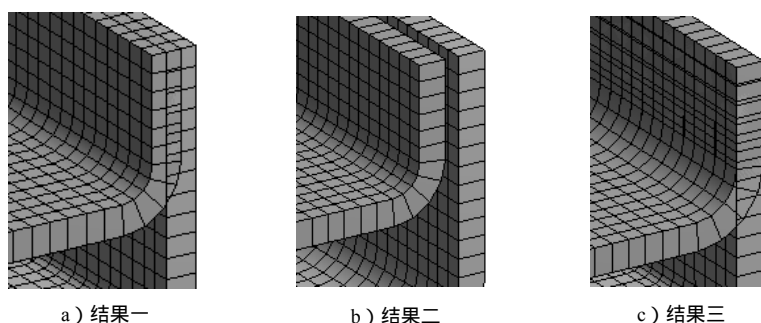
图 7.6.81 壳体厚度方向与网格划分之间的关系
