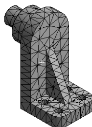
图 4.3.4 自动网格划分（不规则）
