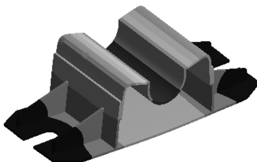
图 7.7.26 位移变形结果图解
