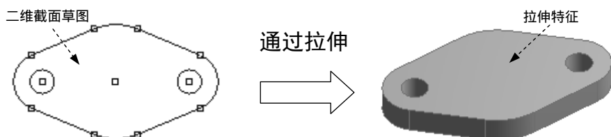
图 3.3.10 拉伸特征
