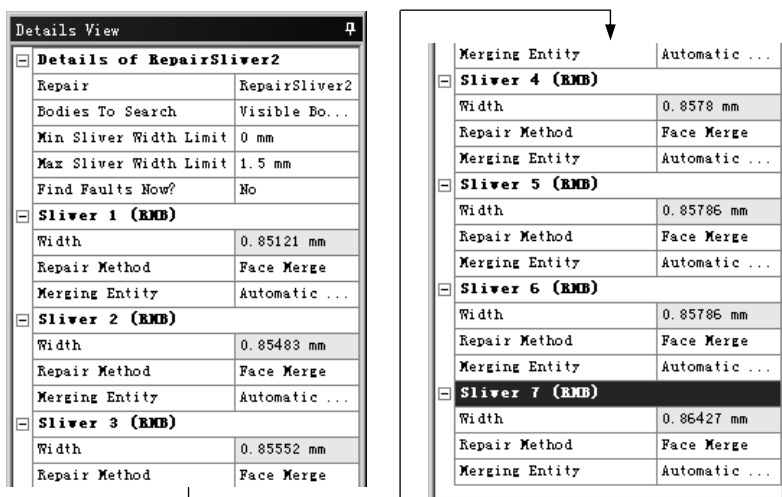
图 3.5.41 “Details View”对话框（二）
