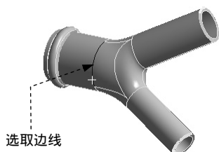
图 4.4.20 分割边（一）
