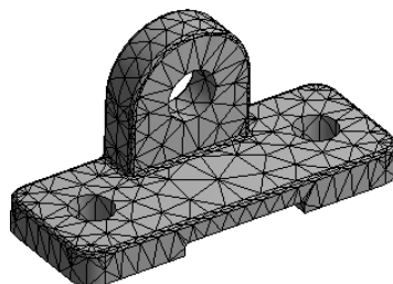
图 4.7.6 网格划分结果
