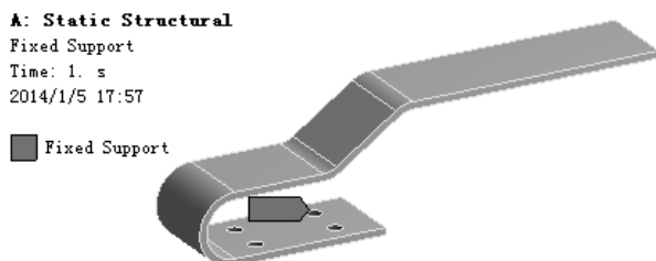
图 8.6.12 添加固定约束条件
