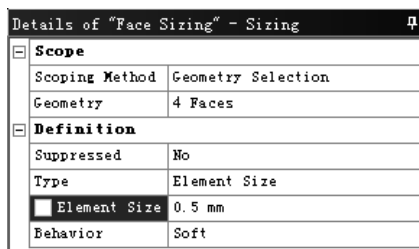
图 4.7.13 “Details of “Sizing” -Sizing”对话框
