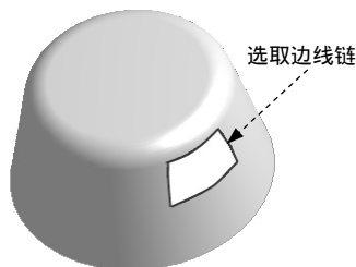
图 3.5.12 定义修补边界
