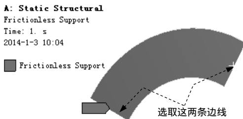
图 7.5.39 添加无摩擦支撑约束
