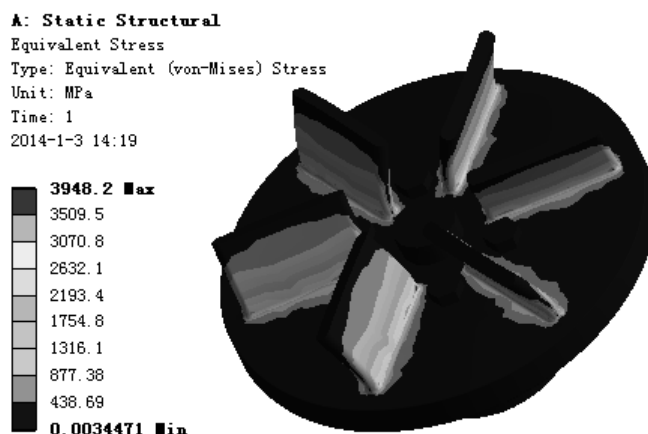
图 7.6.13 应力结果图解
