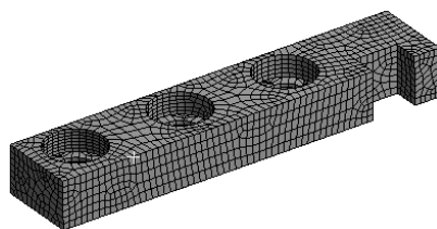
图 4.3.10 六面体网格划
