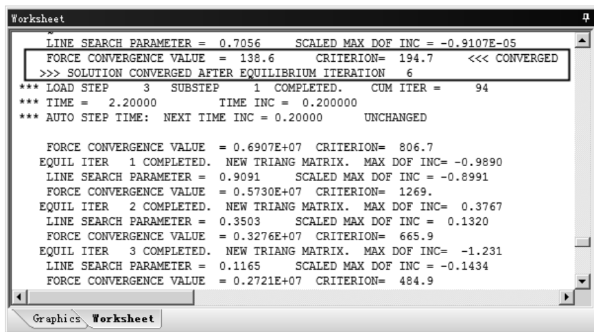
图 8.5.2 力收敛信息
