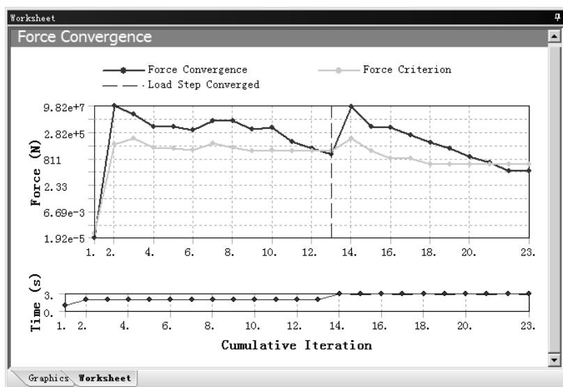
图 9.7.30 力收敛图解
