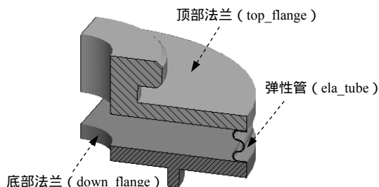
图 9.7.2 弹性管连接组件结构
