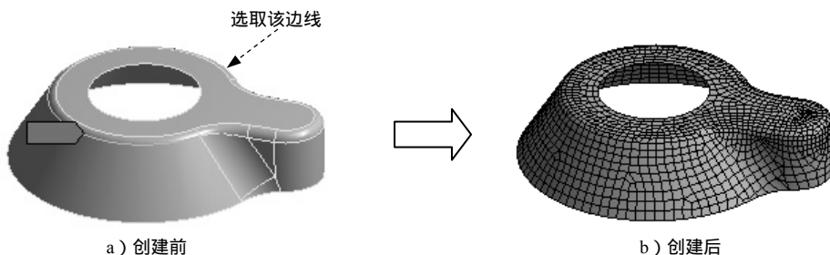
图 4.3.23 划分网格
