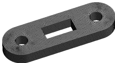
图 4.4.56 调整后的网格结果
