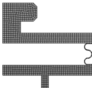
图 9.7.21 划分网格
