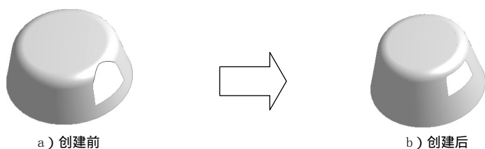
图 3.5.4 延伸曲面
