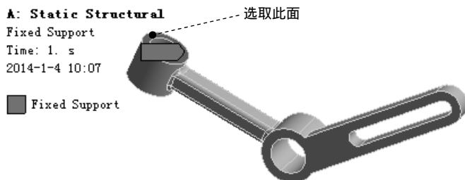
图 9.1.7 添加固定约束
