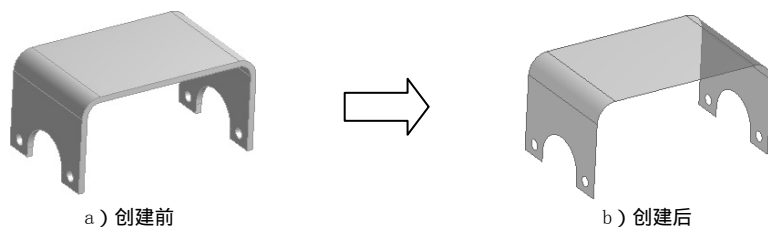
图 3.7.13 从面生成面体
