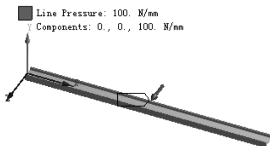
图 5.2.17 添加线压力载荷
