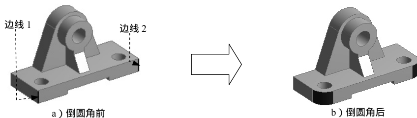
图 3.3.35 固定半径圆角
