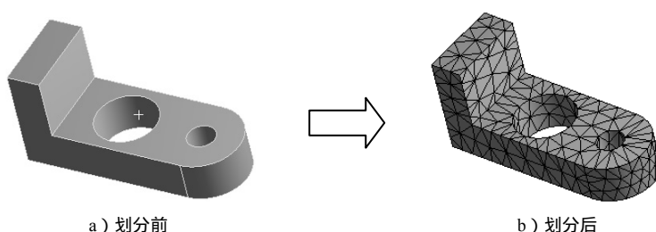
图 4.2.2 划分网格
