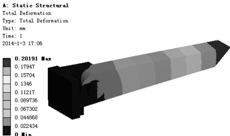
图 7.6.74 位移变形结果图解
