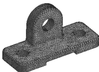
图 4.7.8 全局控制网格划分结果
