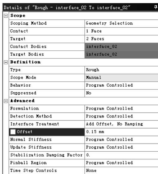
图 7.6.44 定义粗糙接触
