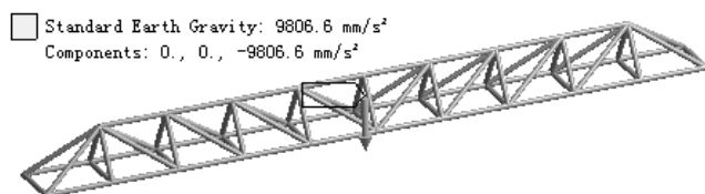
图 9.3.23 添加重力加速度
