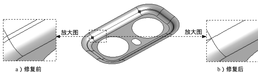
图 3.5.27 修复缝隙
