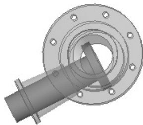
图 3.13.34 布尔求差操作 2
