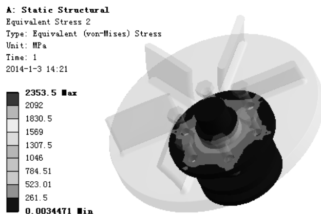
图 7.6.15 应力结果图解 (shaft)
