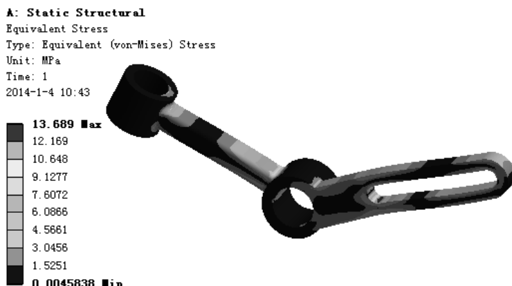
图 9.1.9 应力结果图解
