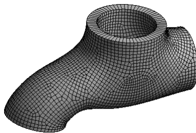
图 9.4.6 划分网格
