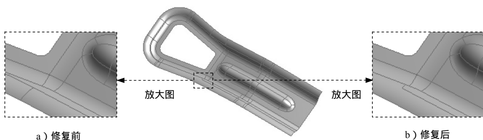
图 3.5.43 修复小边毛刺面
