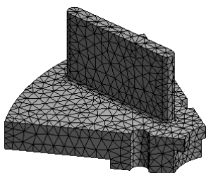
图 9.2.10 划分网格
