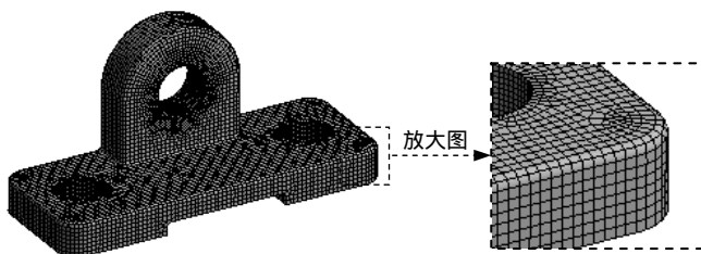
图 4.7.2 支架网格划分
