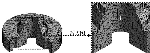
图 4.3.40 匹配控制
