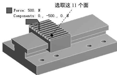
图 7.6.26 添加载荷力
