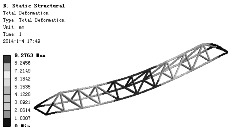
图 9.3.24 位移变形结果图解
