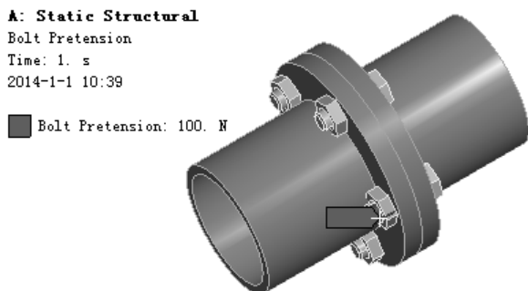
图 5.2.26 添加螺栓载荷
