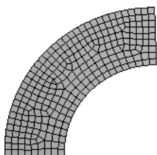
图 7.5.33 划分网格
