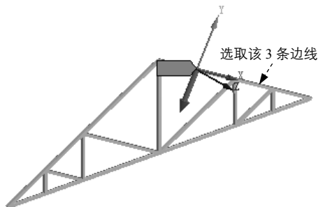
图 7.8.12 添加力载荷 2
