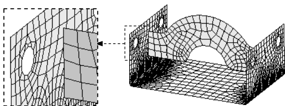
图 7.6.61 划分网格
