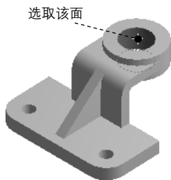
图 5.6.5 选取边界面对象（一）
