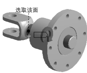
图 7.10.8 添加力矩约束
