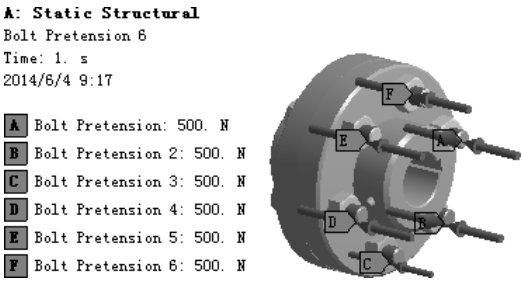
图 4.2.33 添加螺栓载荷
