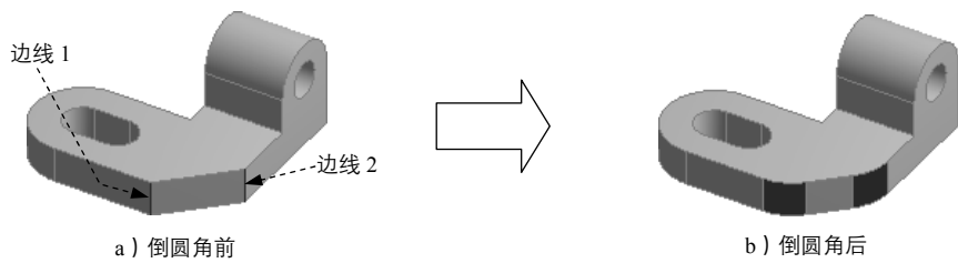
图 3.3.33 固定半径圆角
