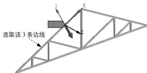
图 7.8.11 添加力载荷 1
