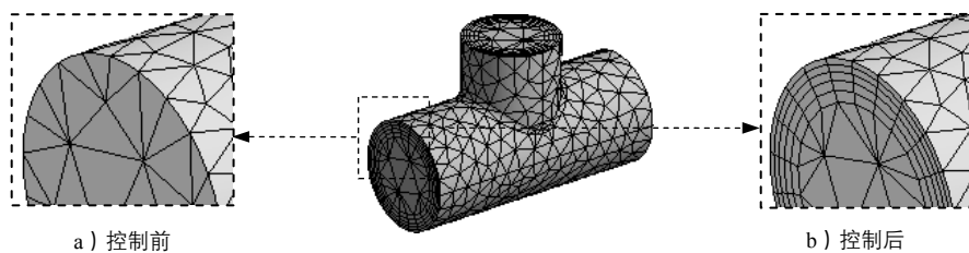
图 5.3.47 分层网格控制网格划分
