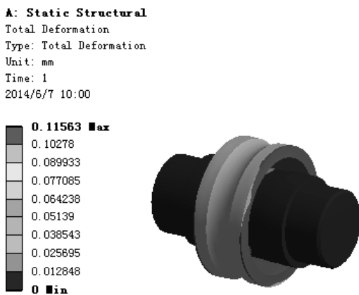
图 7.6.37 位移变形结果图解
