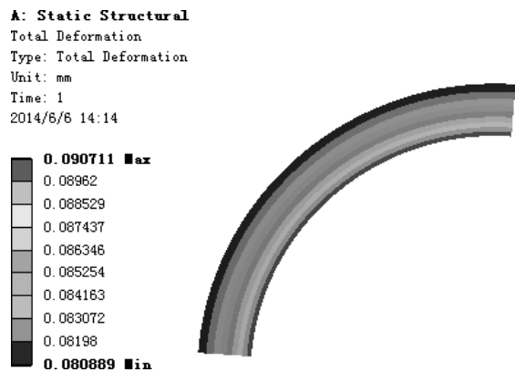
图 7.5.28 位移变形结果图解
