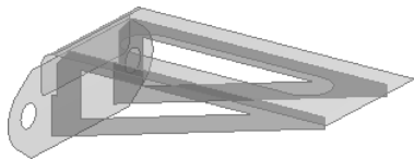
图 7.11.6 中面 3 和中面 4
