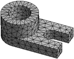
图 5.3.4 自动网格划分（不规则）
