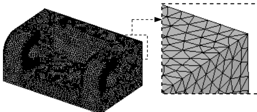
图 5.2.10 网格划分结果
