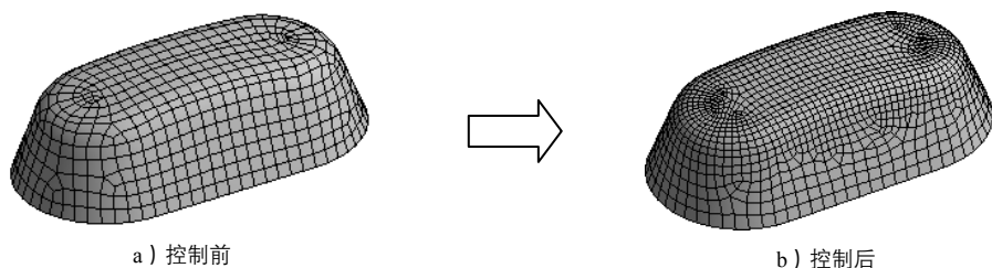
图 5.3.23 边界分段控制网格划分
