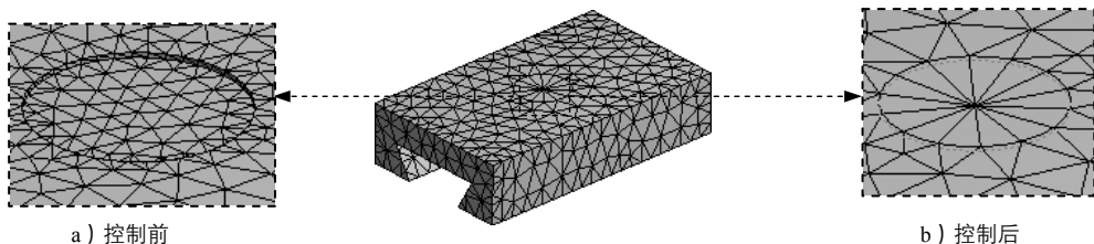
图 5.3.44 简化控制网格划分
