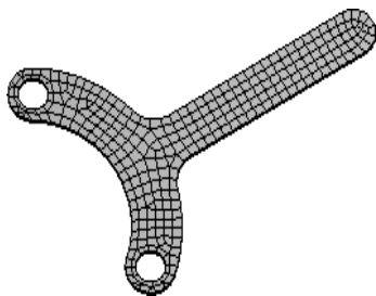
图 7.5.9 划分网格
