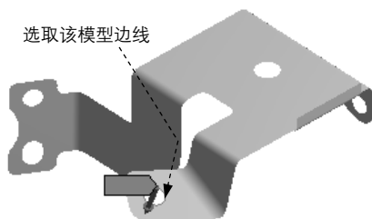
图 7.9.4 添加载荷力 1
