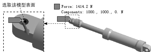
图 7.6.27 添加载荷力
