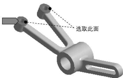
图 7.7.6 添加固定约束
