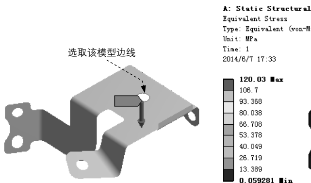
图 7.9.5 添加载荷力 2
