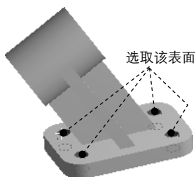
图 7.2.4 添加固定约束条件
