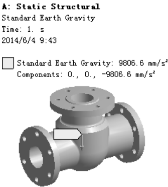
图 4.2.6 添加重力加速度条件
