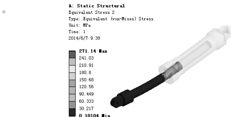
图 7.6.30 应力结果图解 (frictionless)
