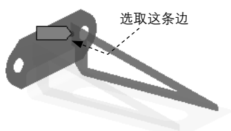
图 7.11.16 定义 Slave 几何对象
