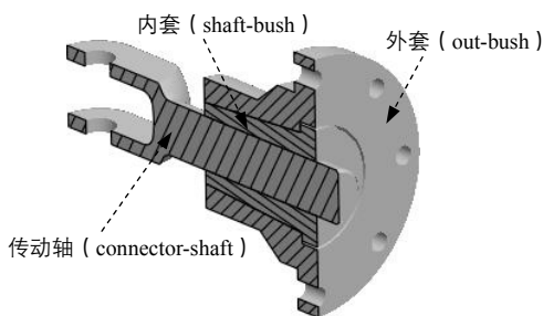
图 7.10.2 锥形胀套结构组成
