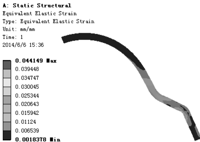
图 7.5.46 应变结果图解
