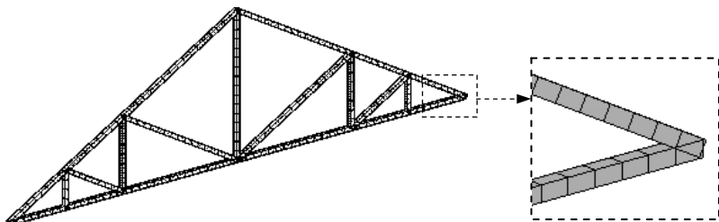
图 7.8.7 划分网格
