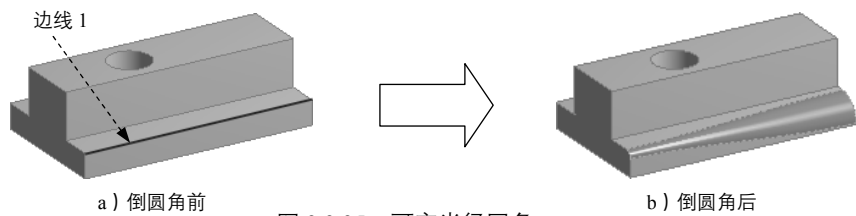
图 3.3.35 可变半径圆角
