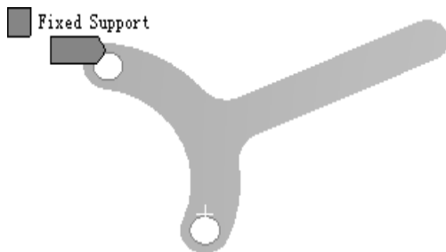
图 7.5.13 添加固定约束条件
