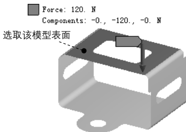
图 7.6.57 添加载荷力
