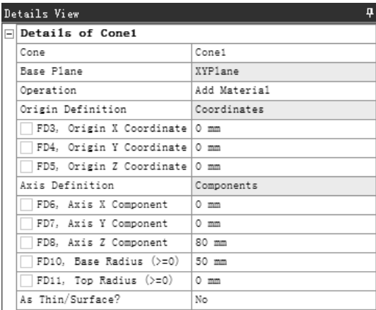
图 3.3.8 “Details View” 对话框
