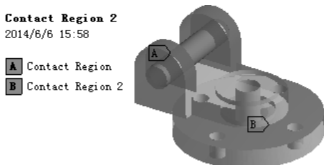
图 7.6.4 接触区域
