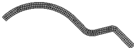
图 7.5.41 划分网格
