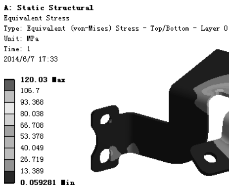
图 7.9.6 查看应力结果图解
