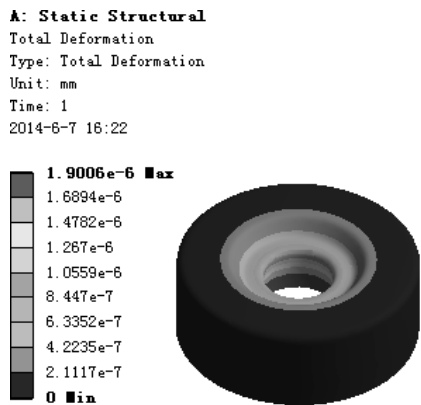
图 7.4.8 位移变形结果图解
