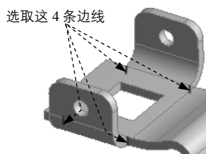
图 3.10.22 定义倒圆角边线
