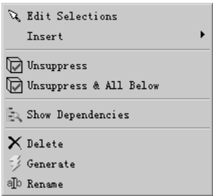
图 3.3.25 快捷菜单
