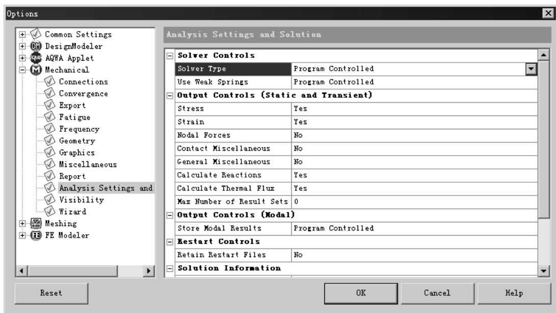
图 6.1.1 “Options”对话框
