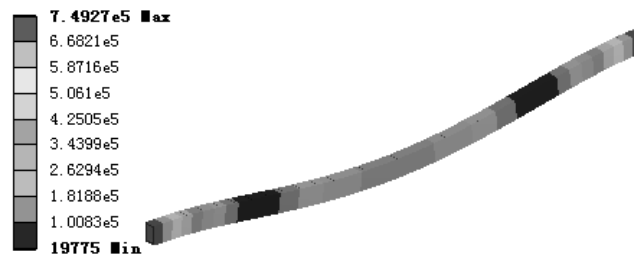
图 7.3.10 弯矩变形结果图解
