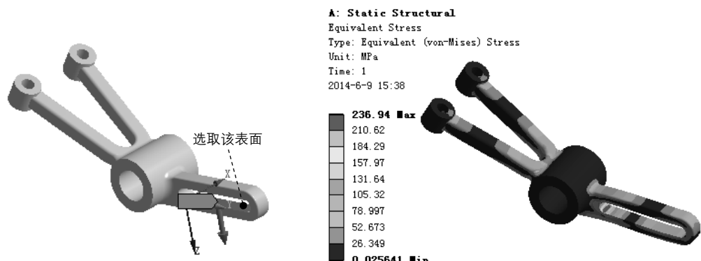
图 7.7.7 添加力载荷
