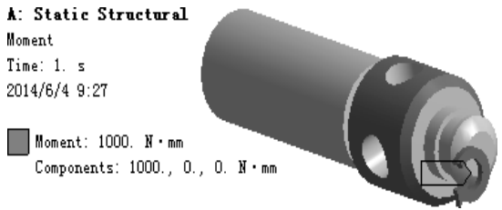
图 4.2.22 添加力矩载荷
