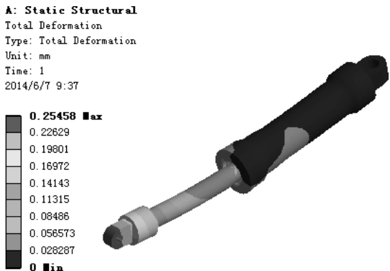
图 7.6.29 位移变形结果图解
