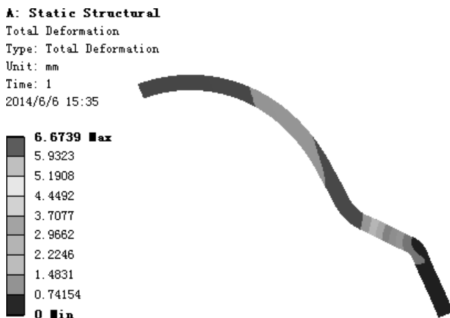
图 7.5.45 位移变形结果图解
