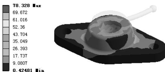
图 7.6.48 应力结果图解 (base-down)
