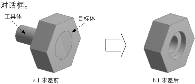
图 3.4.22 布尔求差操作
