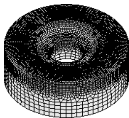
图 7.4.4 划分网格
