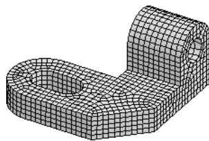
图 5.3.10 六面体网格划分结果
