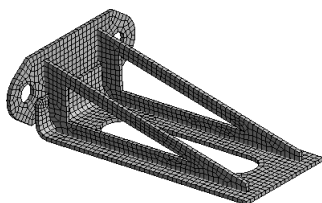
图 7.11.17 网格划分
