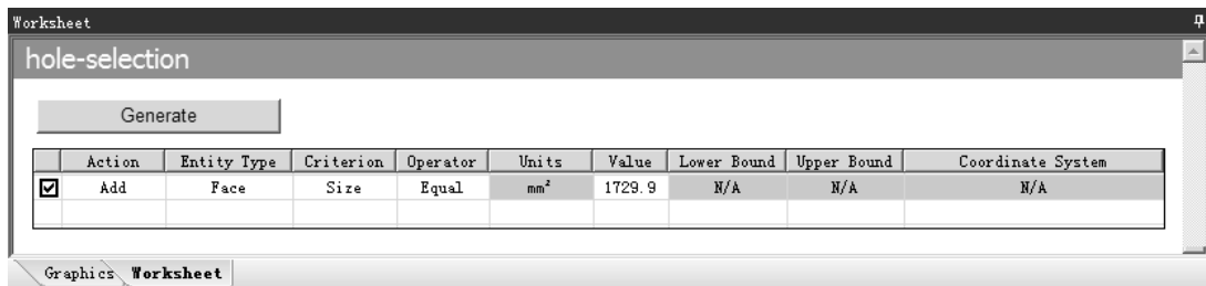
图 2.6.14 “Worksheet”窗口
