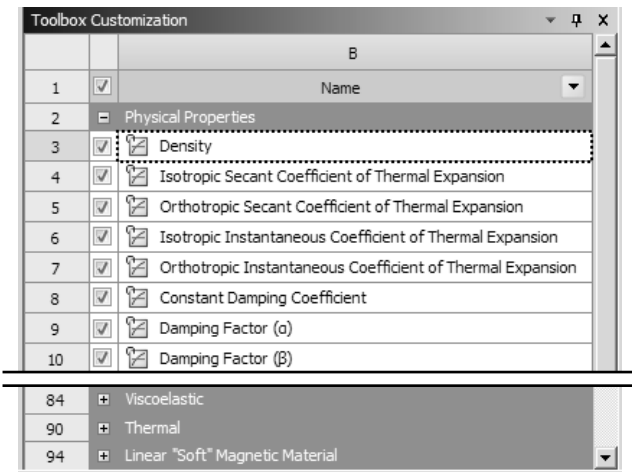
图 2.2.3 用户工具箱
