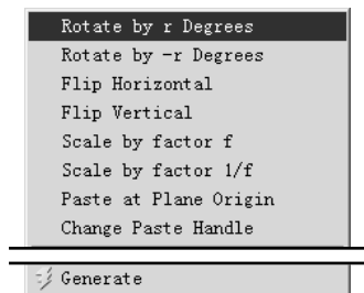
图 3.2.37 快捷菜单（二）
