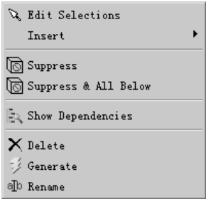
图 3.3.23 快捷菜单
