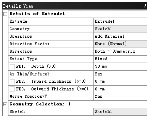
图 3.1.9 详细列表
