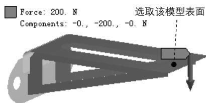
图 7.11.19 添加载荷力
