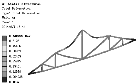
图 7.8.14 位移变形结果图解
