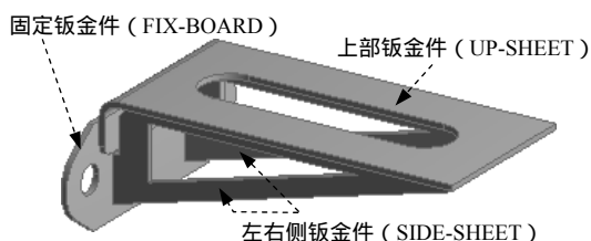
图 7.11.1 钣金组件结构分析
