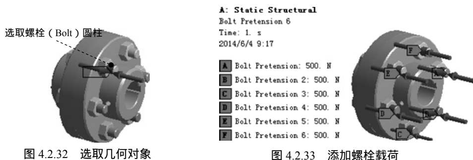
图 4.2.33 添加螺栓载荷
