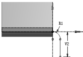
图 3.10.6 草图 2
