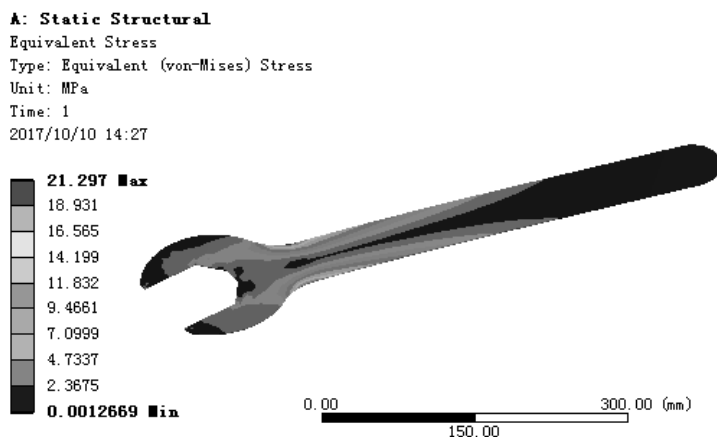
图 7.5.23 应力结果图解
