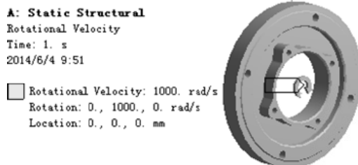
图 4.2.8 添加旋转速度条件
