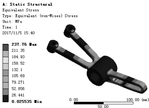
图 7.7.8 应力结果图解
