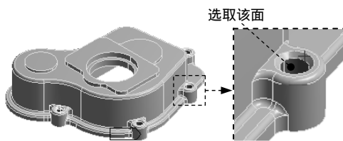
图 2.6.19 选取曲面 (四)
