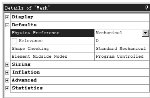
图 5.2.4 “Details of ‘Mesh’”对话框（一）
