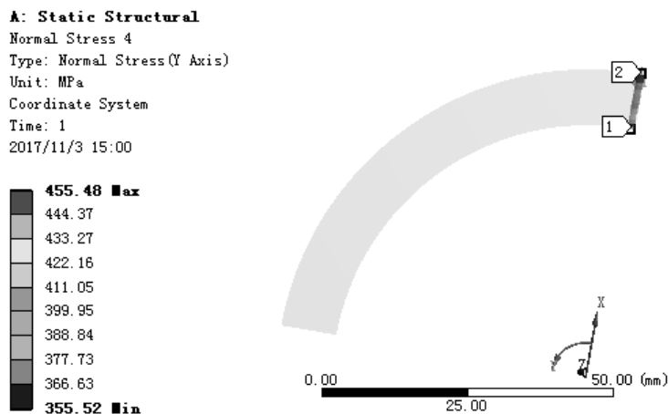
图 7.5.41 切向应力 (路径 Path) 结果图解
