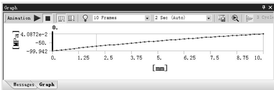
图 7.5.40 径向应力 (路径 Path) 图表
