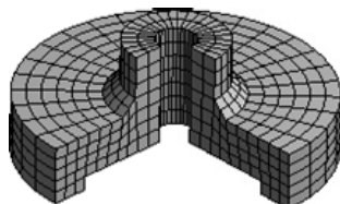
图 5.3.41 匹配控制网格划分
