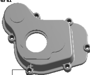
图 2.6.23 添加固定约束 (二)
