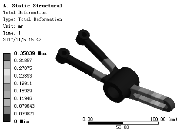
图 7.7.9 位移变形结果图解
