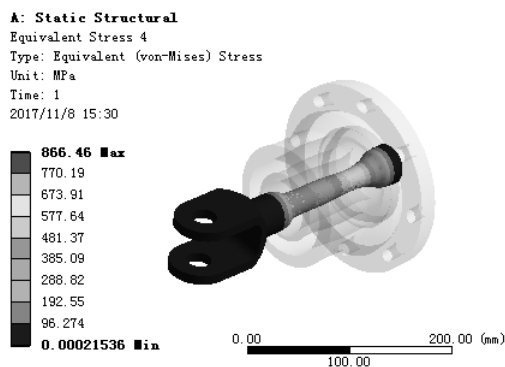
图 7.10.13 应力结果图解 (connector-shaft)
