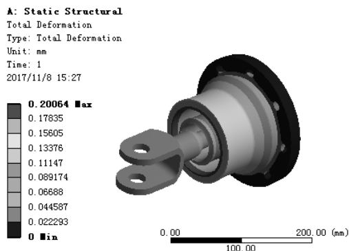
图 7.10.10 位移变形结果图解
