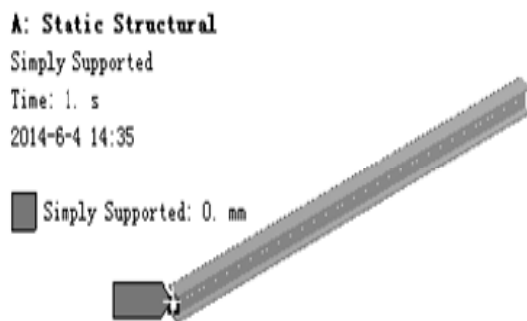
图 4.1.22 定义简支约束
