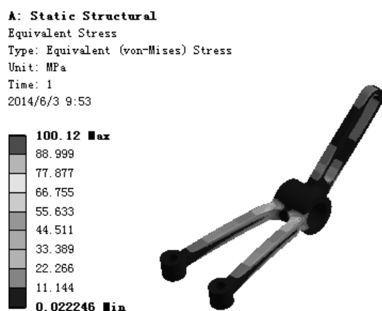
图 6.2.9 等效应力结果图解
