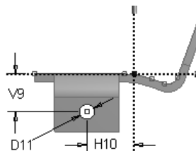
图 3.10.18 草图 5
