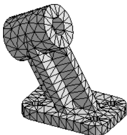
图 7.2.2 初步划分网格
