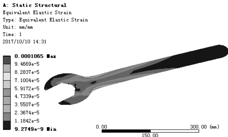
图 7.5.25 应变结果图解
