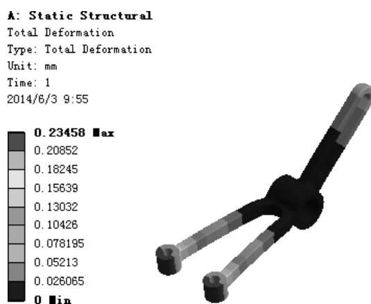
图 6.2.10 总位移变形结果图解
