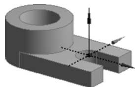
图 3.2.10 从坐标系创建平面
