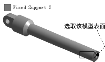
图 7.6.26 添加固定约束 2
