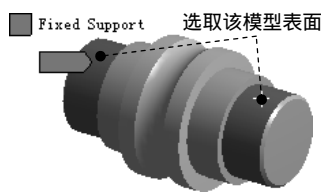
图 7.6.34 添加固定约束
