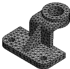
图 5.6.4 全局控制网格划分
