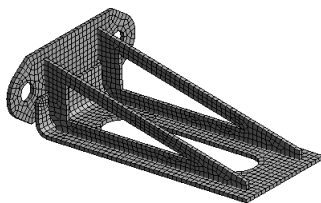
图 7.11.17 网格划分
