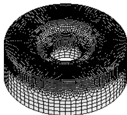
图 7.4.4 划分网格
