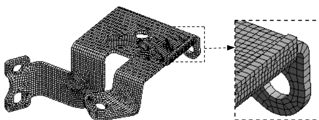
图 7.9.3 网格划分结果
