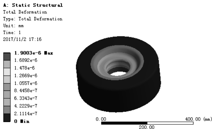
图 7.4.8 位移变形结果图解
