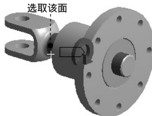
图 7.10.8 添加力矩约束
