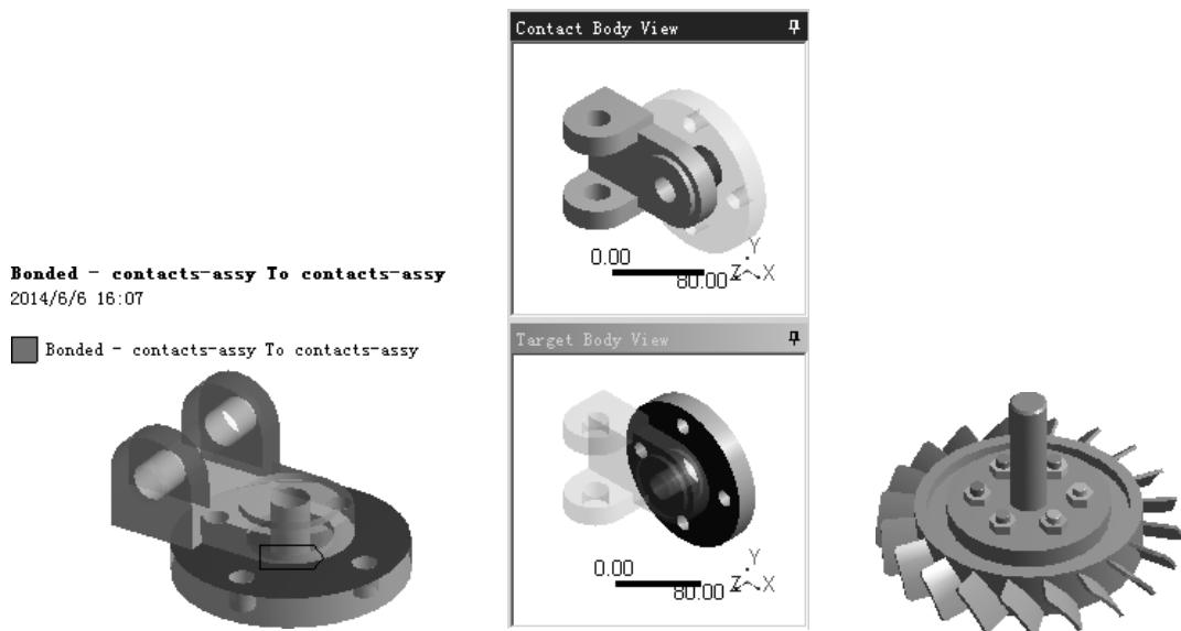
图 7.6.7 显示接触
