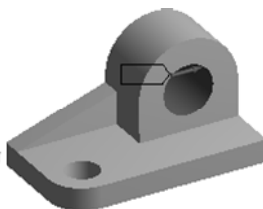
图 4.2.30 添加轴承载荷
