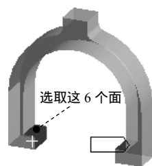
图 7.6.18 定义目标面
