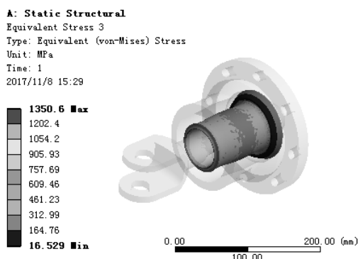
图 7.10.12 应力结果图解 (shaft-bush)
