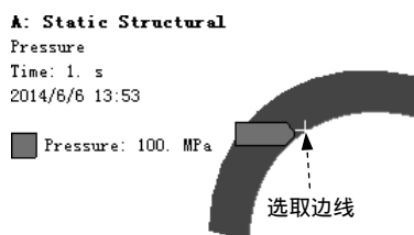
图 7.5.34 添加压力载荷
