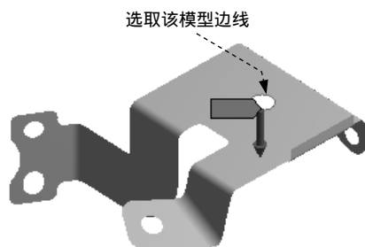
图 7.9.5 添加载荷力 2
