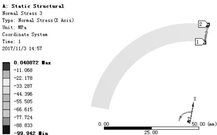
图 7.5.39 径向应力（路径 Path）结果图解
