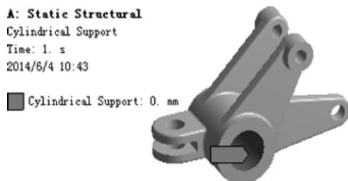
图 4.1.19 定义圆柱面约束
