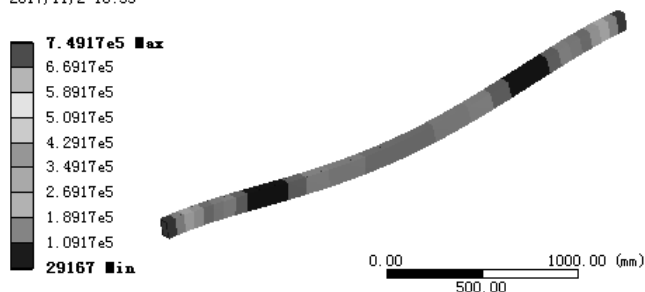
图 7.3.10 弯矩变形结果图解
