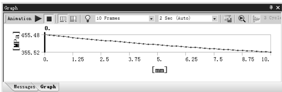
图 7.5.42 切向应力 (路径 Path) 图表
