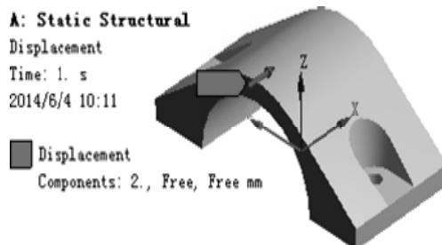
图 4.1.7 定义强迫位移
