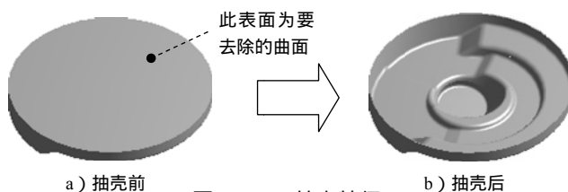
图 3.3.41 抽壳特征
