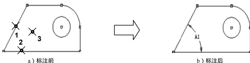
图 3.2.51 标注角度
