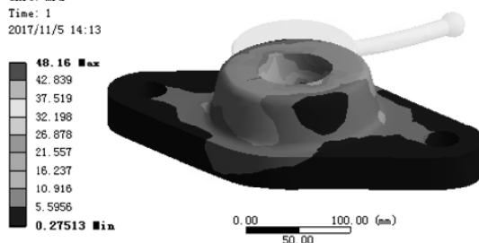
图 7.6.48 应力结果图解 (base-down)
