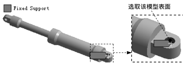
图 7.6.25 添加固定约束 1
