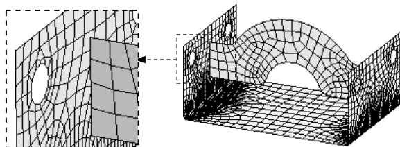
图 7.6.61 划分网格
