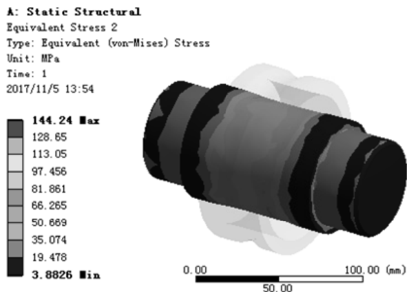
图 7.6.38 应力结果图解 (几何体 1)
