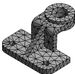
图 5.6.3 初步网格划分
