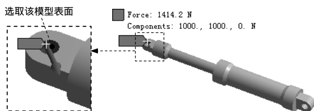
图 7.6.27 添加载荷力
