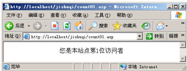
图 4-17 网页计数器
