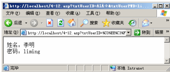
图 4-9 读取数据
