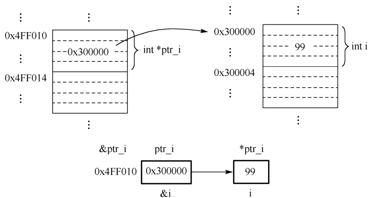
图 6-4 运算符 & 与 * 关系示意图
