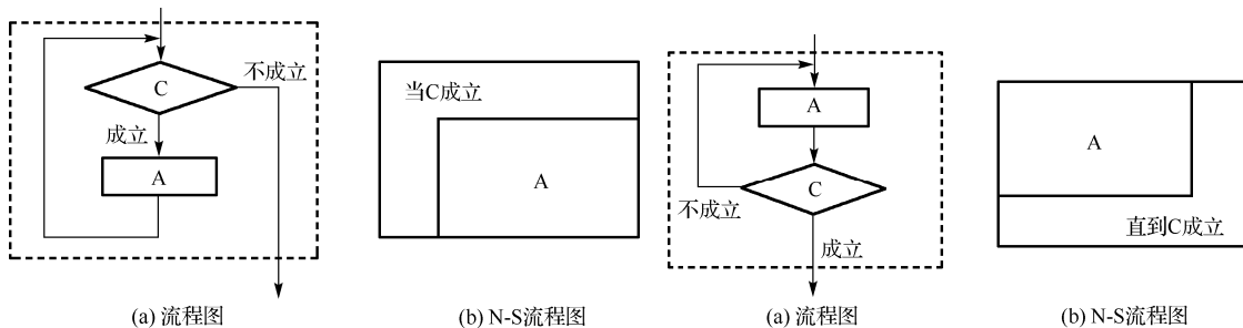
图 1-8 当型循环结构
