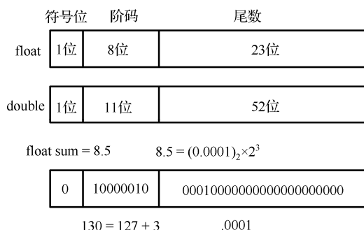
图 2-2 浮点数表示法
