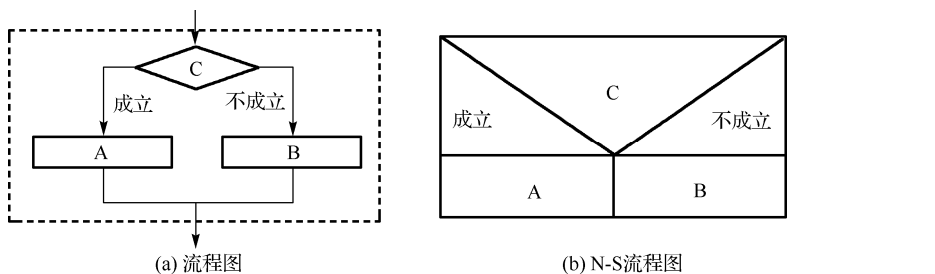
图 1-7 选择结构
