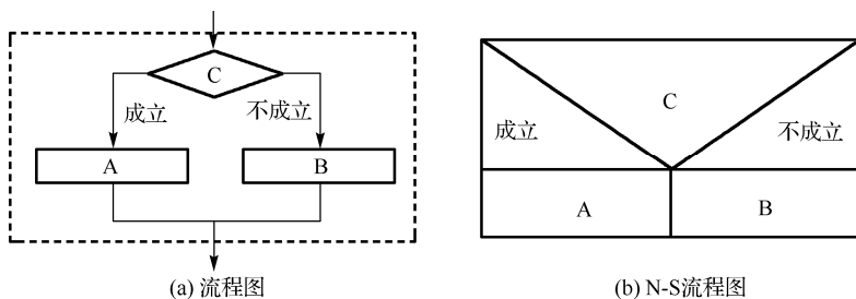
图 1-7 选择结构
