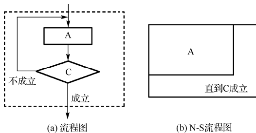
图 1-9 直到型循环结构
