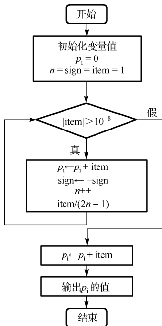
图 4-11 计算 \pi 的流程图
