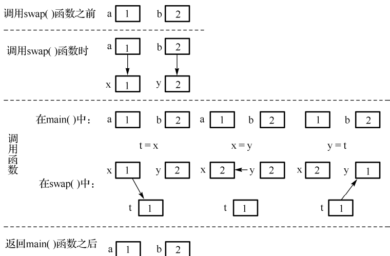
图 7-5 值传递示意图
