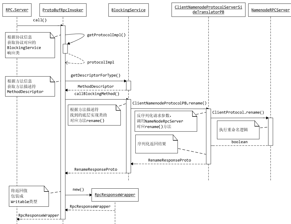
图 2-8 客户端响应 rename 请求流程
