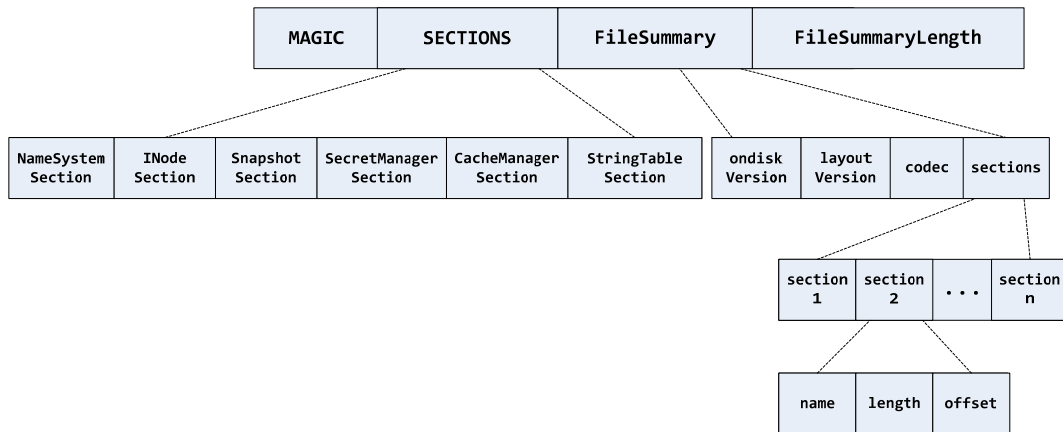
图 3-27 fsimage 文件格式
