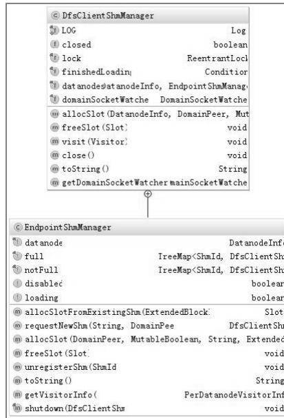
图 5-24 DfsClientShmManager 类结构
