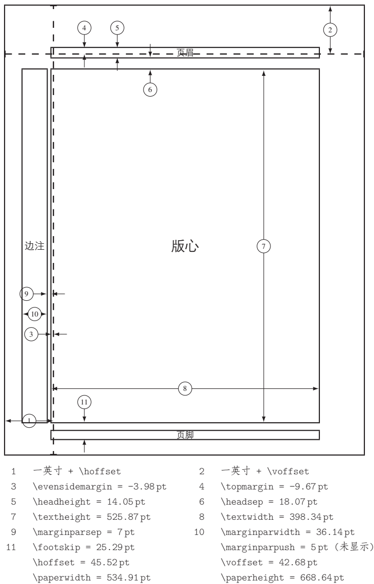
图 2.4 本书的页面尺寸设置示意图（偶数页）
