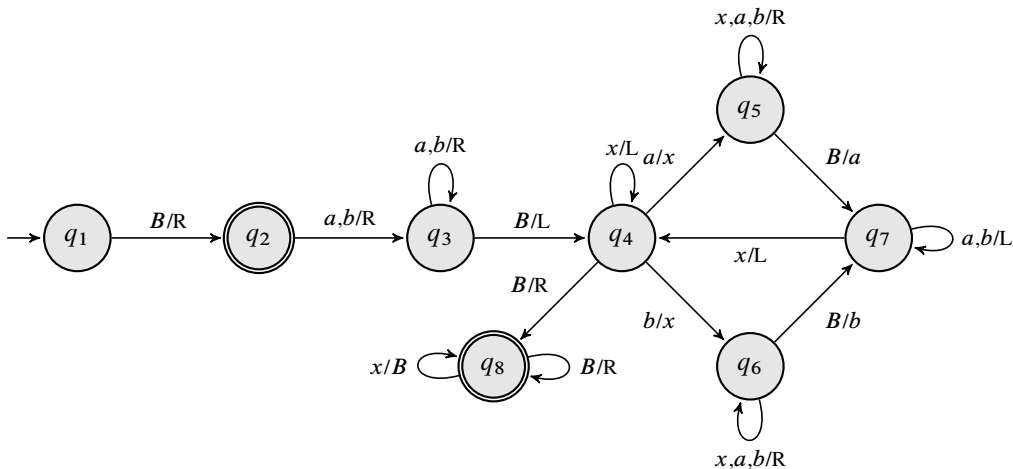
流程图 5.1 求逆字符串的图灵机
