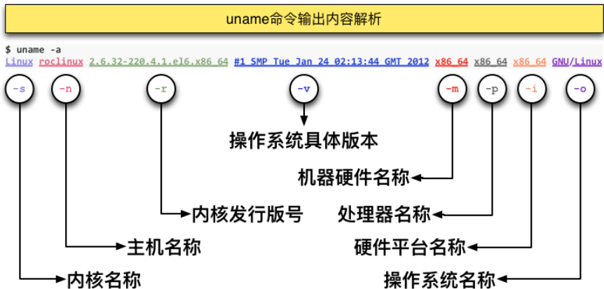
图 20 uname 命令输出内容解析
