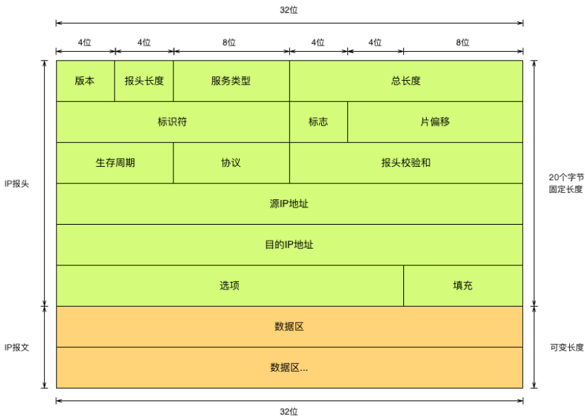
图 6 IP 协议头
