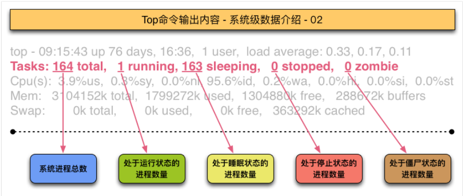
图 13 top 命令输出图（二）
