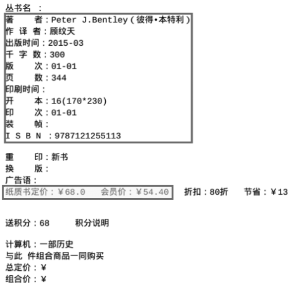
图 3-17 定价信息
