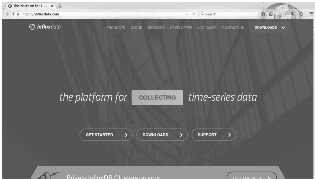
图 8-1 InfluxDB 首页
