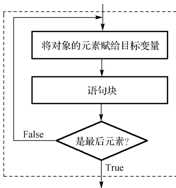
图 4-3 for 语句执行过程
