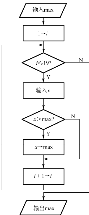
图 2-2 用传统流程图描述例 2-2 的算法
