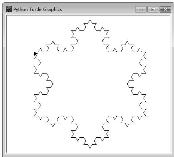
图 12-34 科赫雪花曲线
