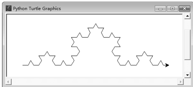
图 12-33 科赫曲线
