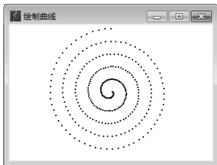
图 12-8 绘制曲线
