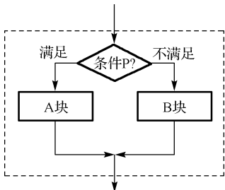
图 2-4 选择结构
