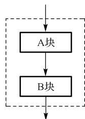
图 2-3 顺序结构
